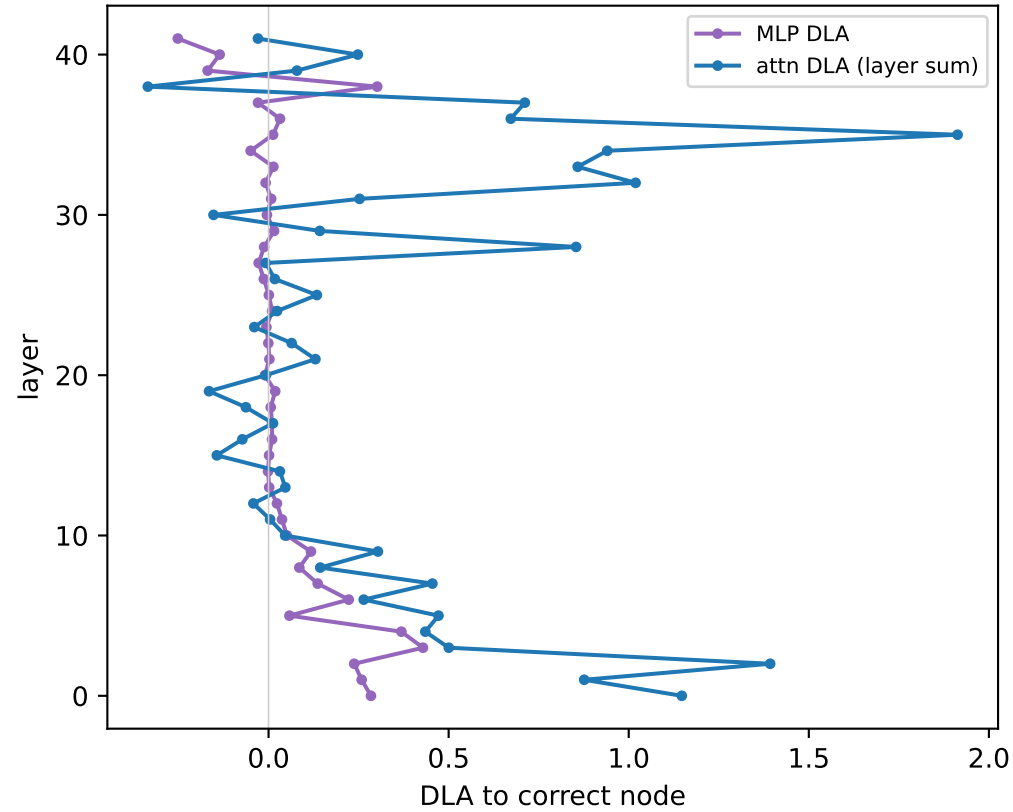
Gemma: per-layer attention vs MLP DLA
