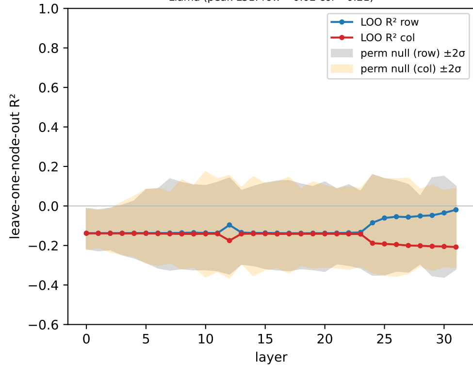
Llama (peak L31: row=-0.02 col=-0.21)
