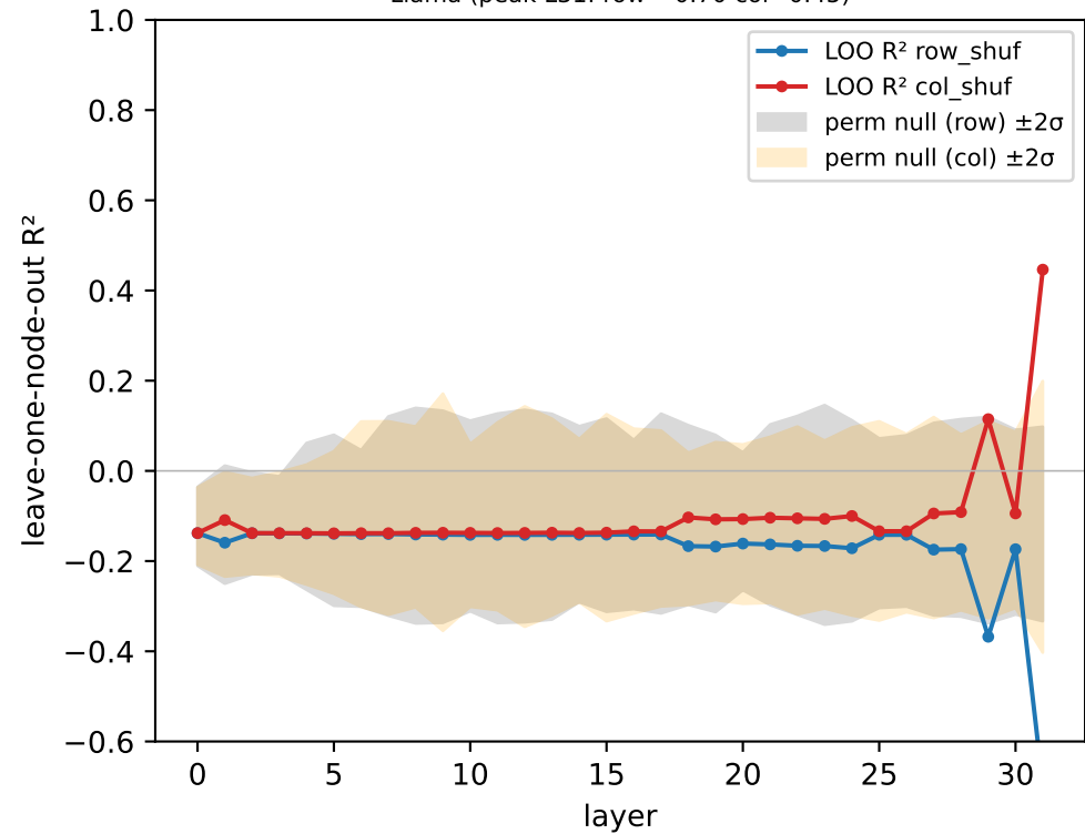
Llama (peak L31: row=-0.70 col=0.45)
