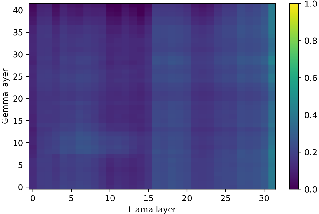
predict Llama from Gemma (max 0.44)
