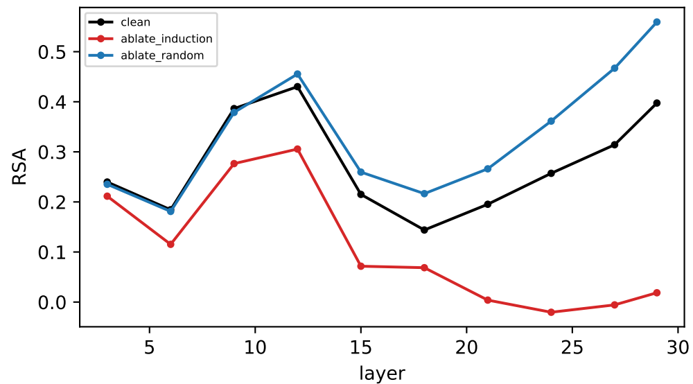
Gemma raw node-mean RSA
