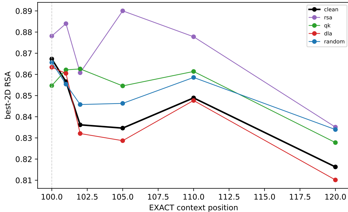
Llama [square_grid]
