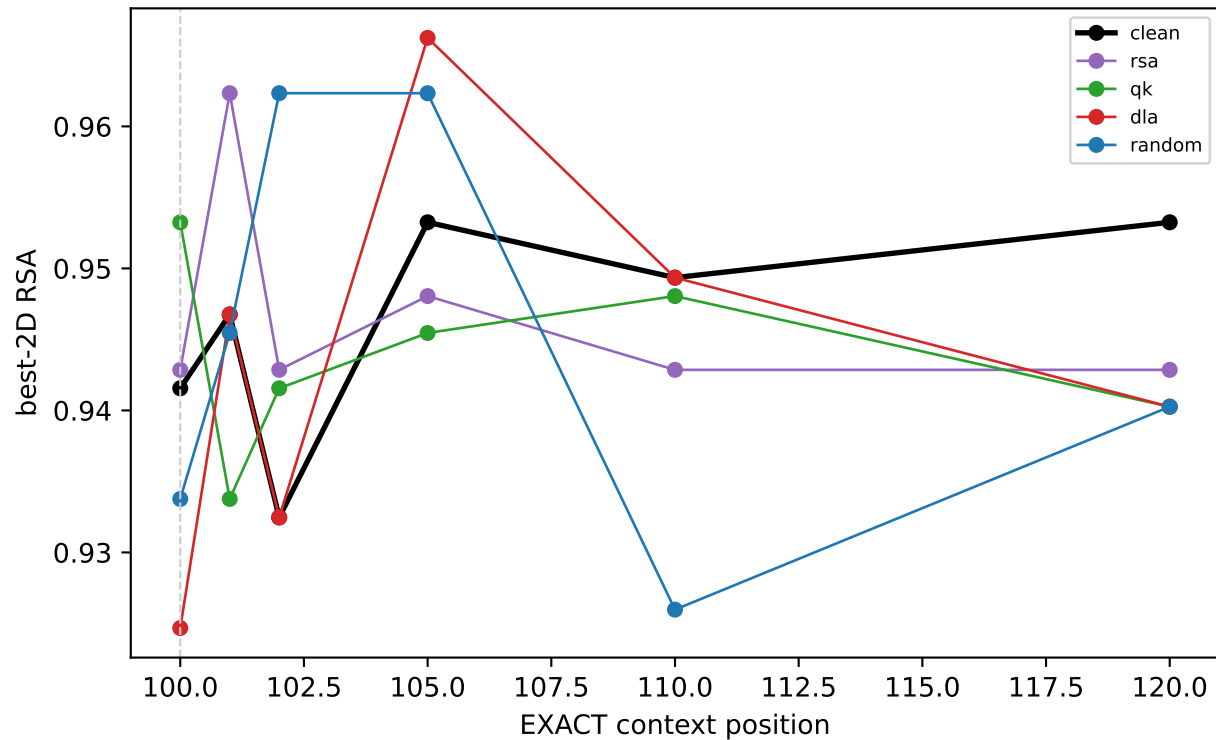
Llama [days]
