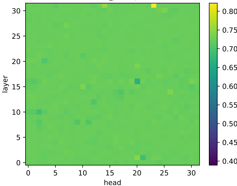
Llama: \Delta RSA (restoration)
