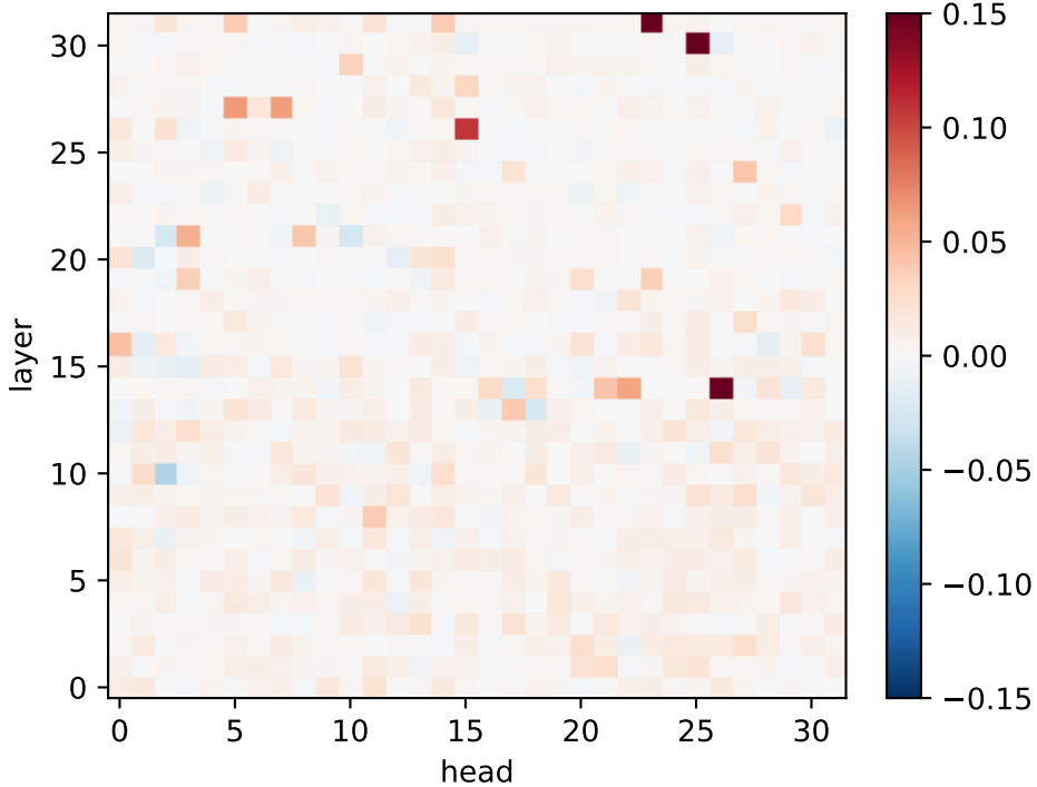
Llama: \Delta RSA (restoration)
