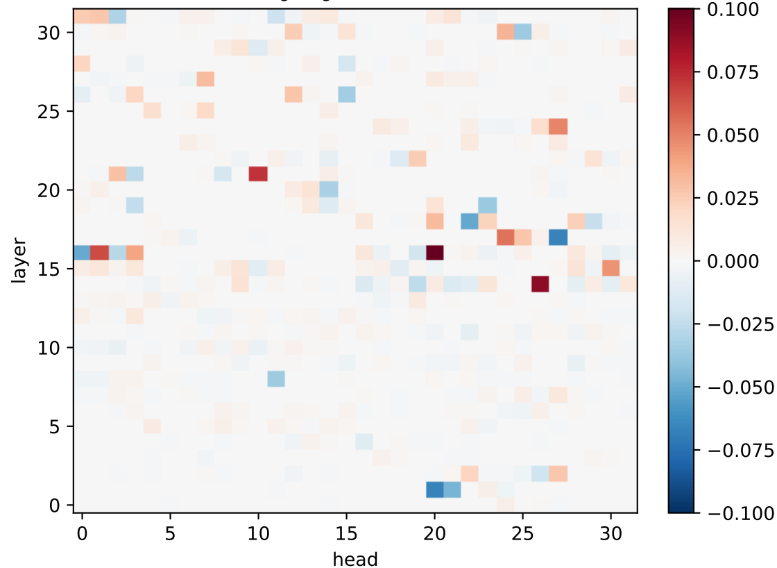
Llama: \Delta ring-neighbour mass (behaviour)
