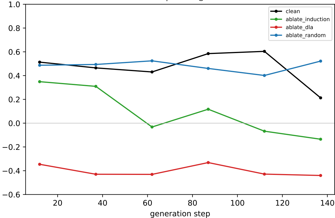
Llama coord-probe R 2 @ LAYER 31
