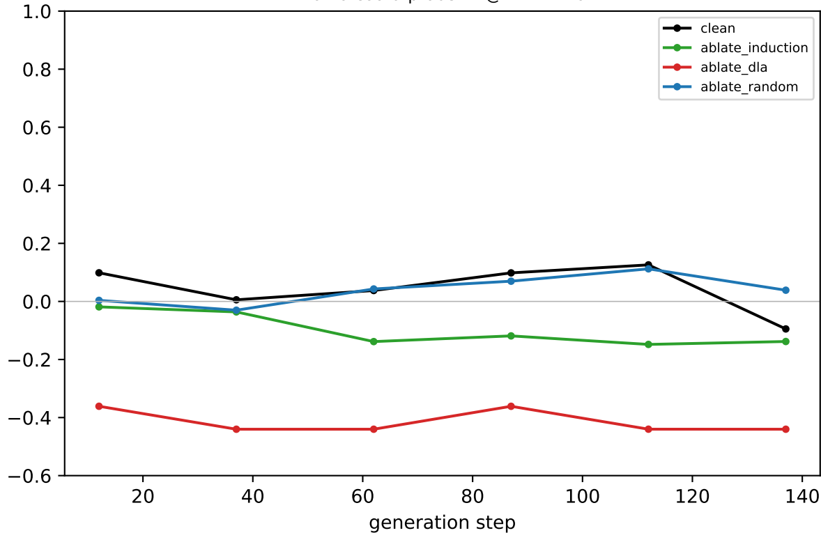
Llama coord-probe R^2 @ LAYER 20
