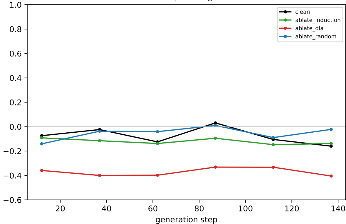
Llama coord-probe R^2 @ LAYER 5
