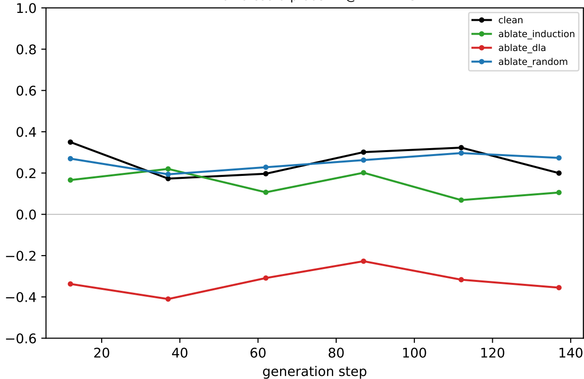
Llama coord-probe R^2 @ LAYER 13
