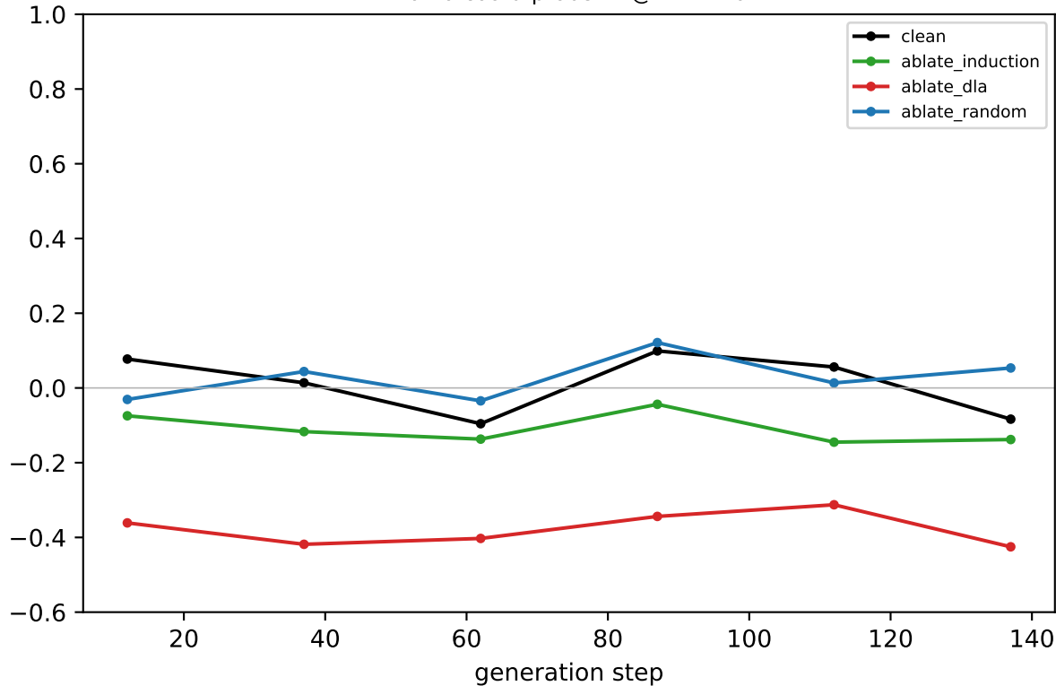
Llama coord-probe R 2 @ LAYER 6
