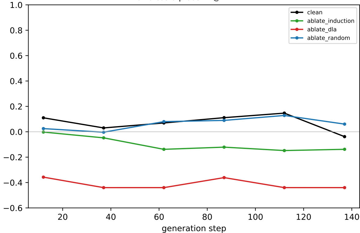
Llama coord-probe R 2 @ LAYER 21
