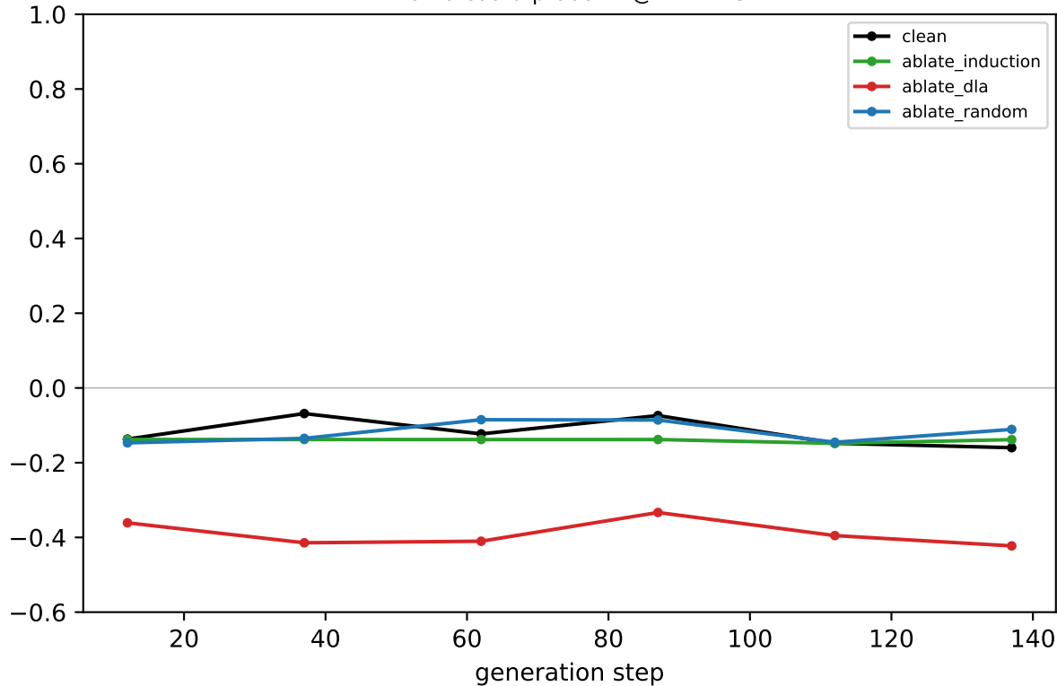
Llama coord-probe R 2 @ LAYER 3
