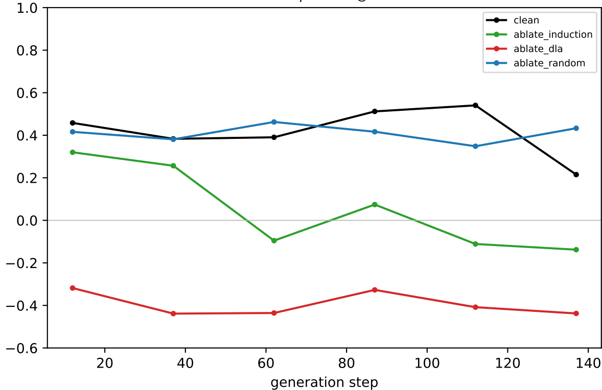
Llama coord-probe R 2 @ LAYER 29
