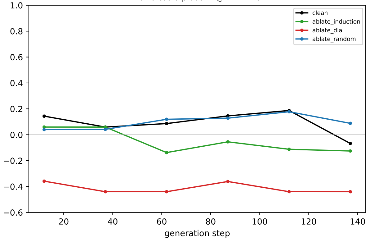
Llama coord-probe R 2 @ LAYER 19
