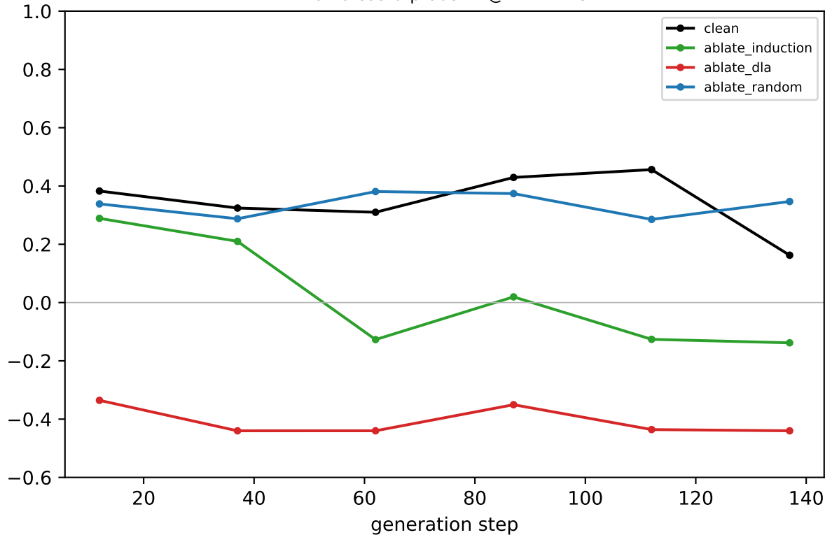
Llama coord-probe R 2 @ LAYER 25
