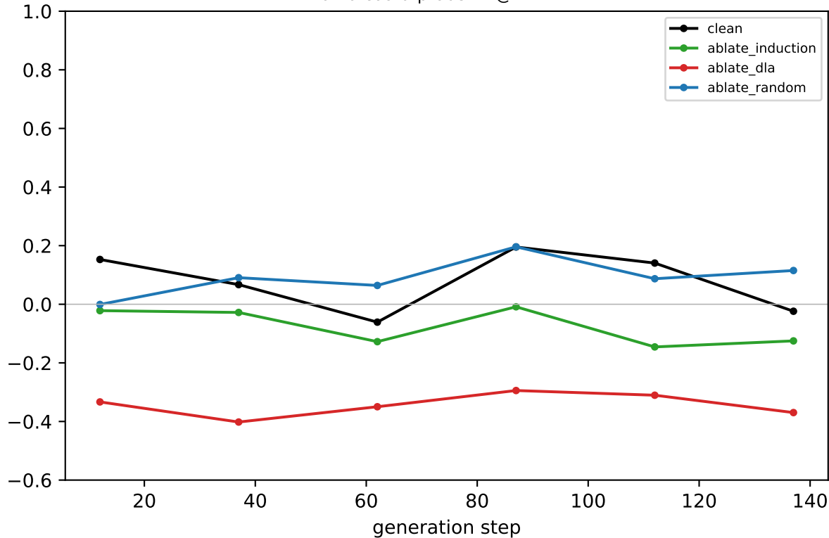
Llama coord-probe R 2 @ LAYER 7
