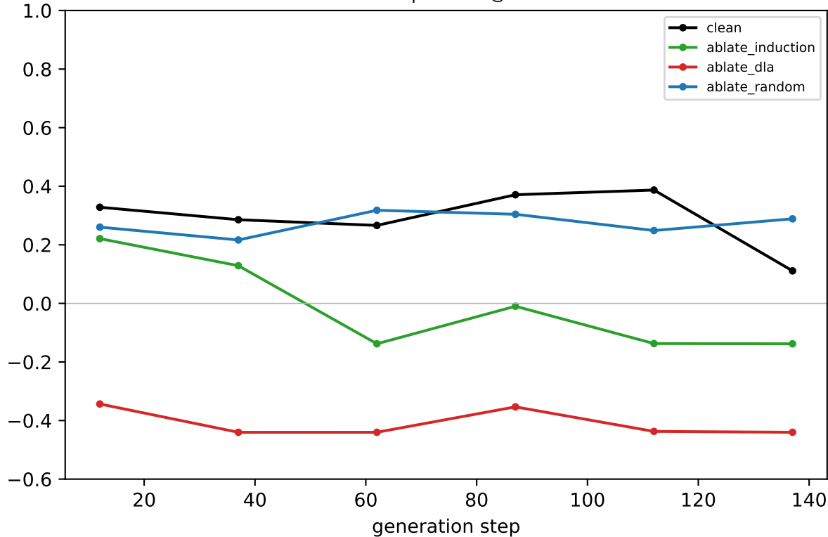
Llama coord-probe R^2 @ LAYER 24
