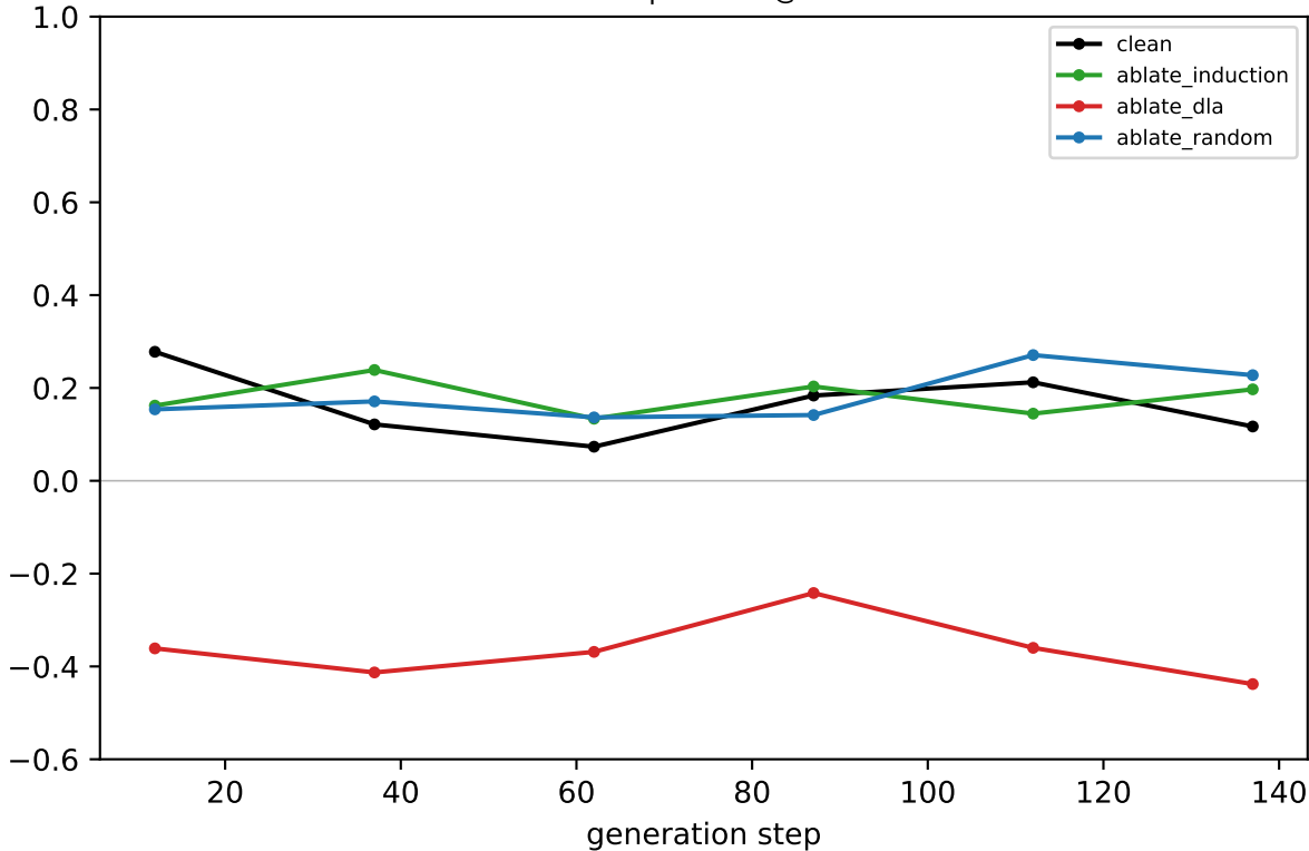
Llama coord-probe R^2 @ LAYER 11
