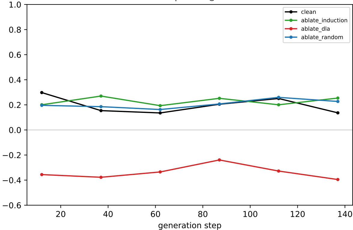
Llama coord-probe R^2 @ LAYER 10
