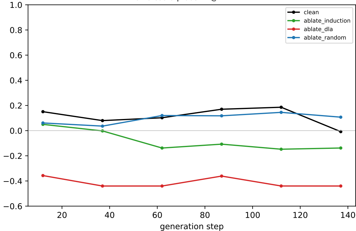
Llama coord-probe R^2 @ LAYER 22
