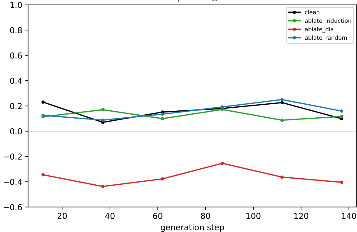
Llama coord-probe R 2 @ LAYER 14
