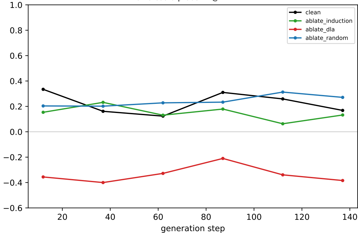
Llama coord-probe R^2 @ LAYER 12
