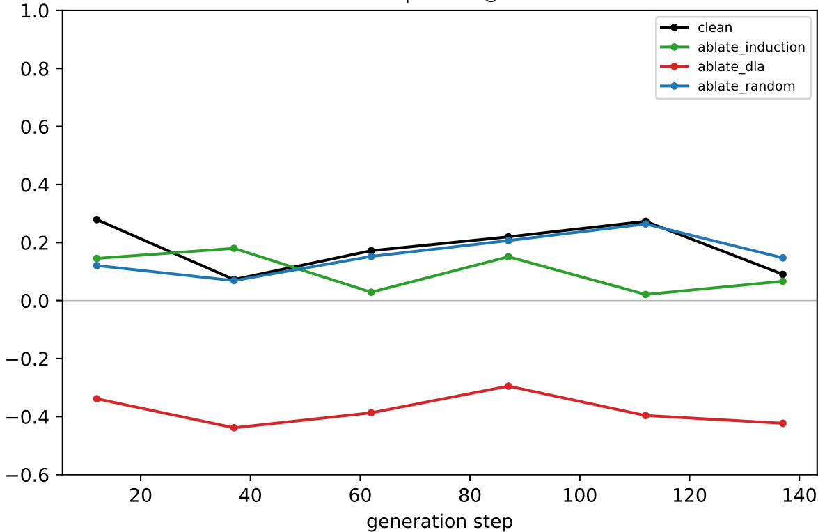
Llama coord-probe R 2 @ LAYER 15
