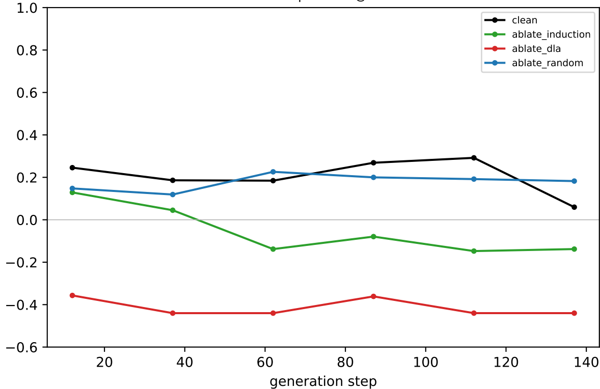
Llama coord-probe R^2 @ LAYER 23
