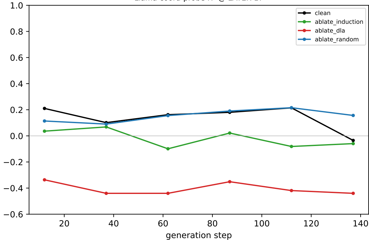
Llama coord-probe R^2 @ LAYER 17
