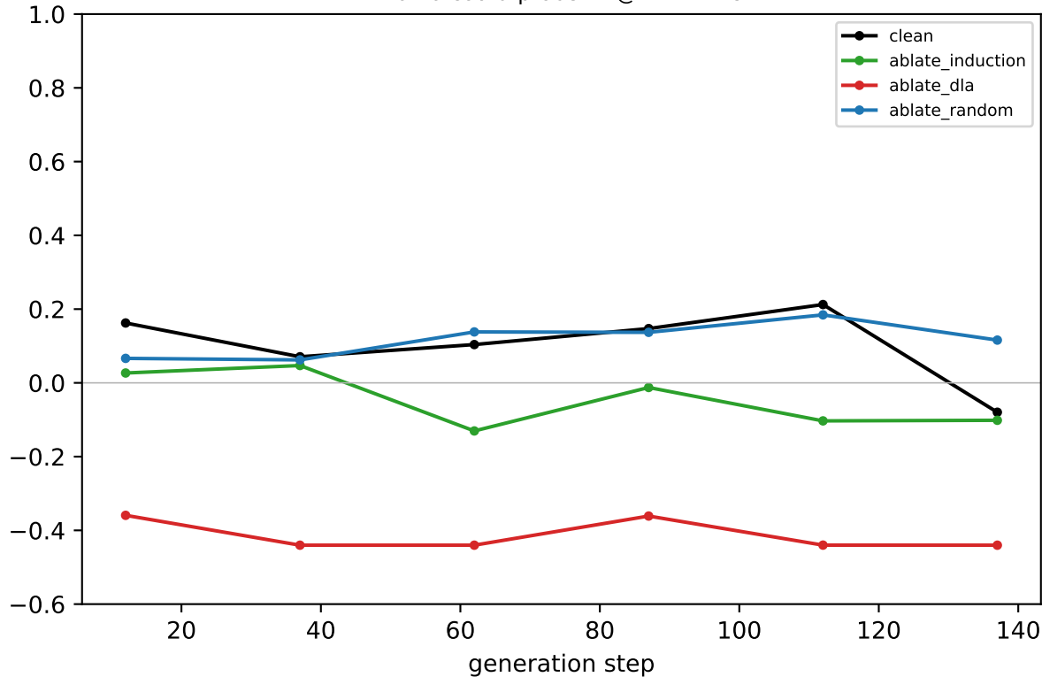
Llama coord-probe R 2 @ LAYER 18
