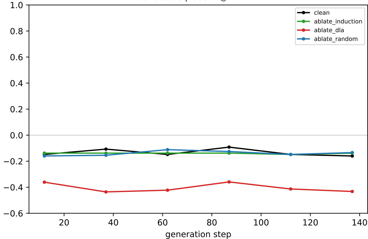
Llama coord-probe R^2 @ LAYER 2
