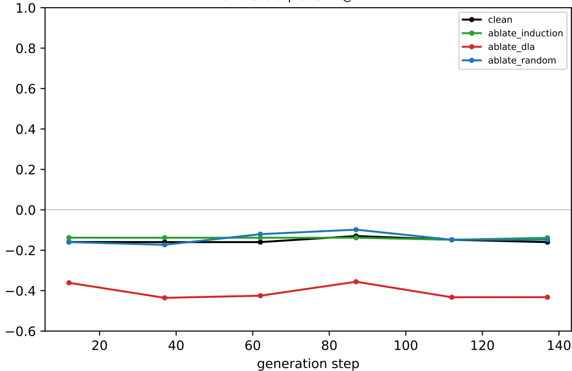
Llama coord-probe R 2 @ LAYER 1
