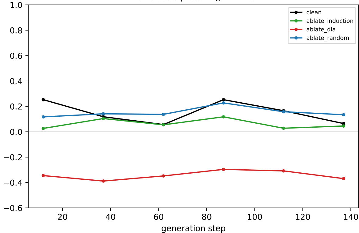
Llama coord-probe R 2 @ LAYER 8
