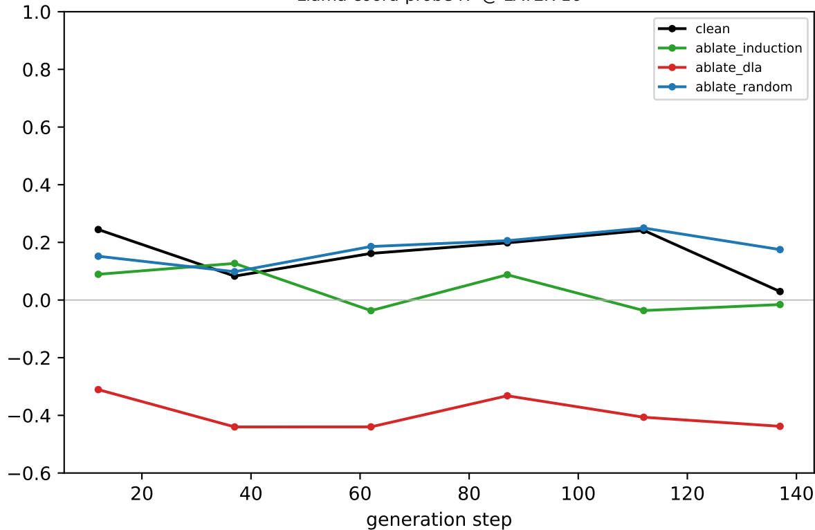
Llama coord-probe R 2 @ LAYER 16
