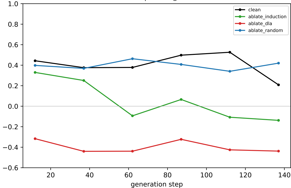
Llama coord-probe R 2 @ LAYER 28
