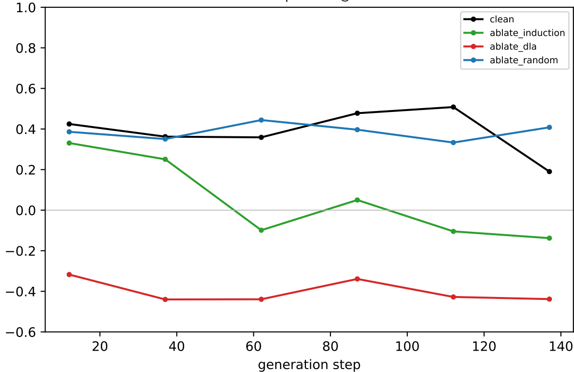
Llama coord-probe R^2 @ LAYER 27
