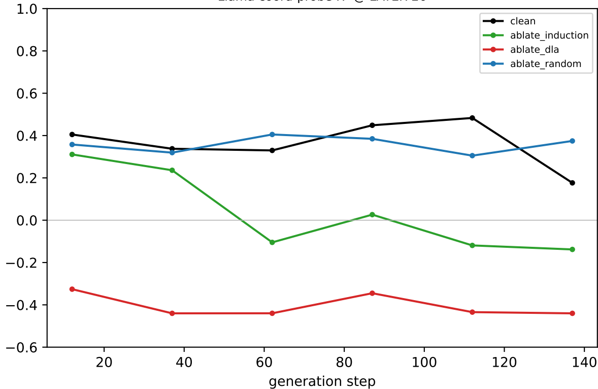
Llama coord-probe R 2 @ LAYER 26
