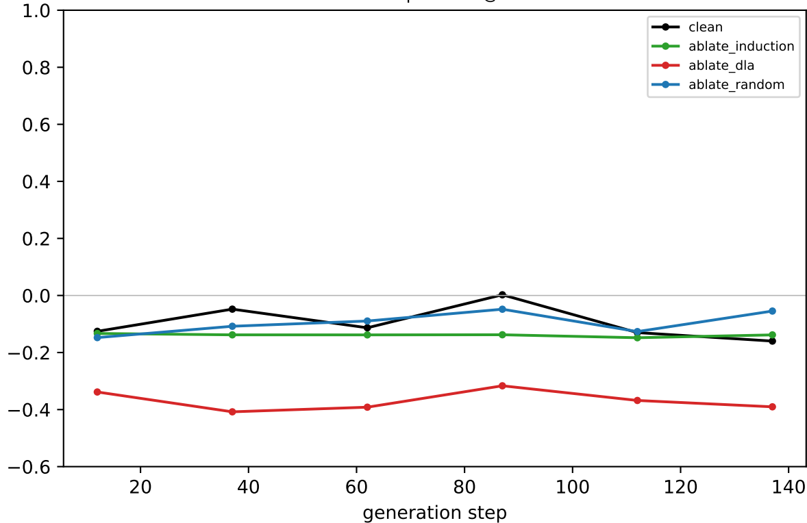
Llama coord-probe R 2 @ LAYER 4
