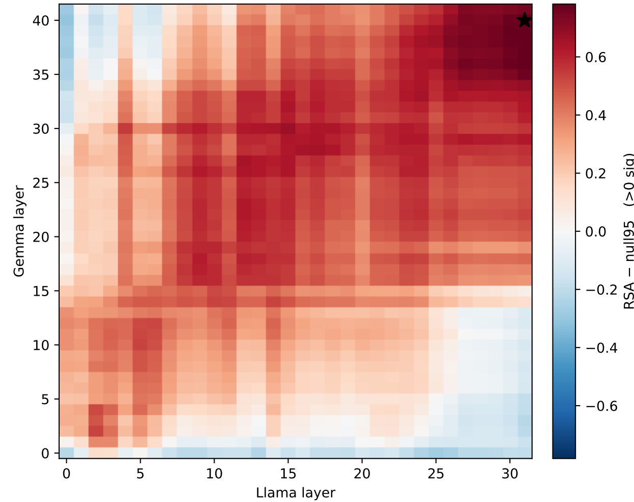
Gemma vs Llama (null95=0.16; 88% sig)
