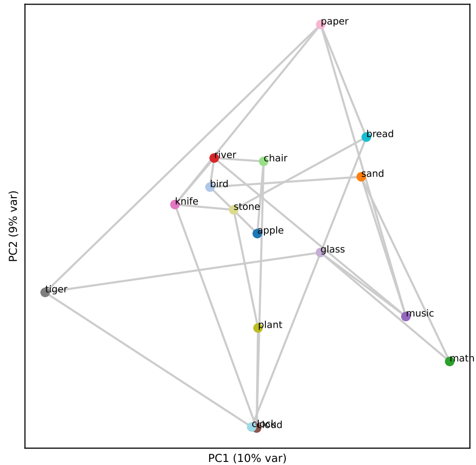
Qwen L8 (RSA 0.11)
