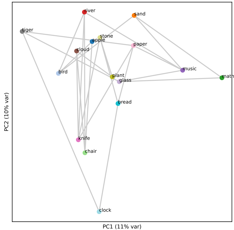
Gemma L8 (RSA 0.09)
