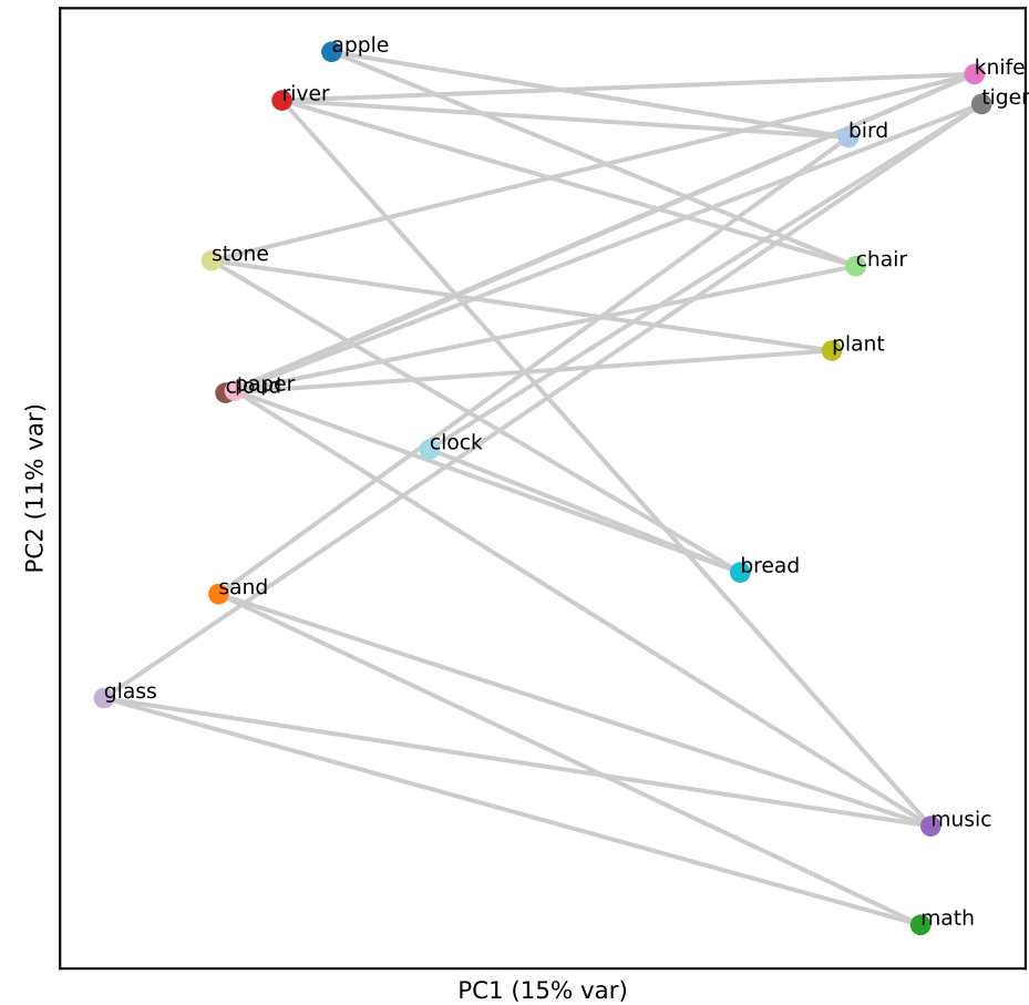
Qwen L20 (RSA -0.04)
