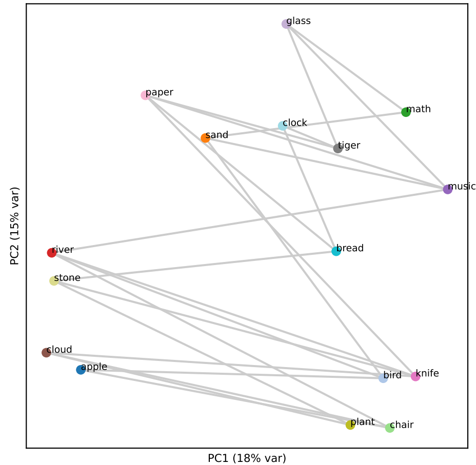
Gemma L35 (RSA 0.20)
