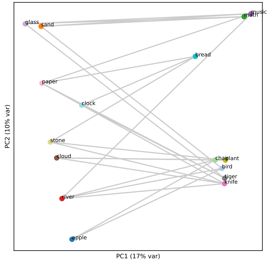
Qwen L23 (RSA -0.04)
