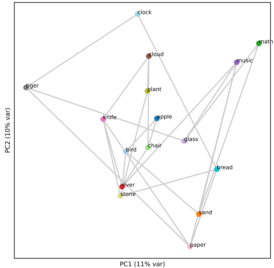
Qwen L9 (RSA 0.11)
