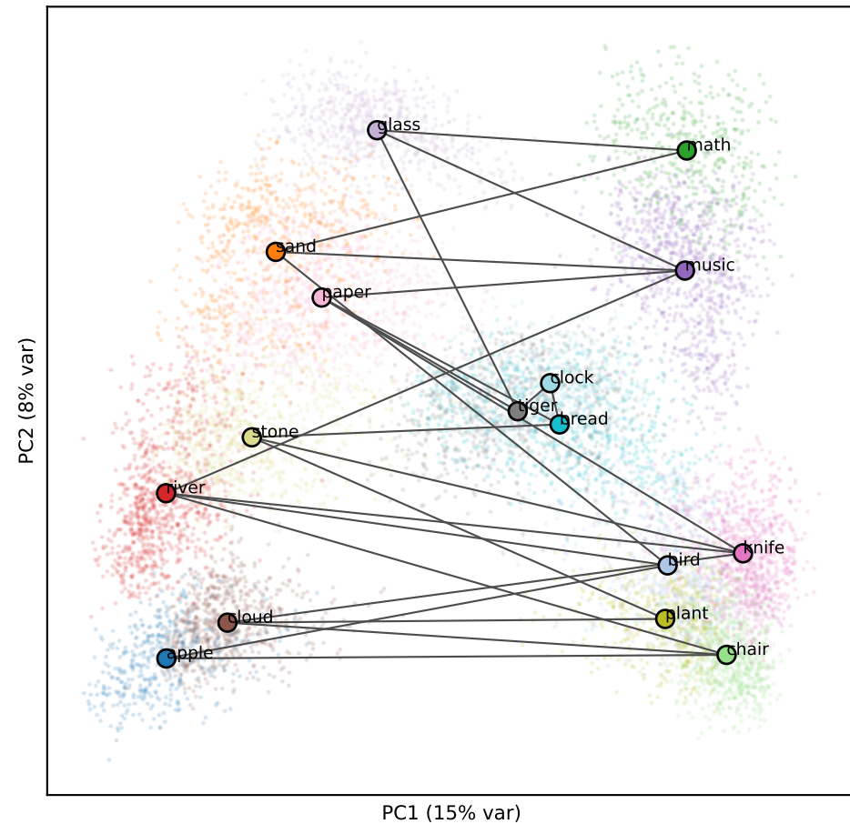
Llama L22 (RSA 0.11)
