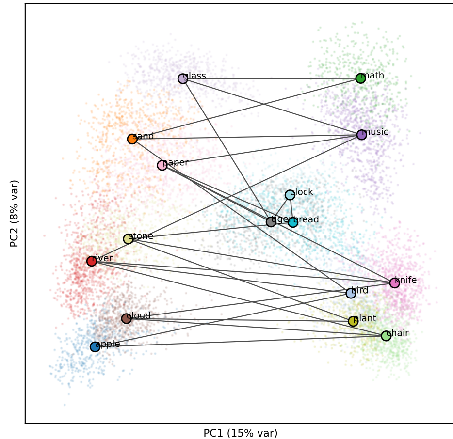
Llama L21 (RSA 0.11)
