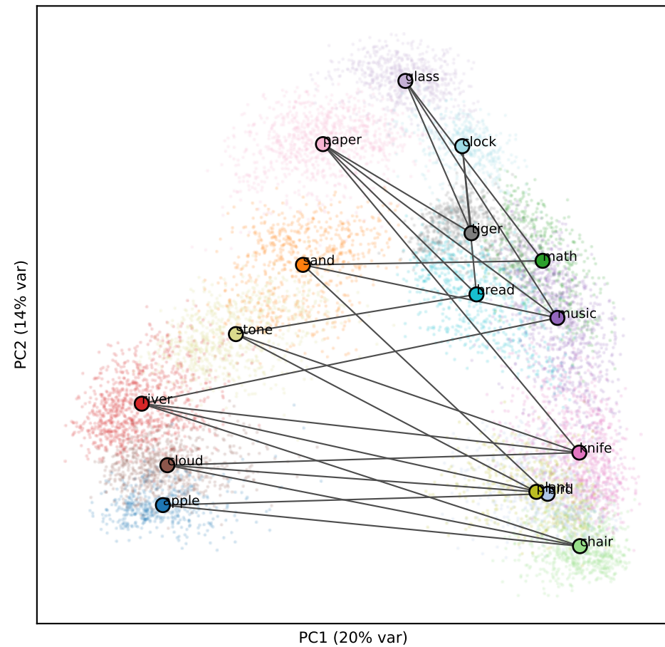
Llama L29 (RSA 0.15)
