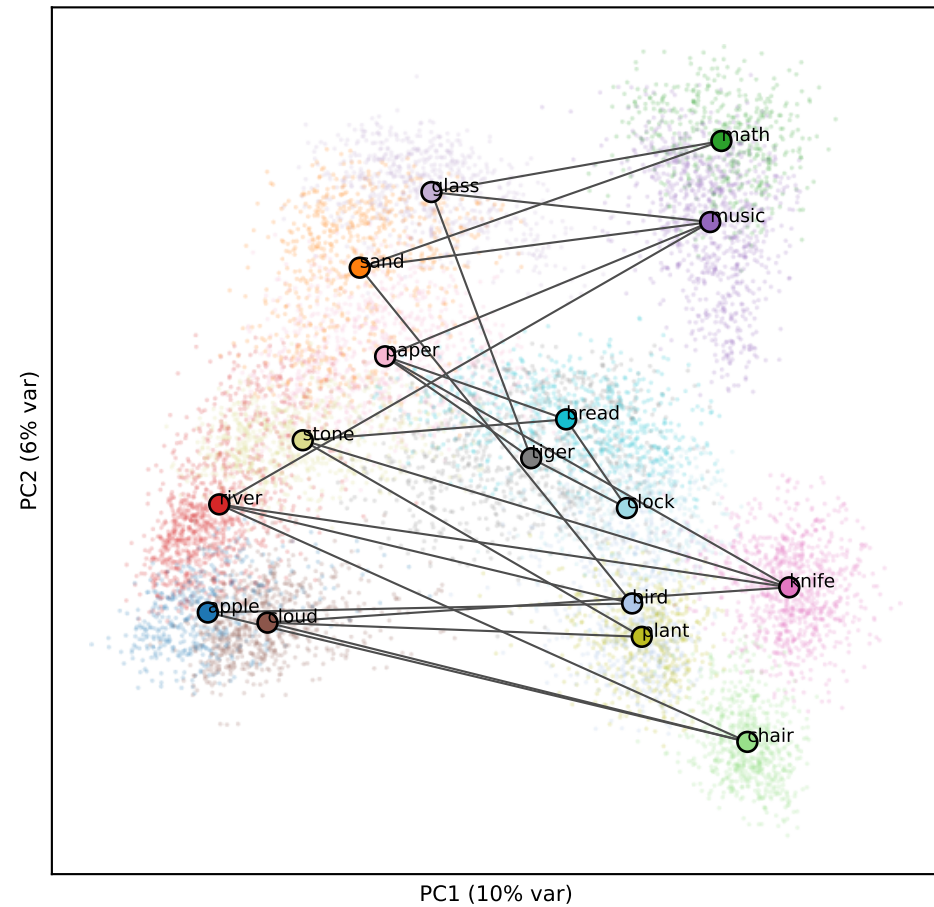
Llama L15 (RSA 0.11)
