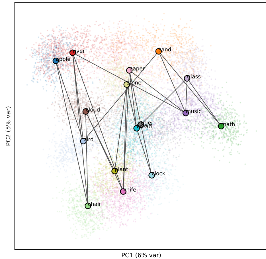
Llama L13 (RSA 0.27)
