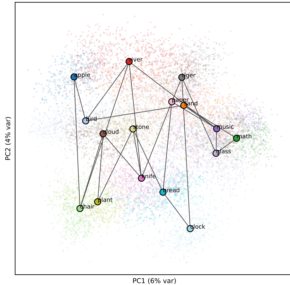
Gemma L16 (RSA 0.48)
