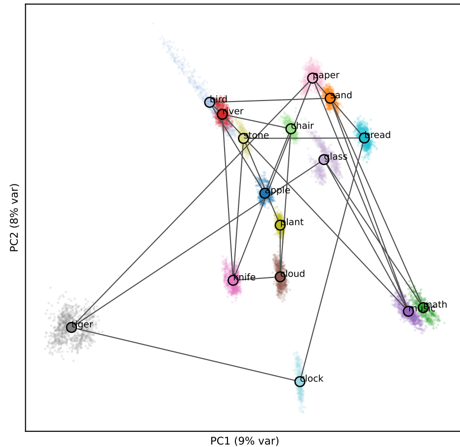
Qwen L7 (RSA 0.08)
