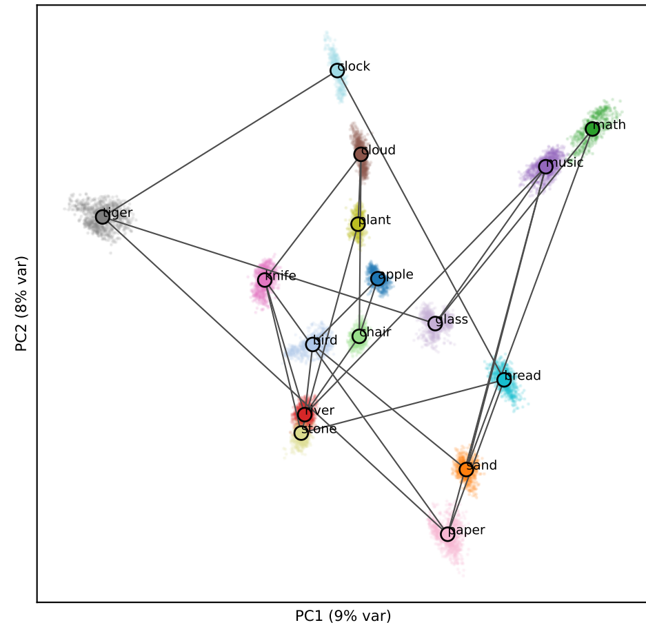
Qwen L9 (RSA 0.11)
