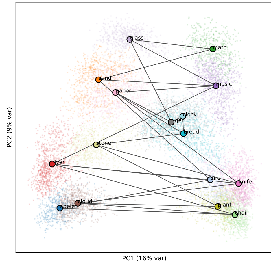
Llama L23 (RSA 0.13)
