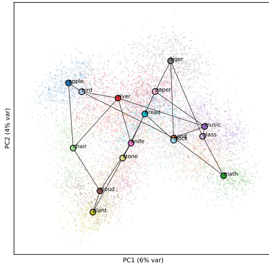
Gemma L17 (RSA 0.48)
