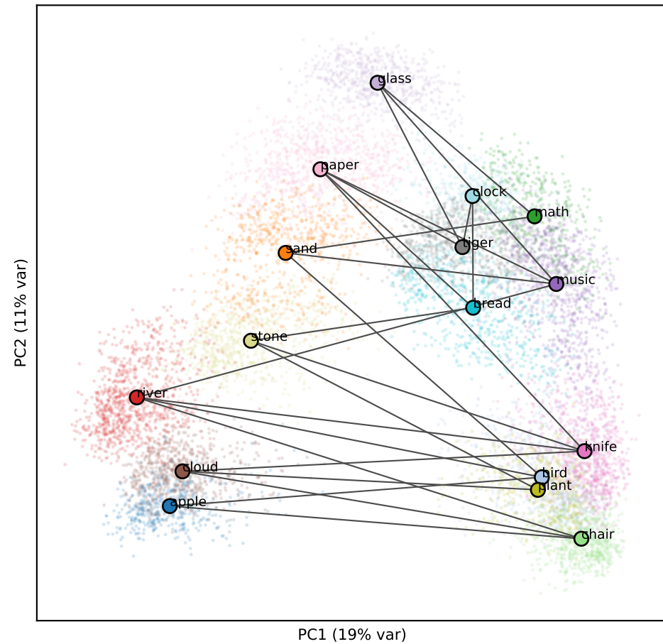
Llama L26 (RSA 0.12)
