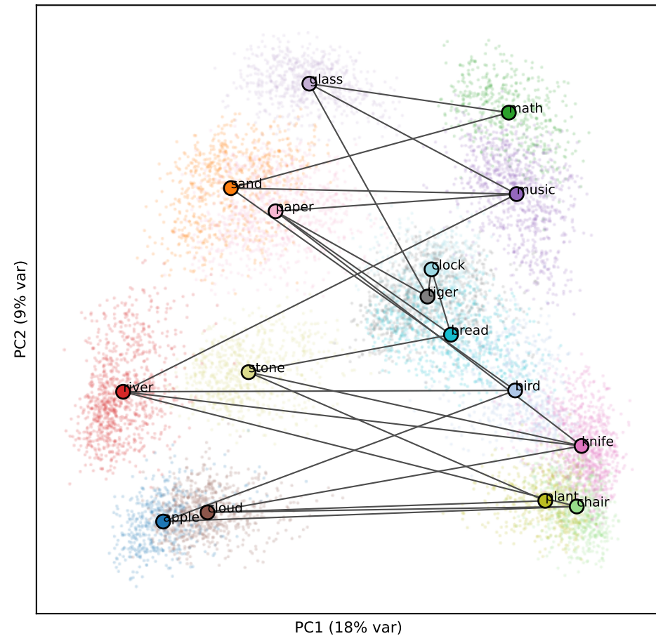
Llama L24 (RSA 0.12)
