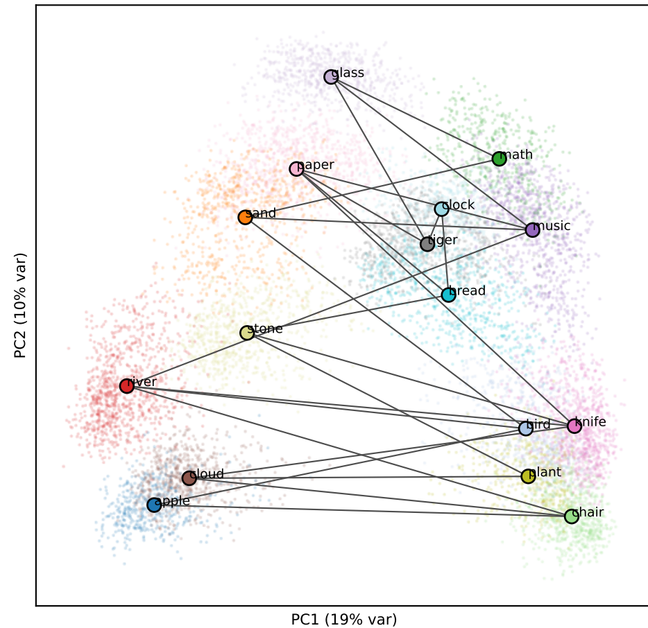
Llama L25 (RSA 0.12)
