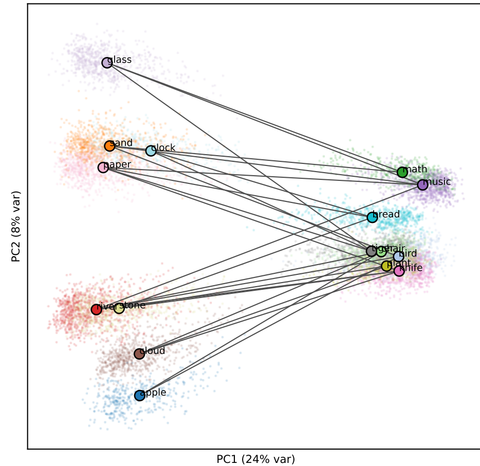
Qwen L30 (RSA -0.04)
