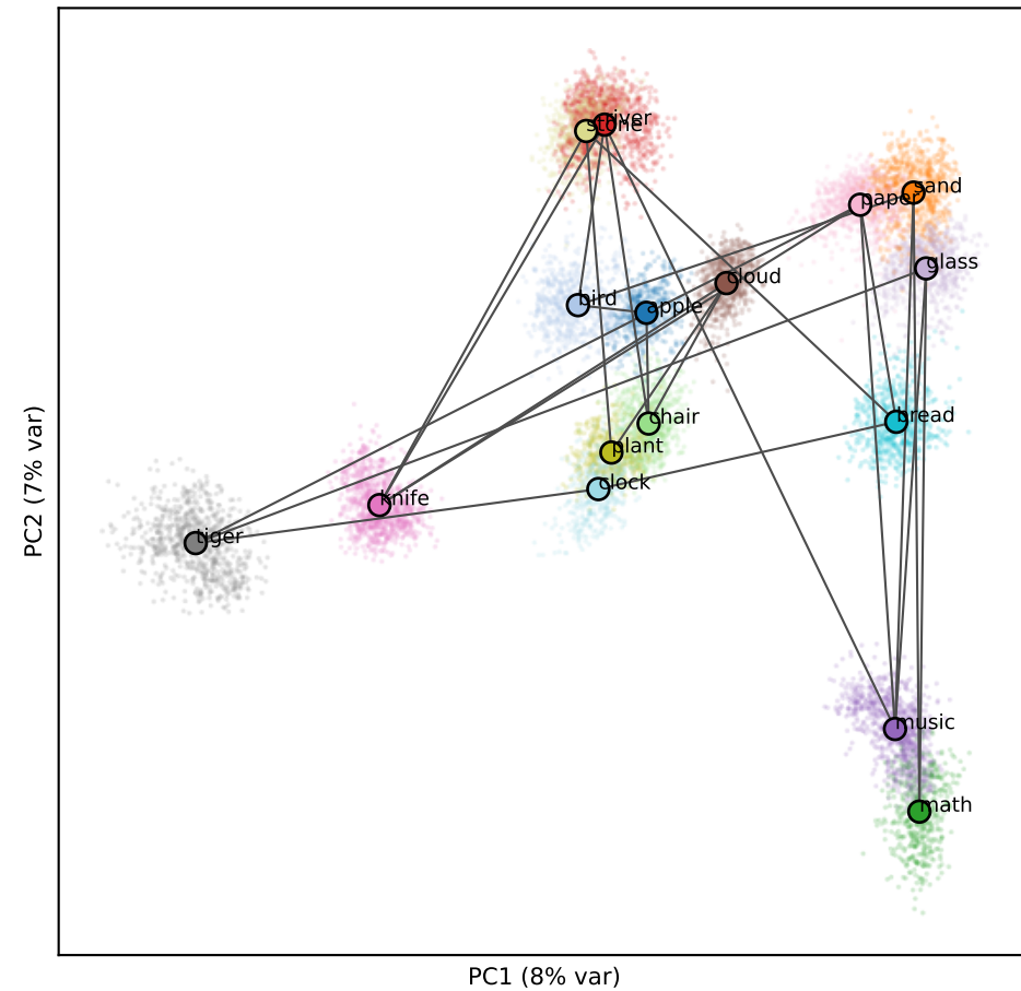
Qwen L17 (RSA 0.04)
