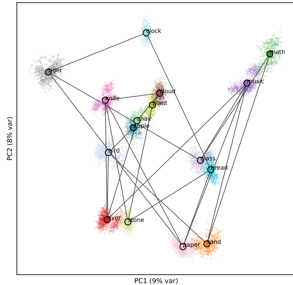
Qwen L13 (RSA 0.08)
