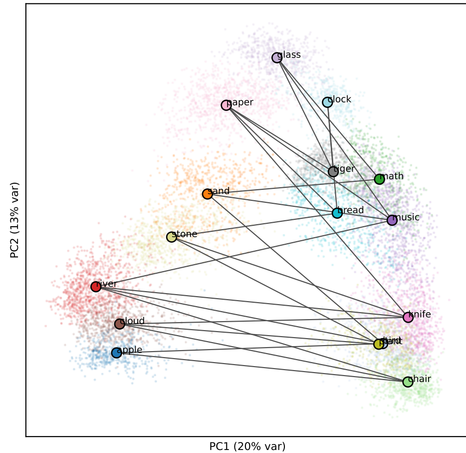
Llama L28 (RSA 0.14)
