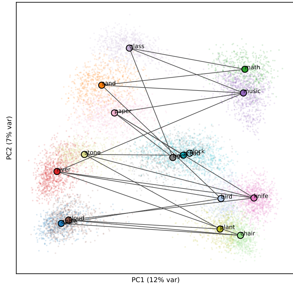
Llama L16 (RSA 0.09)
