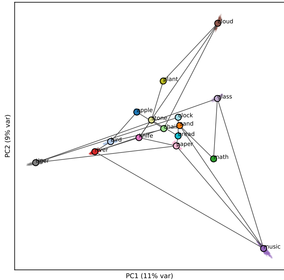
Qwen L0 (RSA -0.07)
