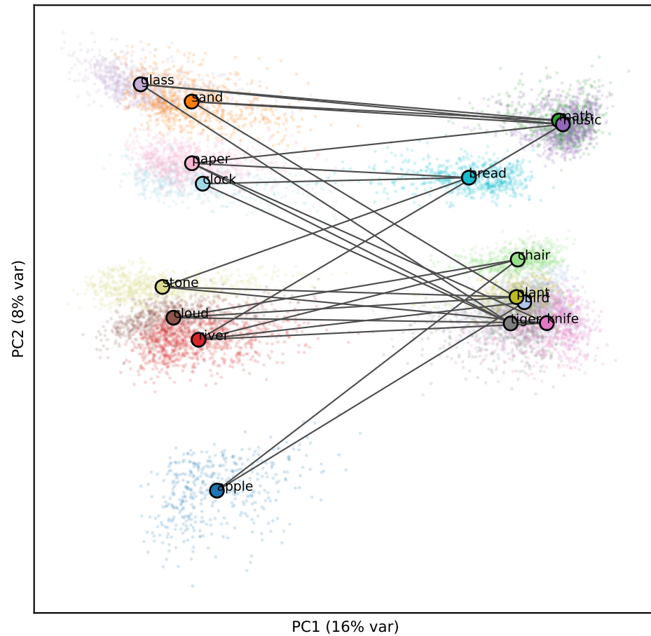
Qwen L26 (RSA -0.02)
