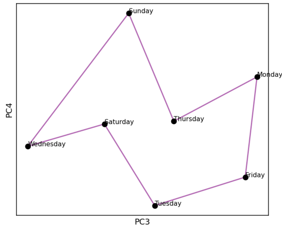
Gemma L33 PC3-4 (context-RSA=+0.51)
