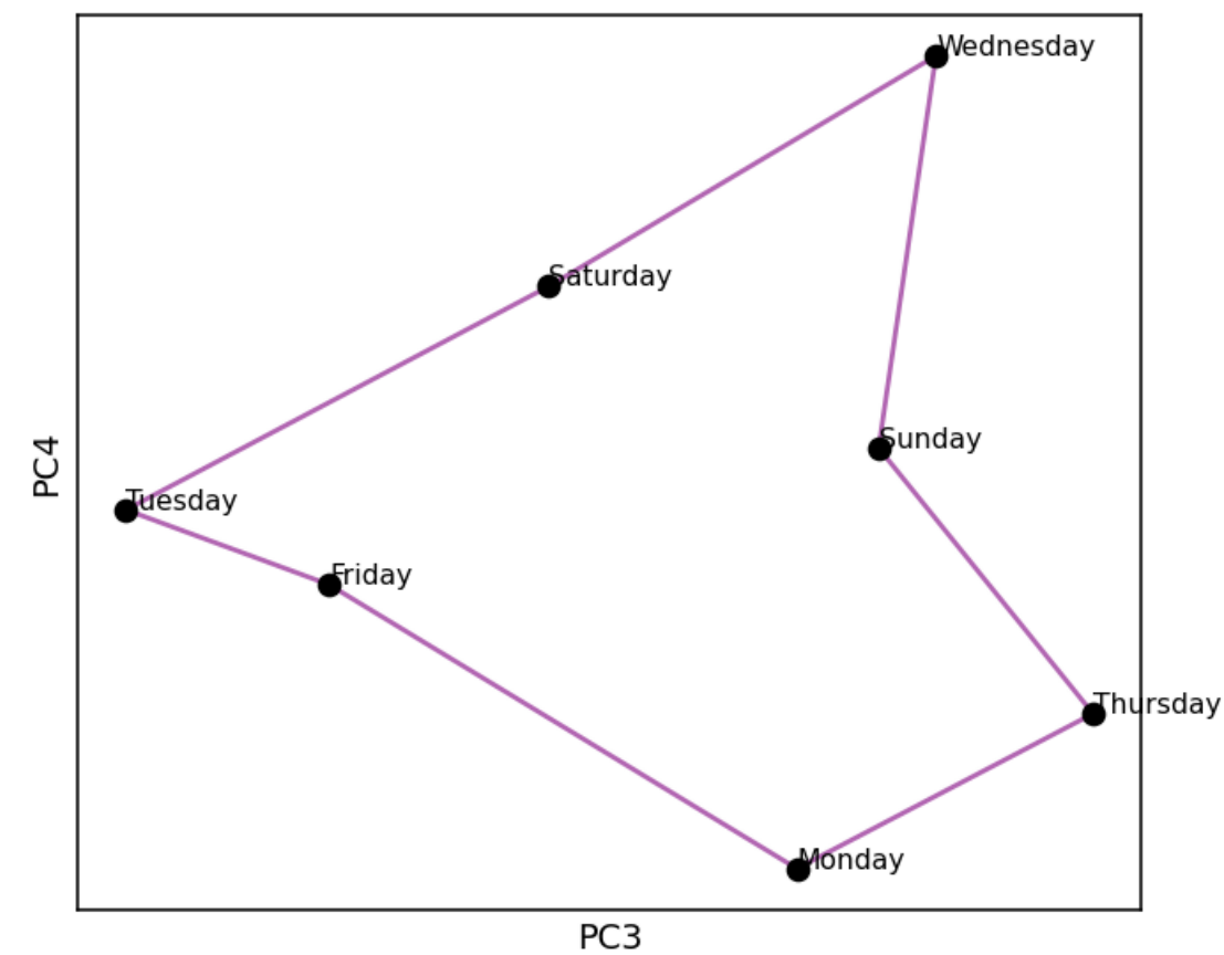
Qwen L28 PC3-4 (context-RSA=+0.65)
