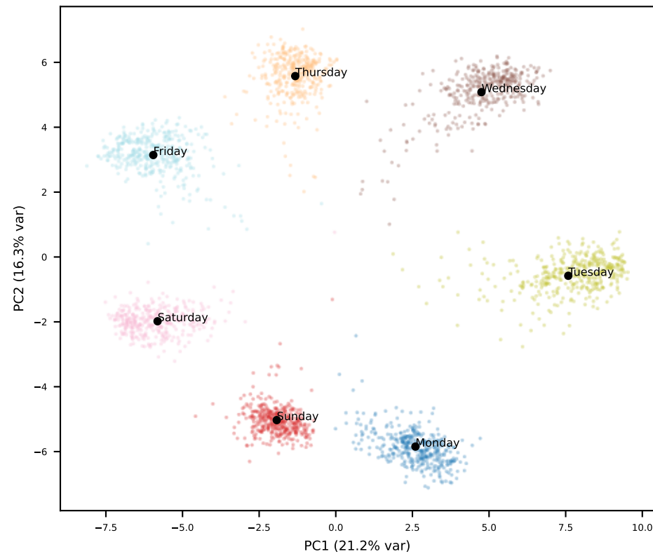
Llama L24
