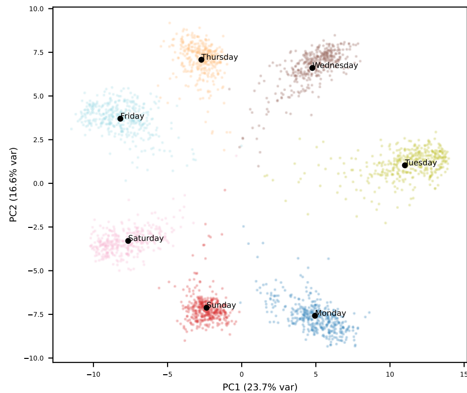
Llama L28
