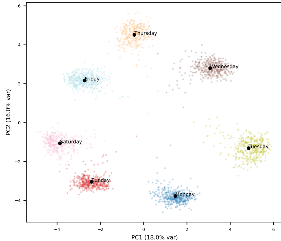
Llama L19
