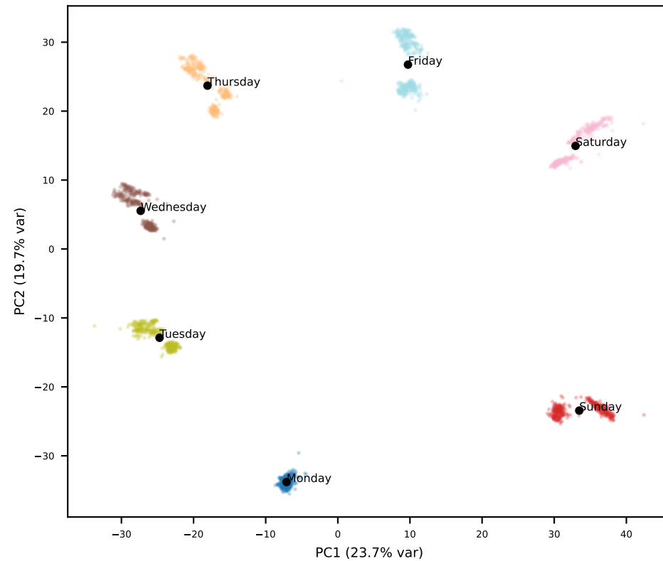
Gemma L9
