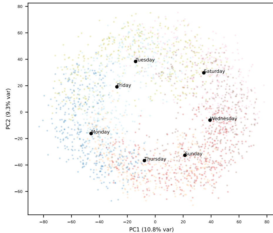
Gemma L27
