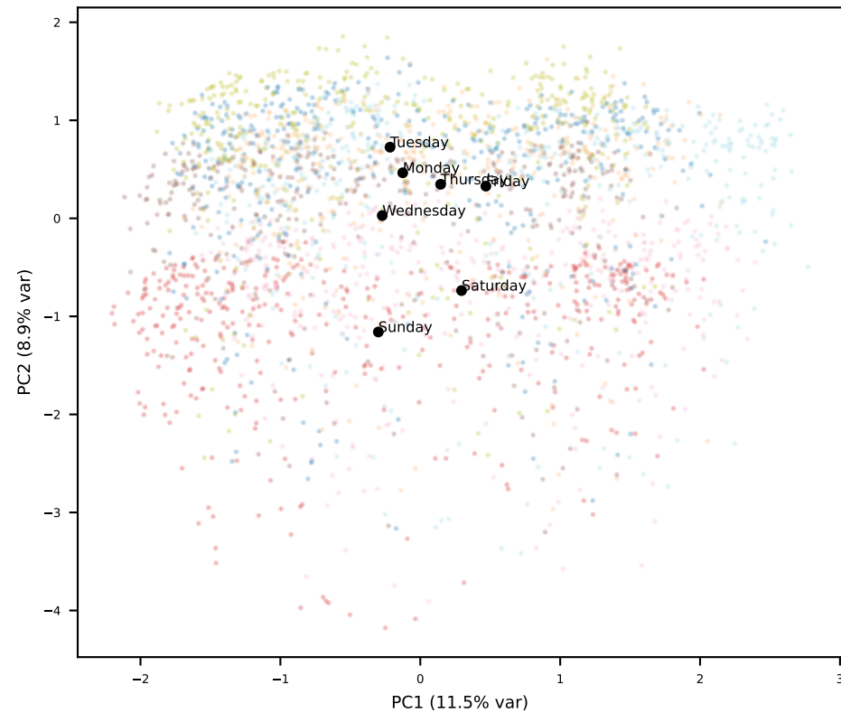
Llama L10
