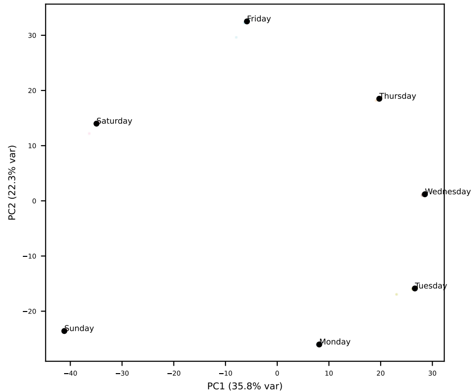
Gemma L0
