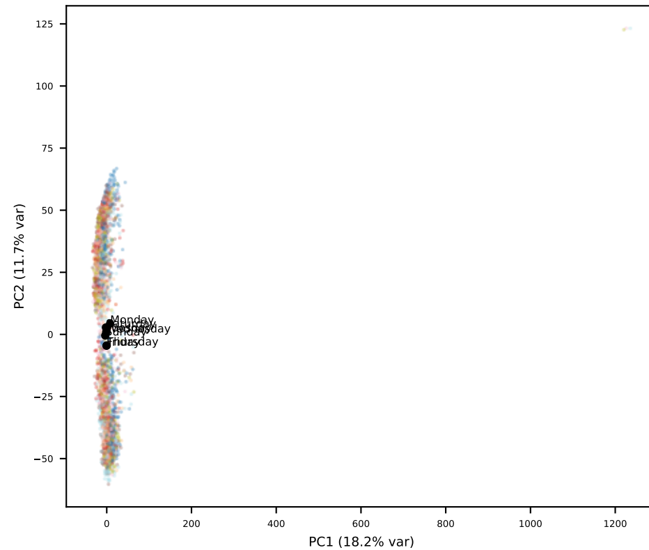
Gemma L17
