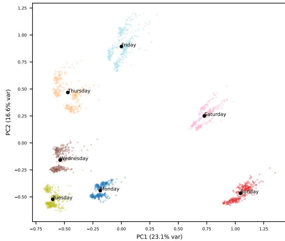
Llama L3
