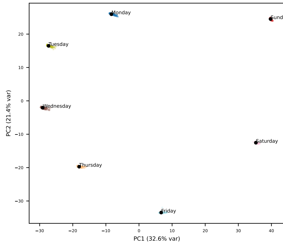
Gemma L1
