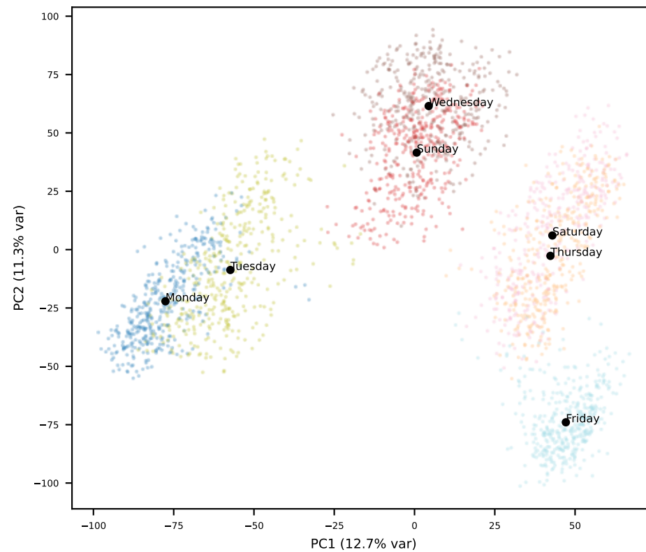
Gemma L29
