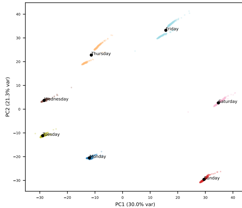
Gemma L3
