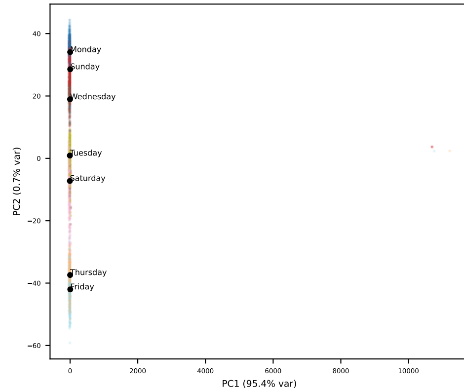
Qwen L23
