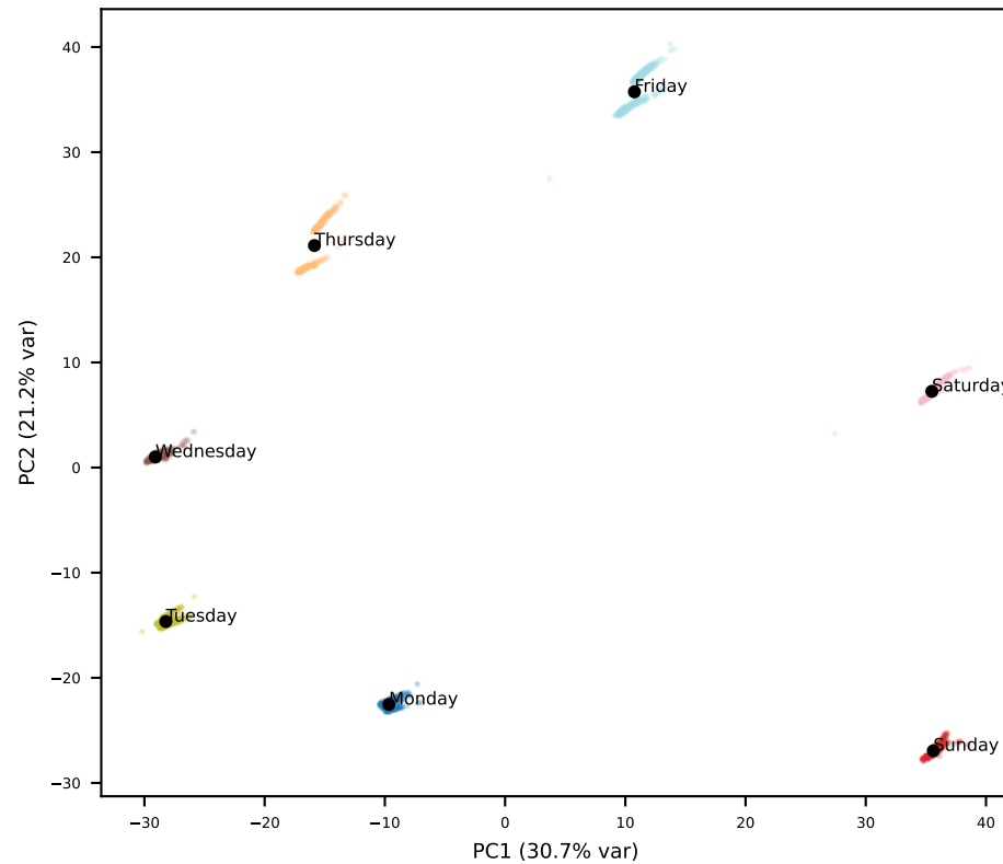
Gemma L2
