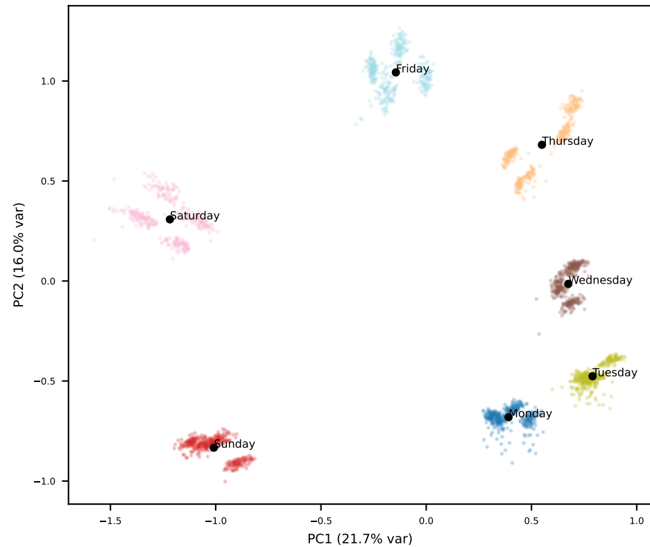
Llama L4
