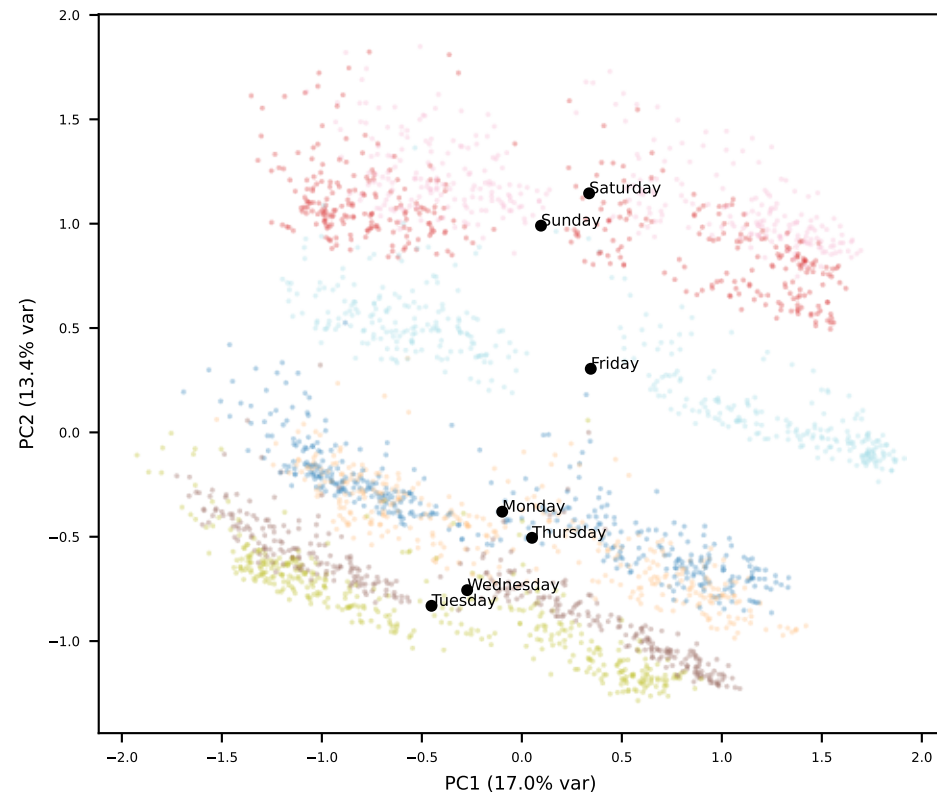
Llama L6
