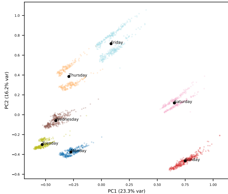
Llama L2
