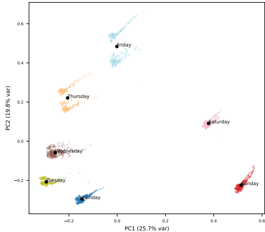
Llama L0
