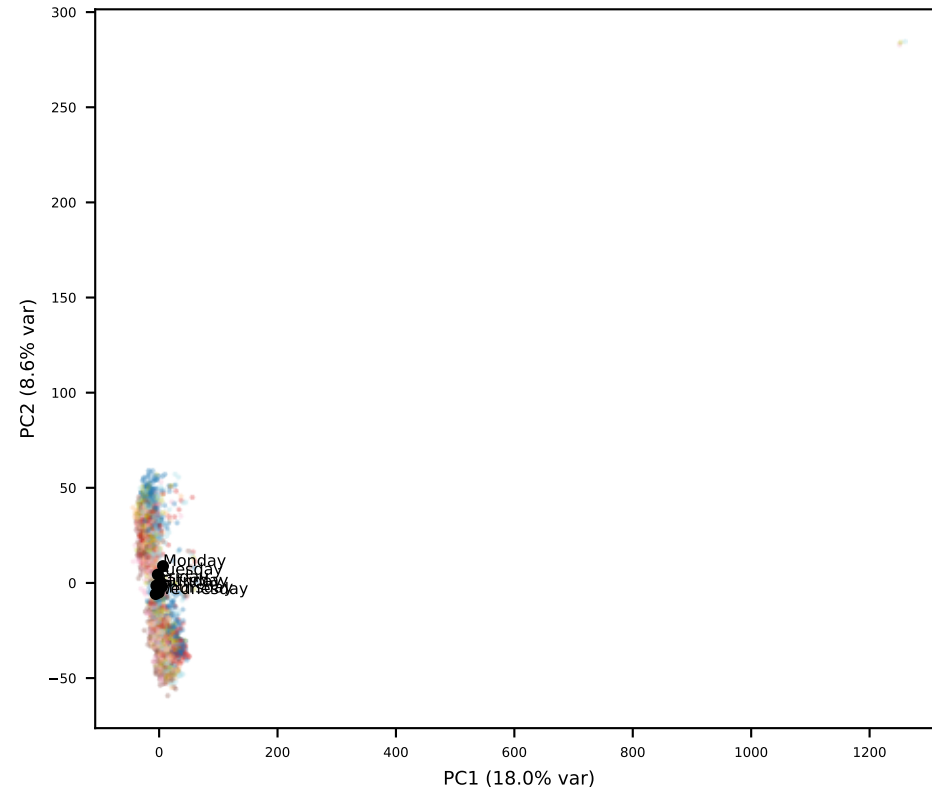
Gemma L21
