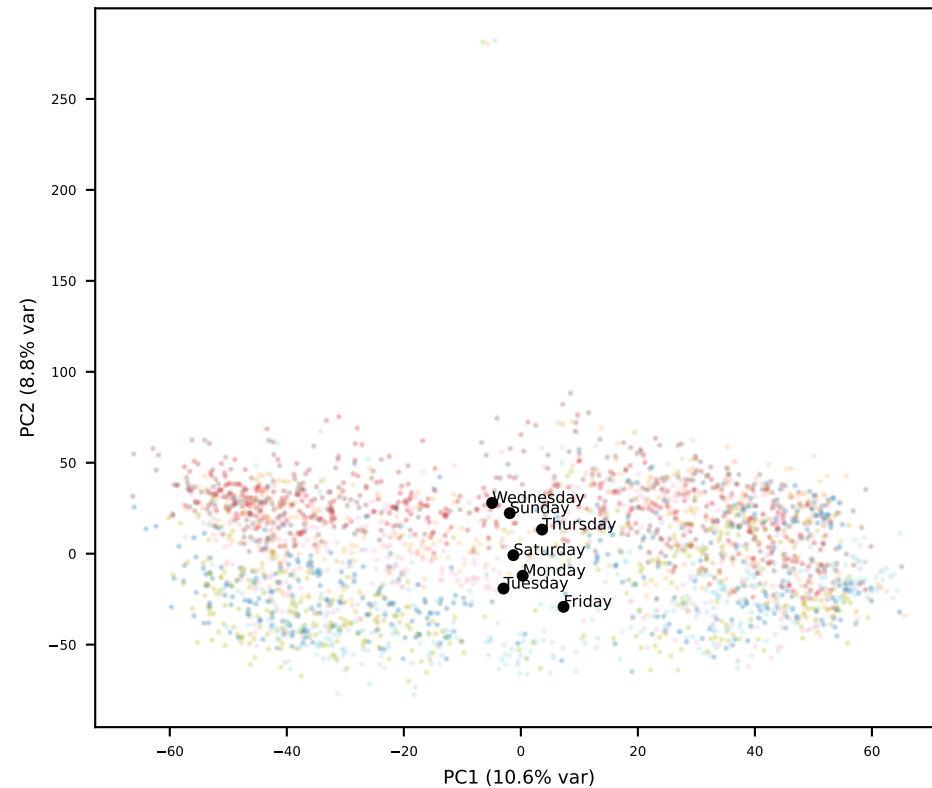
Gemma L23
