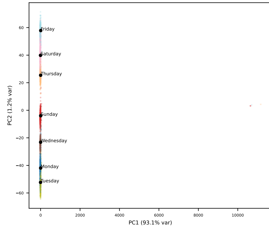
Qwen L25
