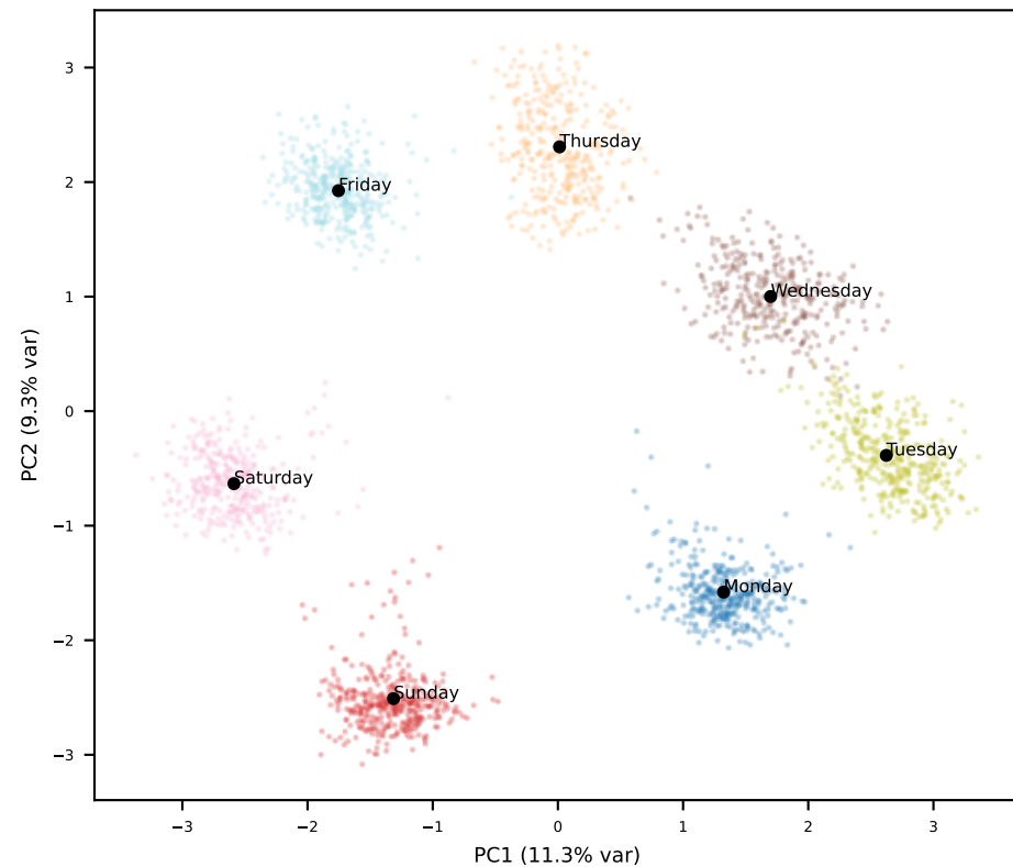
Llama L15
