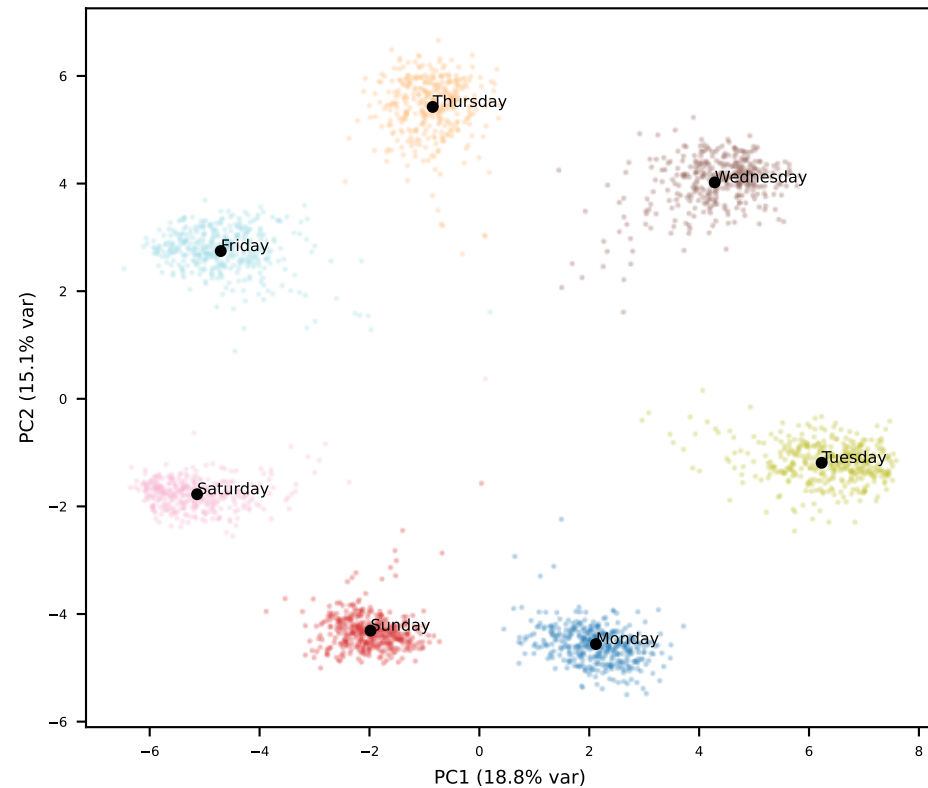
Llama L22
