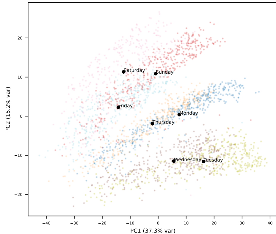
Llama L31
