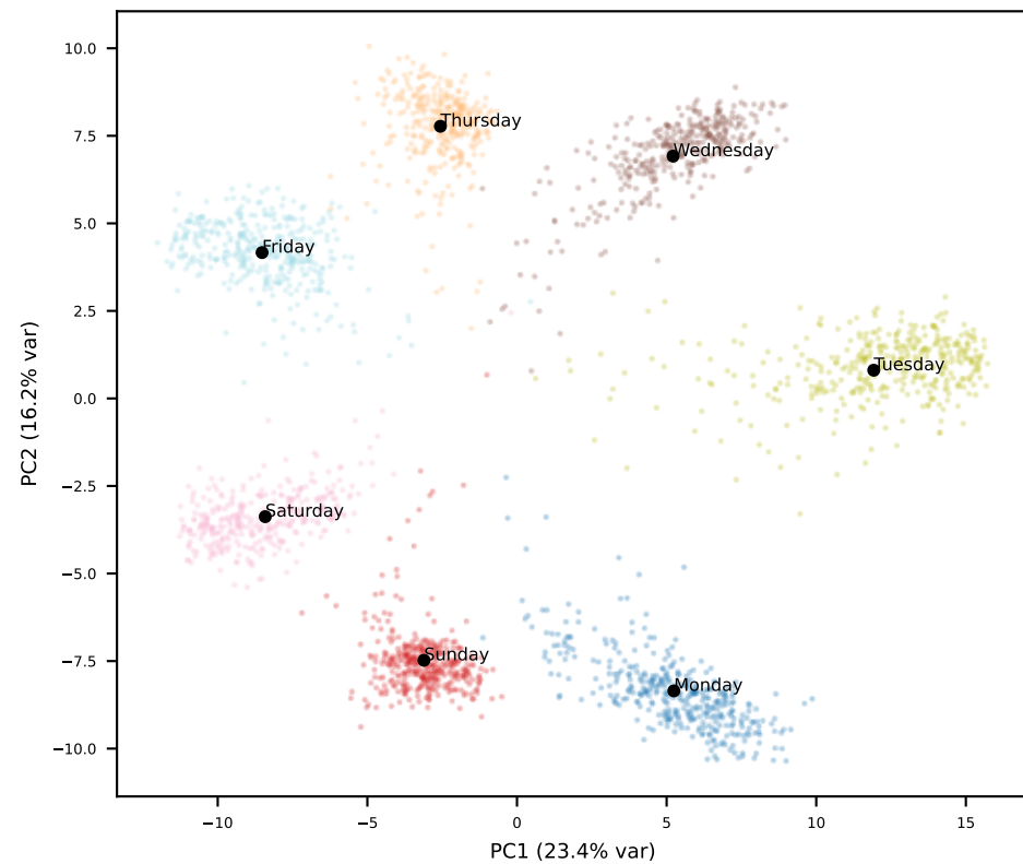
Llama L29
