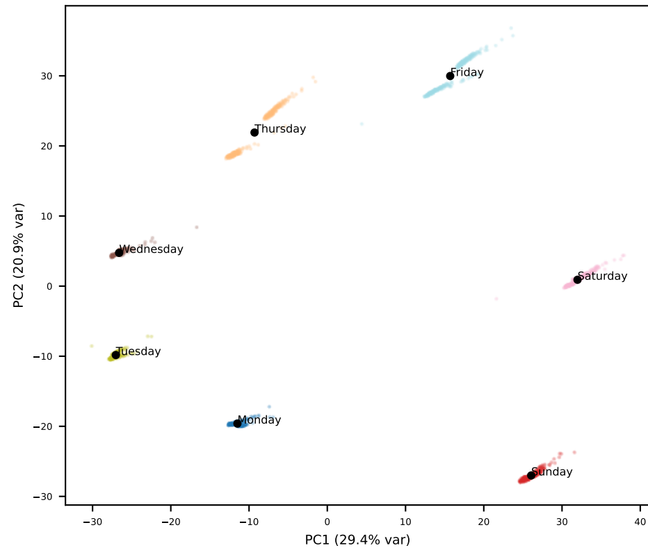
Gemma L4
