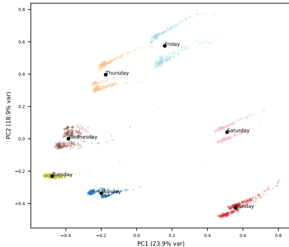
Llama L1
