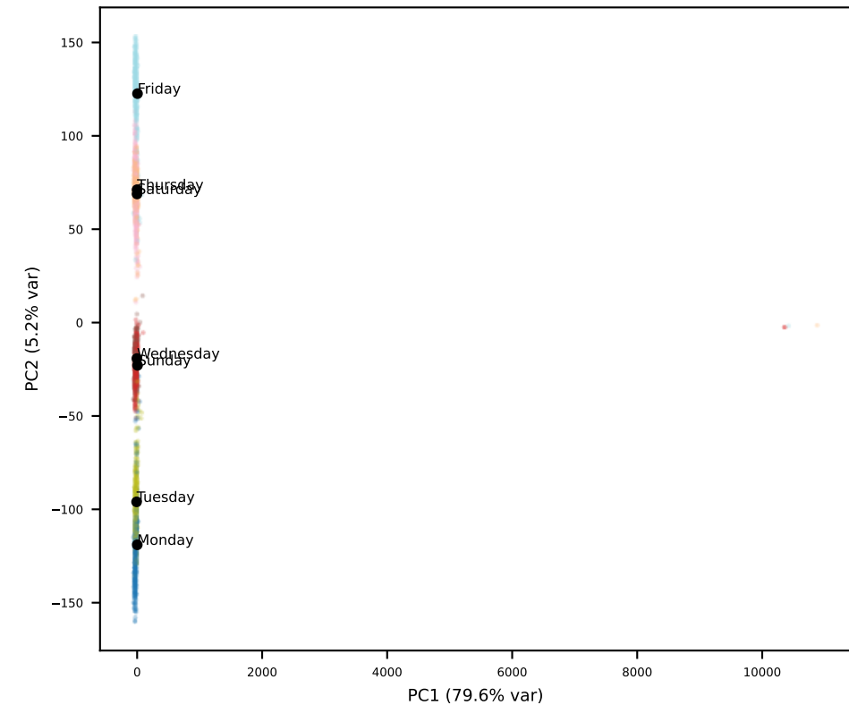
Qwen L31
