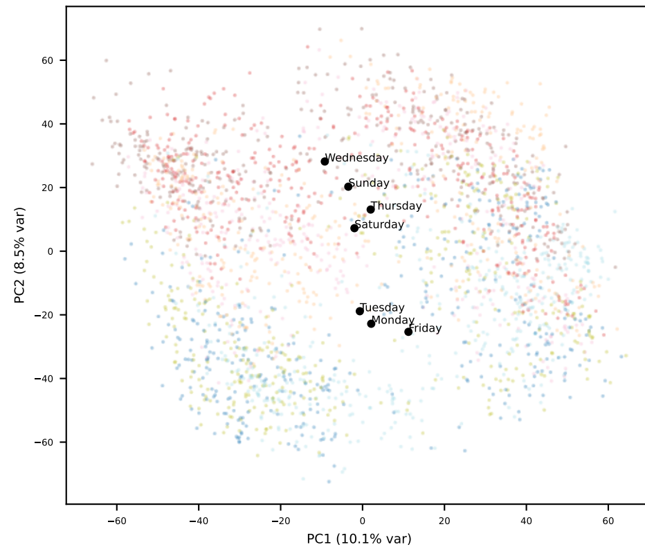
Gemma L24
