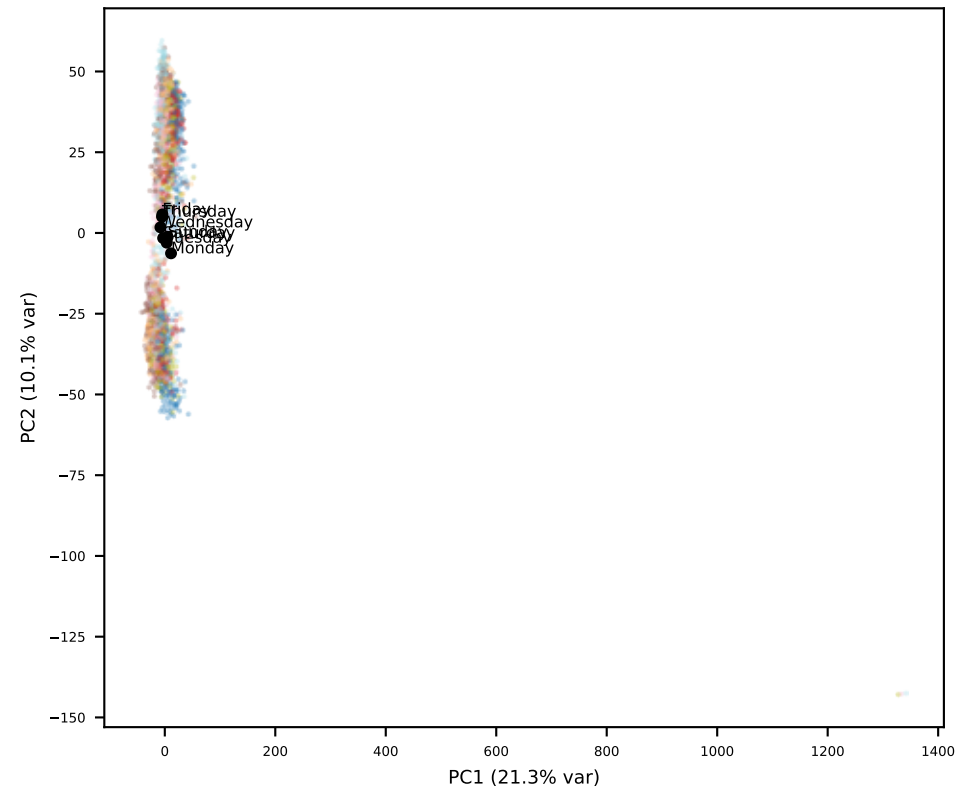
Gemma L19
