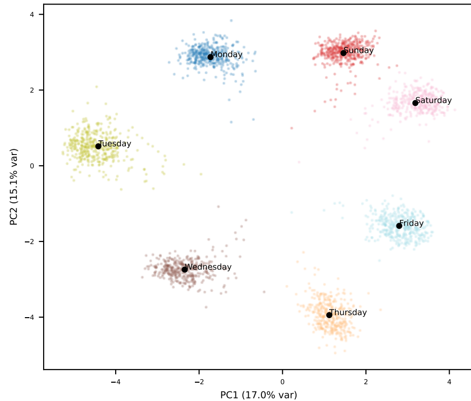
Llama L17
