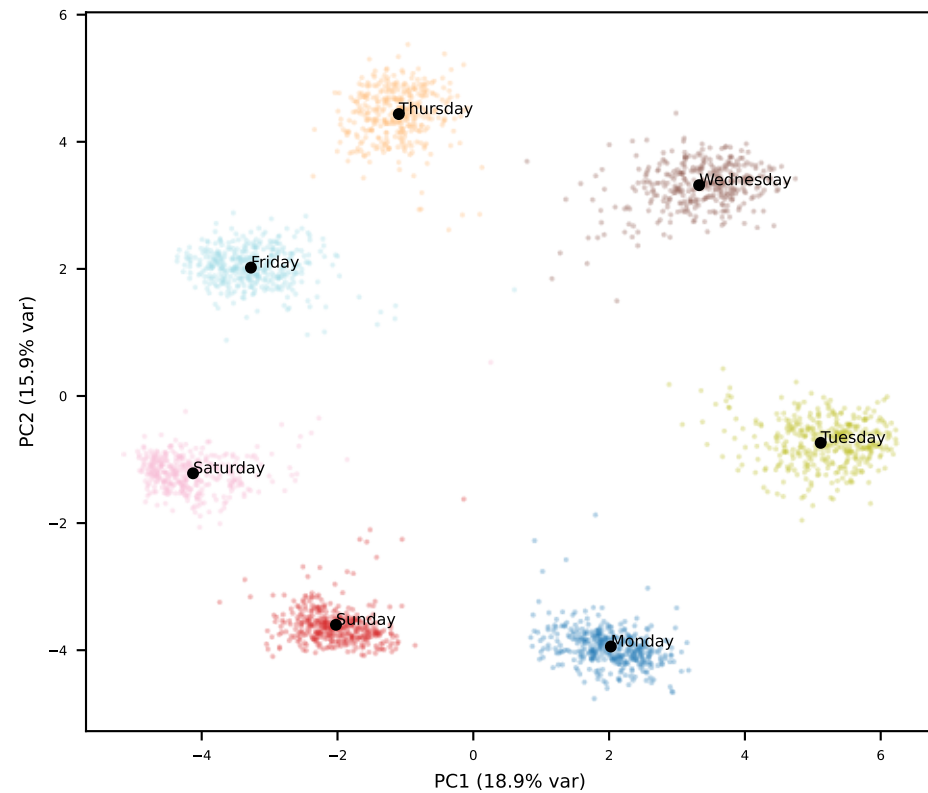
Llama L20
