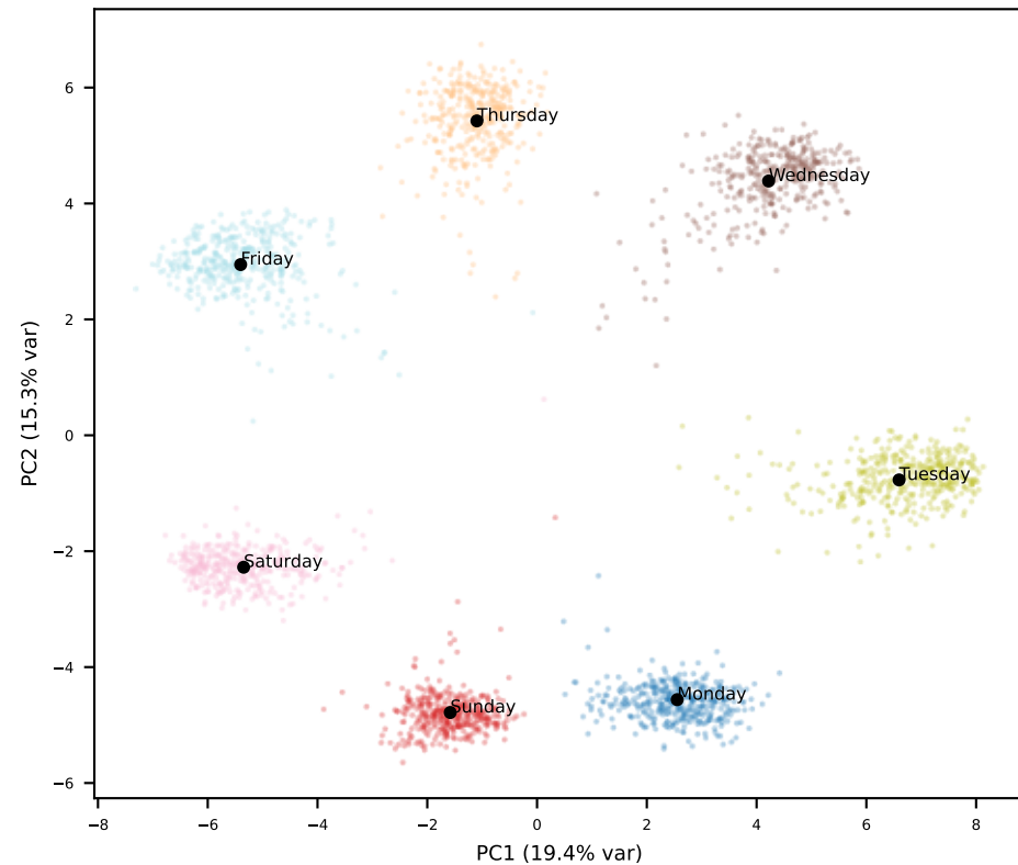
Llama L23
