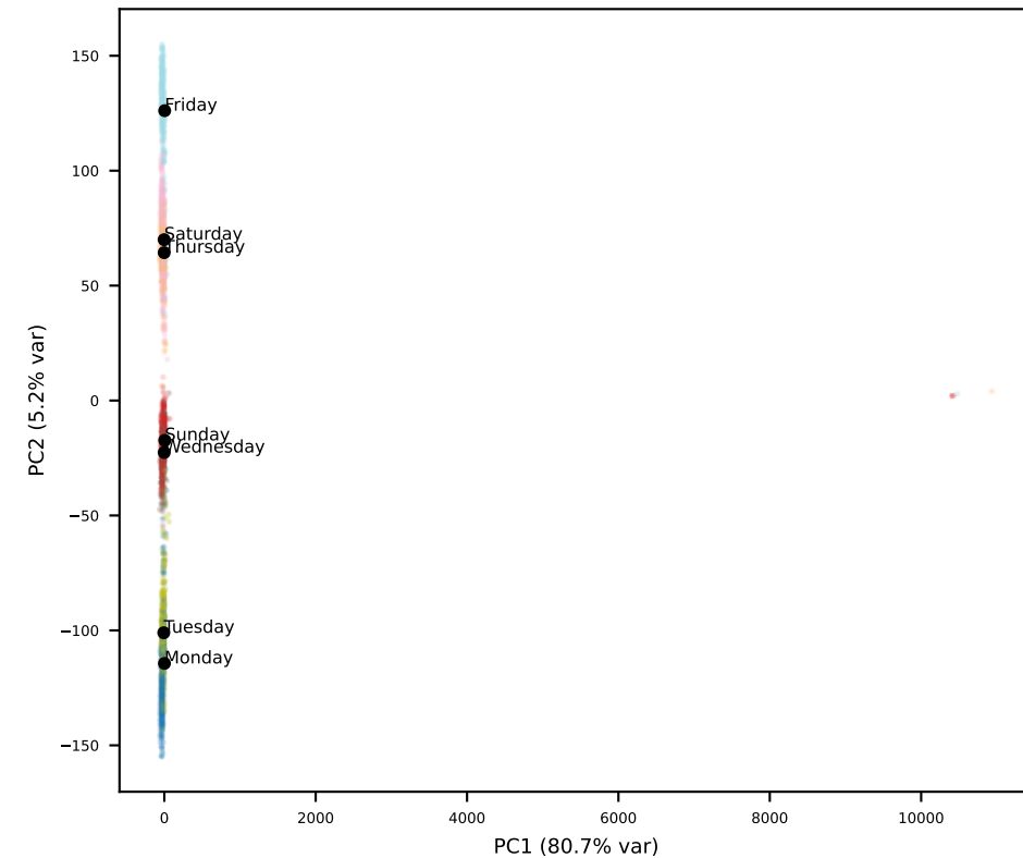
Qwen L30
