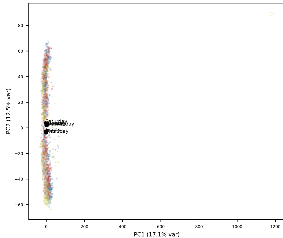
Gemma L16
