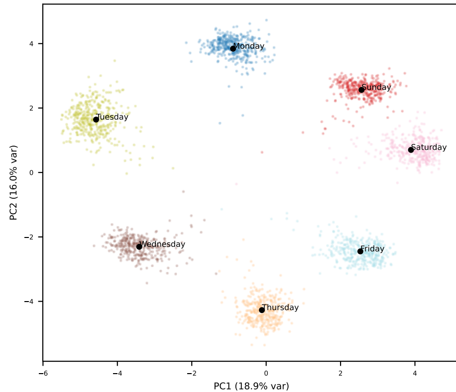
Llama L18
