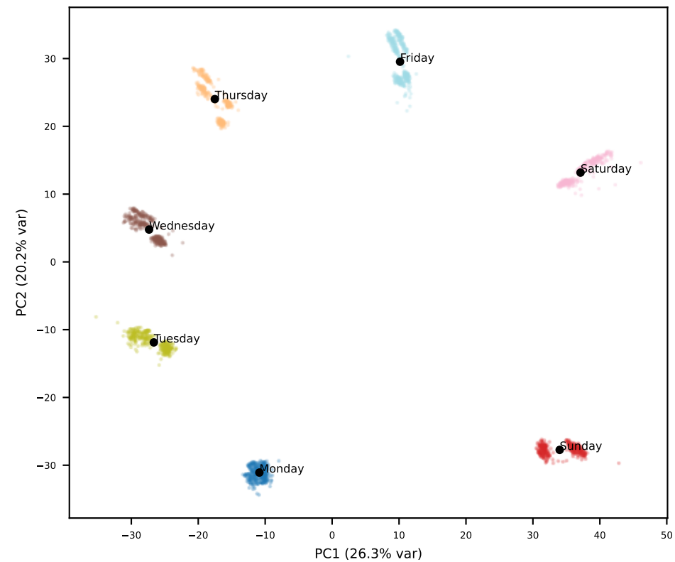
Gemma L8
