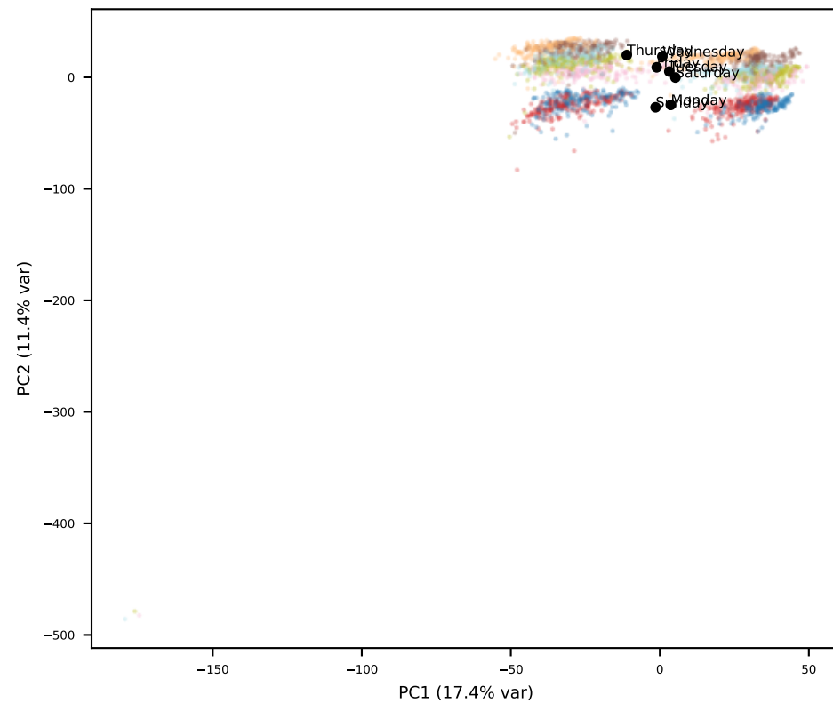
Gemma L14
