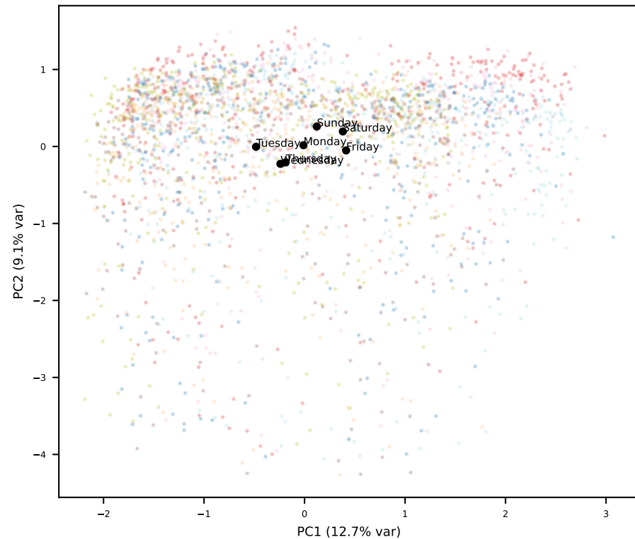
Llama L11
