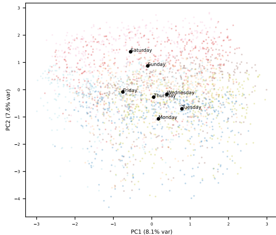
Llama L13
