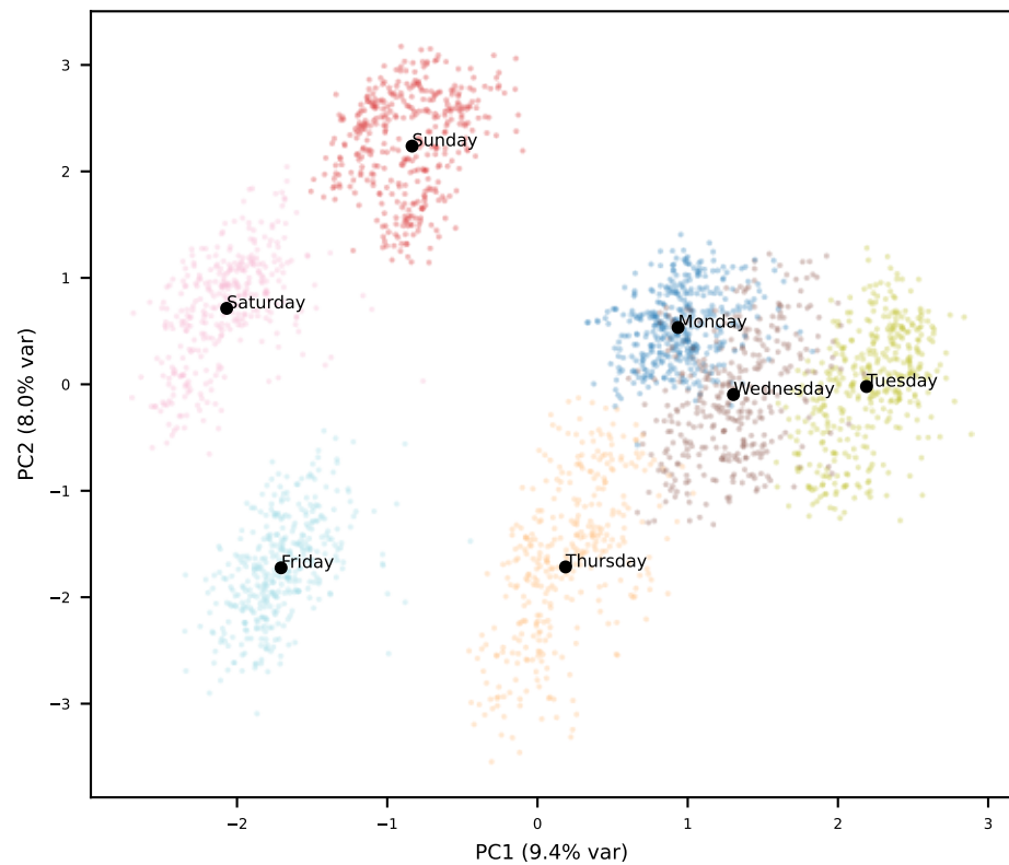
Llama L14
