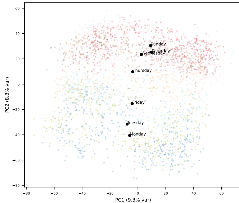
Gemma L26
