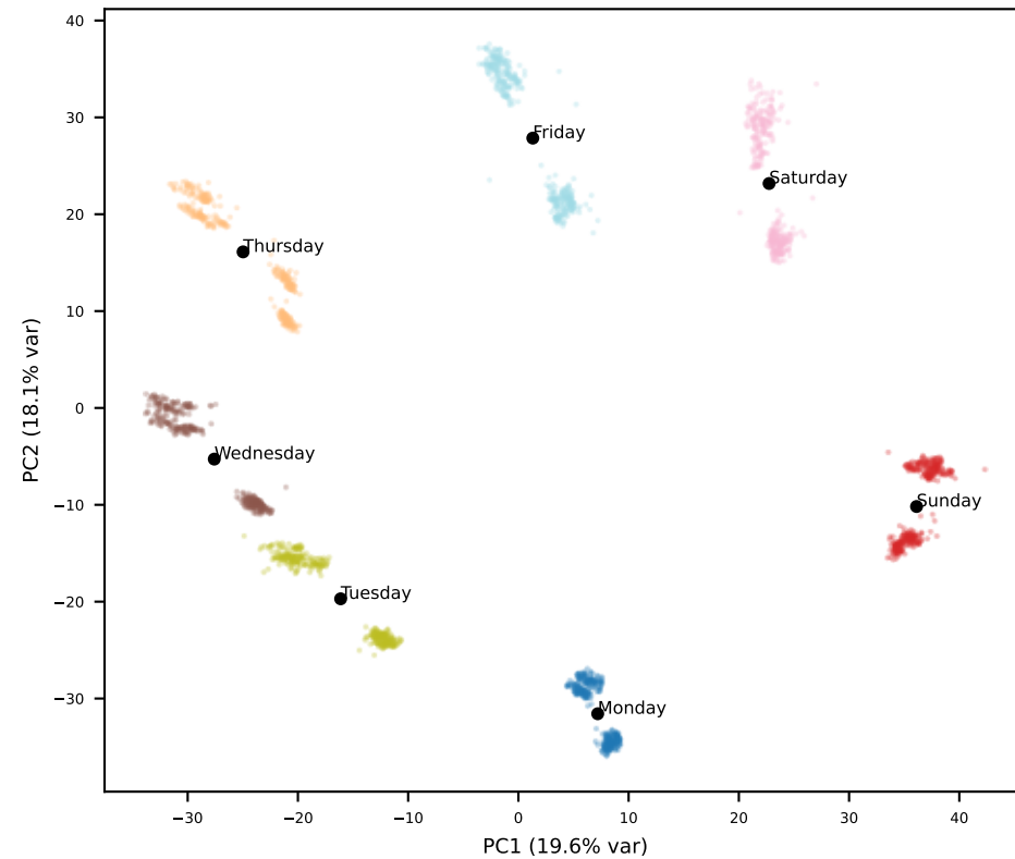
Gemma L10
