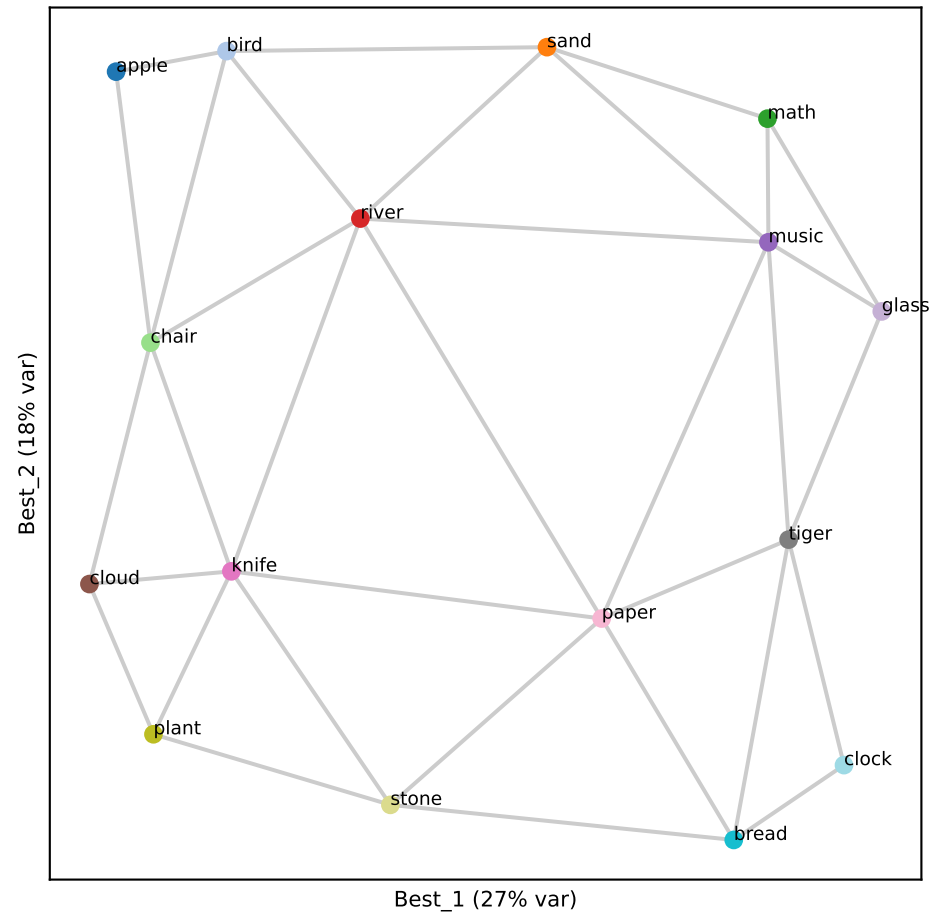
Gemma L39 (RSA 0.89)
