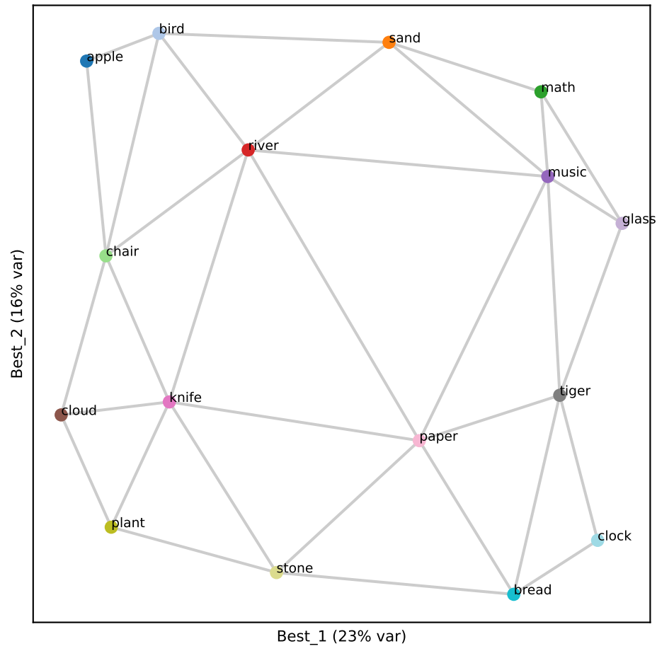
Gemma L38 (RSA 0.89)
