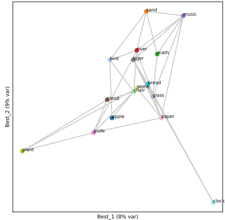
Qwen L1 (RSA 0.23)
