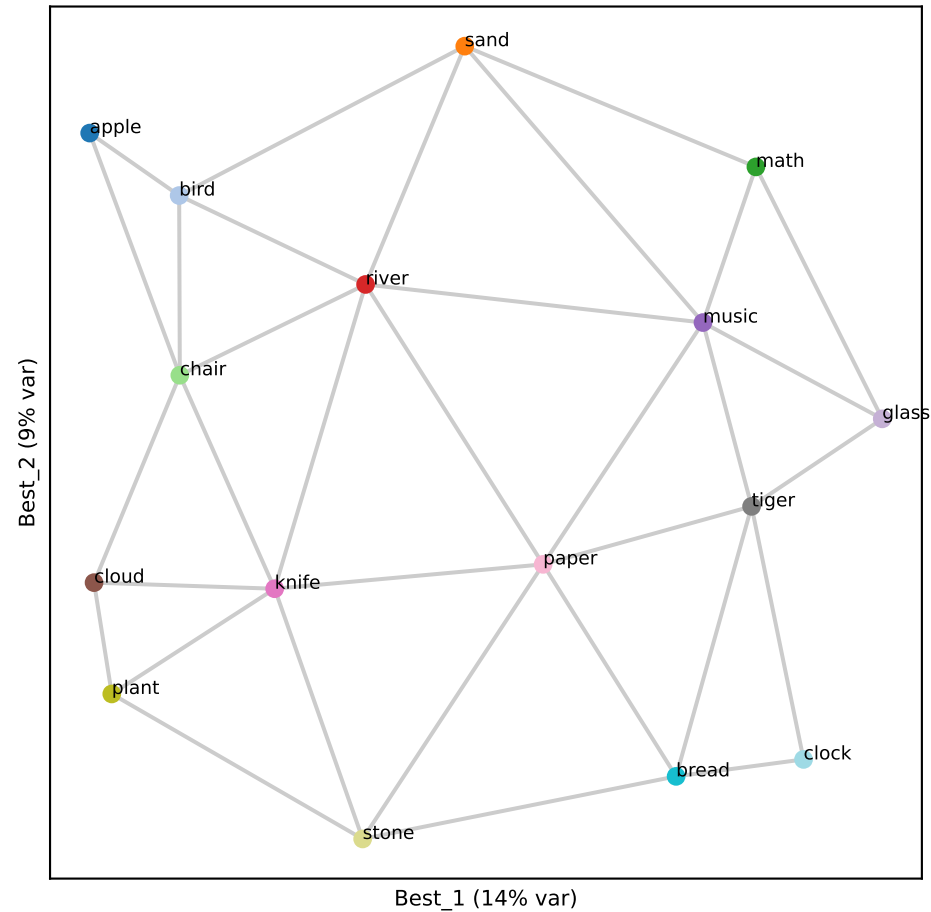
Gemma L32 (RSA 0.90)
