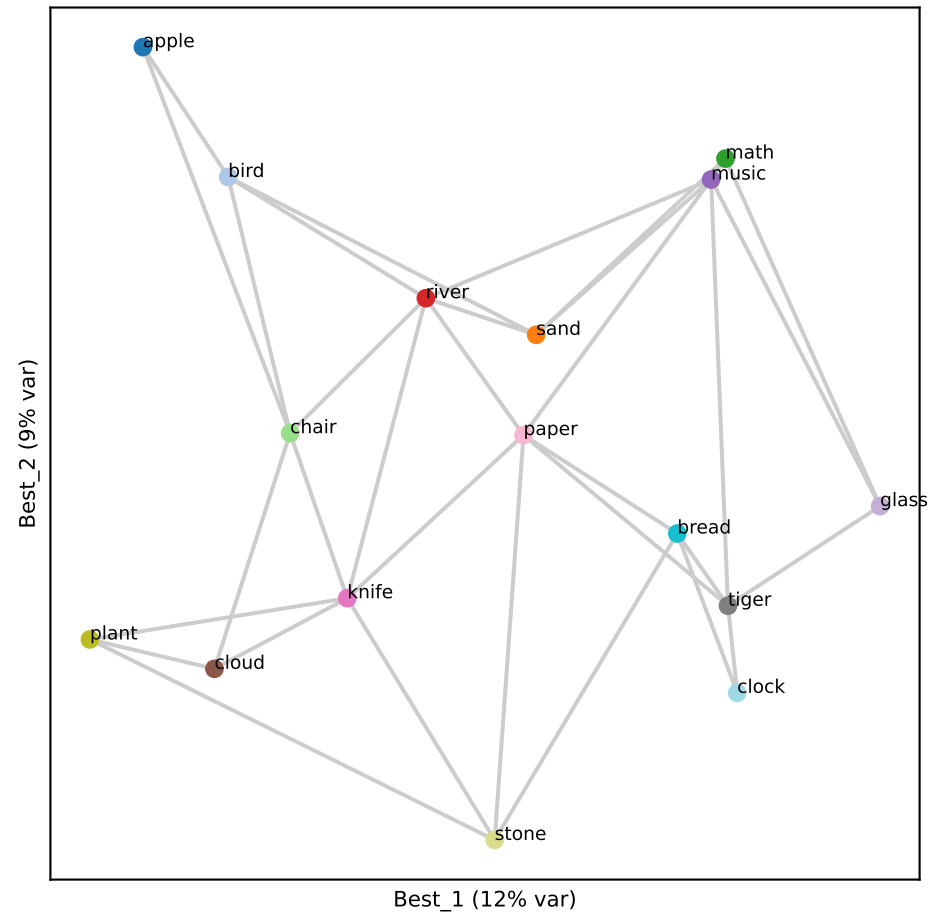
Llama L14 (RSA 0.77)
