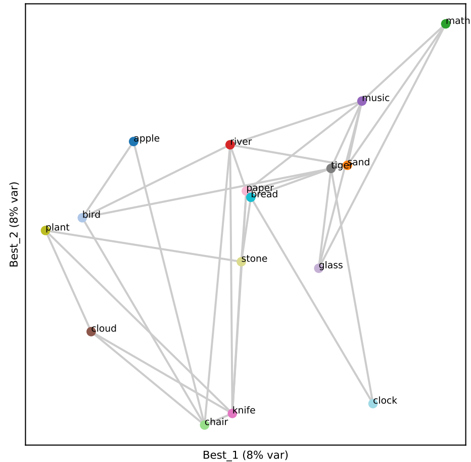
Llama L2 (RSA 0.52)
