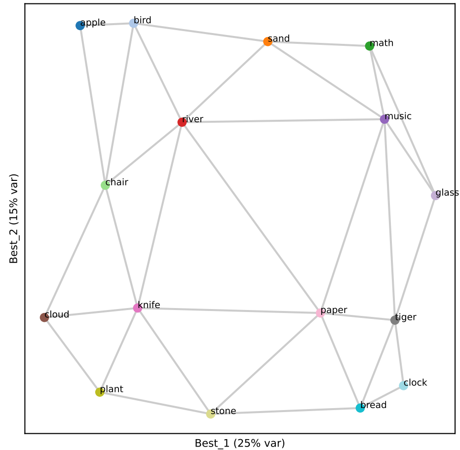
Llama L28 (RSA 0.88)
