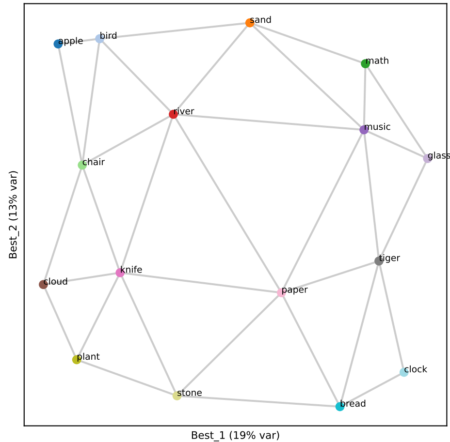
Gemma L35 (RSA 0.90)
