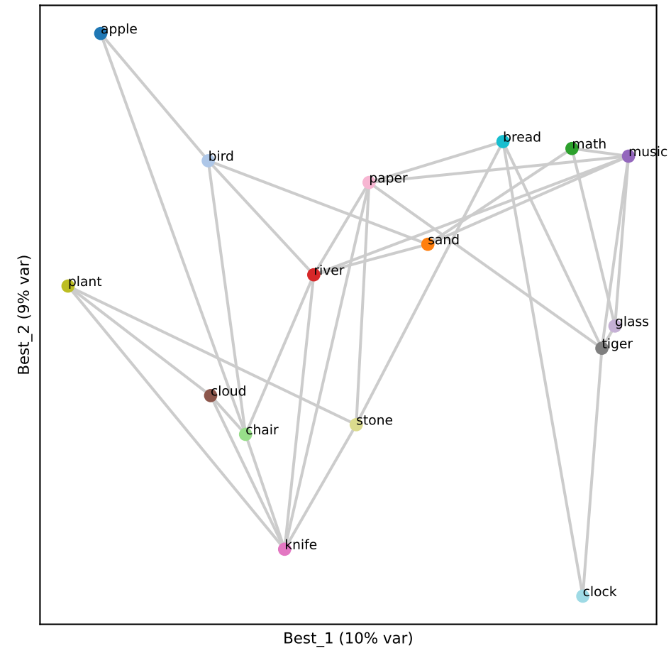
Qwen L21 (RSA 0.64)
