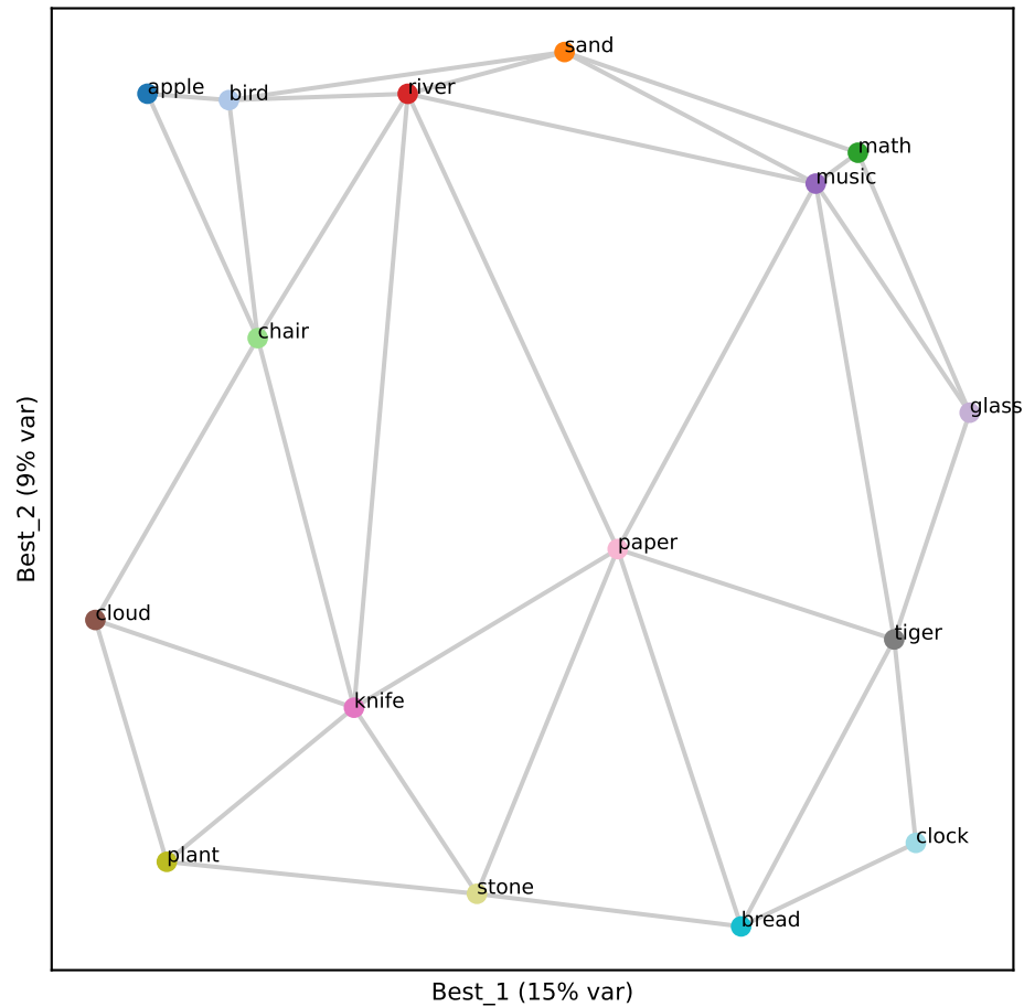
Gemma L28 (RSA 0.85)
