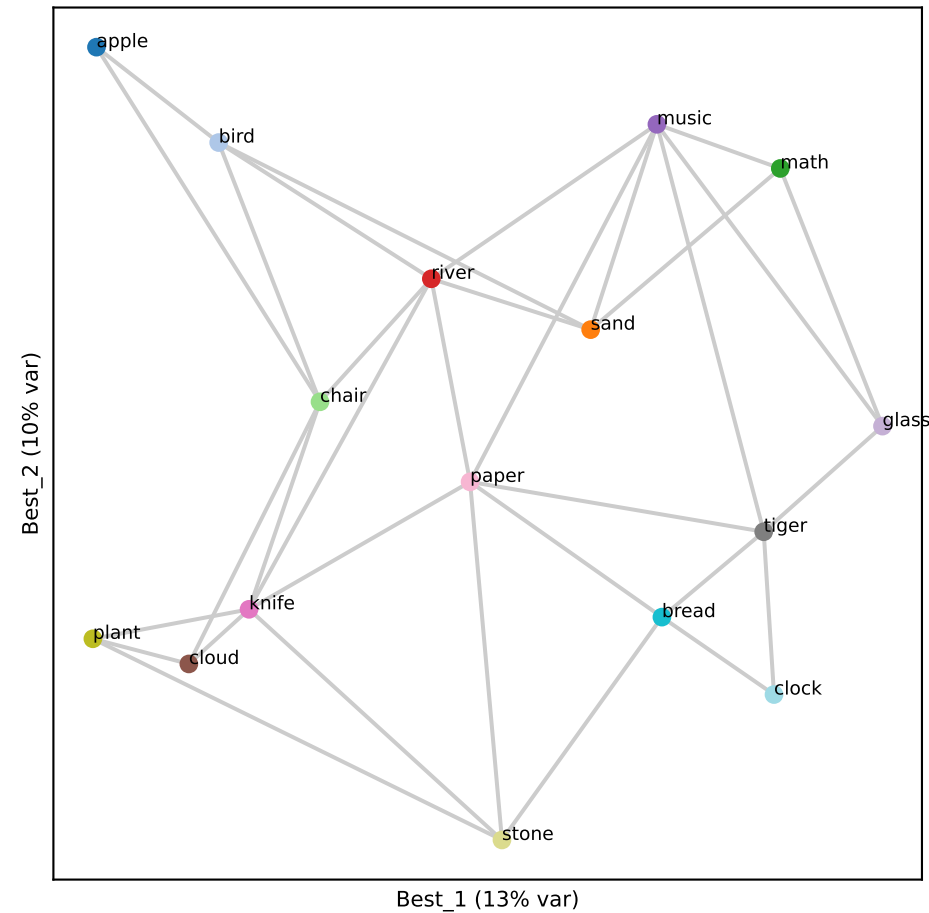
Llama L9 (RSA 0.78)
