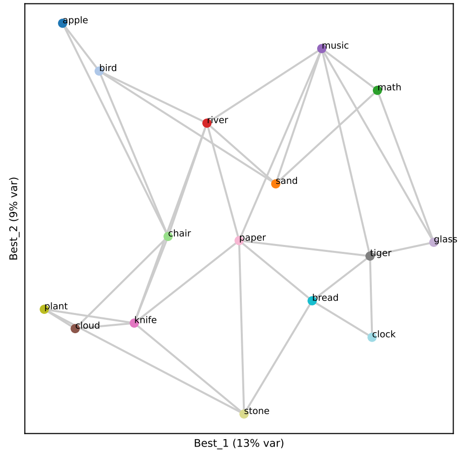
Llama L8 (RSA 0.73)
