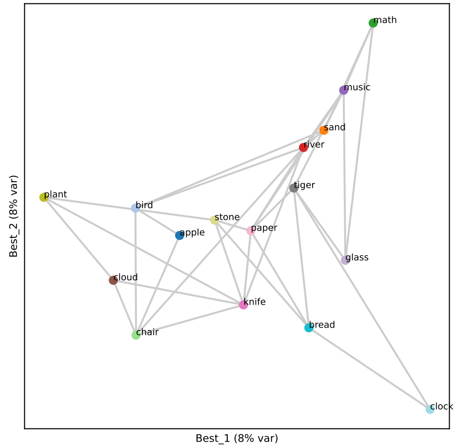
Gemma L2 (RSA 0.56)
