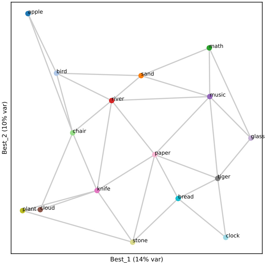
Llama L17 (RSA 0.86)
