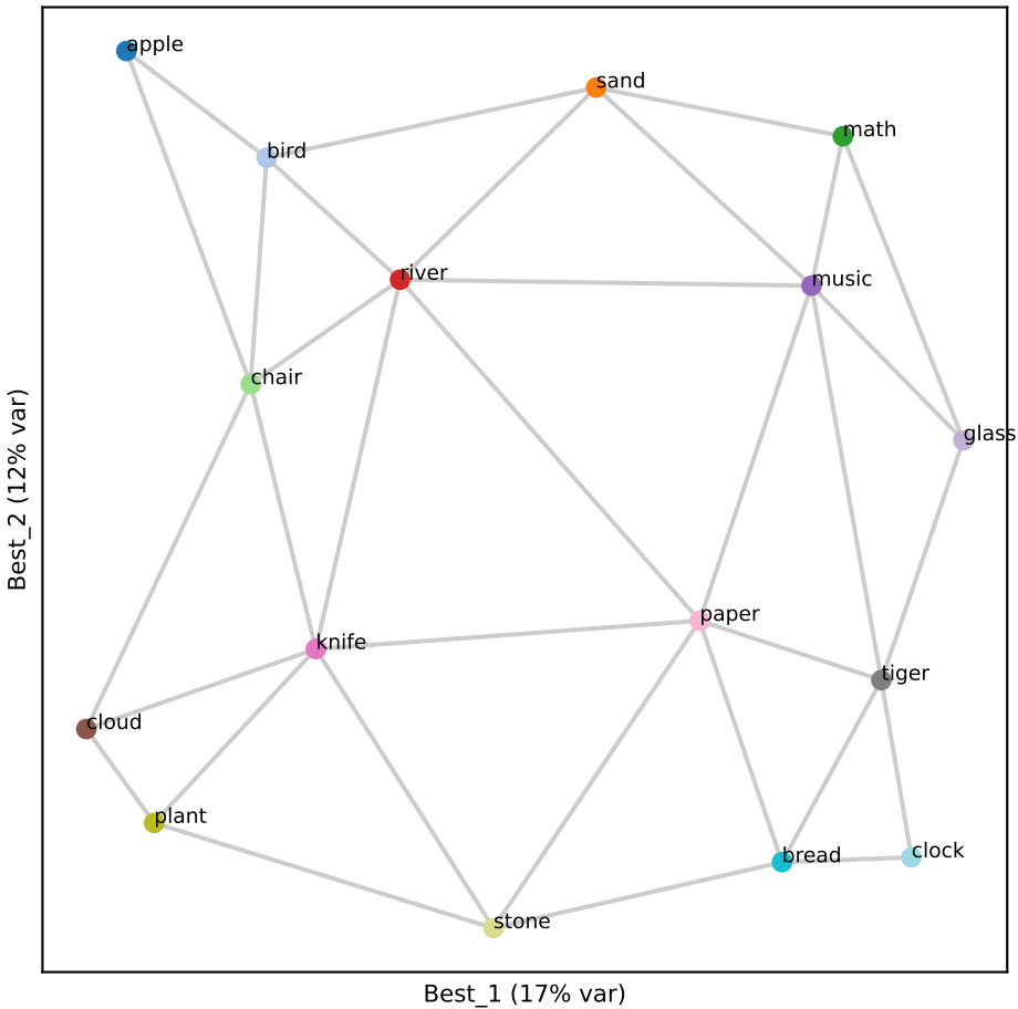
Llama L24 (RSA 0.89)
