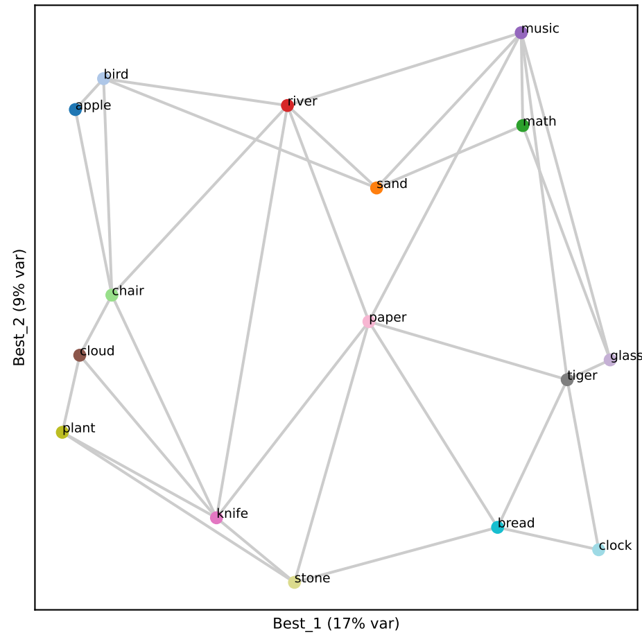
Gemma L20 (RSA 0.76)
