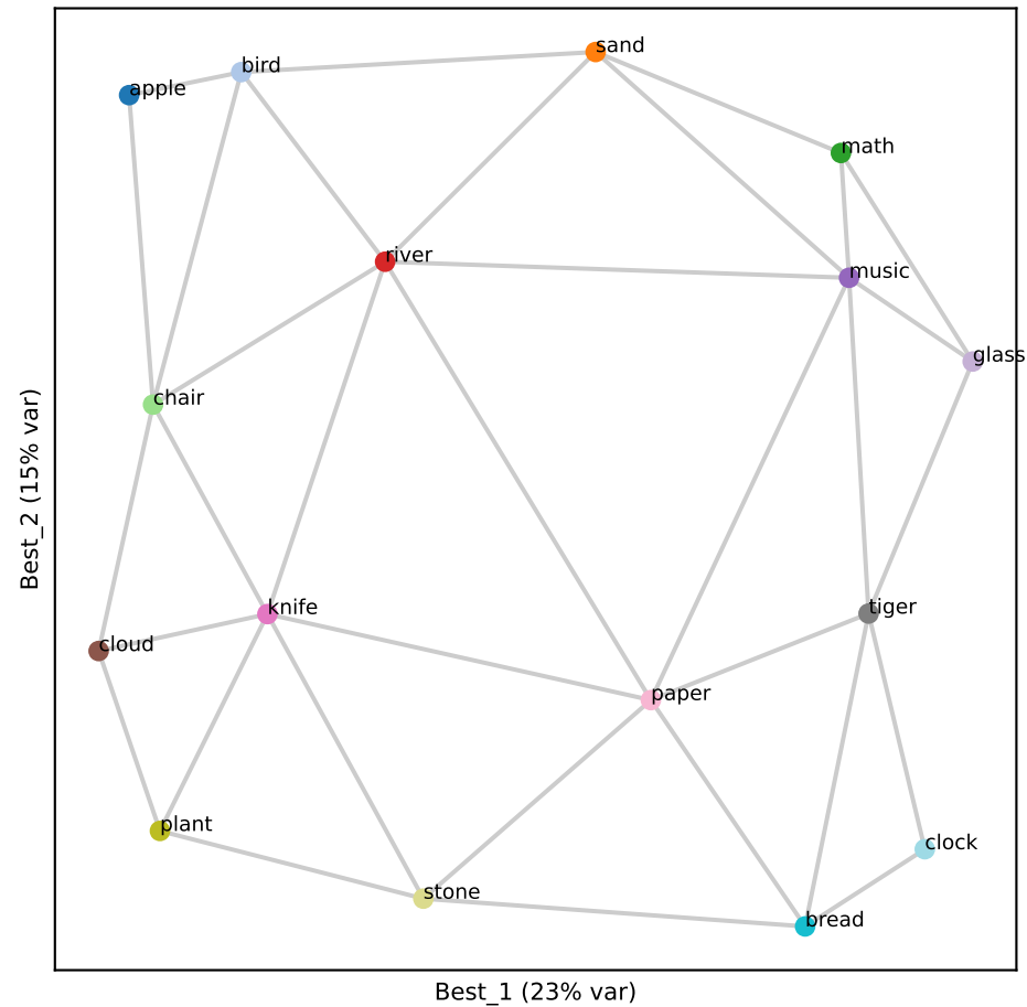
Gemma L37 (RSA 0.90)
