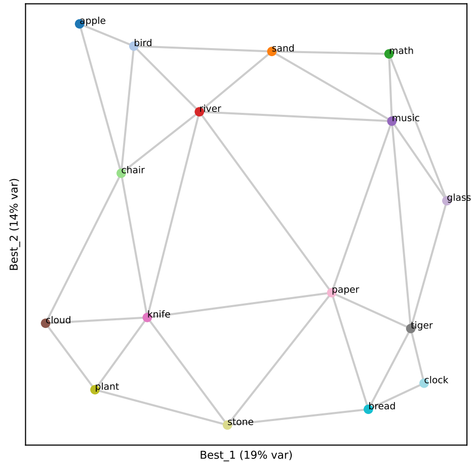
Llama L25 (RSA 0.88)
