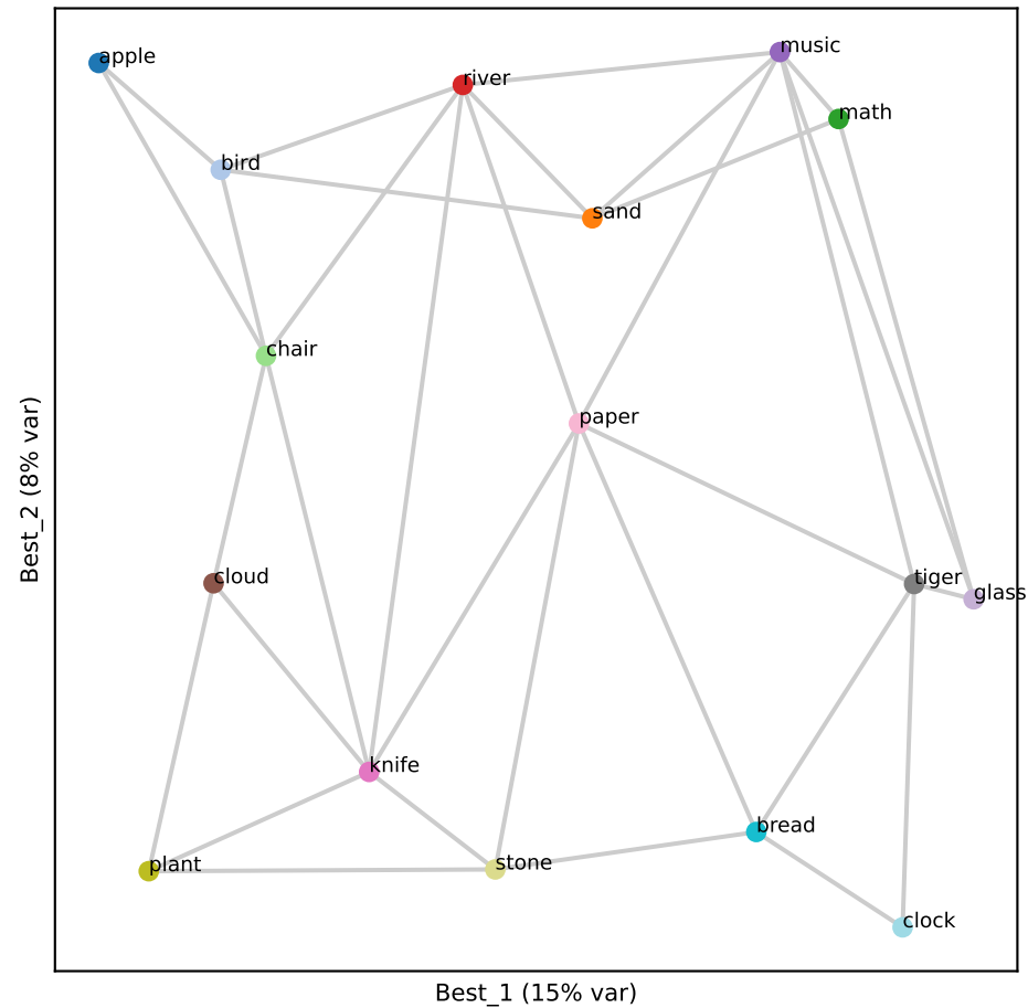
Gemma L27 (RSA 0.80)
