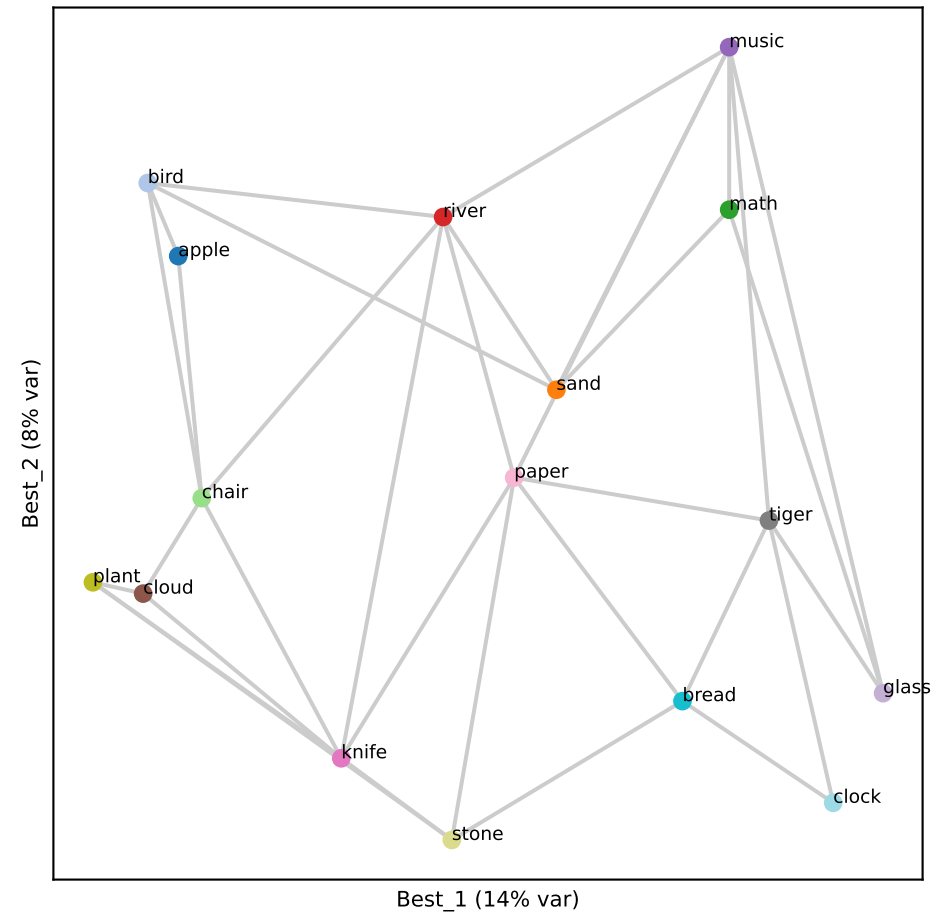
Gemma L19 (RSA 0.68)
