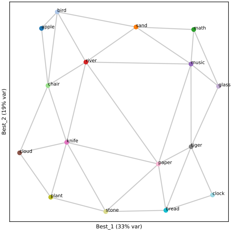
Llama L31 (RSA 0.87)
