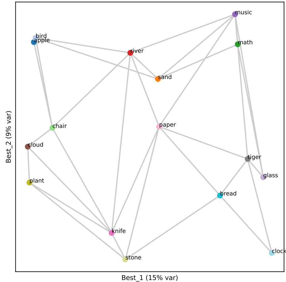
Gemma L16 (RSA 0.74)
