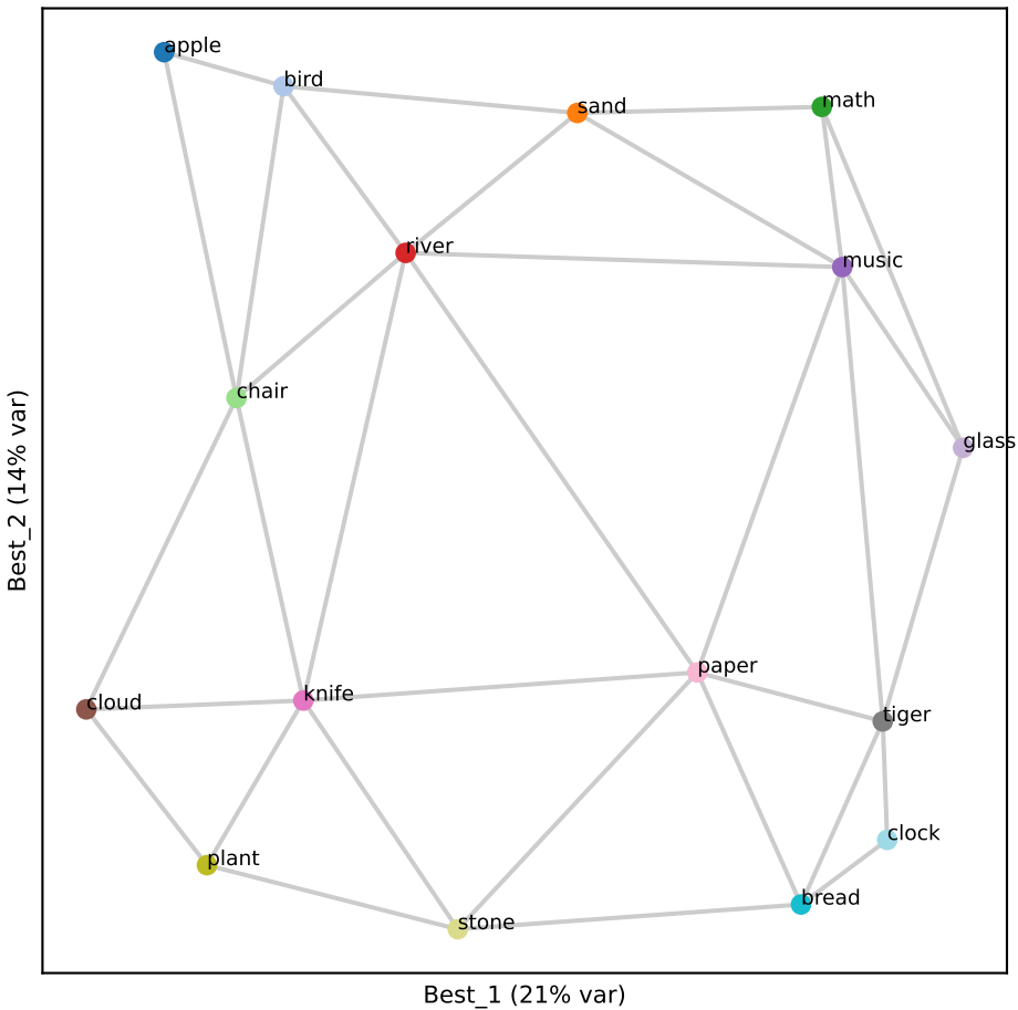
Llama L26 (RSA 0.88)
