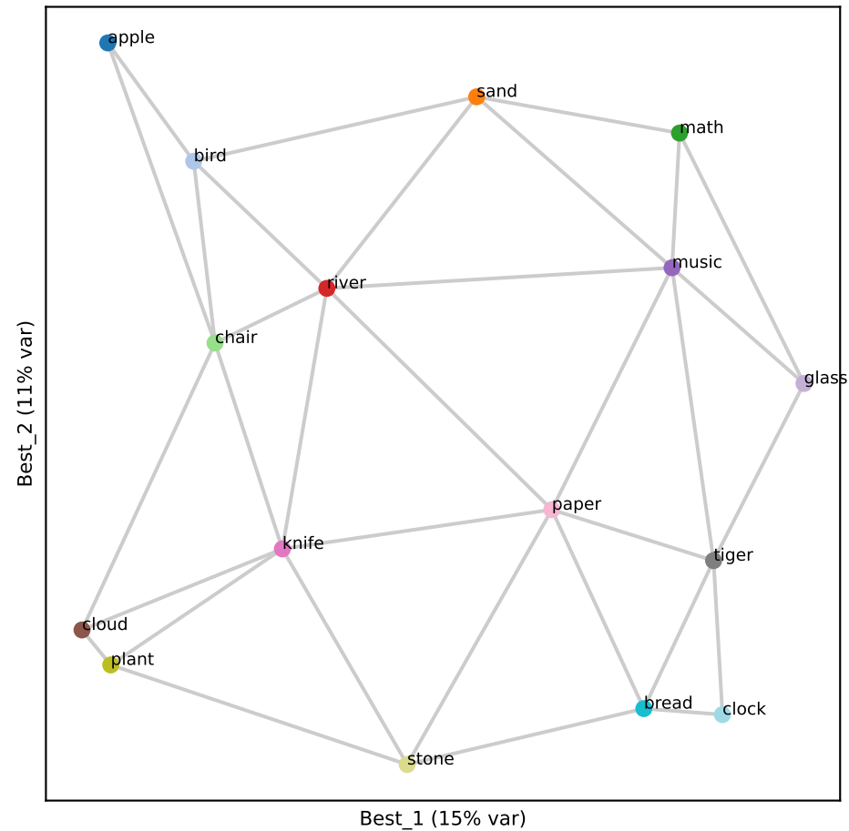
Llama L23 (RSA 0.89)
