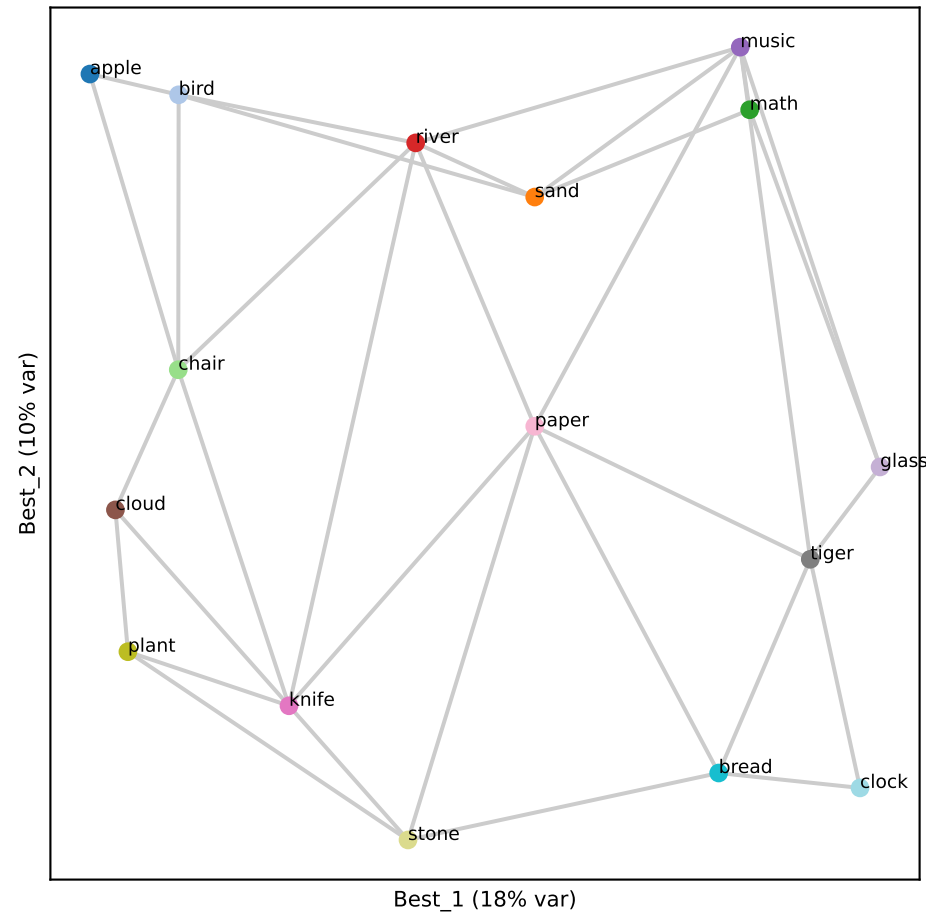
Gemma L23 (RSA 0.81)
