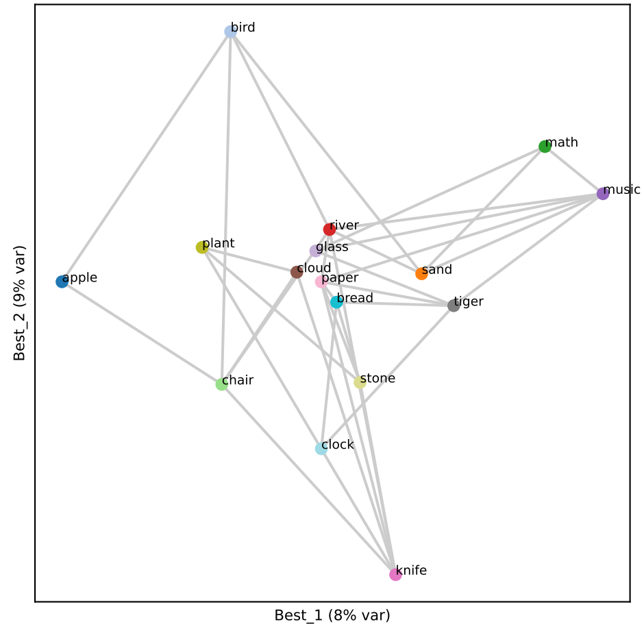
Qwen L5 (RSA 0.21)
