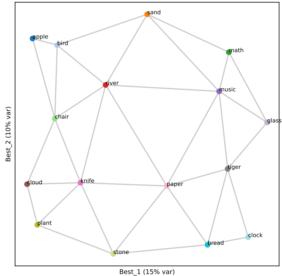
Gemma L34 (RSA 0.90)
