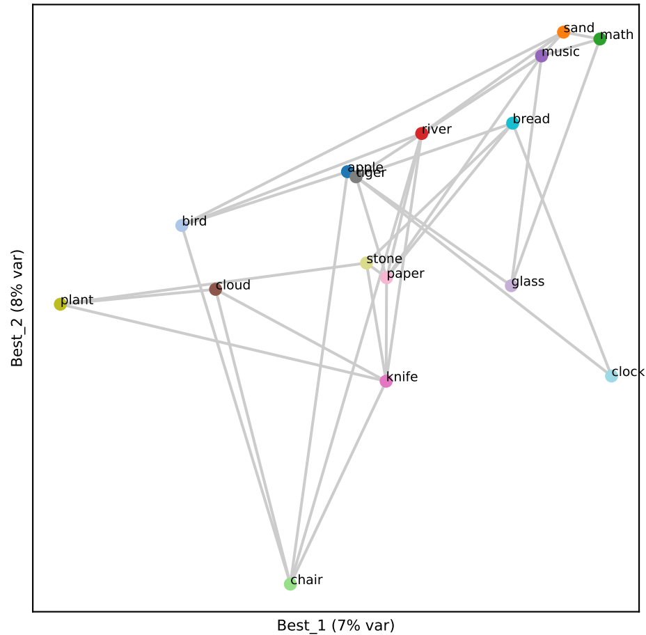
Gemma L0 (RSA 0.41)
