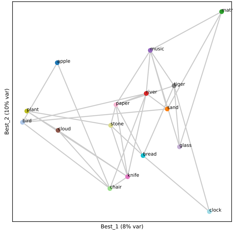
Gemma L8 (RSA 0.52)
