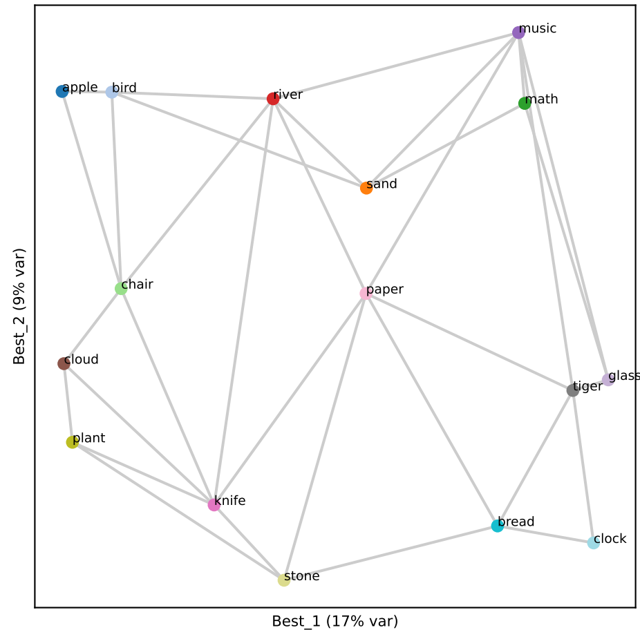
Gemma L24 (RSA 0.77)
