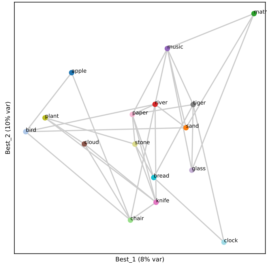
Gemma L9 (RSA 0.46)
