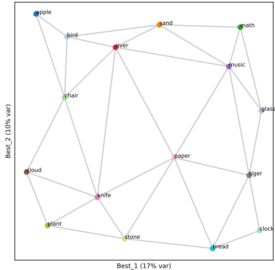
Gemma L29 (RSA 0.88)
