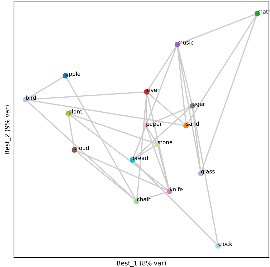
Gemma L6 (RSA 0.44)
