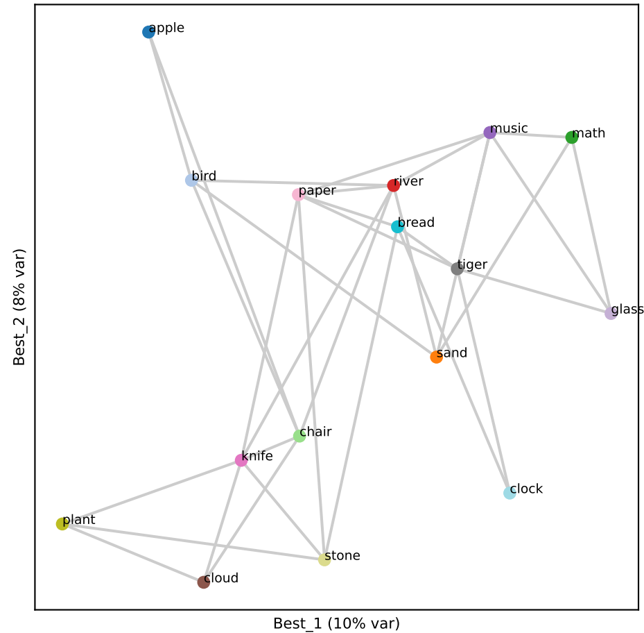
Llama L6 (RSA 0.62)
