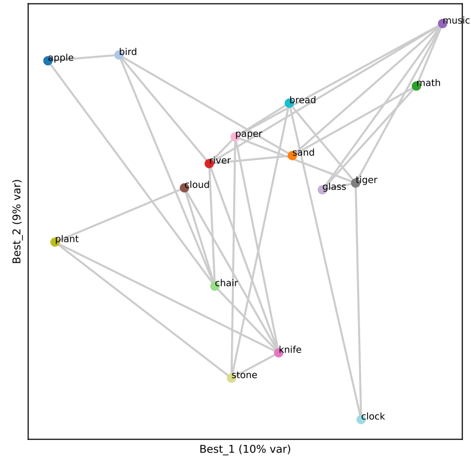
Qwen L16 (RSA 0.43)
