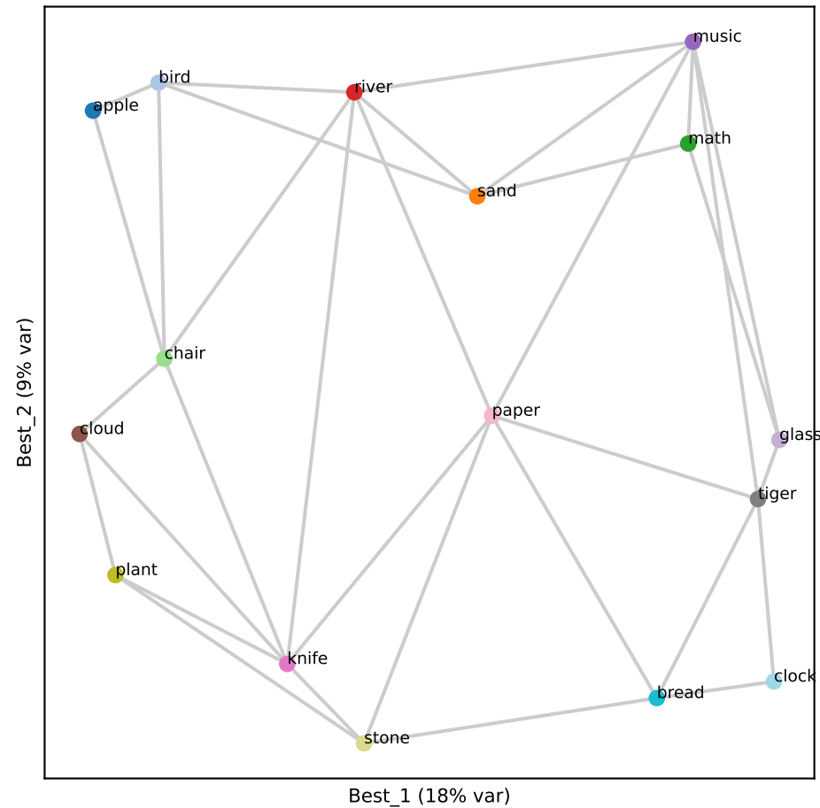
Gemma L25 (RSA 0.77)
