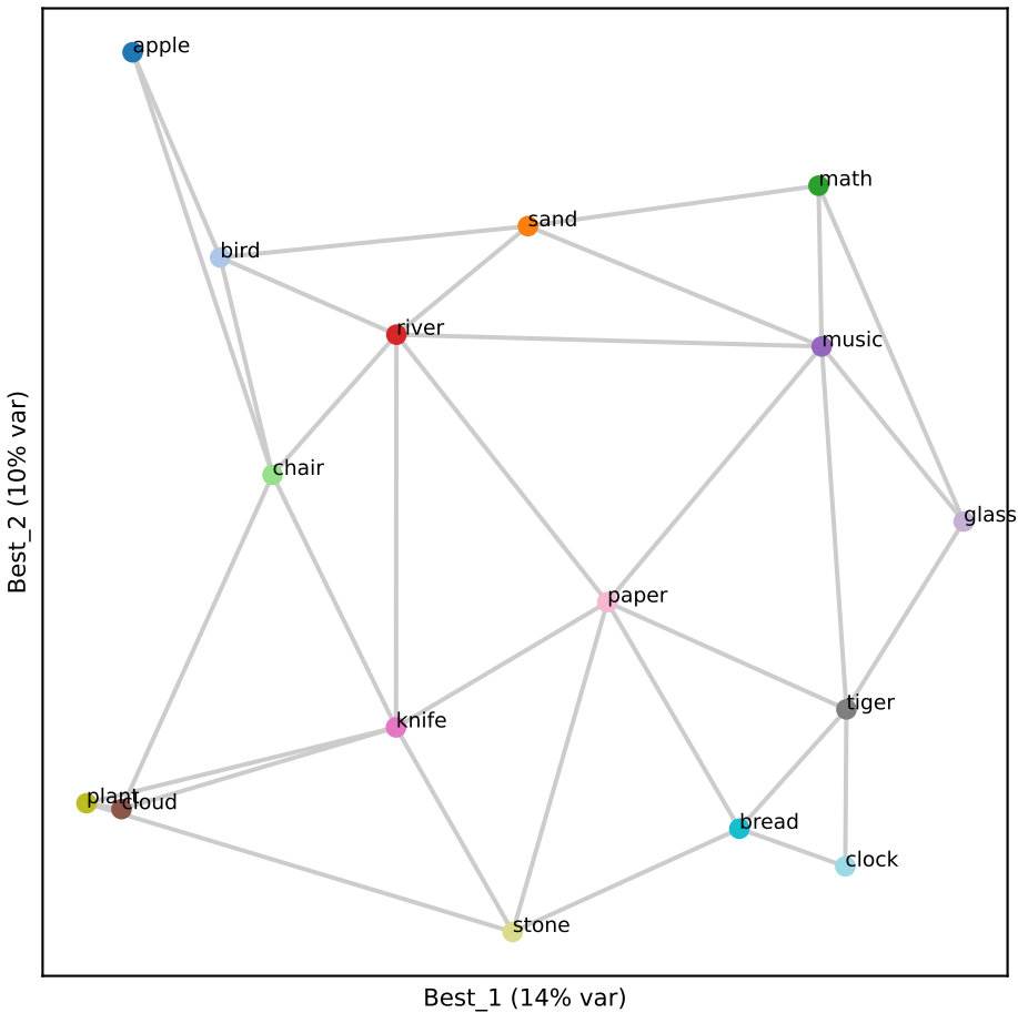
Llama L19 (RSA 0.86)
