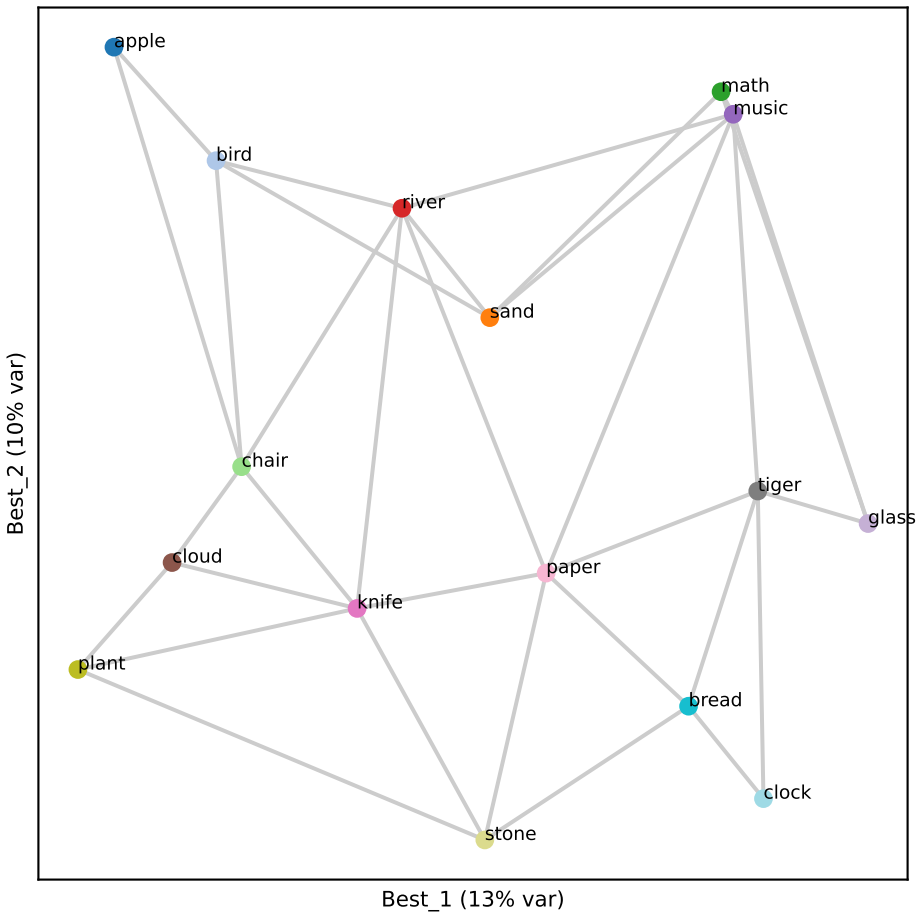
Llama L15 (RSA 0.78)
