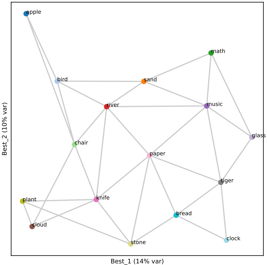
Llama L18 (RSA 0.85)
