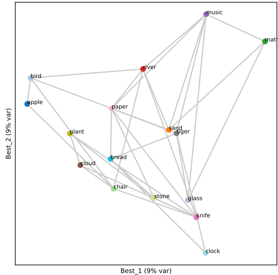
Gemma L12 (RSA 0.33)
