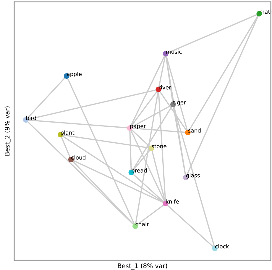
Gemma L5 (RSA 0.42)
