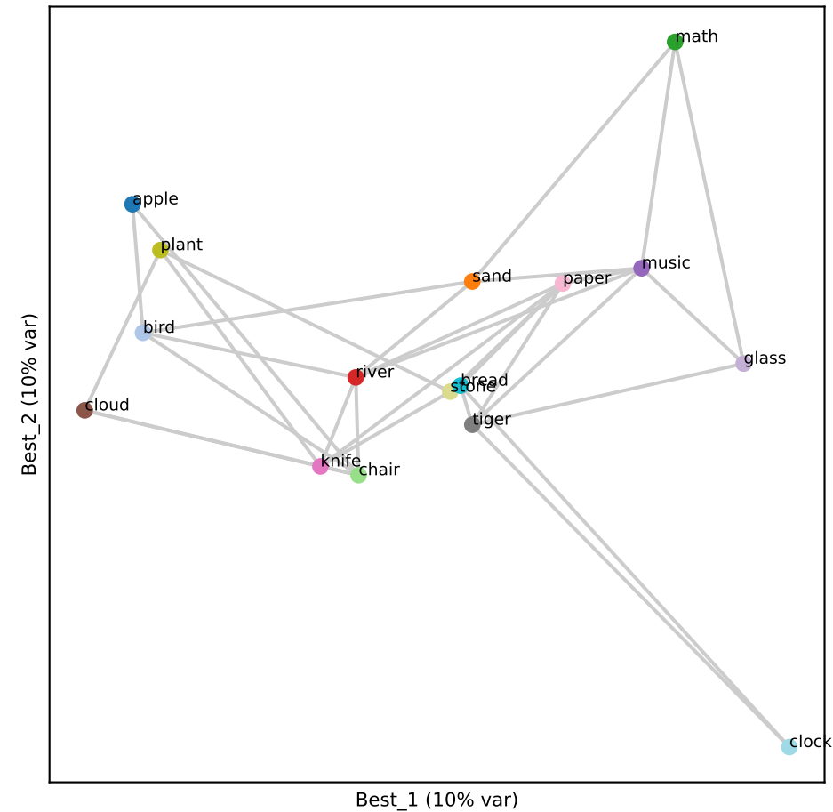
Qwen L25 (RSA 0.54)
