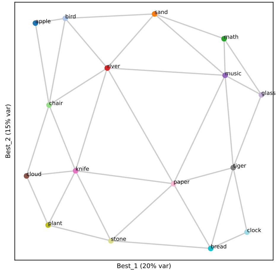
Gemma L36 (RSA 0.90)
