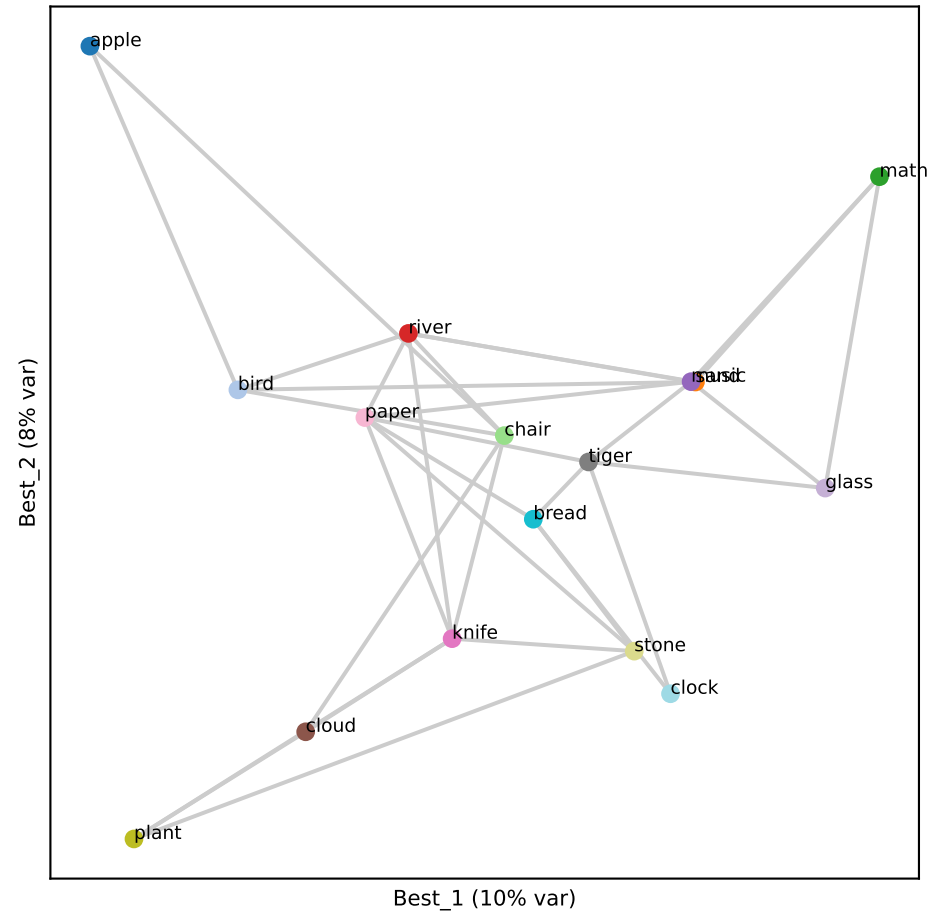
Llama L4 (RSA 0.53)
