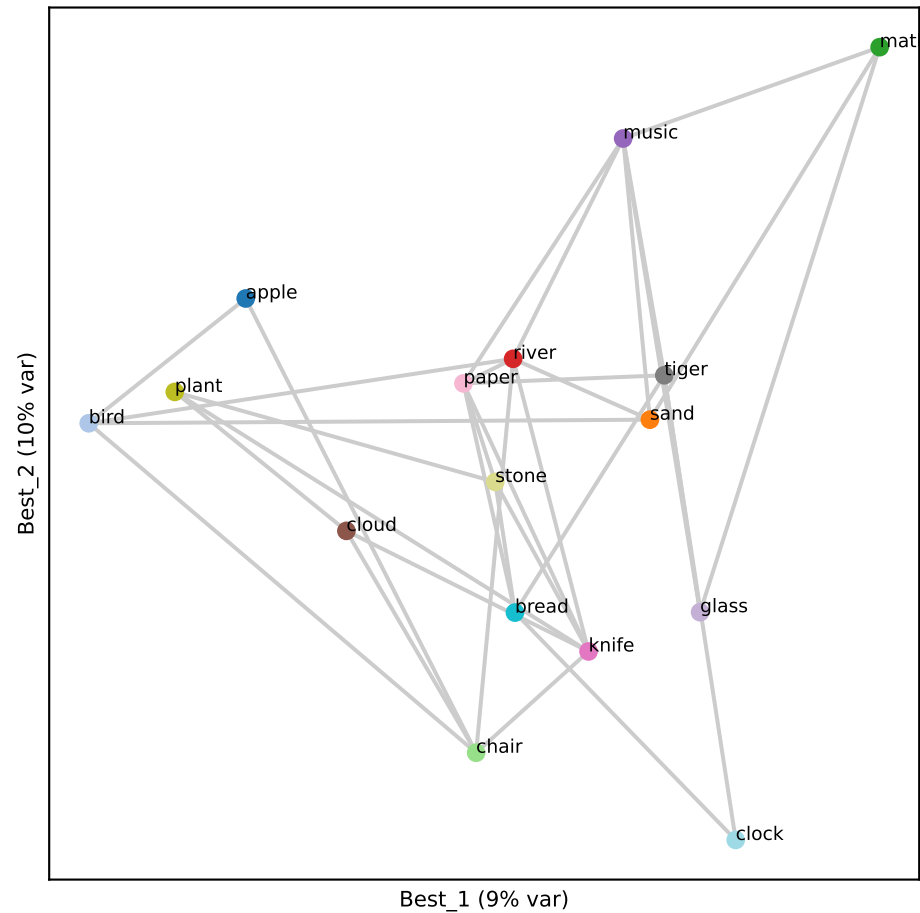
Gemma L11 (RSA 0.44)
