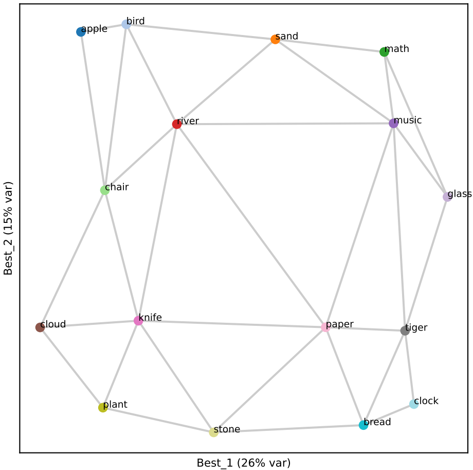
Llama L29 (RSA 0.88)
