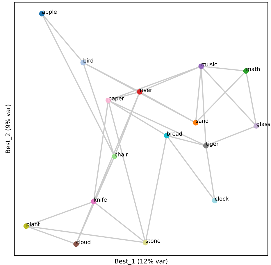
Llama L7 (RSA 0.66)
