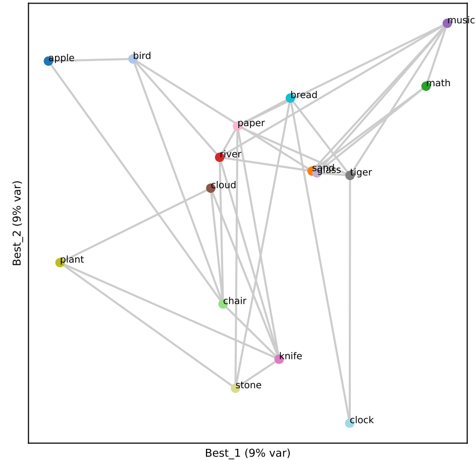
Qwen L14 (RSA 0.41)
