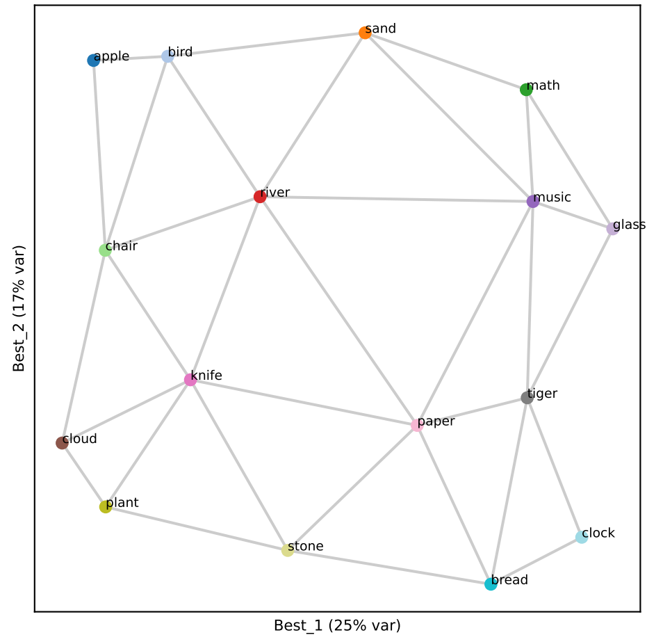
Gemma L41 (RSA 0.90)
