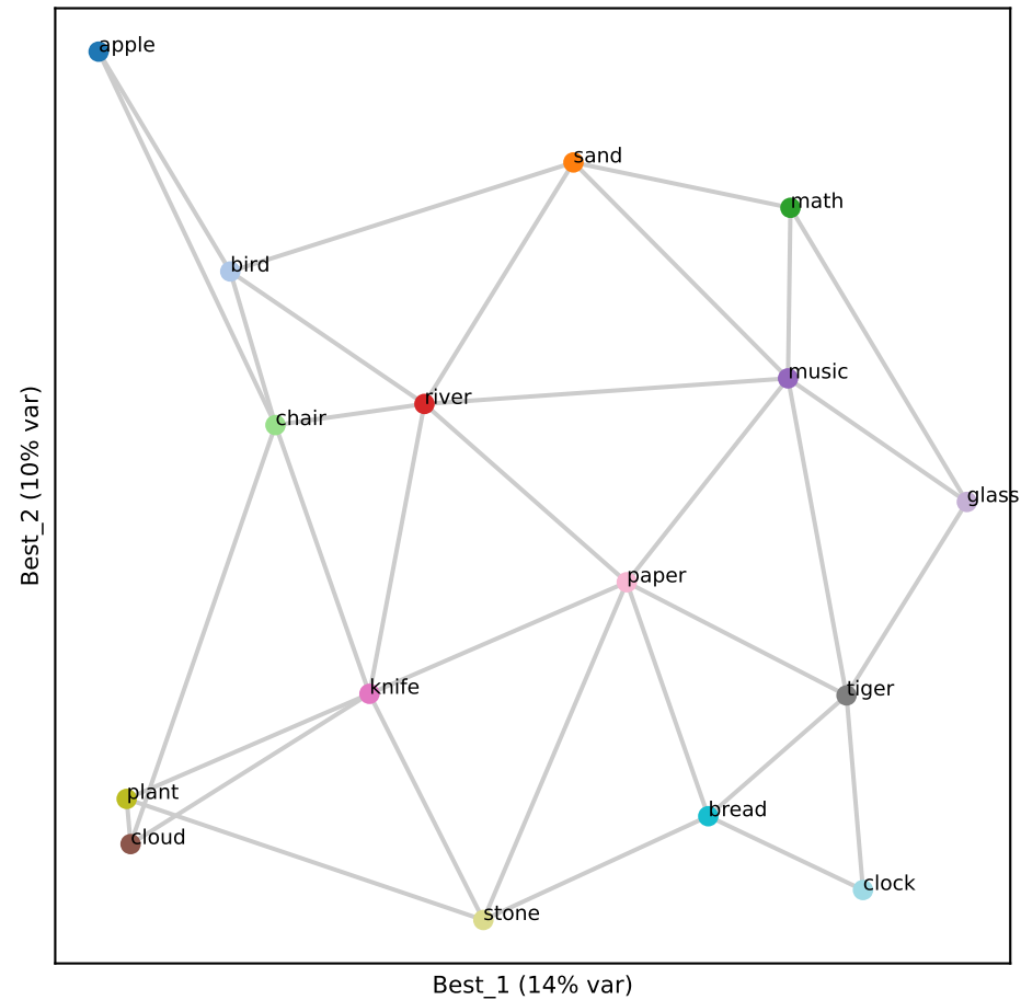
Llama L22 (RSA 0.88)
