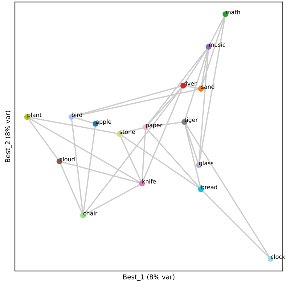
Gemma L3 (RSA 0.55)
