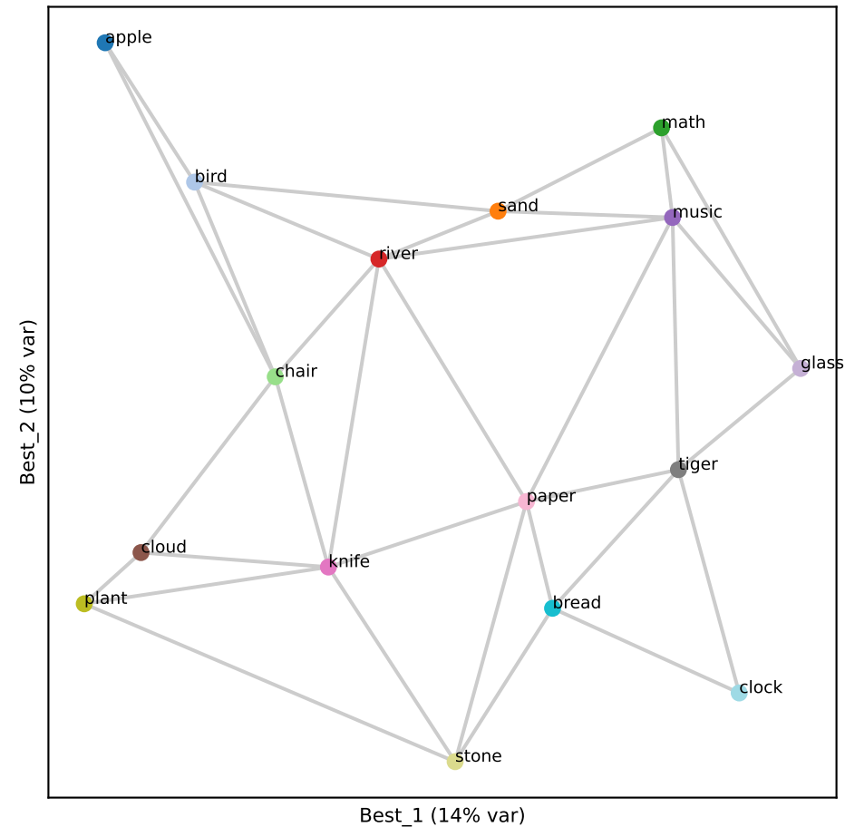
Llama L16 (RSA 0.84)
