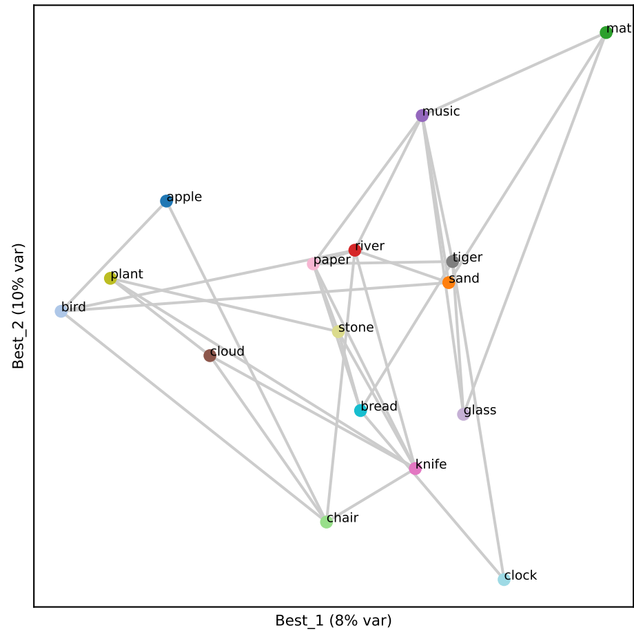
Gemma L10 (RSA 0.43)
