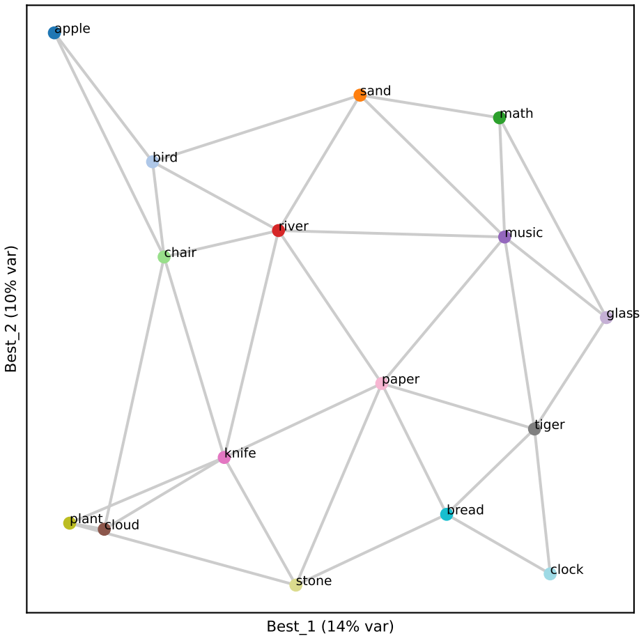
Llama L21 (RSA 0.89)
