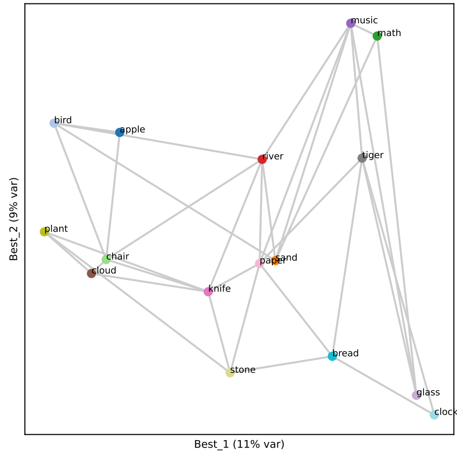
Gemma L15 (RSA 0.63)
