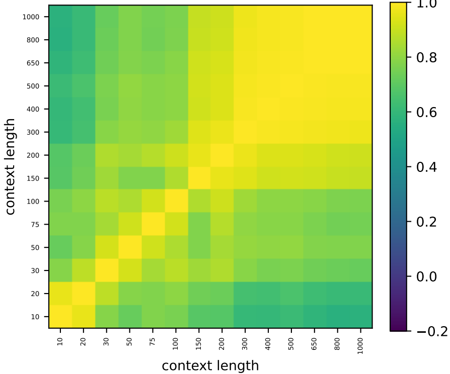
Gemma L33 perm-null 95%
