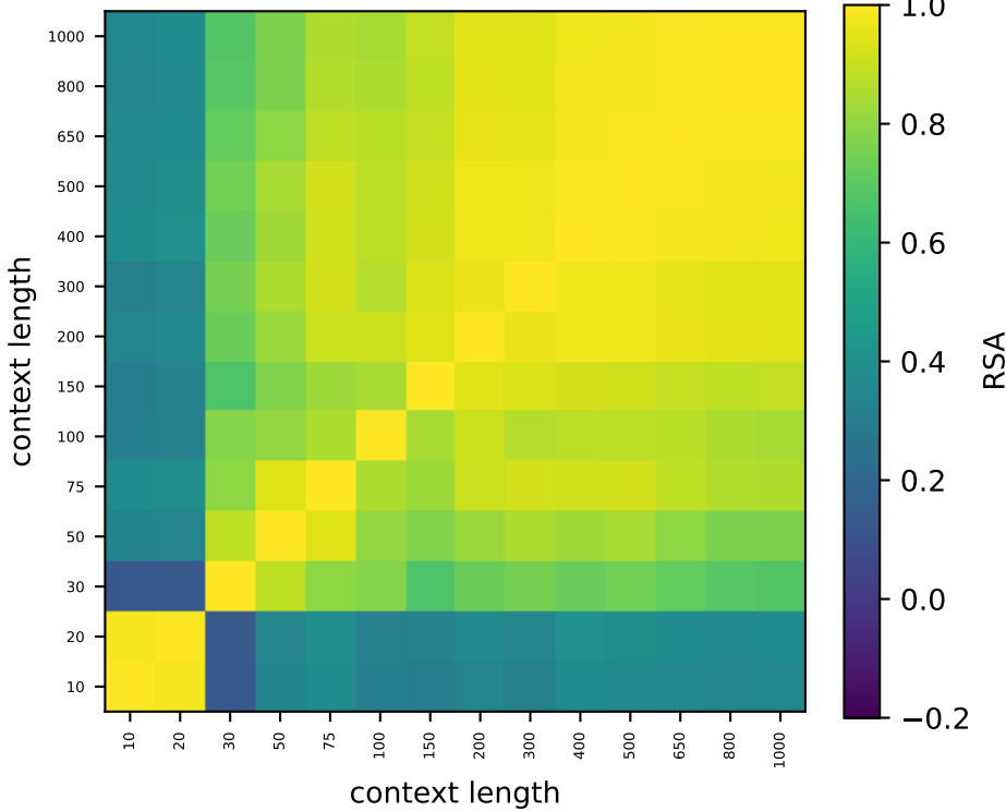
Qwen L23
