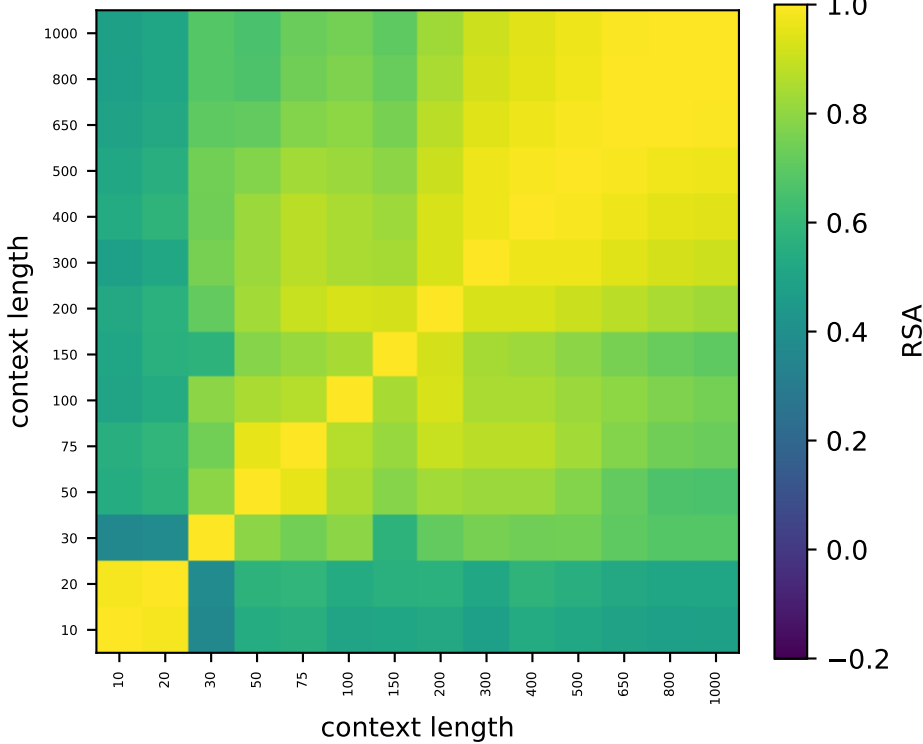
Qwen L30
