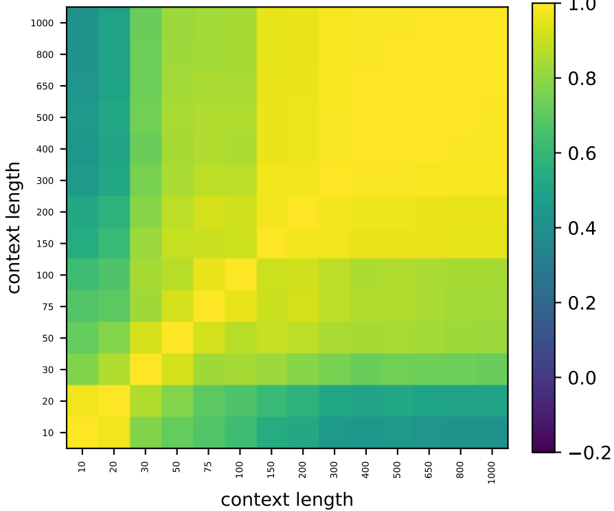
Gemma L38
