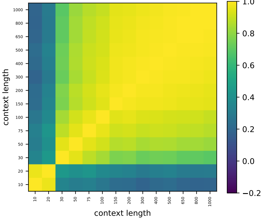
Gemma L19
