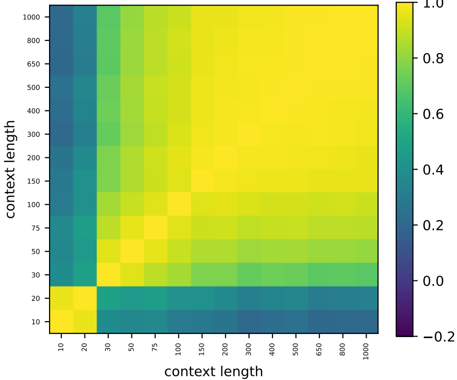
Gemma L18
