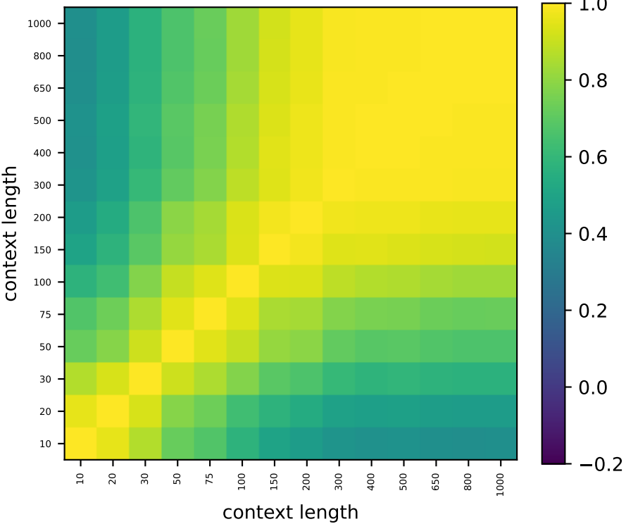
Llama L29
