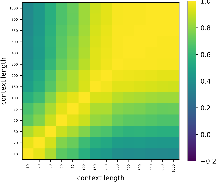
Llama L28
