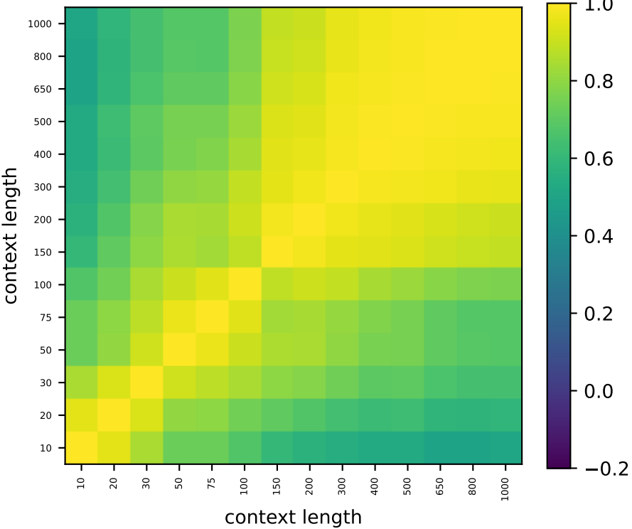
Llama L23
