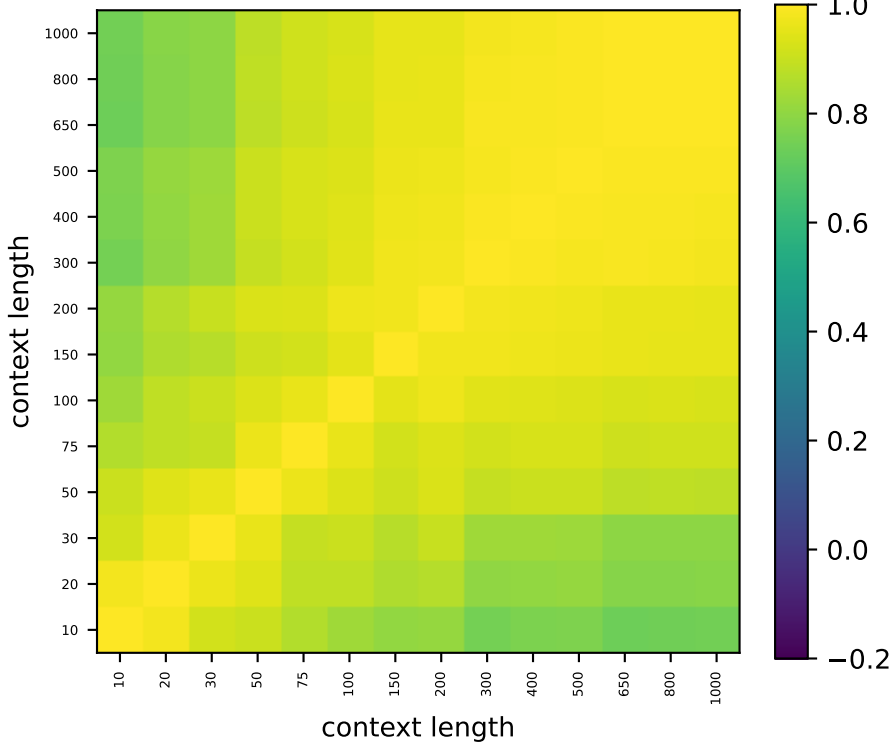
Gemma L27
