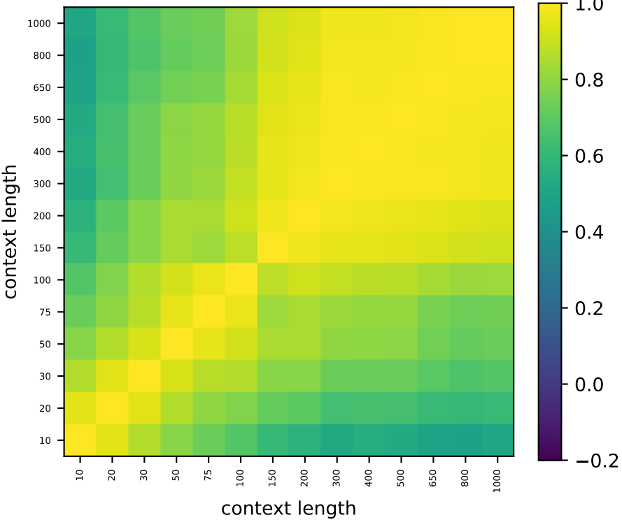
Llama L17
