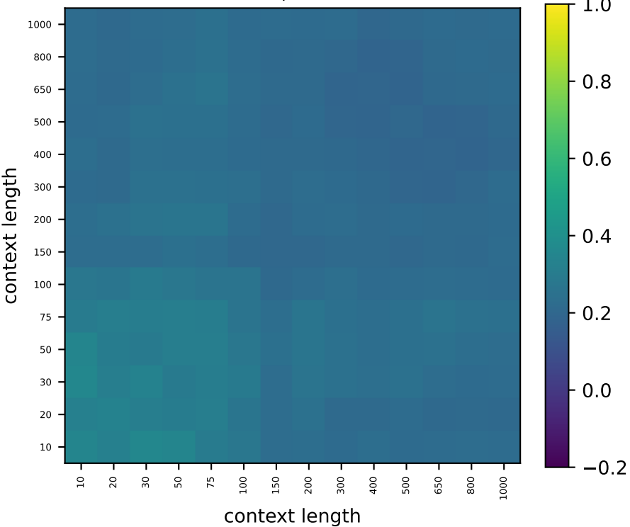
Llama L22 perm-null 95%
