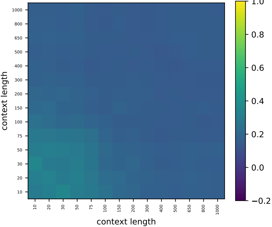
Llama L28 perm-null 95%
