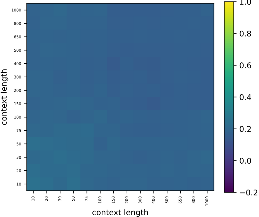
Llama L15 perm-null 95%
