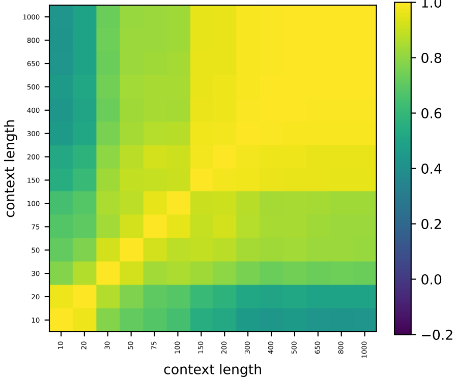
Gemma L37
