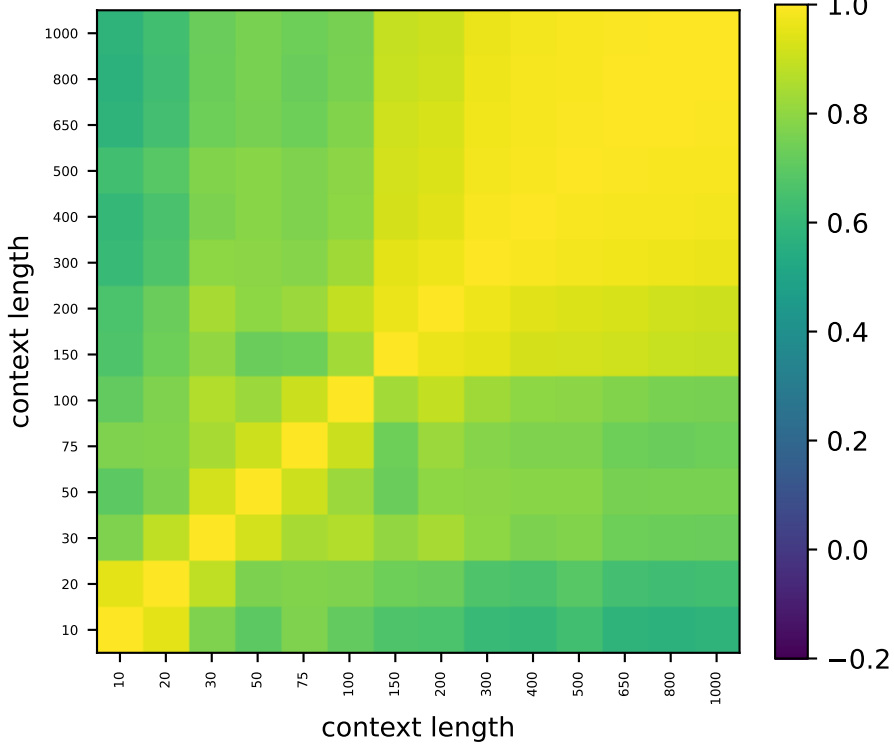
Gemma L31
