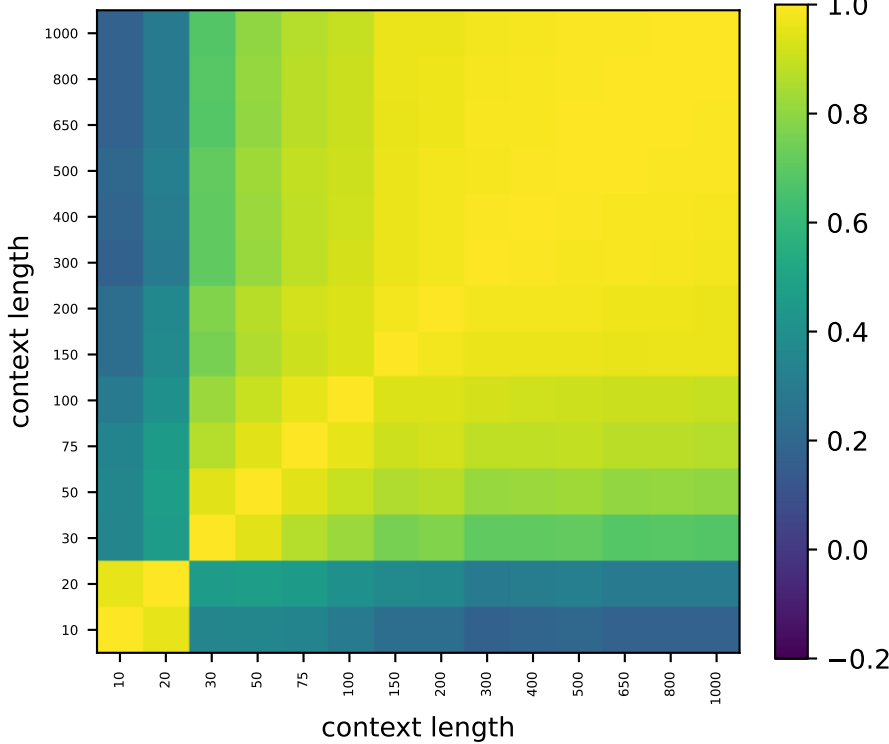
Gemma L22
