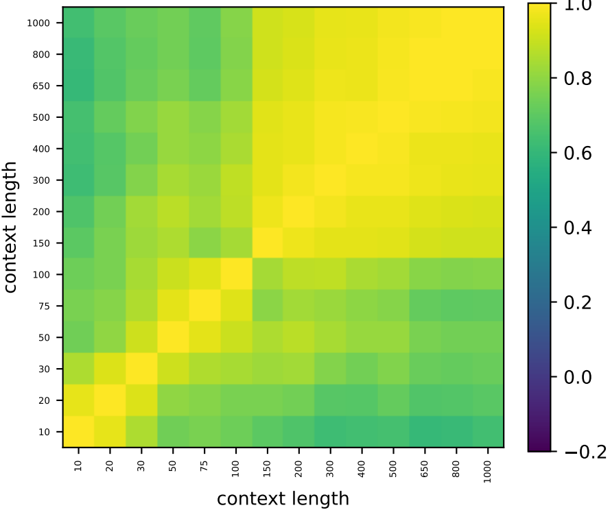
Llama L20
