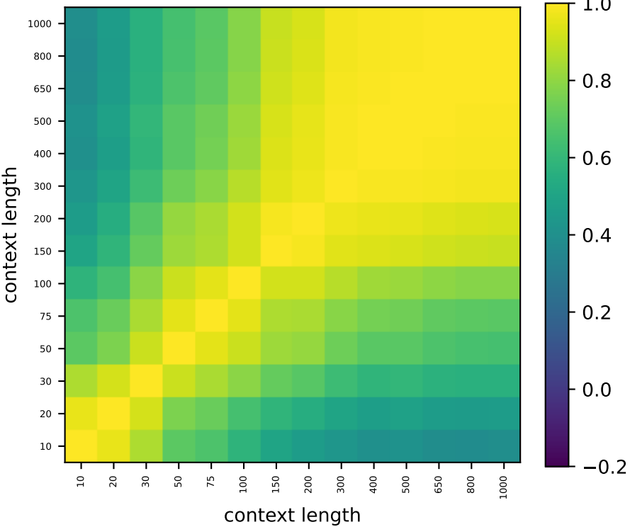
Llama L26
