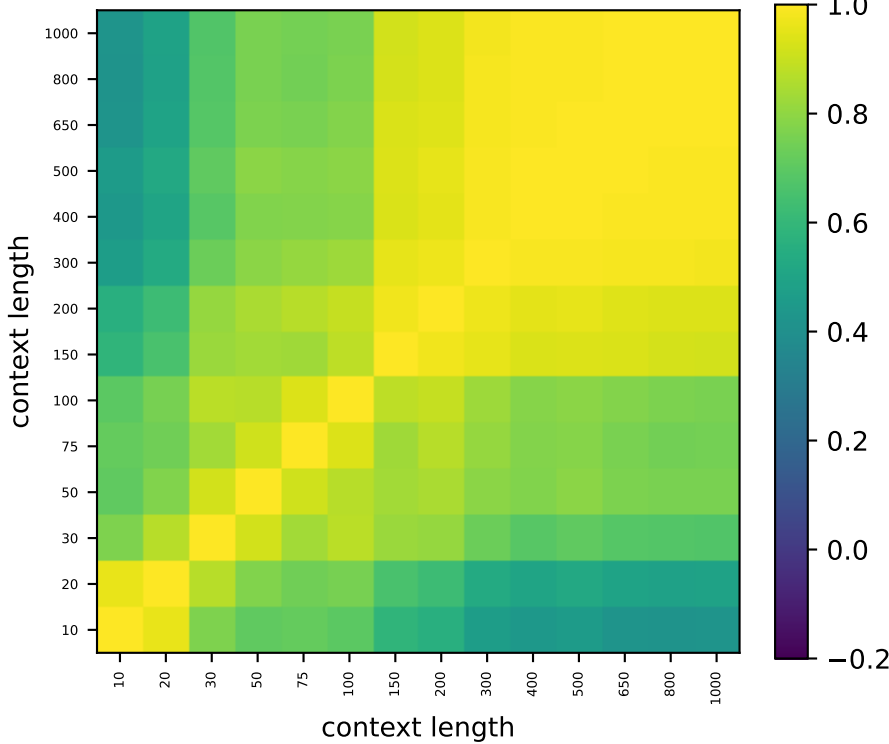
Gemma L35
