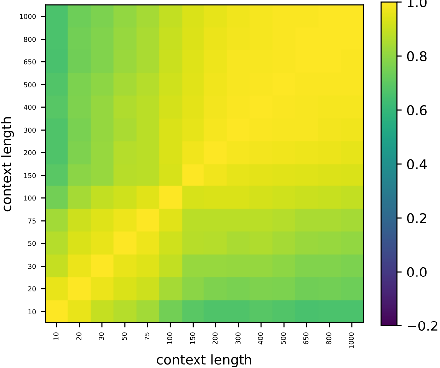
Llama L14
