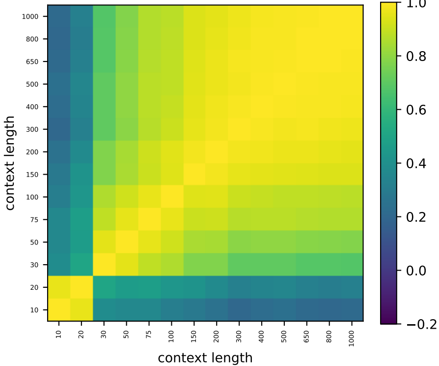
Gemma L17 perm-null 95%
