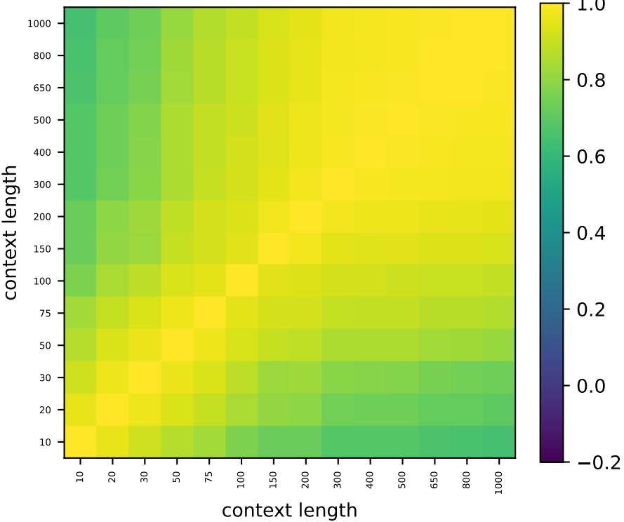
Llama L12 perm-null 95%
