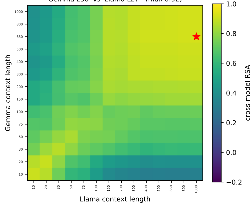
Gemma L36 vs Llama L27 (max 0.92)
