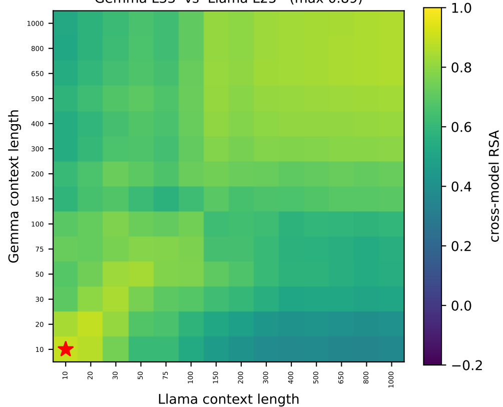
Gemma L33 vs Llama L25 (max 0.89)
