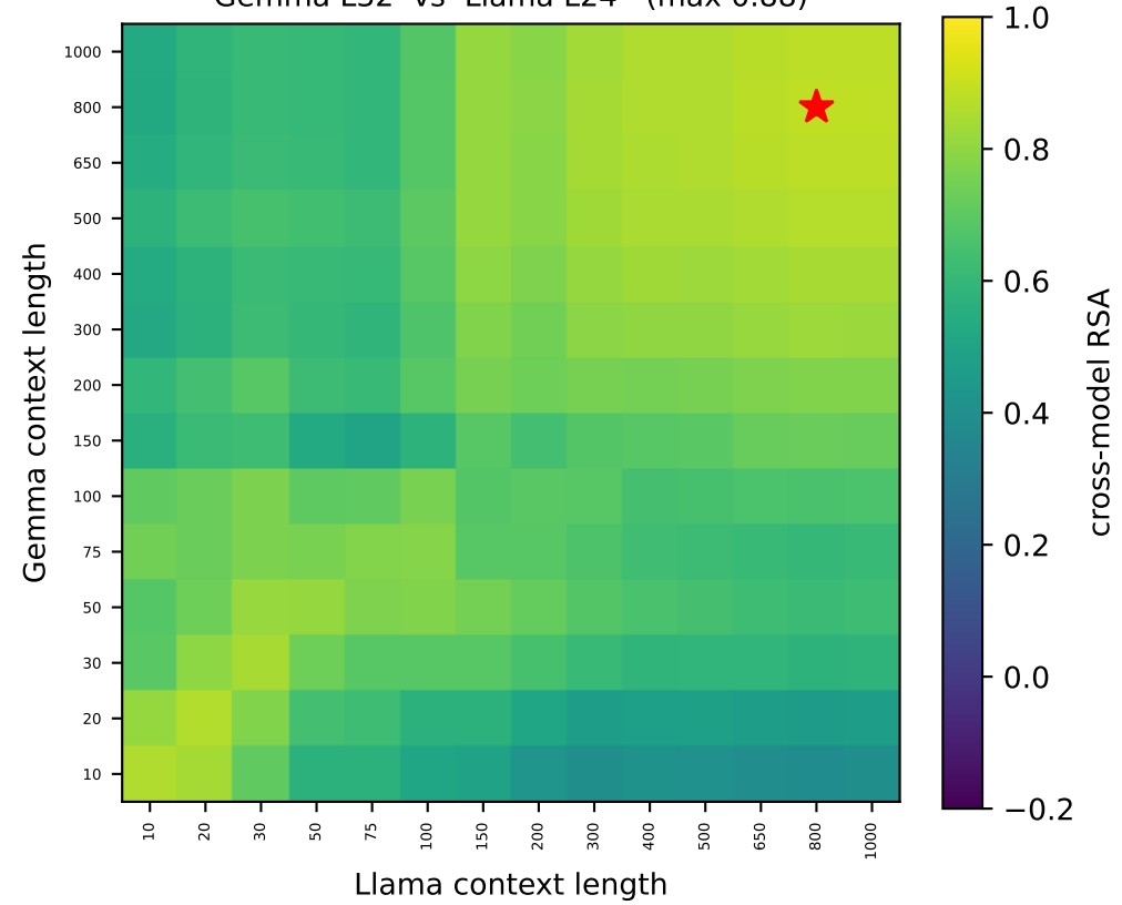
Gemma L32 vs Llama L24 (max 0.88)
