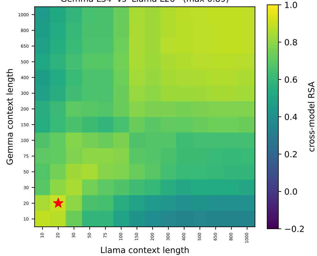
Gemma L34 vs Llama L26 (max 0.89)
