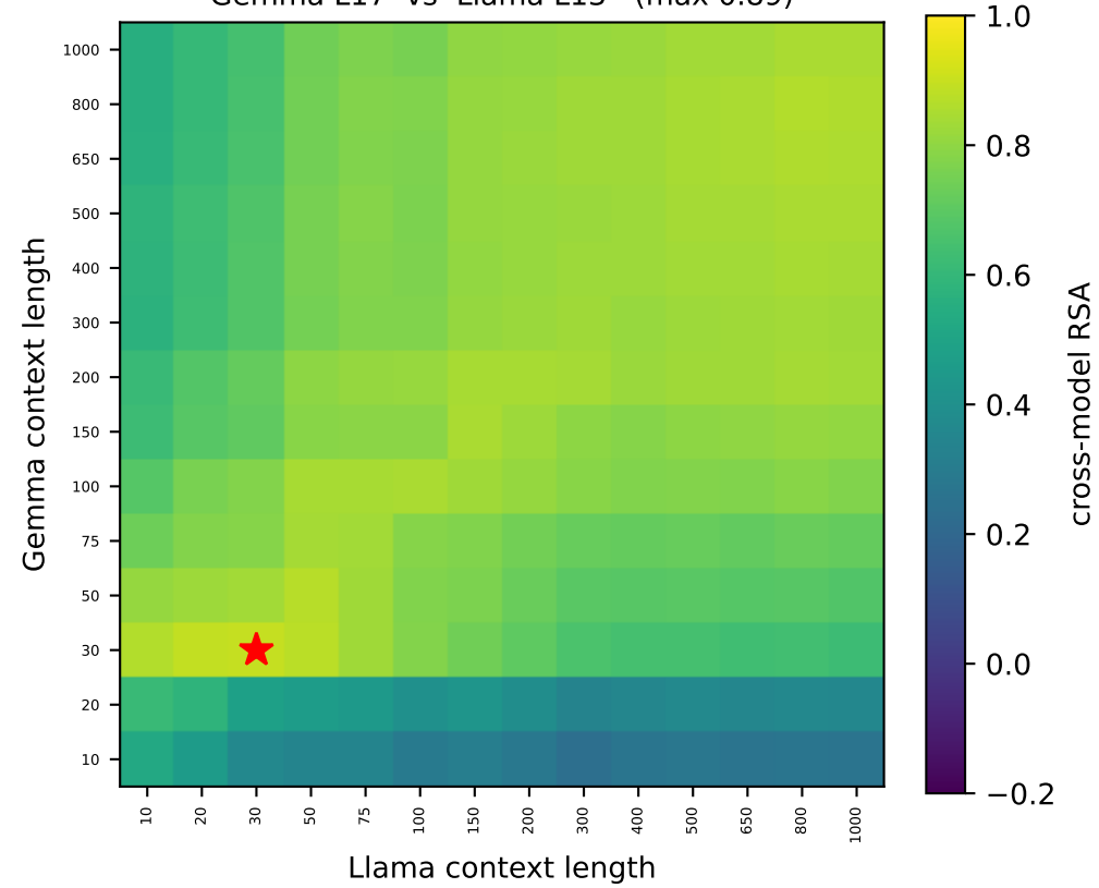
Gemma L17 vs Llama L13 (max 0.89)
