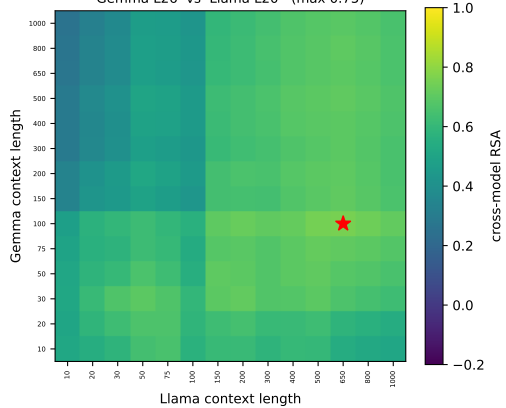
Gemma L26 vs Llama L20 (max 0.75)
