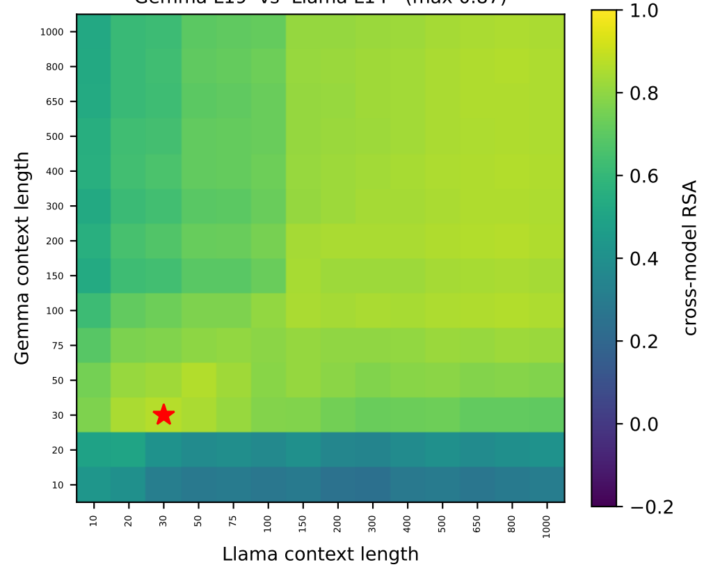
Gemma L19 vs Llama L14 (max 0.87)
