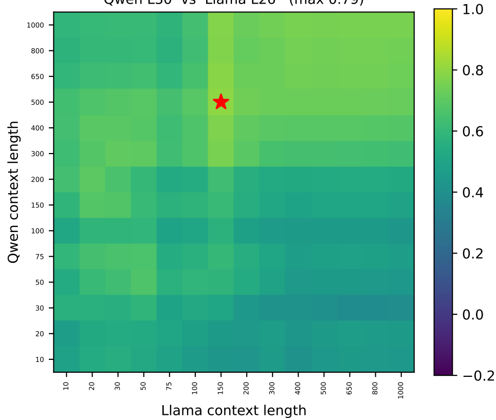
Qwen L30 vs Llama L26 (max 0.79)
