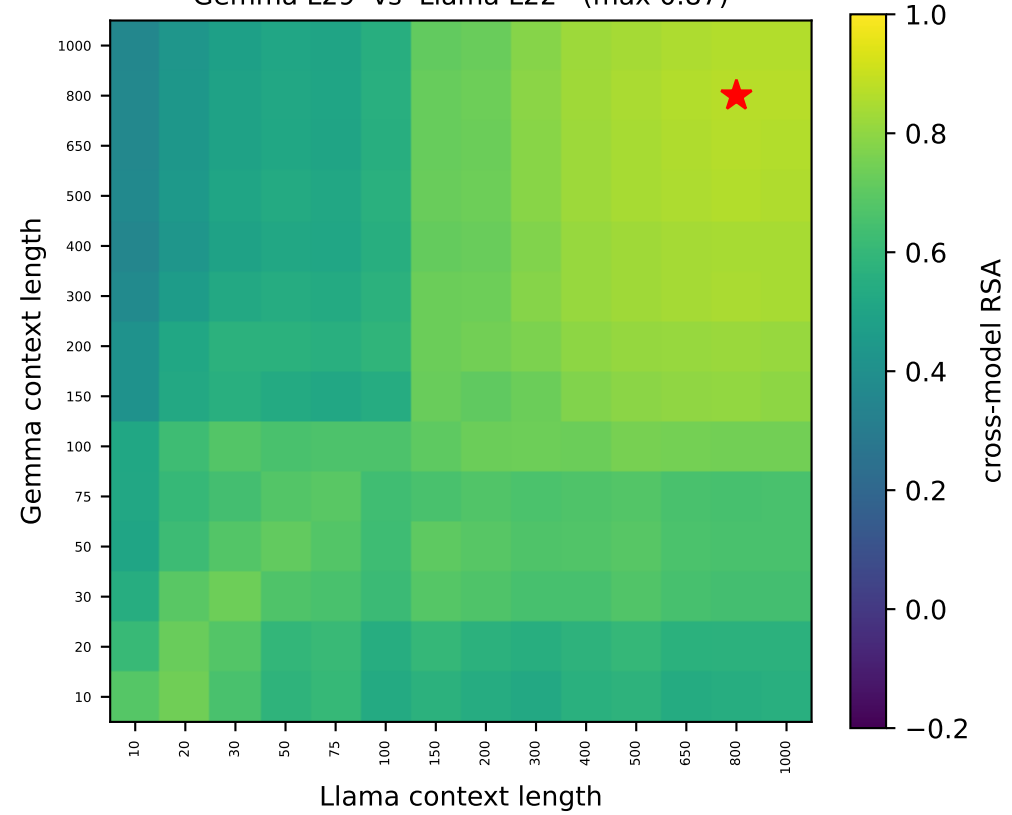
Gemma L29 vs Llama L22 (max 0.87)
