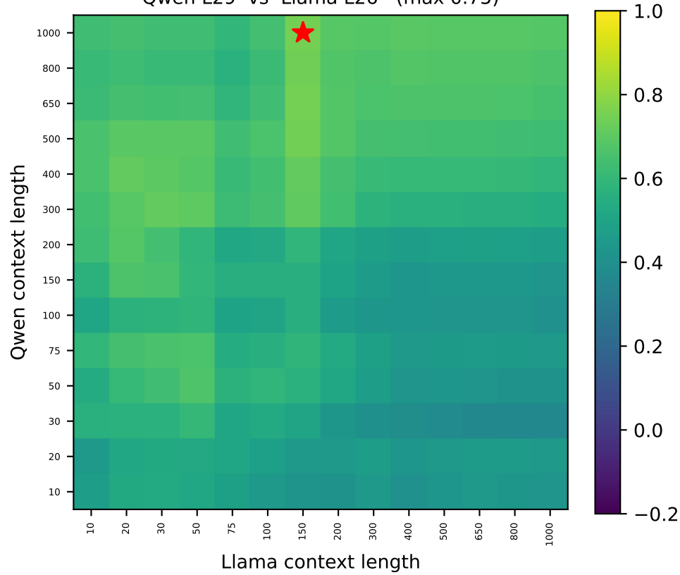
Qwen L29 vs Llama L26 (max 0.75)
