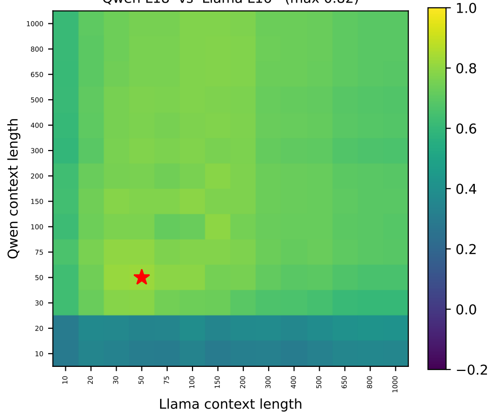
Qwen L18 vs Llama L16 (max 0.82)
