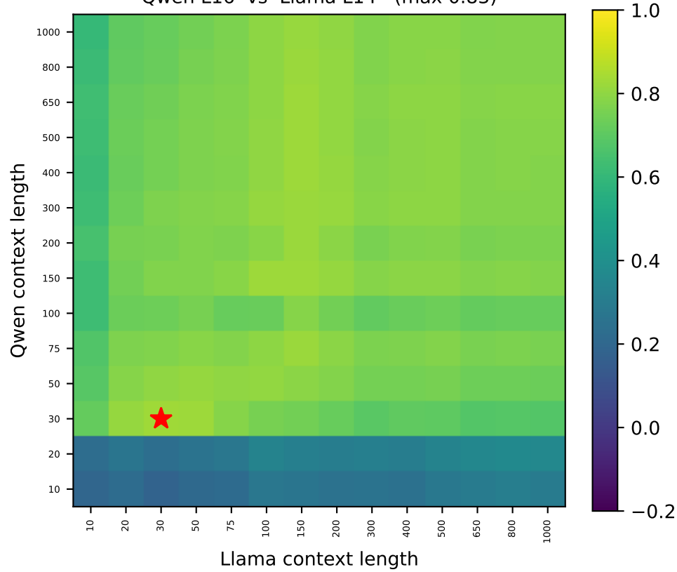
Qwen L16 vs Llama L14 (max 0.83)
