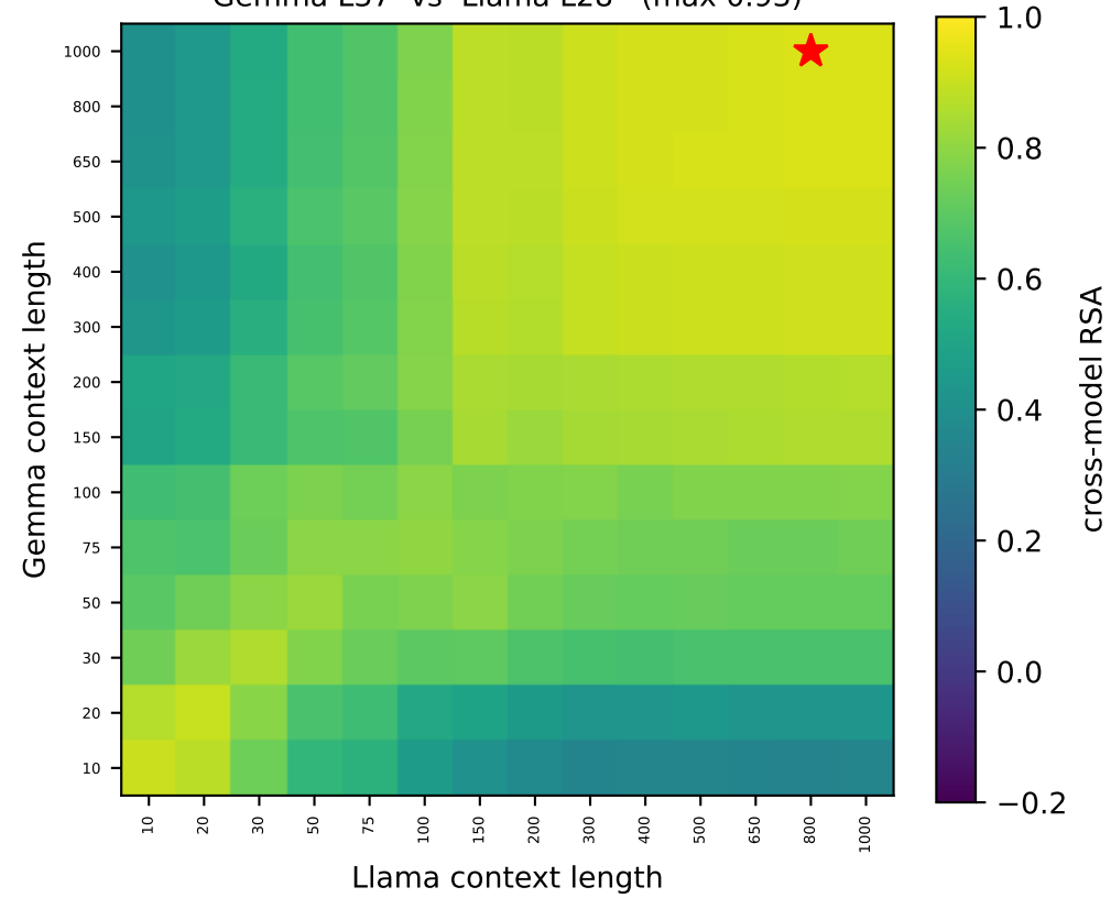
Gemma L37 vs Llama L28 (max 0.93)
