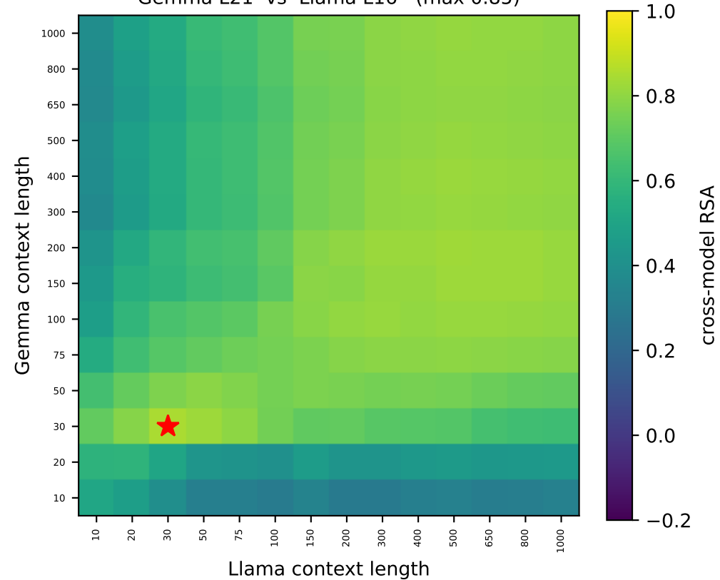
Gemma L21 vs Llama L16 (max 0.85)
