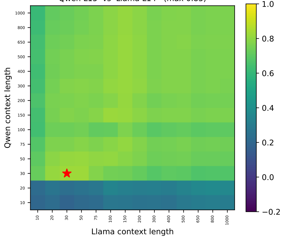
Qwen L15 vs Llama L14 (max 0.83)
