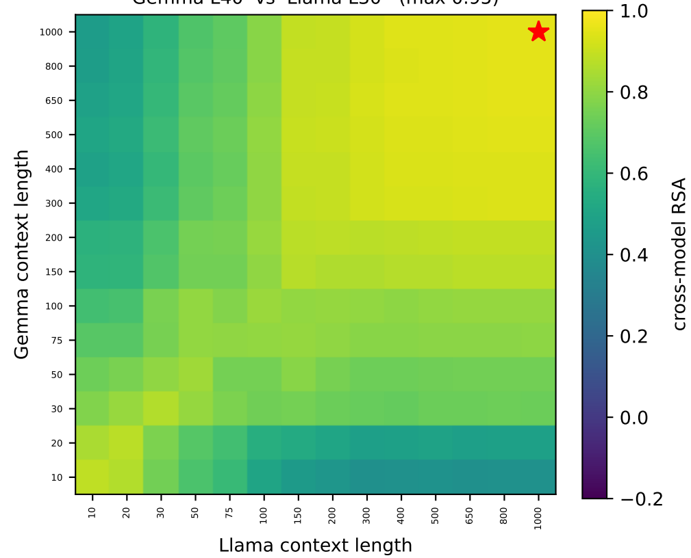
Gemma L40 vs Llama L30 (max 0.95)
