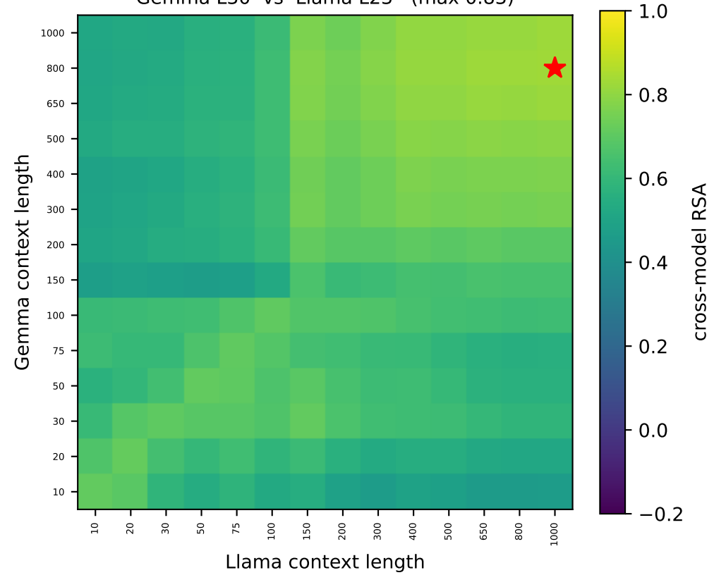
Gemma L30 vs Llama L23 (max 0.83)
