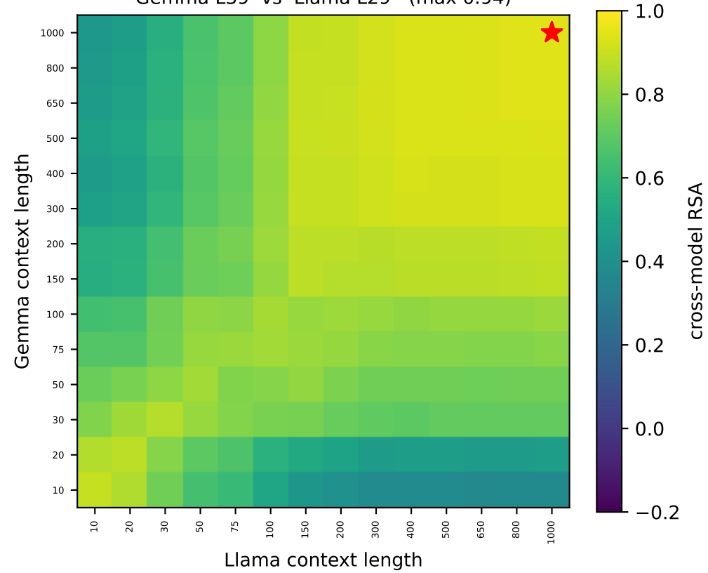
Gemma L39 vs Llama L29 (max 0.94)
