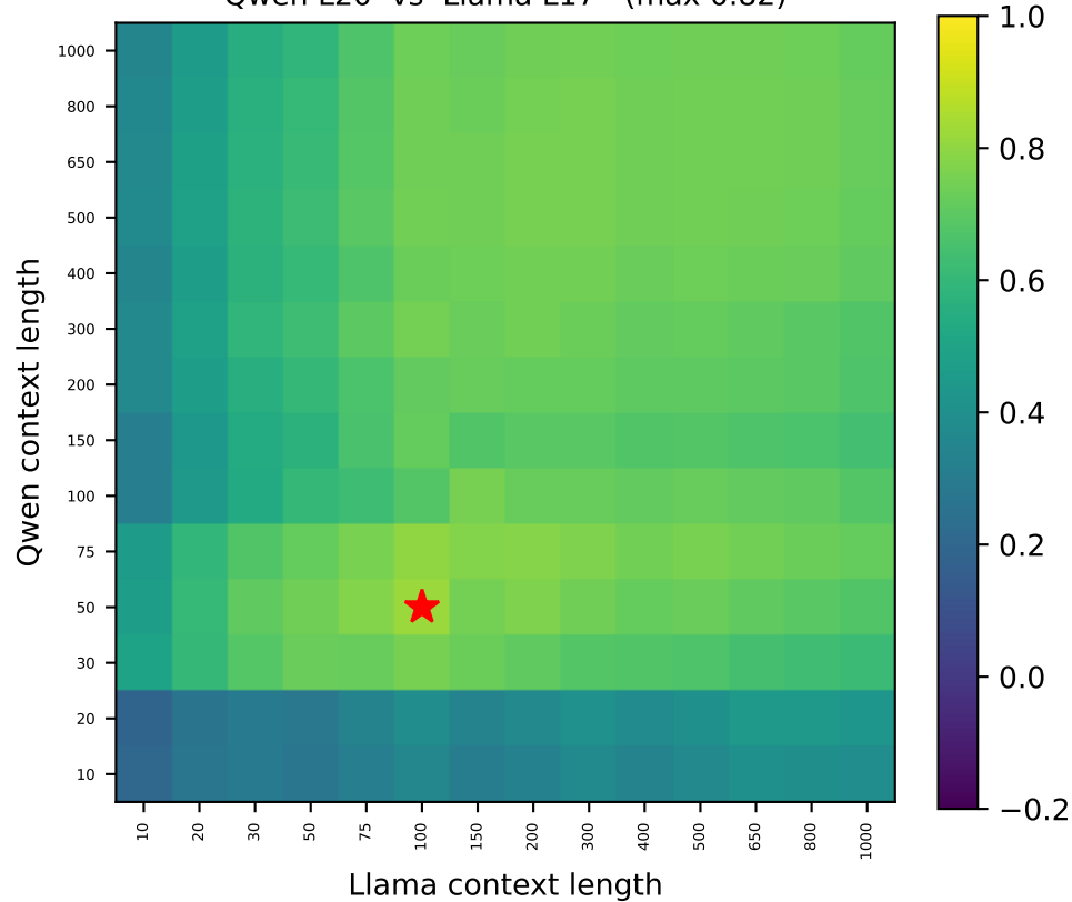
Qwen L20 vs Llama L17 (max 0.82)
