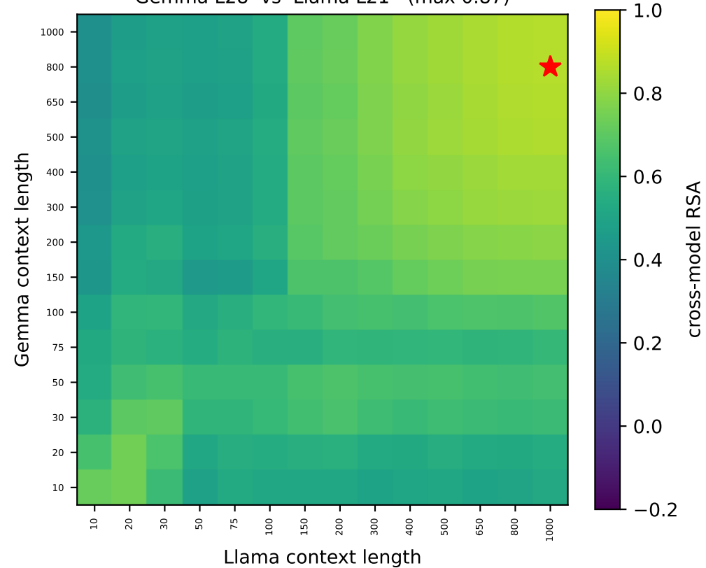
Gemma L28 vs Llama L21 (max 0.87)
