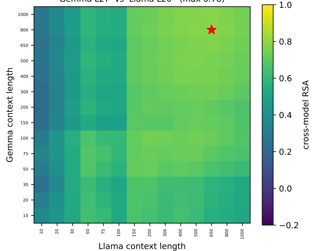
Gemma L27 vs Llama L20 (max 0.78)
