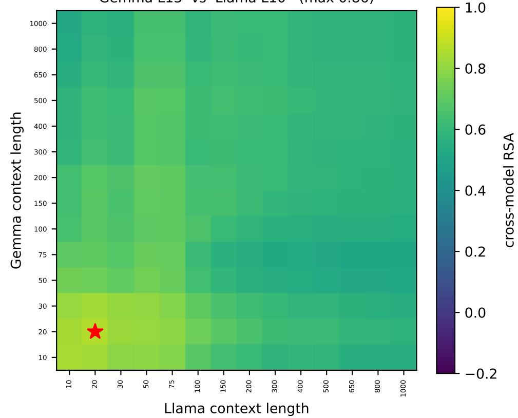
Gemma L13 vs Llama L10 (max 0.86)
