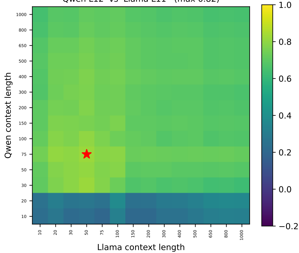
Qwen L12 vs Llama L11 (max 0.82)
