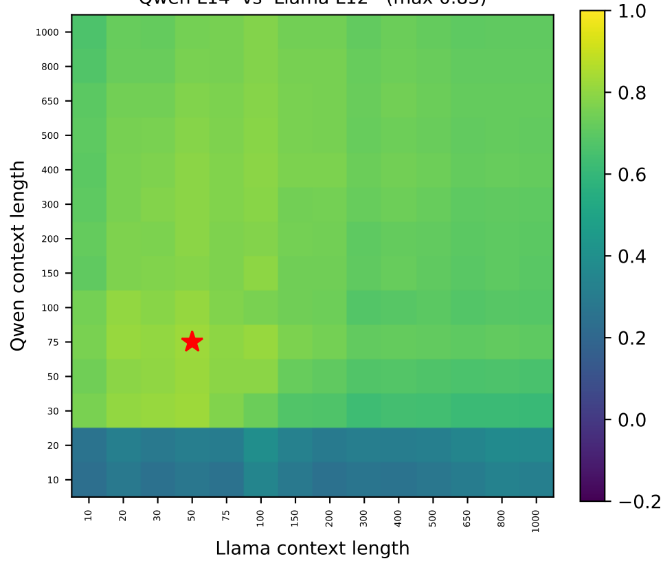
Qwen L14 vs Llama L12 (max 0.83)
