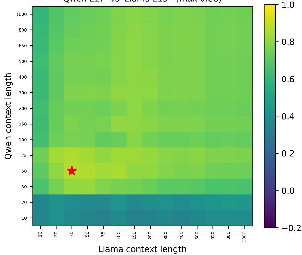
Qwen L17 vs Llama L15 (max 0.86)
