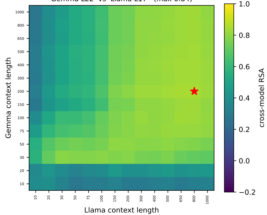
Gemma L22 vs Llama L17 (max 0.84)
