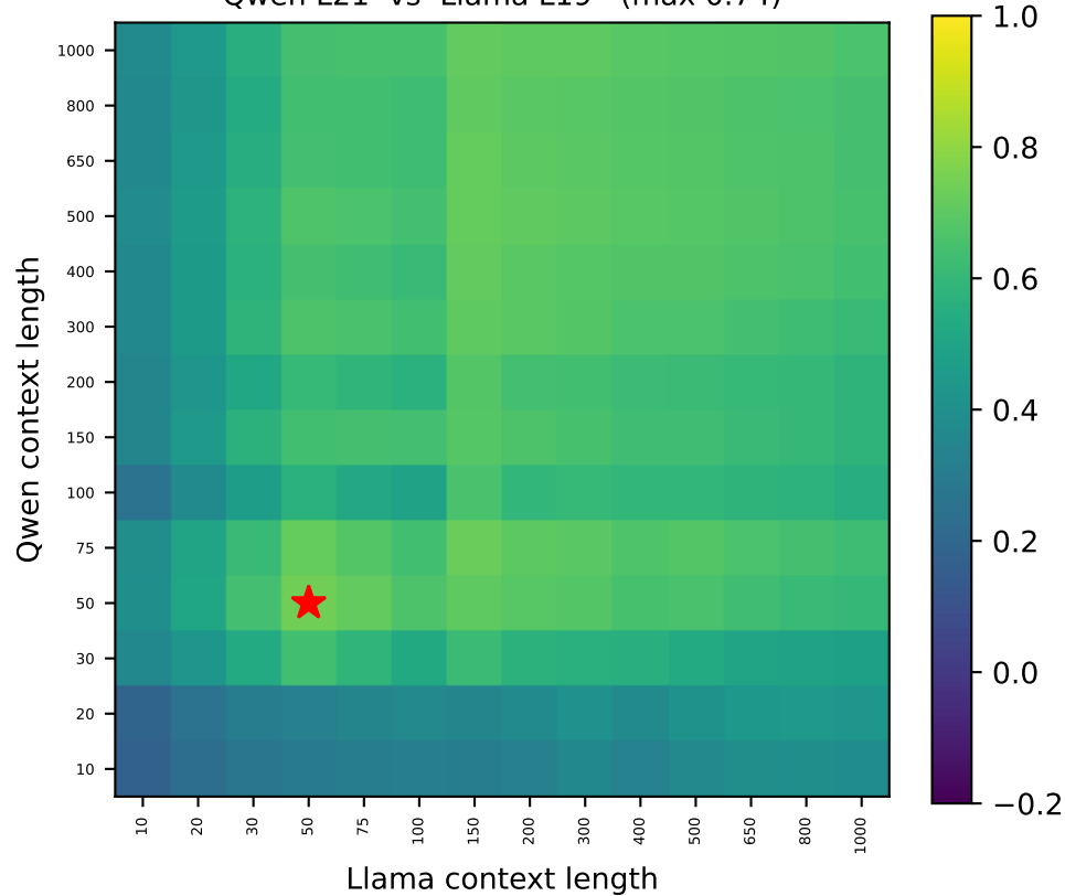
Qwen L21 vs Llama L19 (max 0.74)
