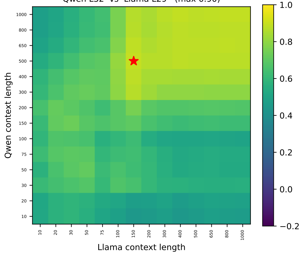
Qwen L32 vs Llama L29 (max 0.90)
