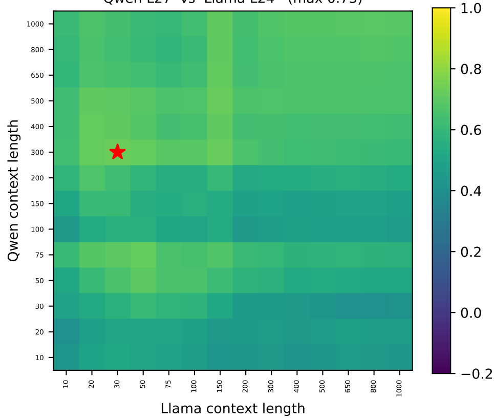
Qwen L27 vs Llama L24 (max 0.73)
