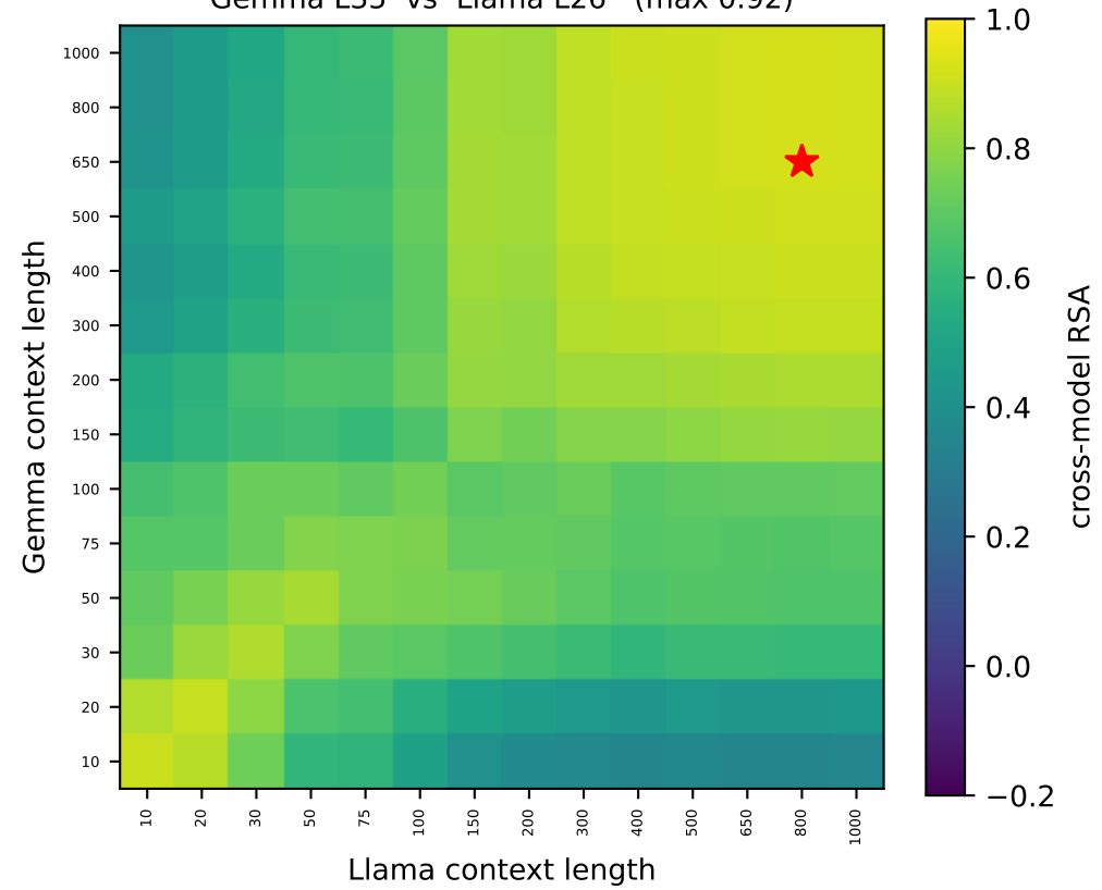
Gemma L35 vs Llama L26 (max 0.92)
