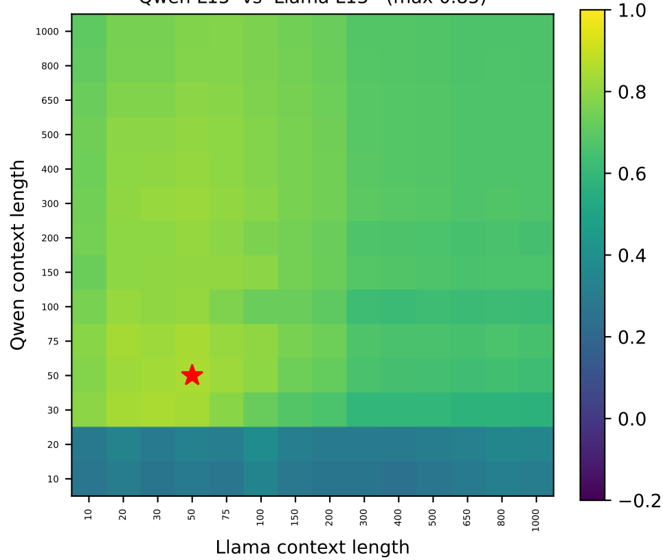
Qwen L15 vs Llama L13 (max 0.85)
