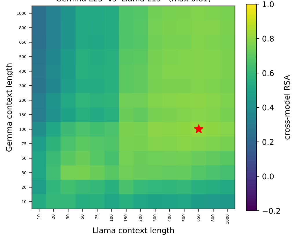
Gemma L25 vs Llama L19 (max 0.81)
