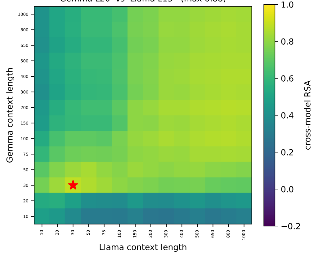
Gemma L20 vs Llama L15 (max 0.88)
