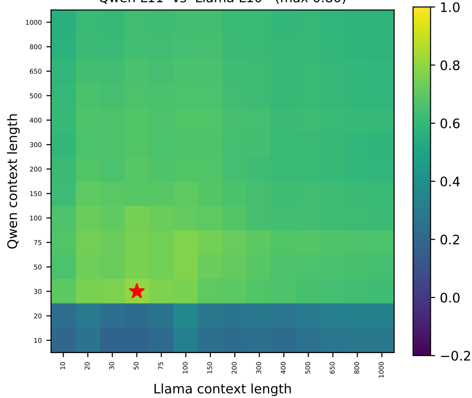
Qwen L11 vs Llama L10 (max 0.80)
