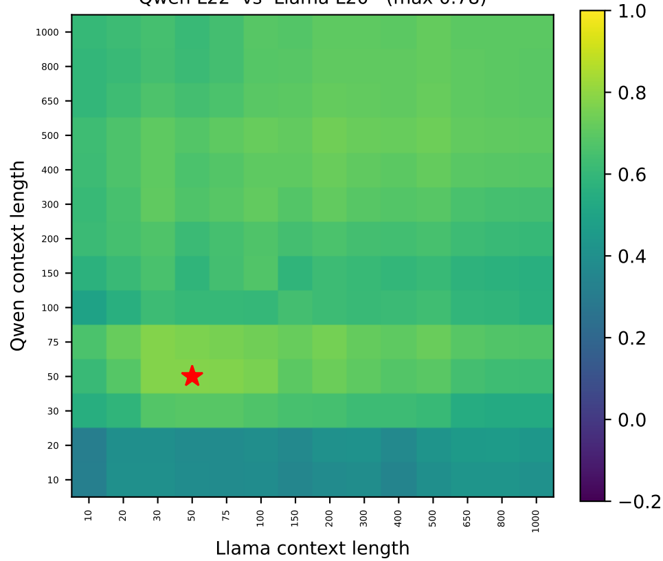
Qwen L22 vs Llama L20 (max 0.78)
