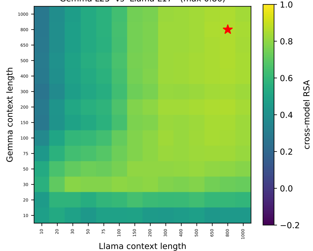
Gemma L23 vs Llama L17 (max 0.86)
