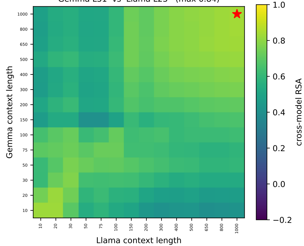
Gemma L31 vs Llama L23 (max 0.84)
