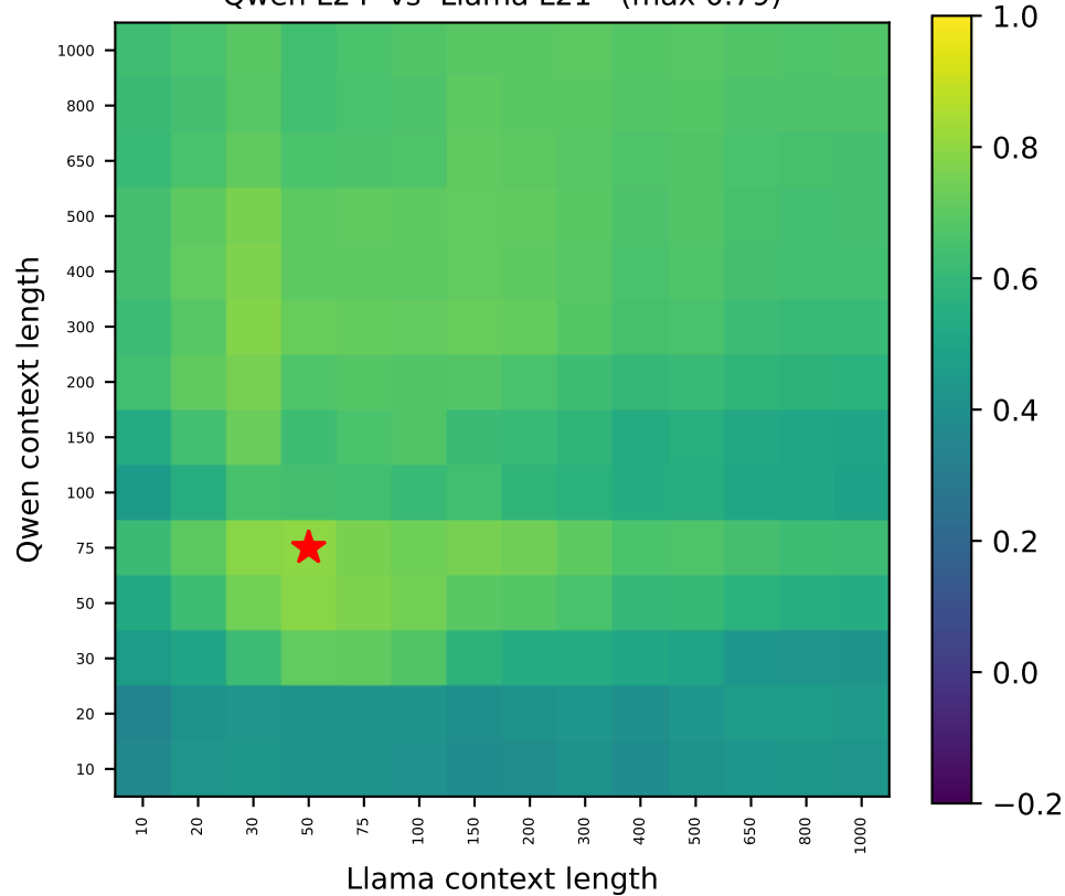
Qwen L24 vs Llama L21 (max 0.79)
