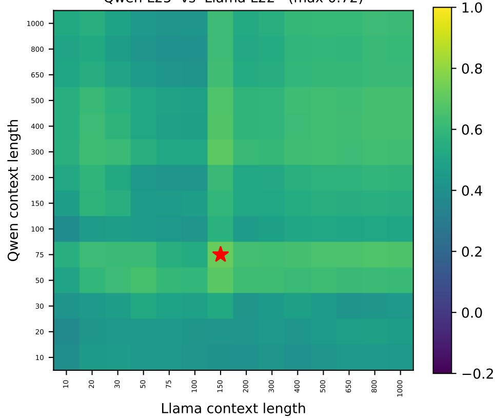
Qwen L25 vs Llama L22 (max 0.72)
