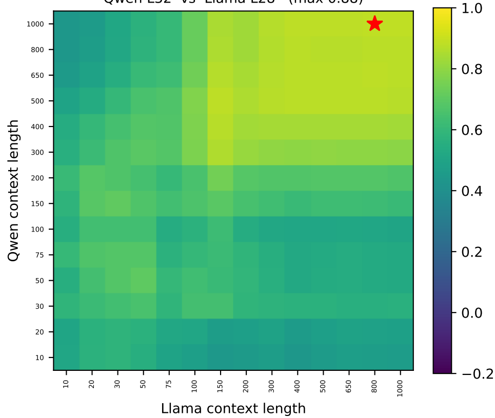
Qwen L32 vs Llama L28 (max 0.88)
