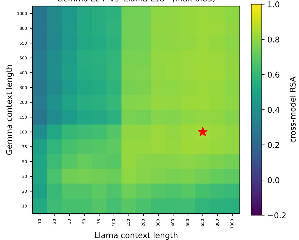
Gemma L24 vs Llama L18 (max 0.83)
