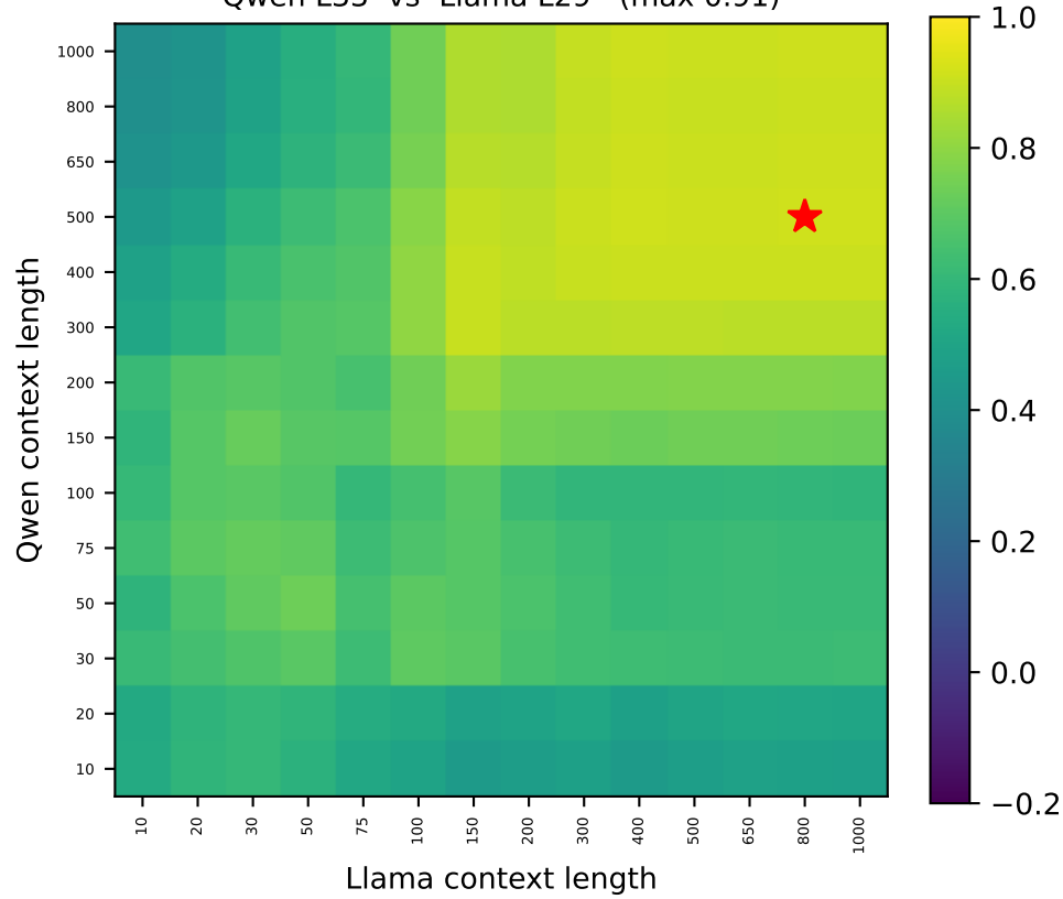
Qwen L33 vs Llama L29 (max 0.91)
