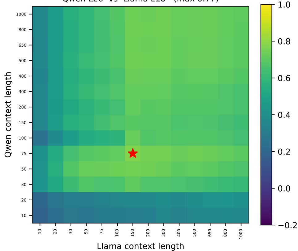
Qwen L20 vs Llama L18 (max 0.77)
