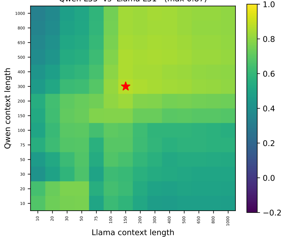
Qwen L35 vs Llama L31 (max 0.87)
