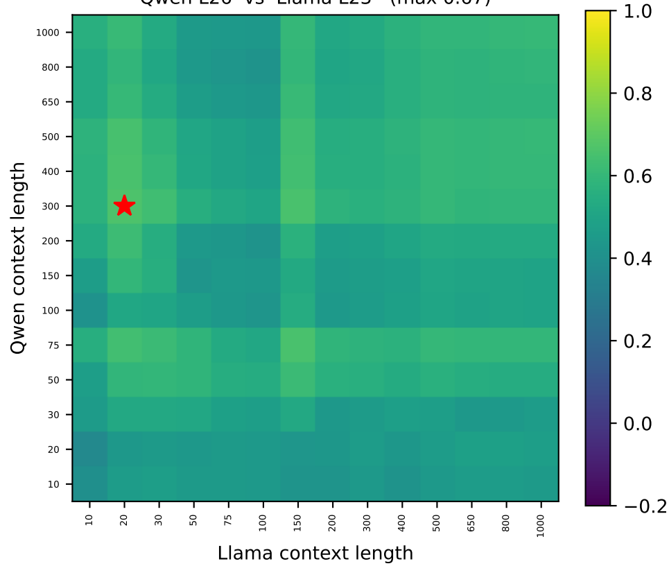
Qwen L26 vs Llama L23 (max 0.67)
