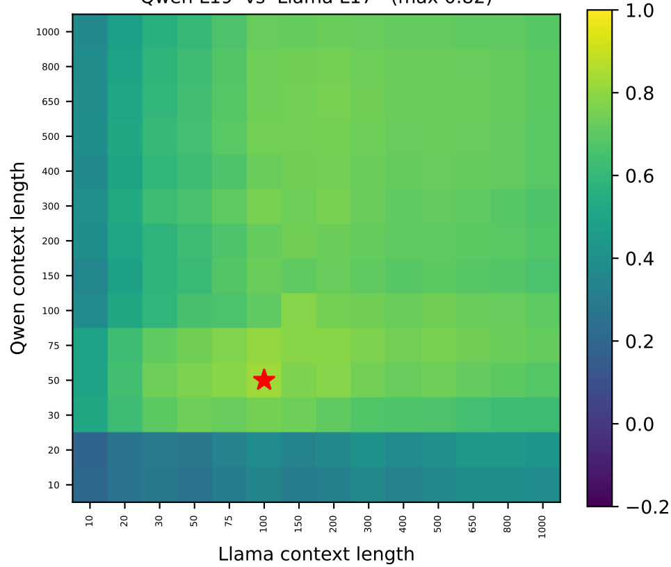
Qwen L19 vs Llama L17 (max 0.82)
