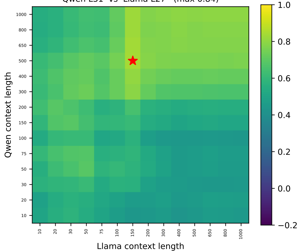
Qwen L31 vs Llama L27 (max 0.84)
