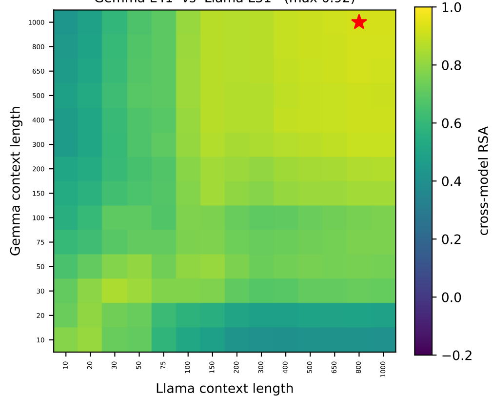
Gemma L41 vs Llama L31 (max 0.92)
