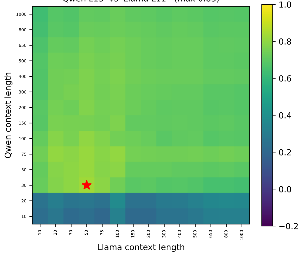
Qwen L13 vs Llama L11 (max 0.83)
