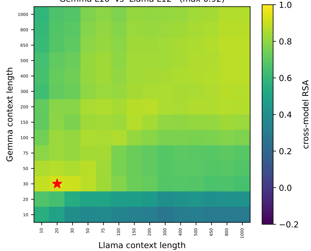
Gemma L16 vs Llama L12 (max 0.92)
