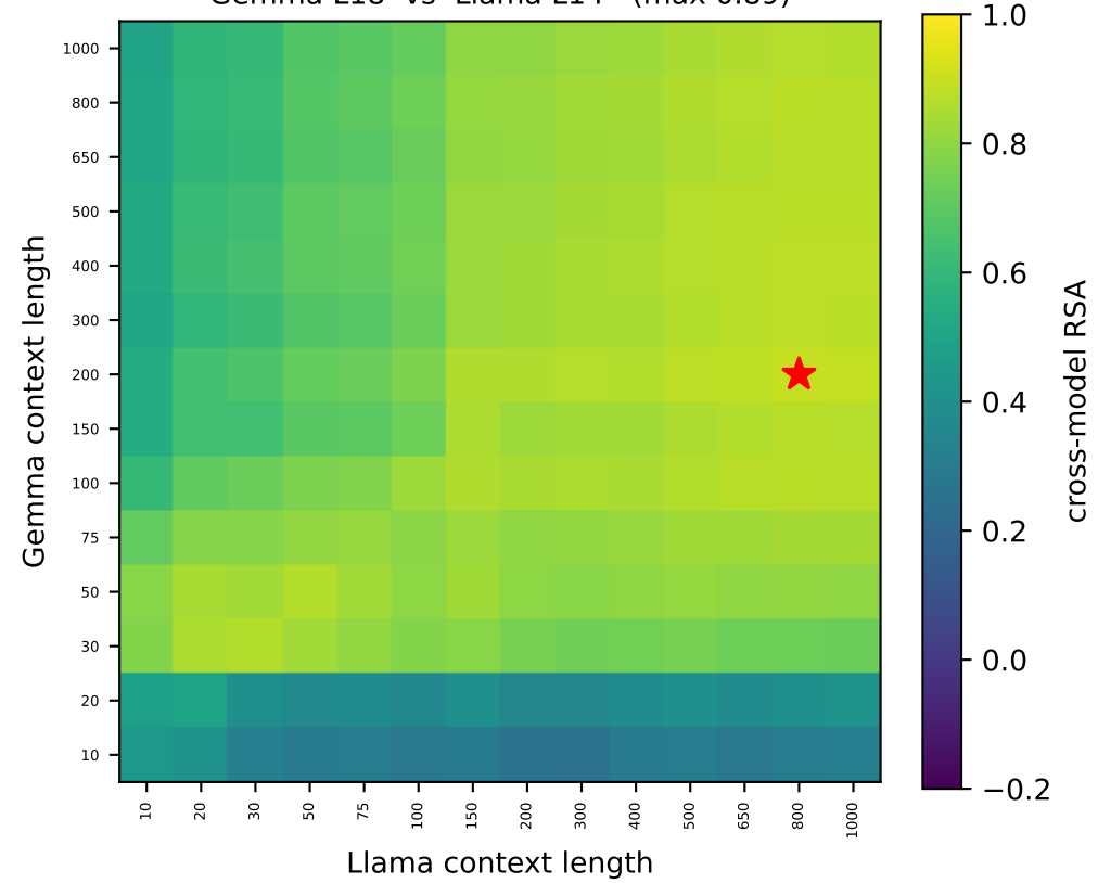
Gemma L18 vs Llama L14 (max 0.89)
