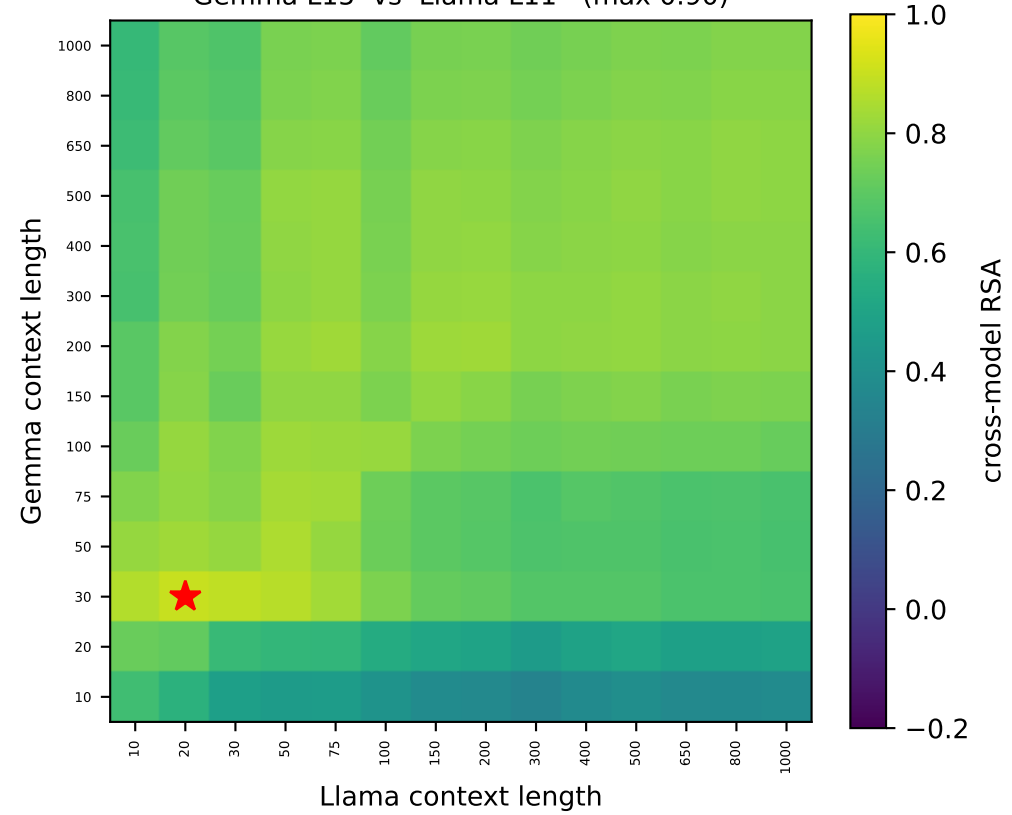
Gemma L15 vs Llama L11 (max 0.90)
