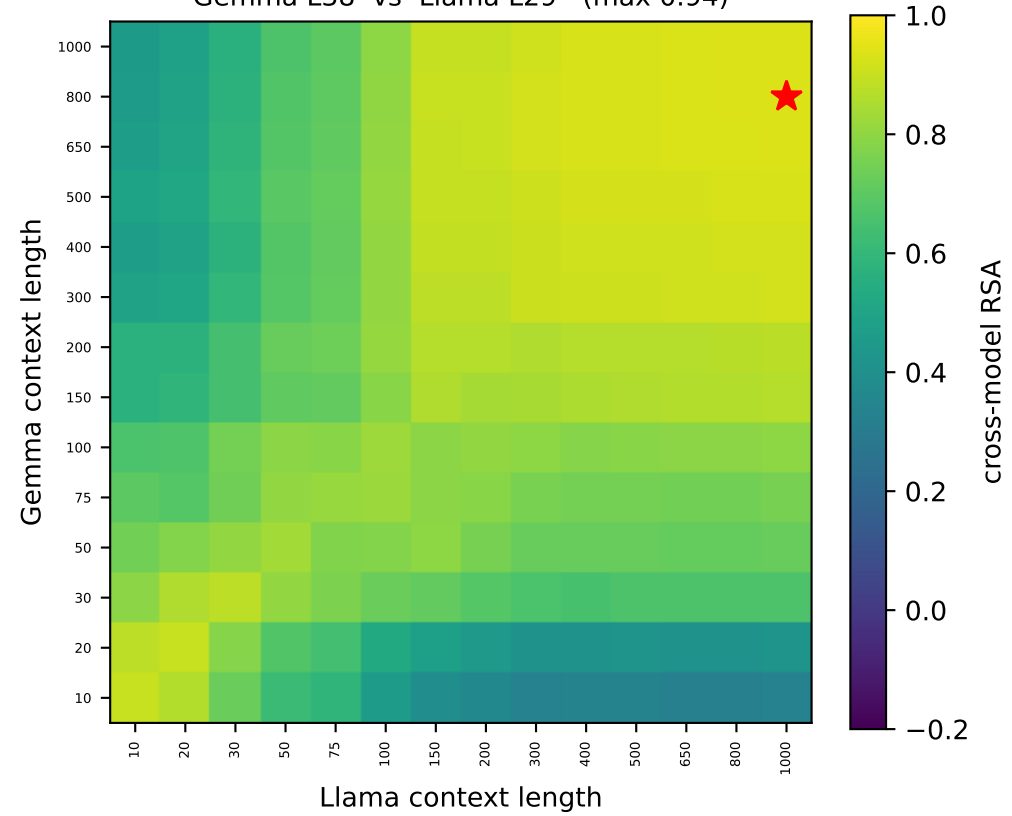
Gemma L38 vs Llama L29 (max 0.94)
