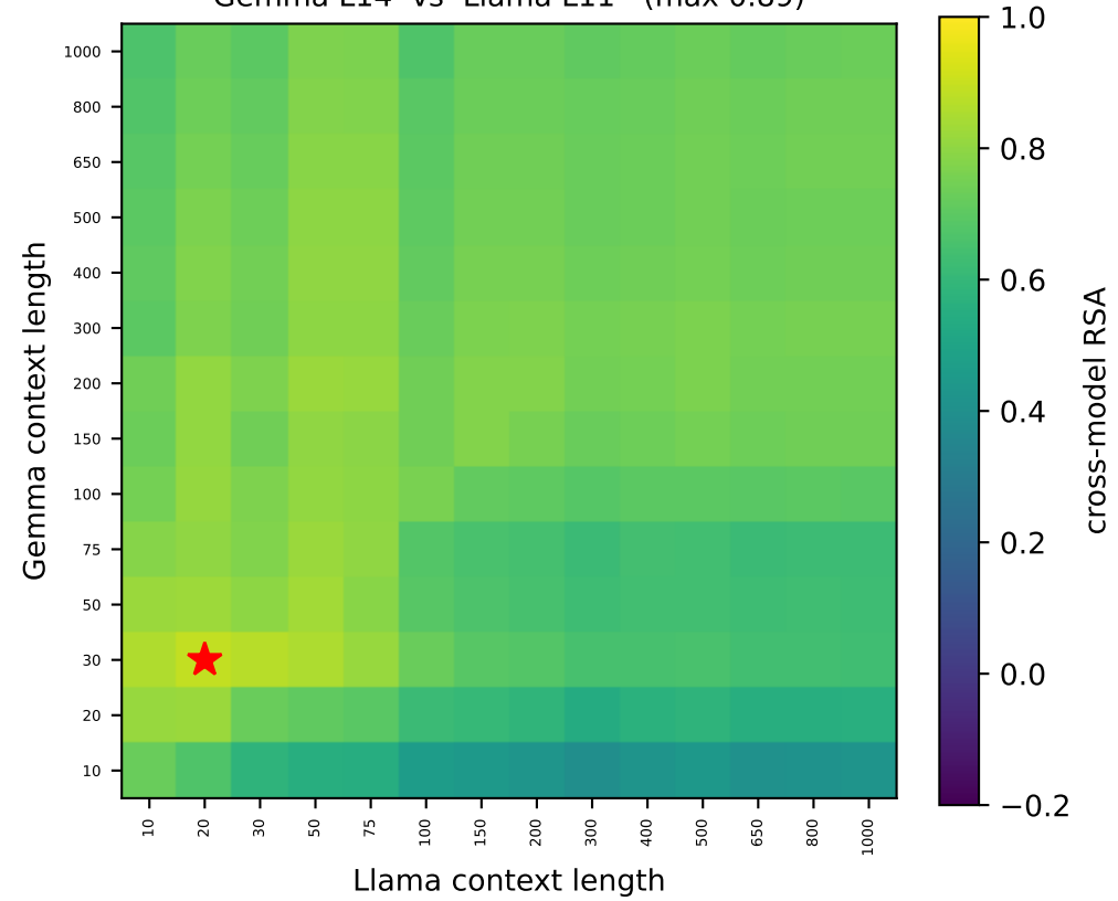
Gemma L14 vs Llama L11 (max 0.89)
