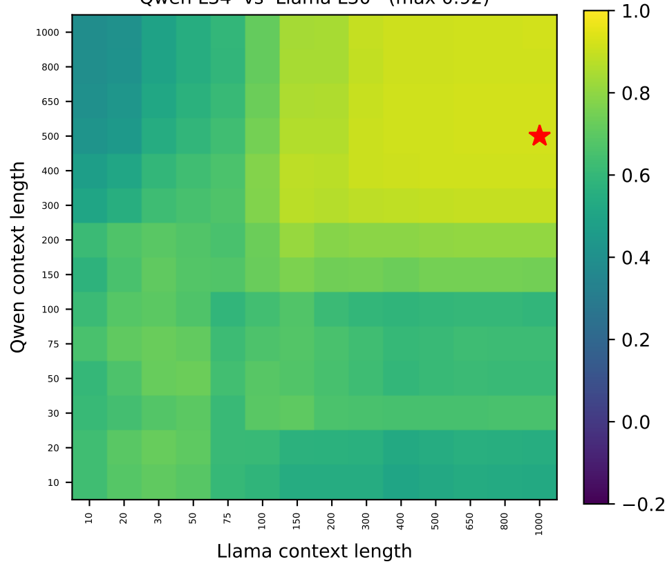
Qwen L34 vs Llama L30 (max 0.92)
