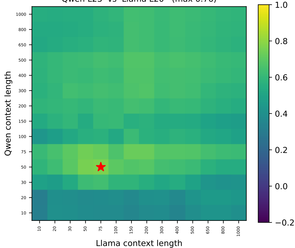
Qwen L23 vs Llama L20 (max 0.76)
