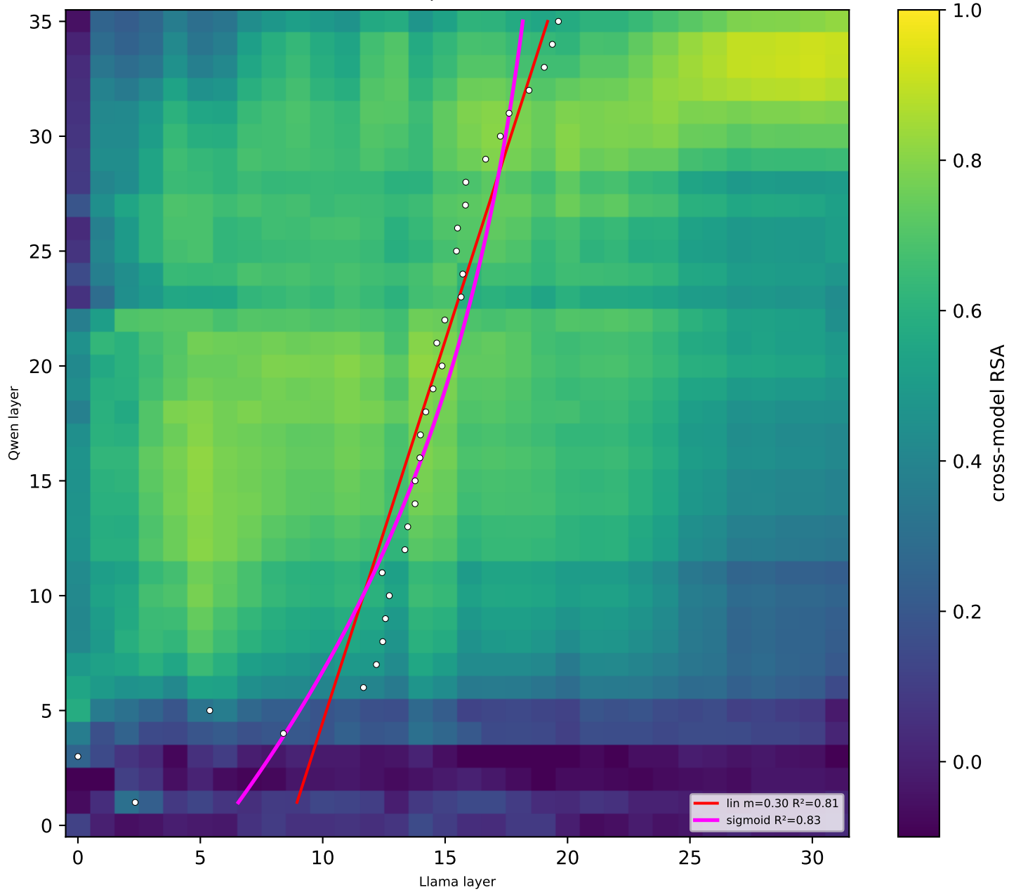
hex Qwen×Llama
