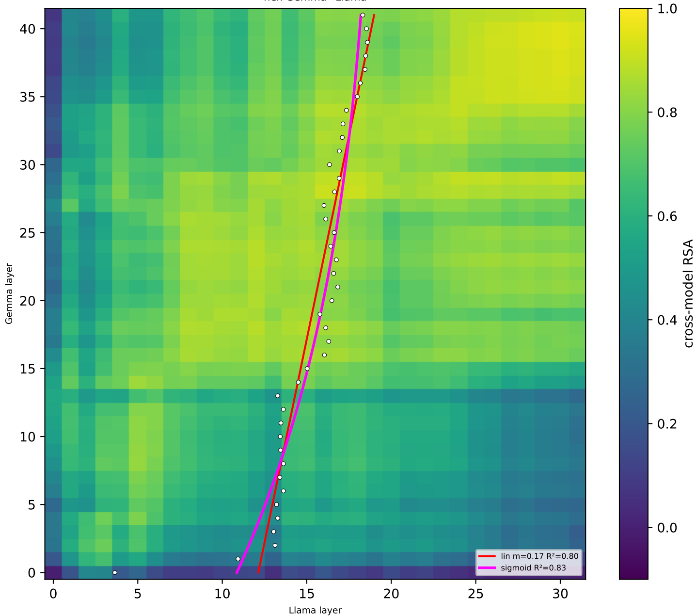
hex Gemma×Llama
