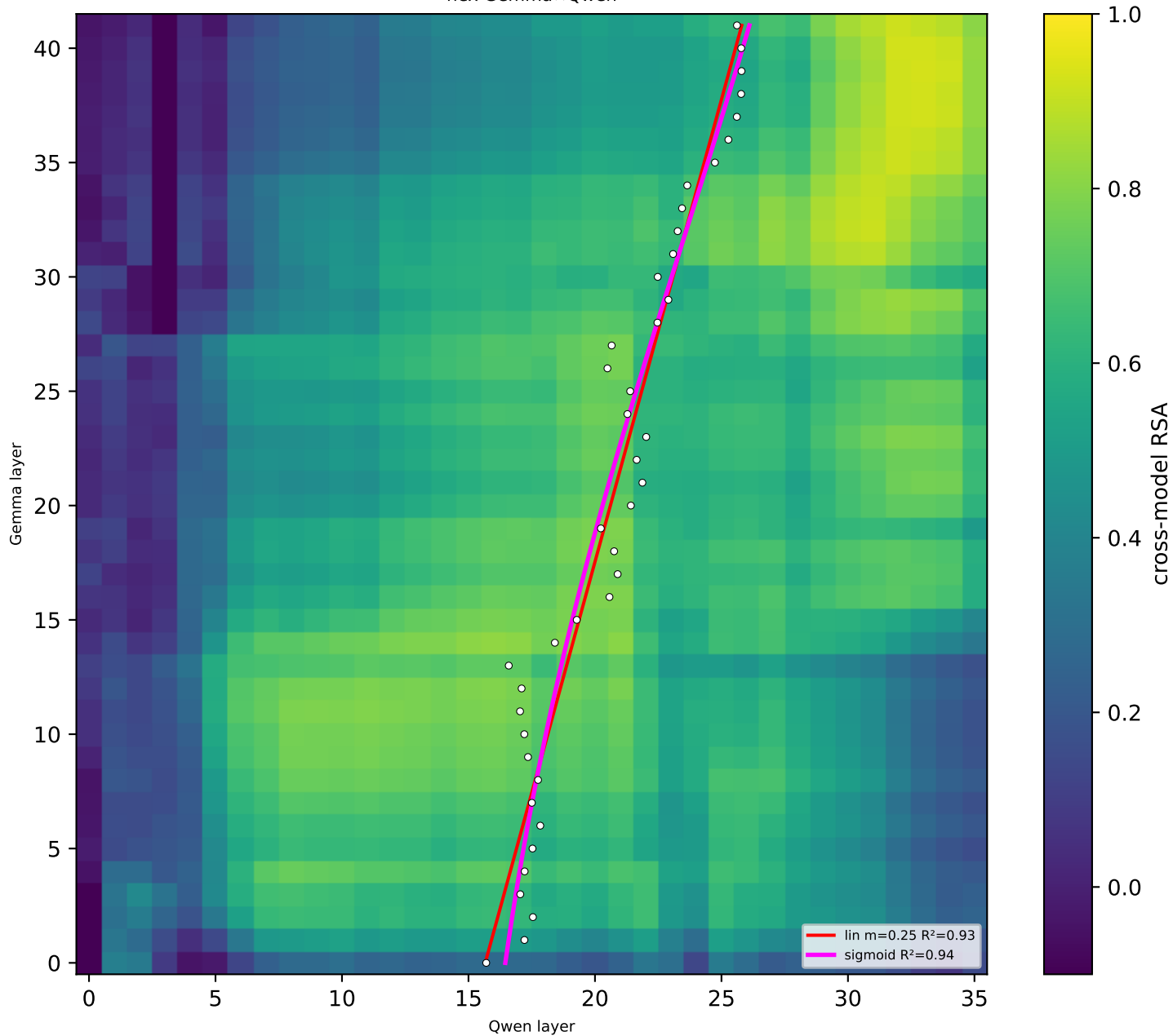
hex Gemma×Qwen
