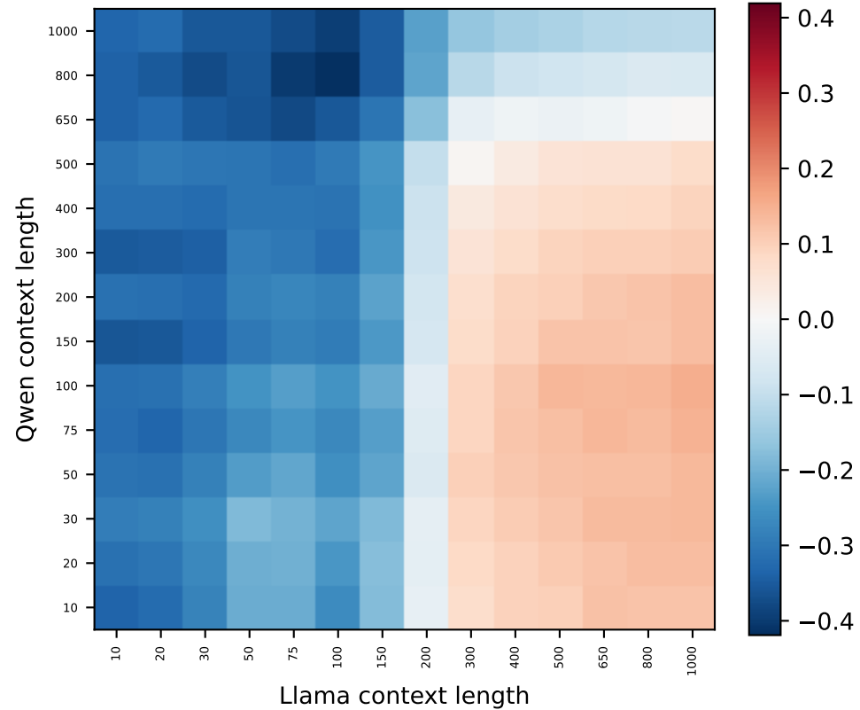
Qwen L5 vs Llama L5 (34% > null)
