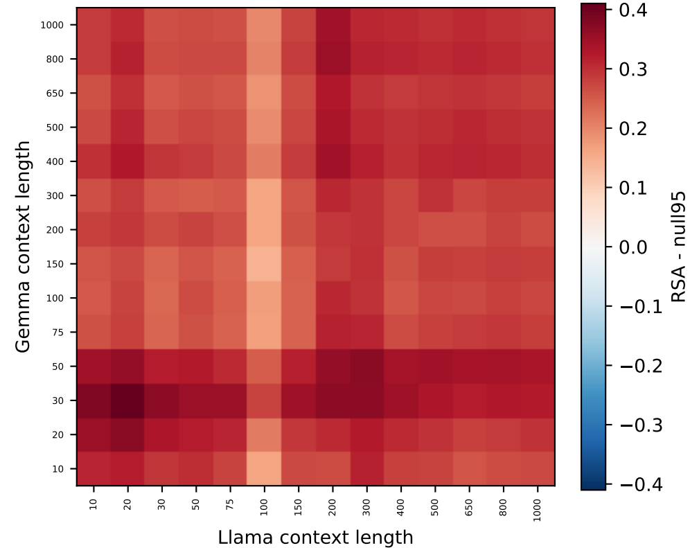
Gemma L4 vs Llama L3 (100% > null)
