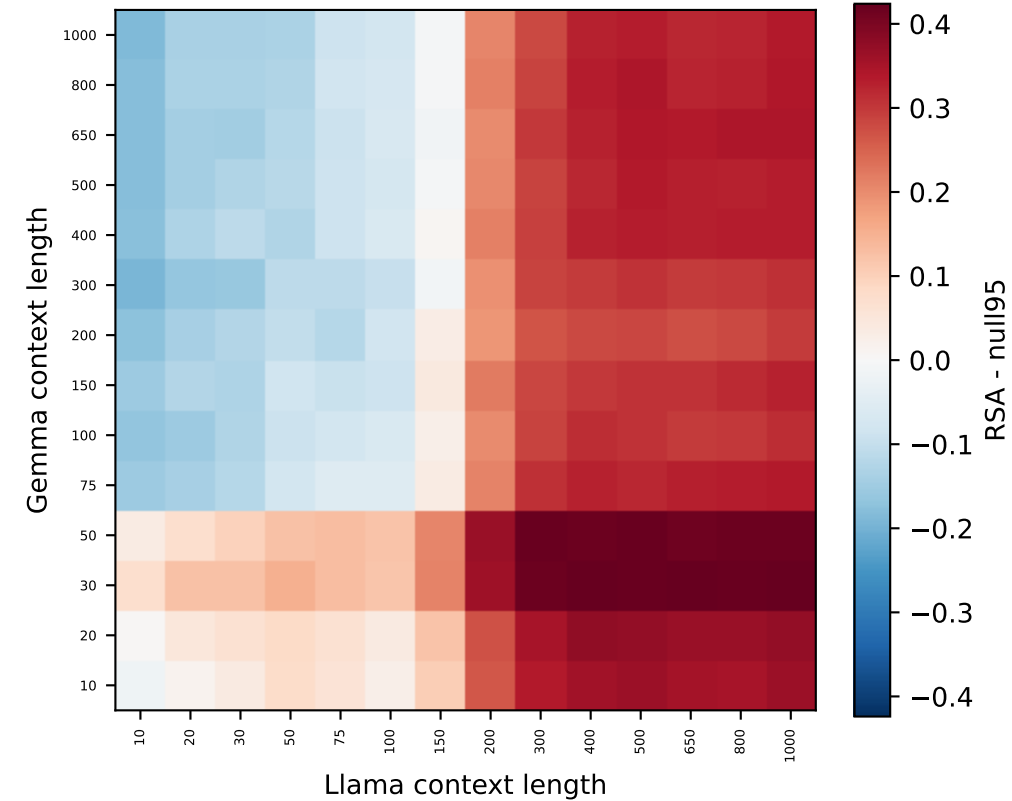
Gemma L6 vs Llama L5 (66% > null)
