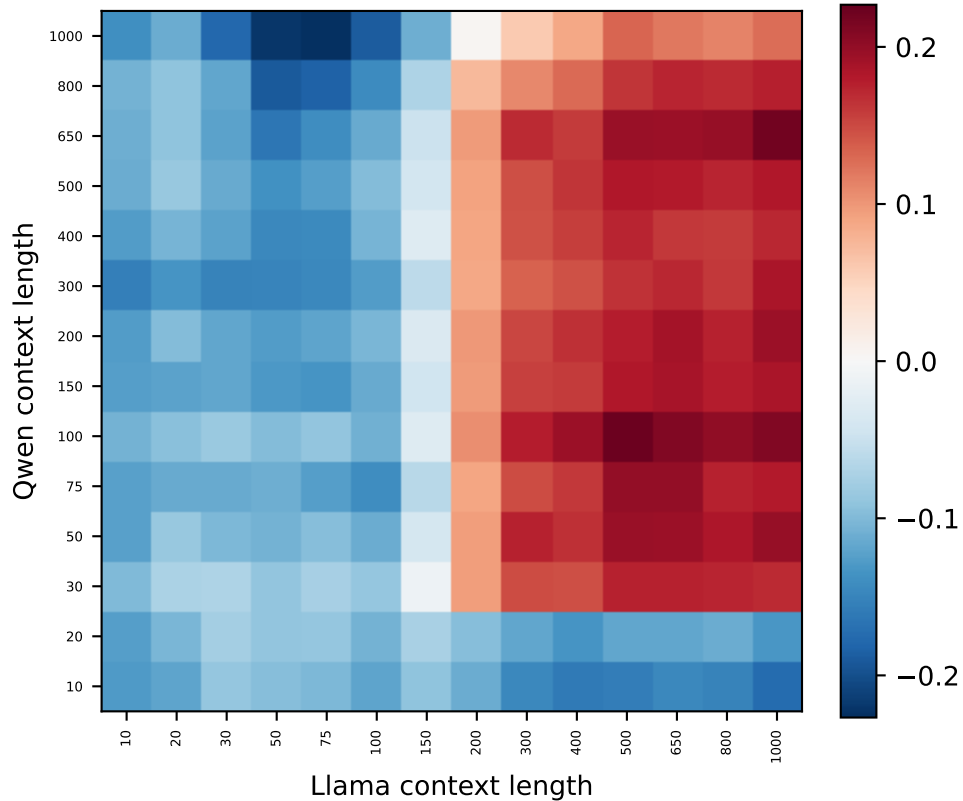
Qwen L7 vs Llama L6 (43% > null)
