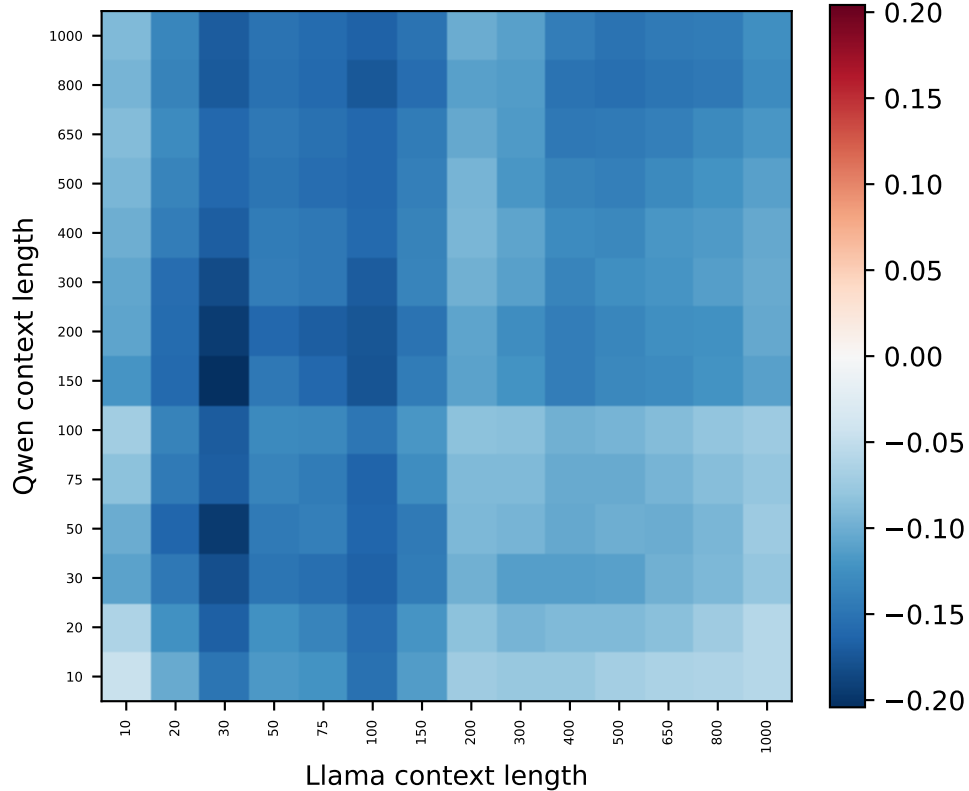
Qwen L3 vs Llama L3 (0% > null)
