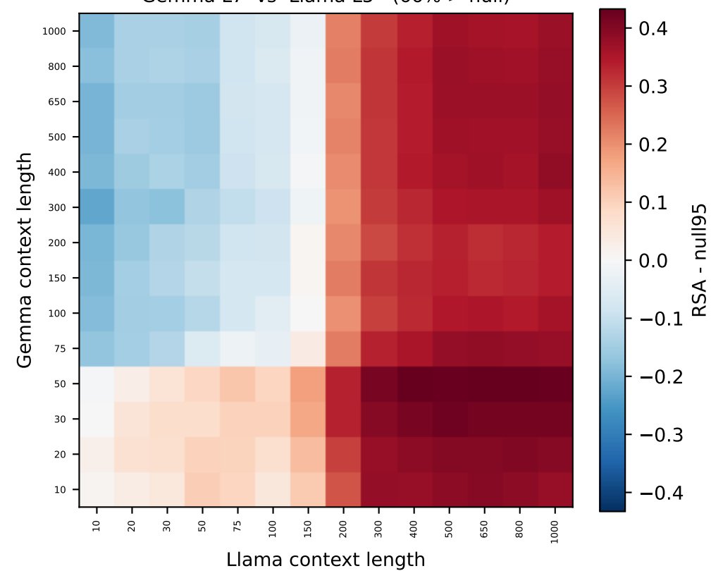
Gemma L7 vs Llama L5 (66% > null)
