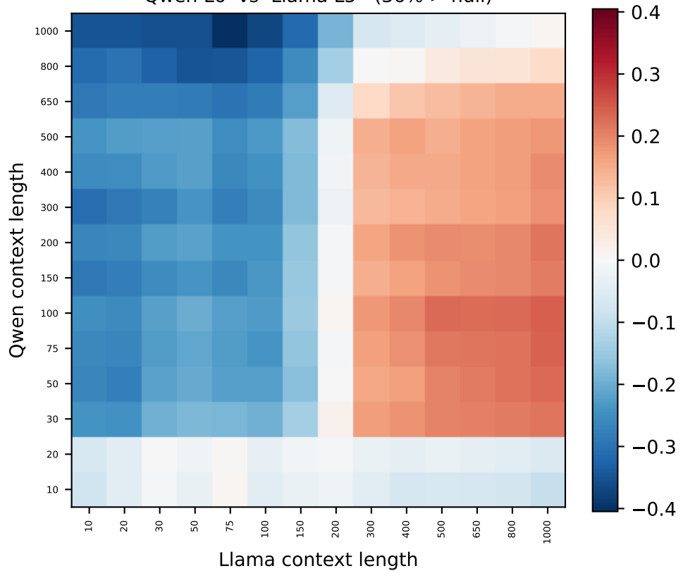
Qwen L6 vs Llama L5 (36% > null)
