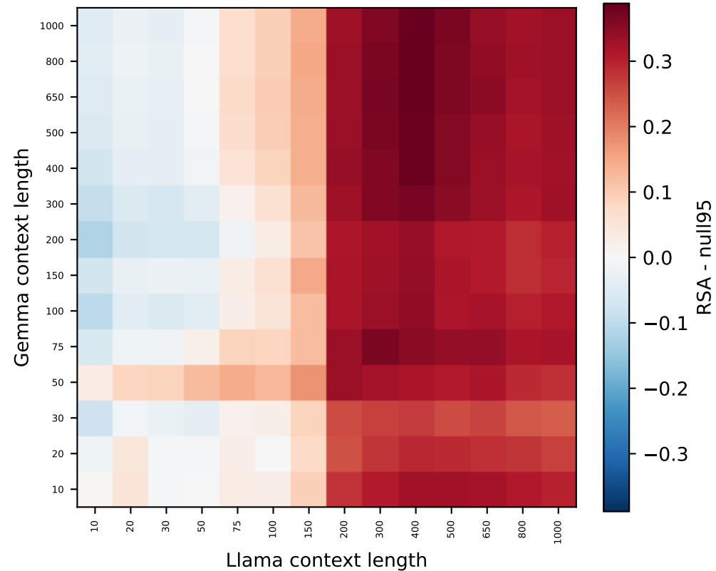
Gemma L9 vs Llama L7 (75% > null)
