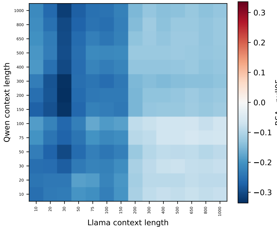
Qwen L4 vs Llama L4 (0% > null)
