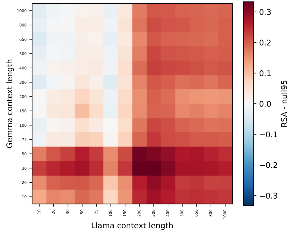
Gemma L5 vs Llama L4 (88% > null)
