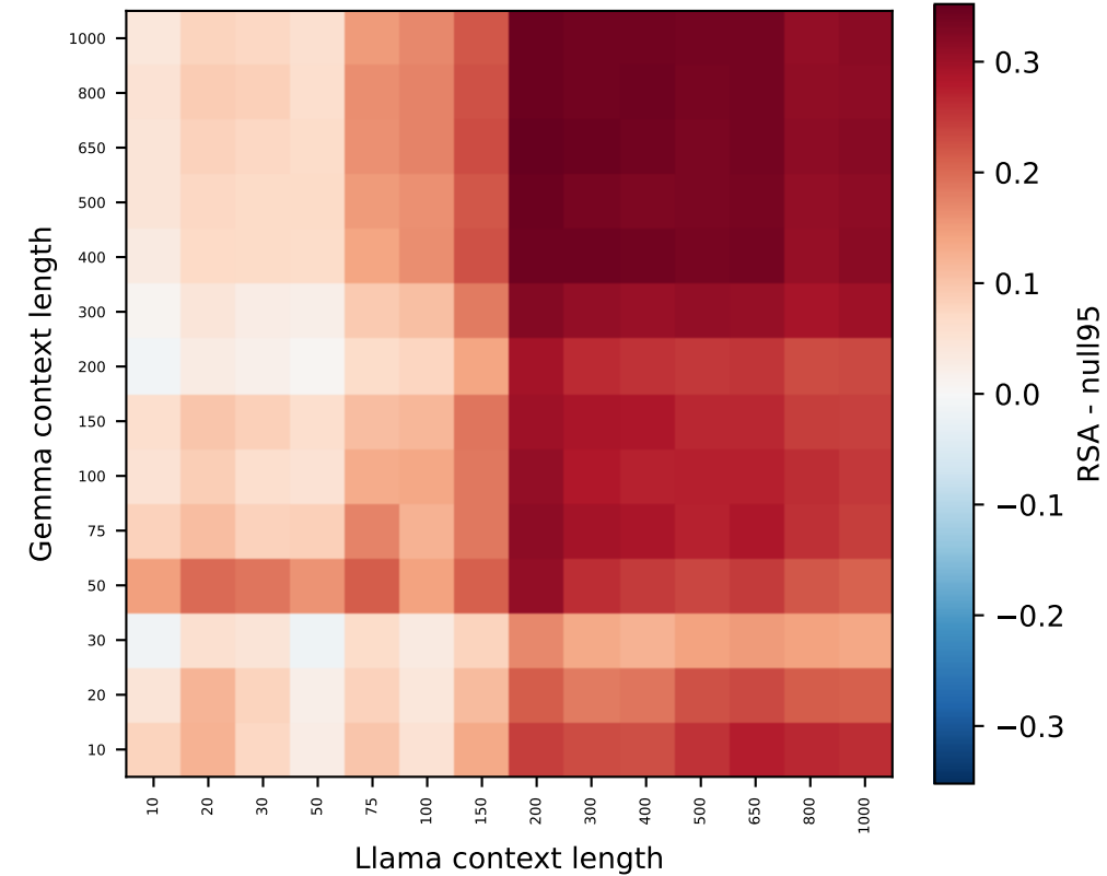
Gemma L10 vs Llama L8 (98% > null)
