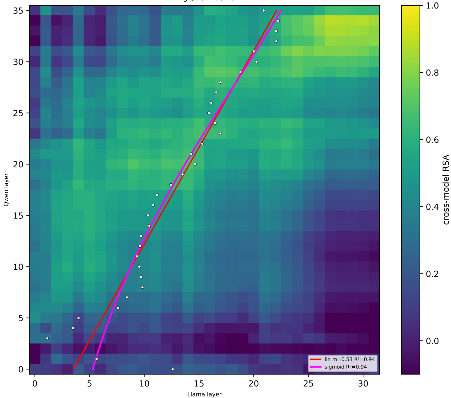
ring Qwen×Llama
