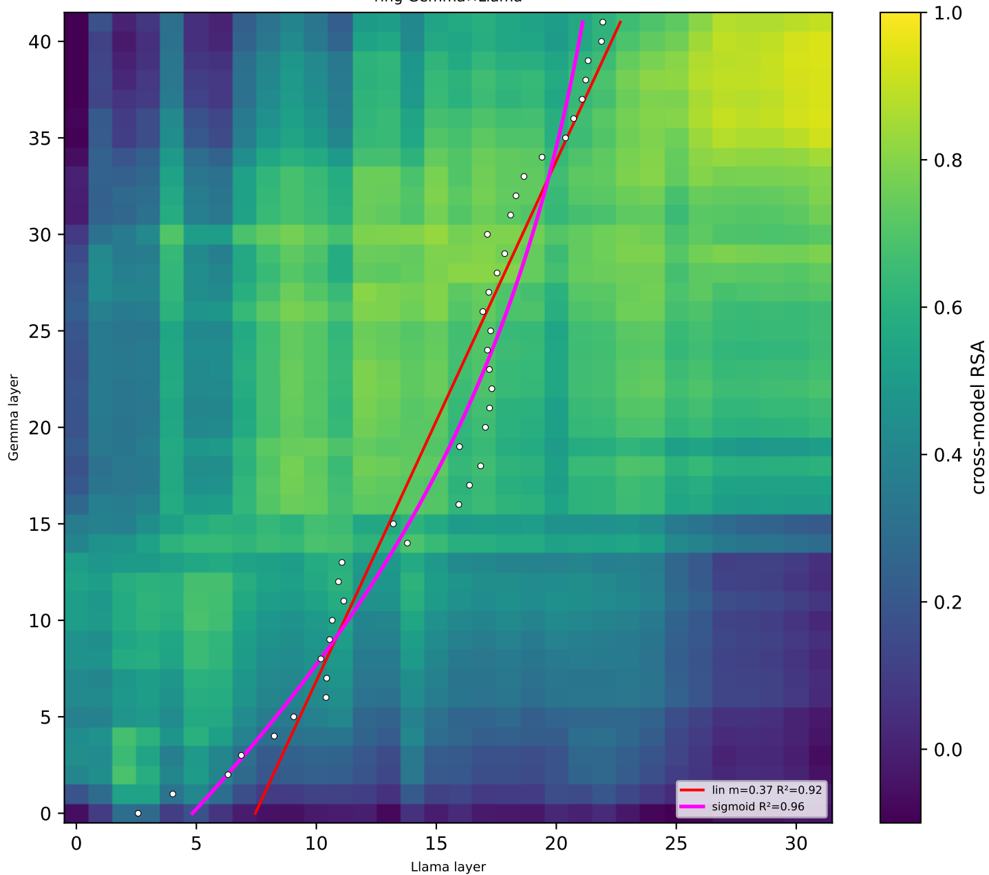
ring Gemma×Llama
