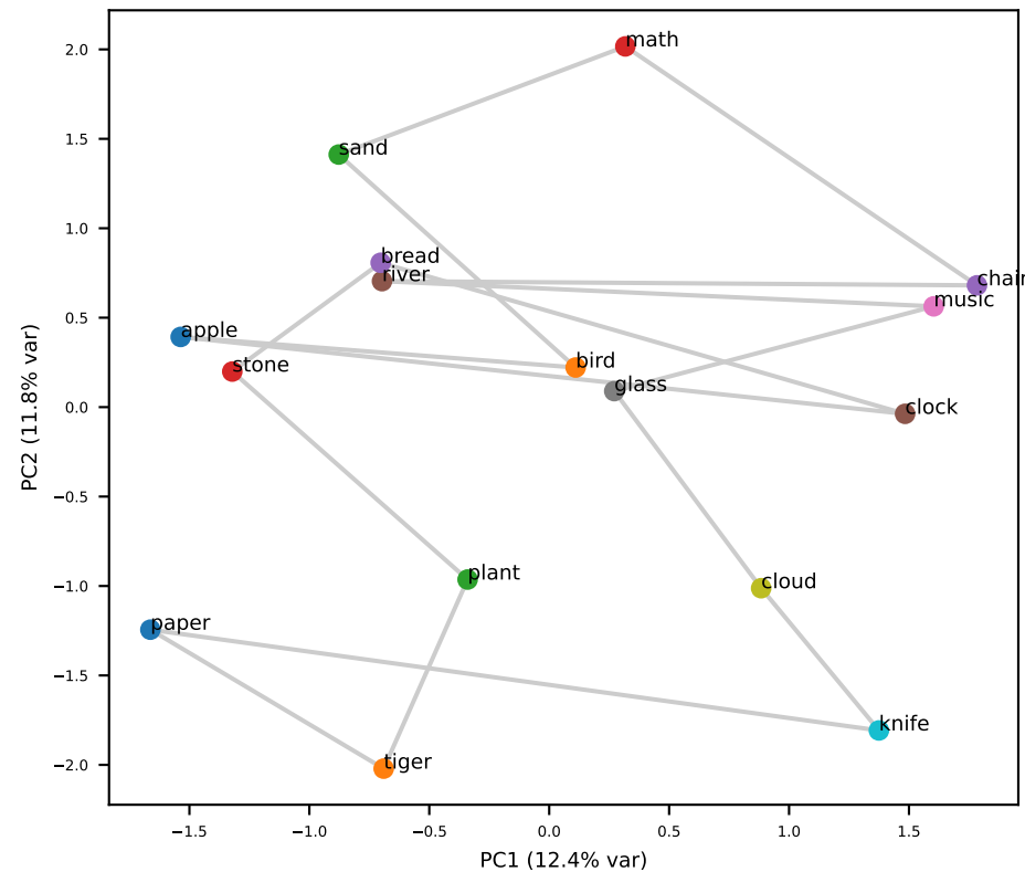
Llama L14 (grid RSA=+0.42)
