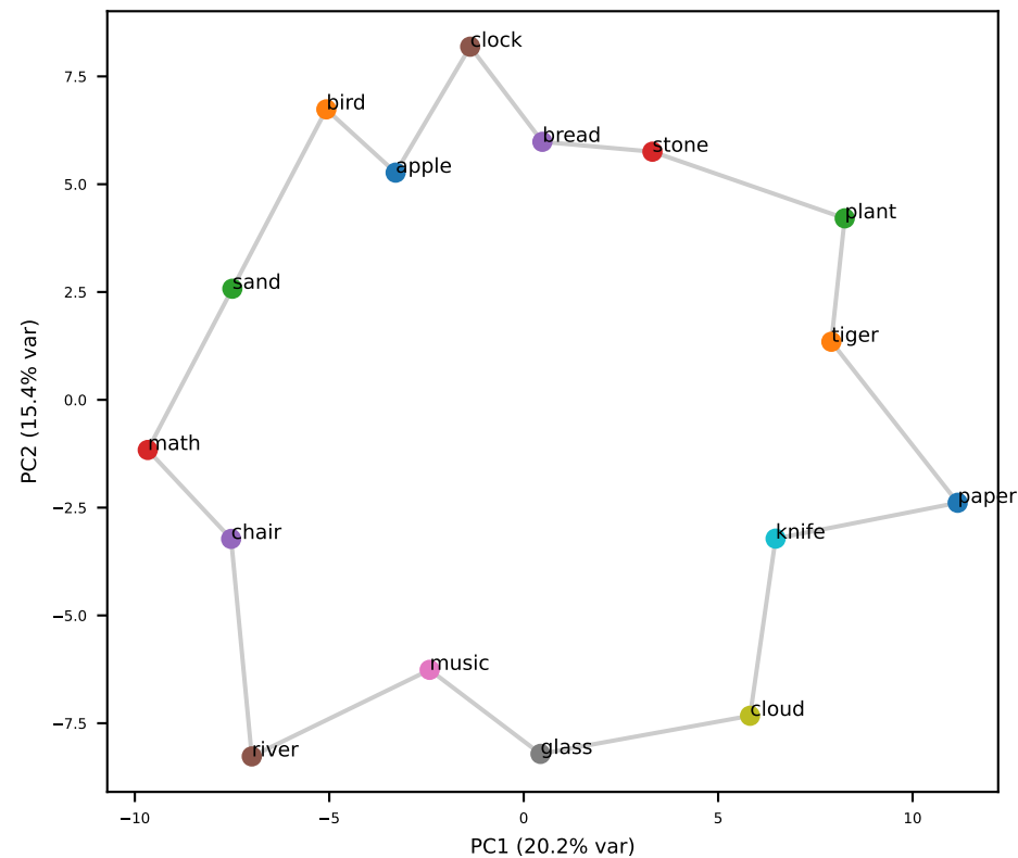
Llama L27 (grid RSA=+0.74)
