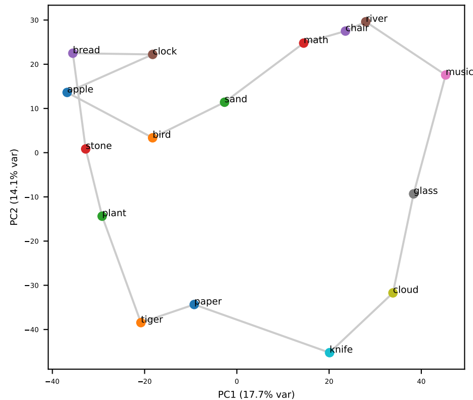
Gemma L23 (grid RSA=+0.62)
