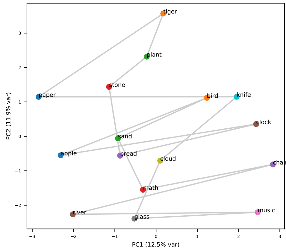
Llama L16 (grid RSA=+0.40)
