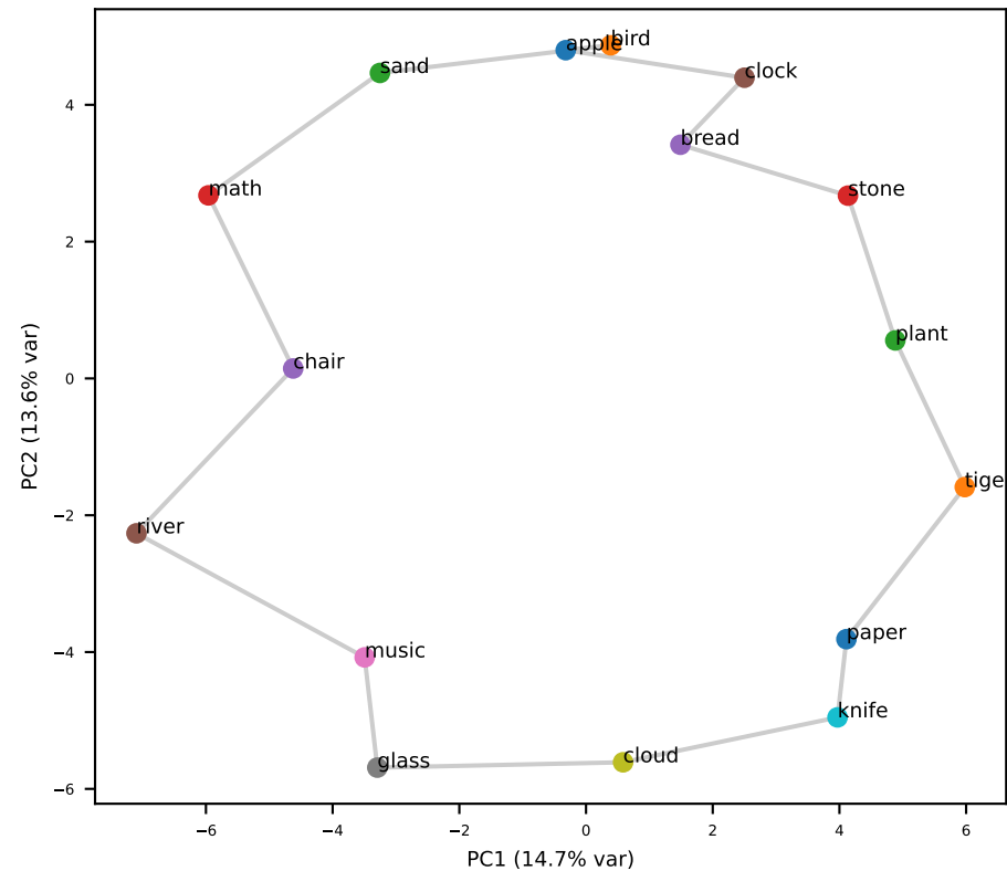
Llama L24 (grid RSA=+0.67)
