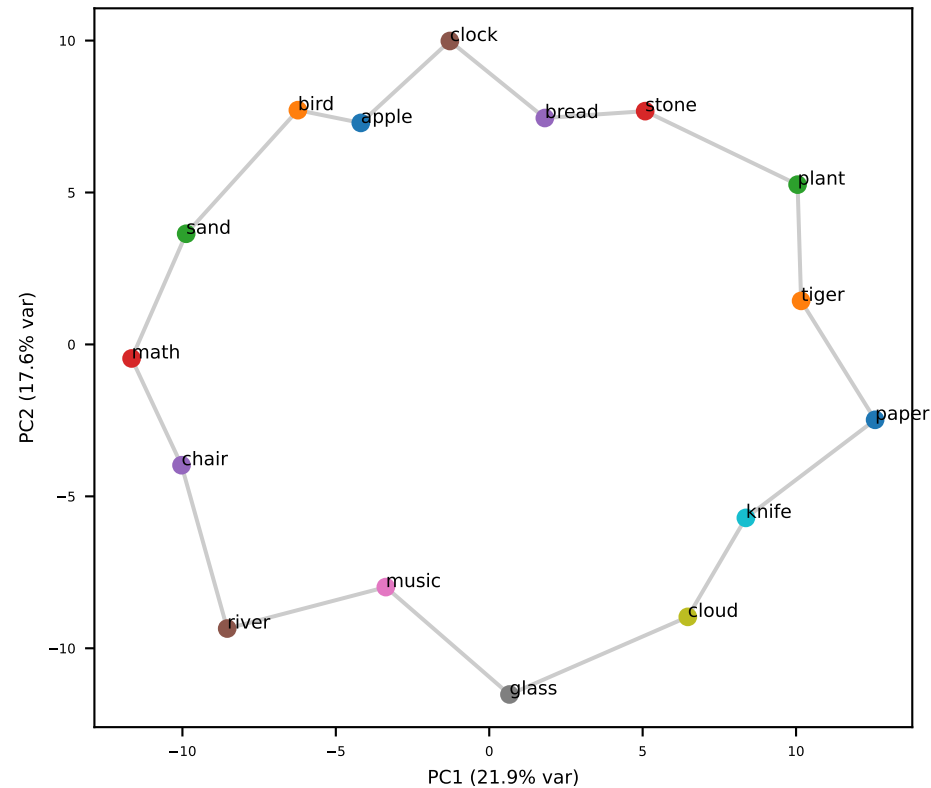
Llama L29 (grid RSA=+0.80)
