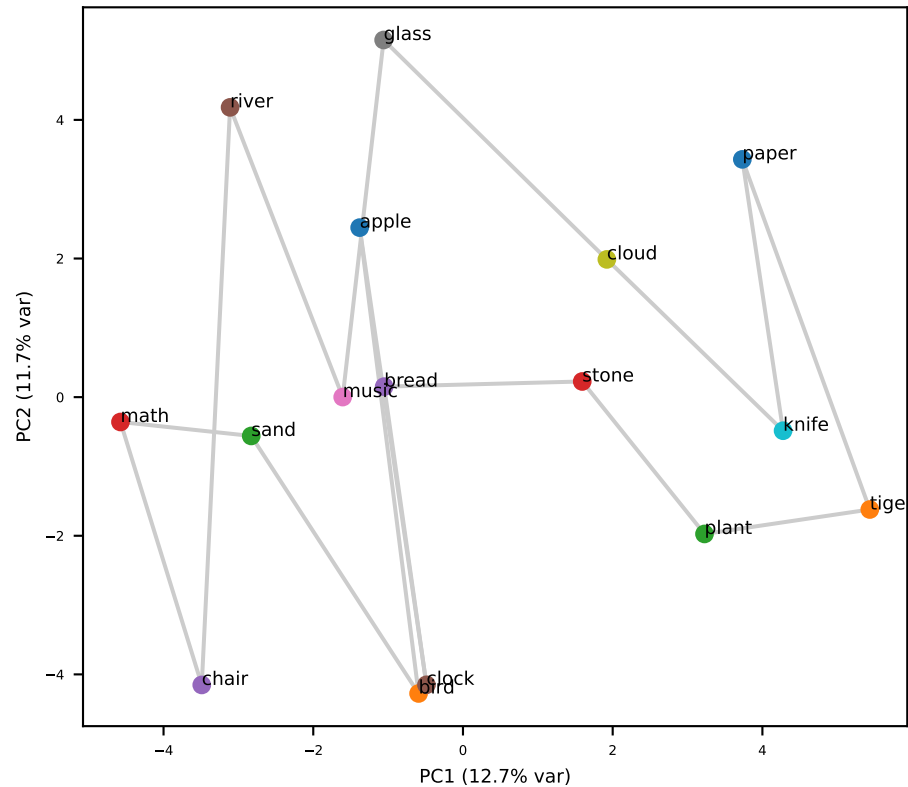
Llama L21 (grid RSA=+0.49)
