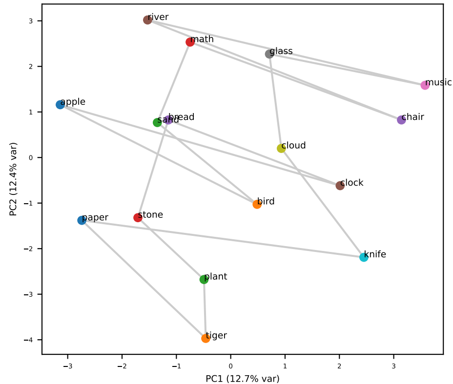
Llama L17 (grid RSA=+0.46)
