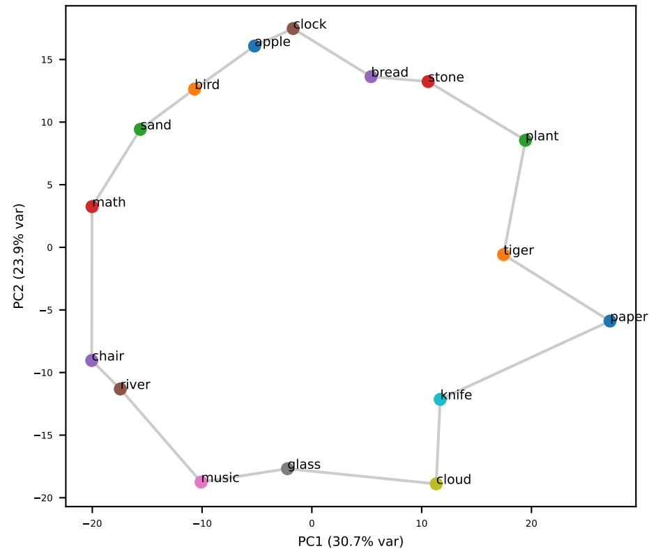
Llama L31 (grid RSA=+0.82)
