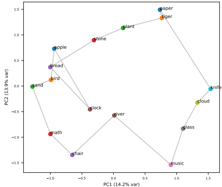
Llama L12 (grid RSA=+0.58)
