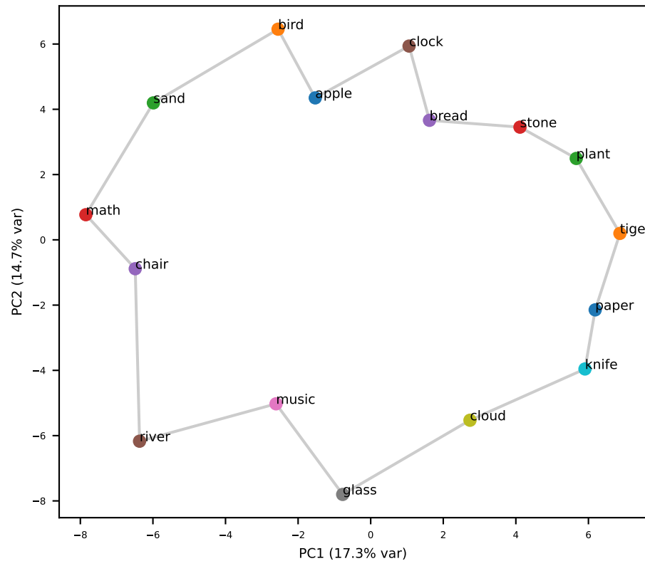
Llama L25 (grid RSA=+0.72)
