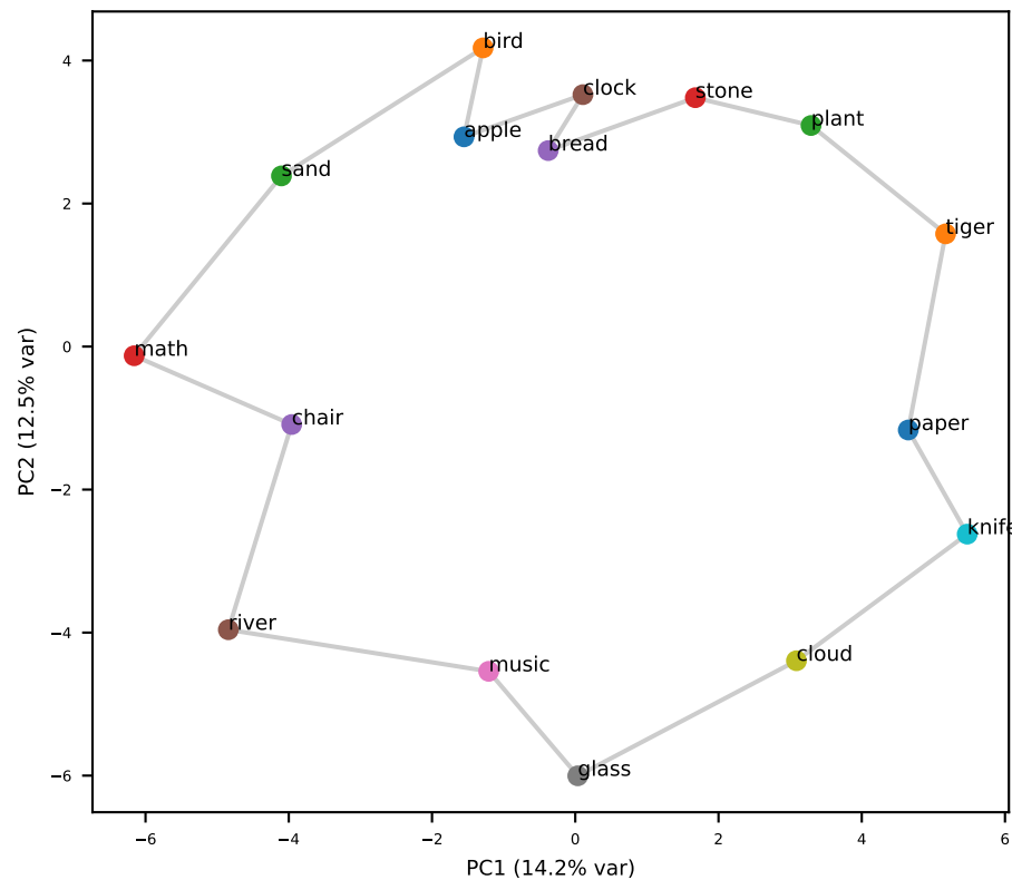
Llama L23 (grid RSA=+0.61)
