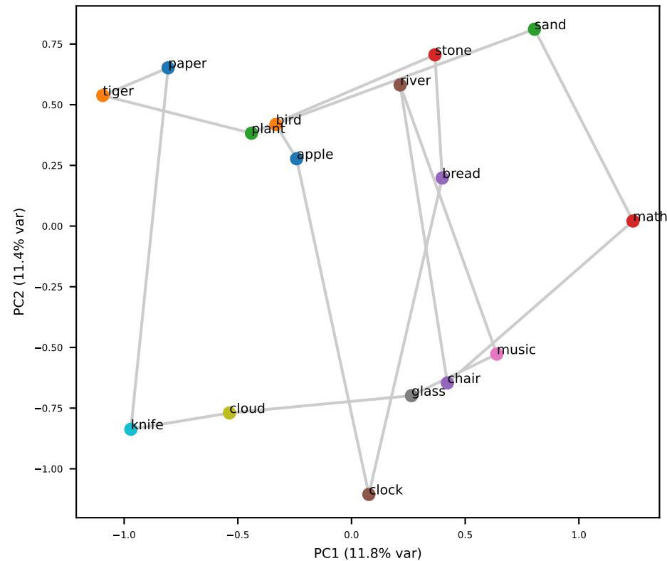
Llama L7 (grid RSA=+0.28)
