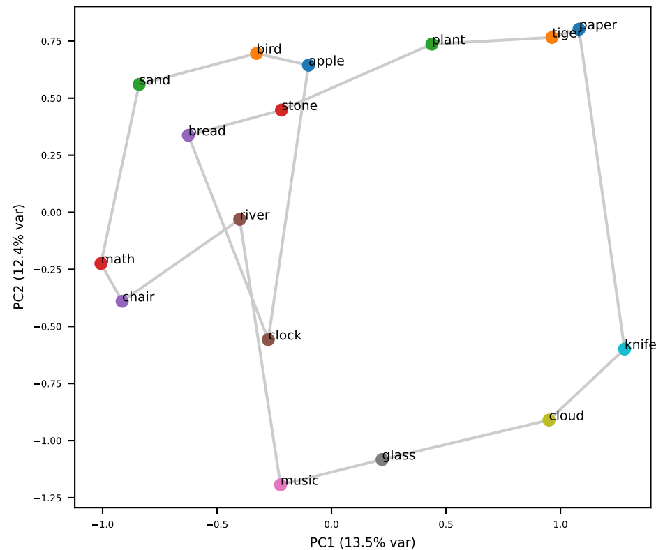
Llama L9 (grid RSA=+0.44)
