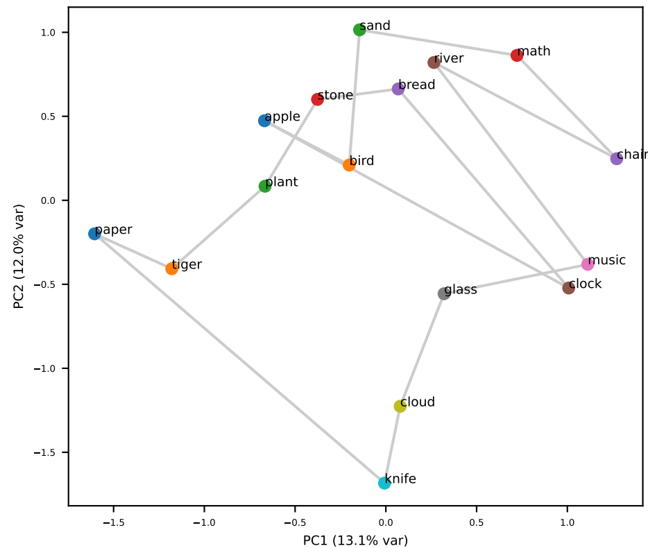
Llama L10 (grid RSA=+0.34)
