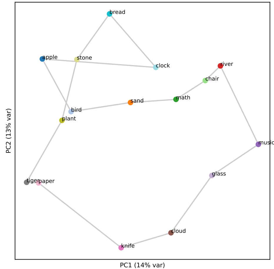
Gemma L19 (RSA 0.53)
