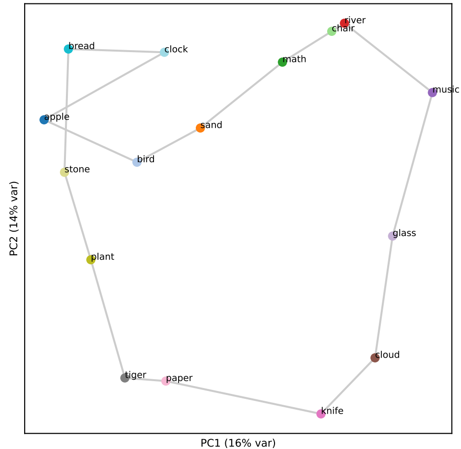
Gemma L24 (RSA 0.69)
