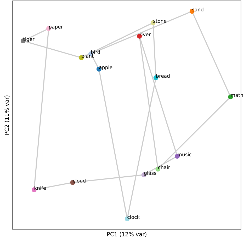
Llama L7 (RSA 0.12)
