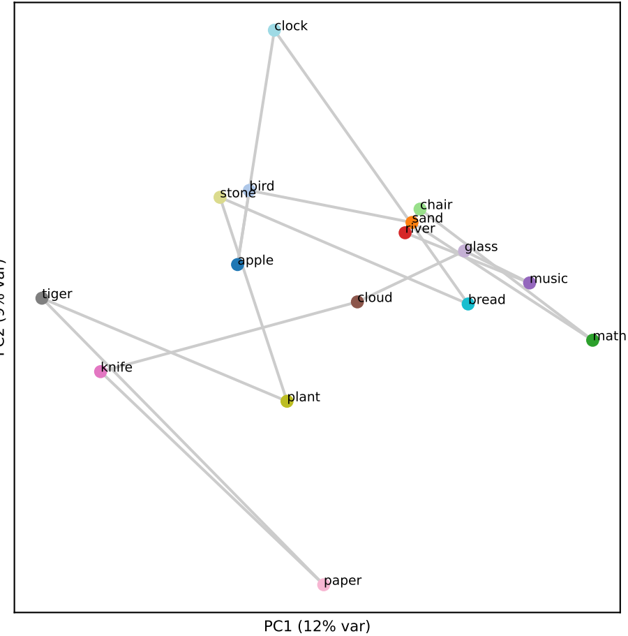
Qwen L26 (RSA 0.17)
