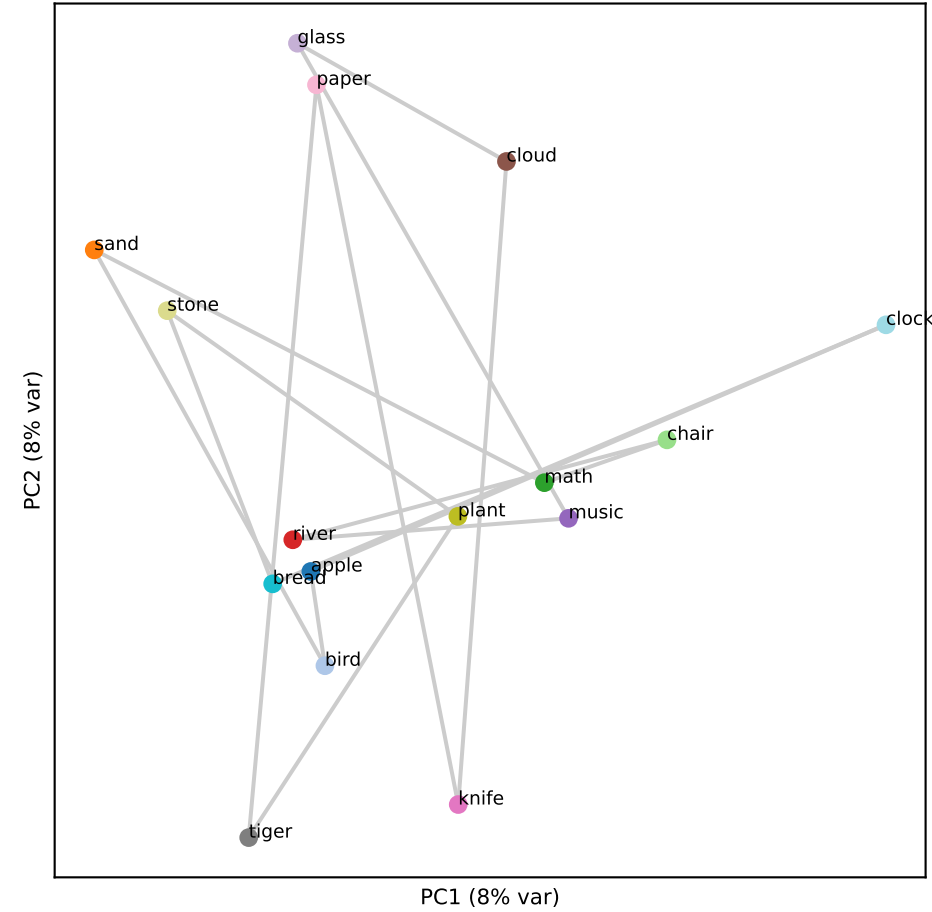
Gemma L0 (RSA -0.01)
