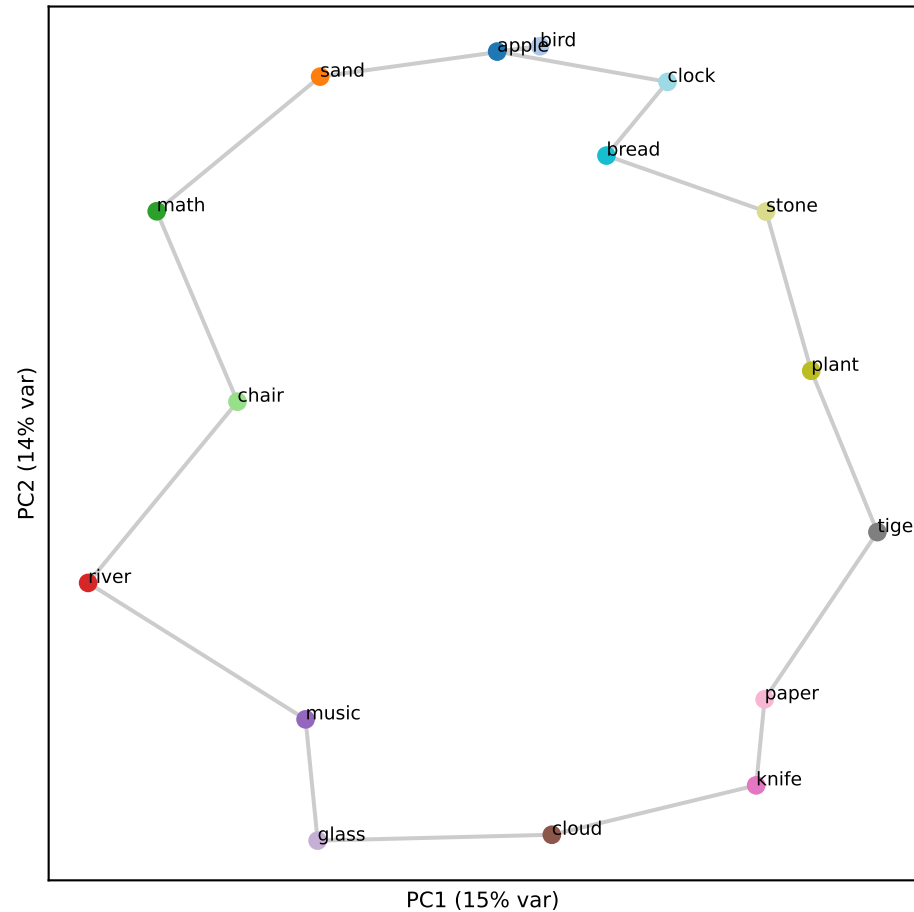
Llama L24 (RSA 0.87)
