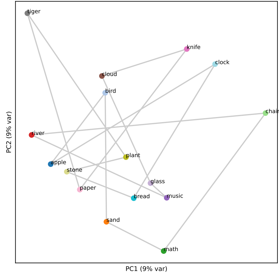
Llama L3 (RSA -0.06)
