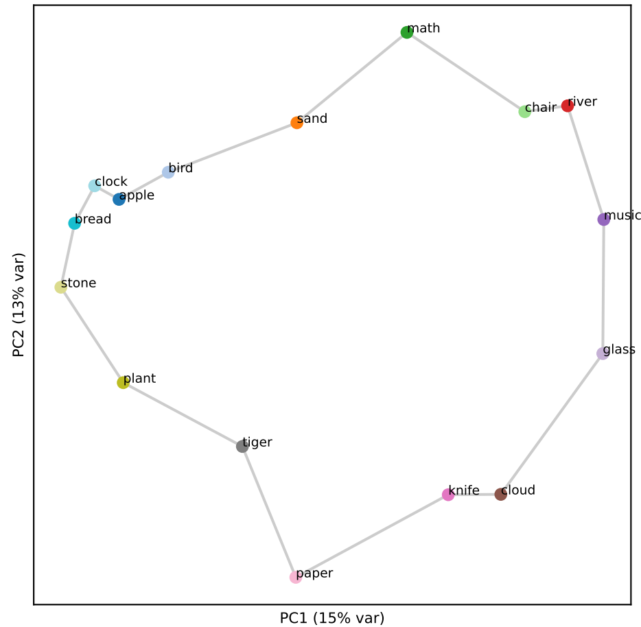
Gemma L34 (RSA 0.86)
