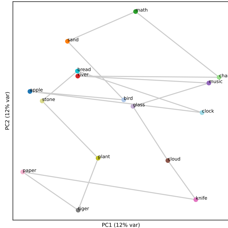
Llama L14 (RSA 0.27)
