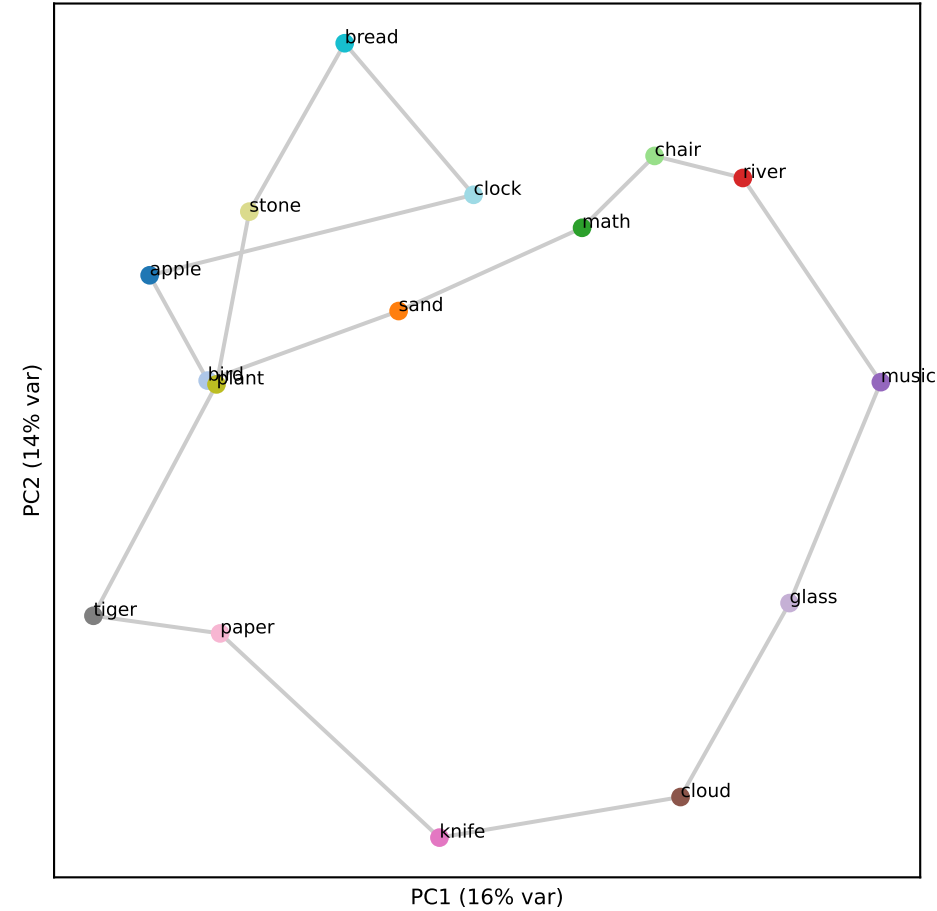
Gemma L17 (RSA 0.51)
