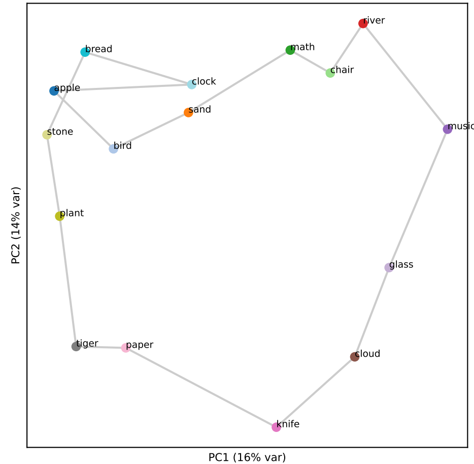
Gemma L26 (RSA 0.66)
