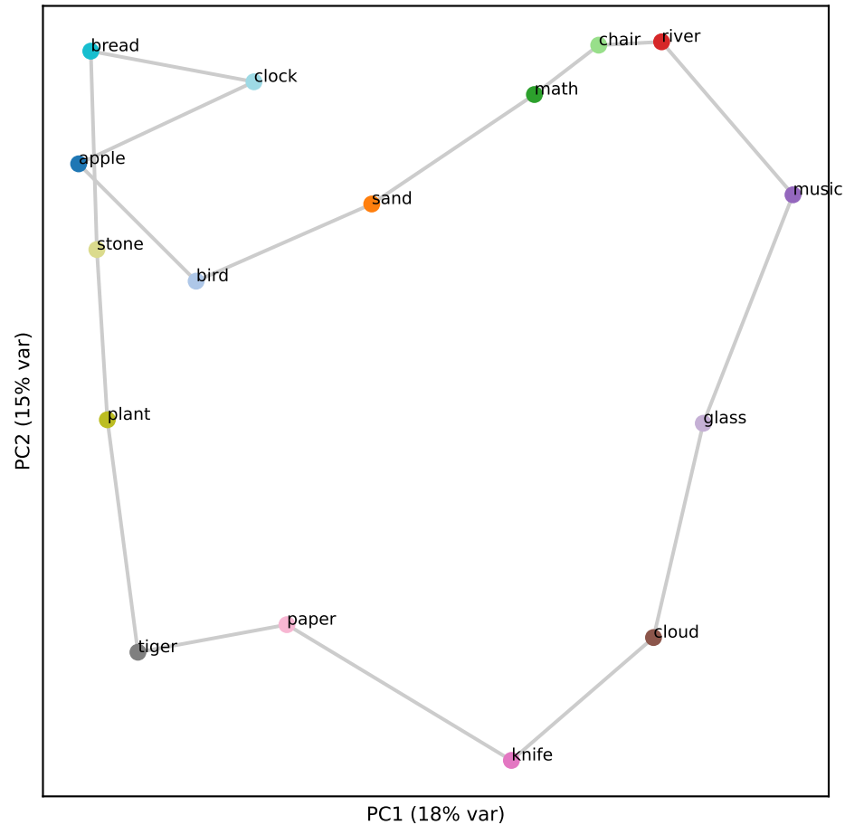
Gemma L21 (RSA 0.70)
