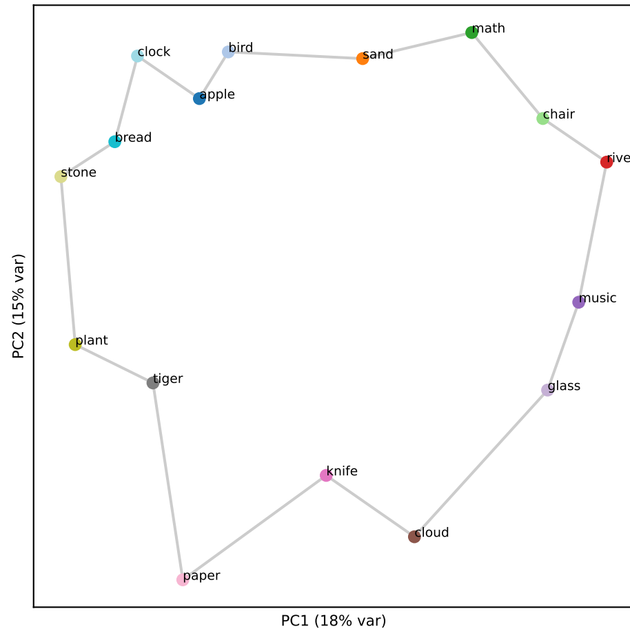
Gemma L35 (RSA 0.87)
