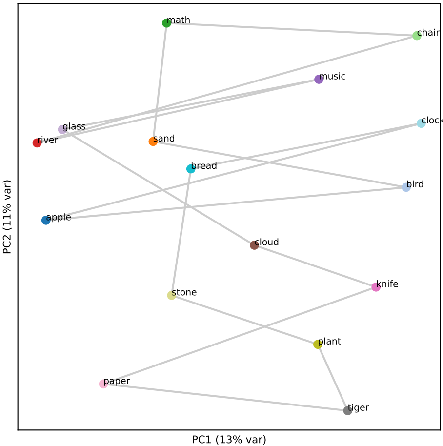
Llama L20 (RSA 0.18)
