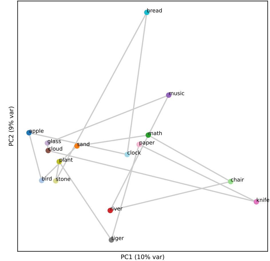
Qwen L4 (RSA -0.06)
