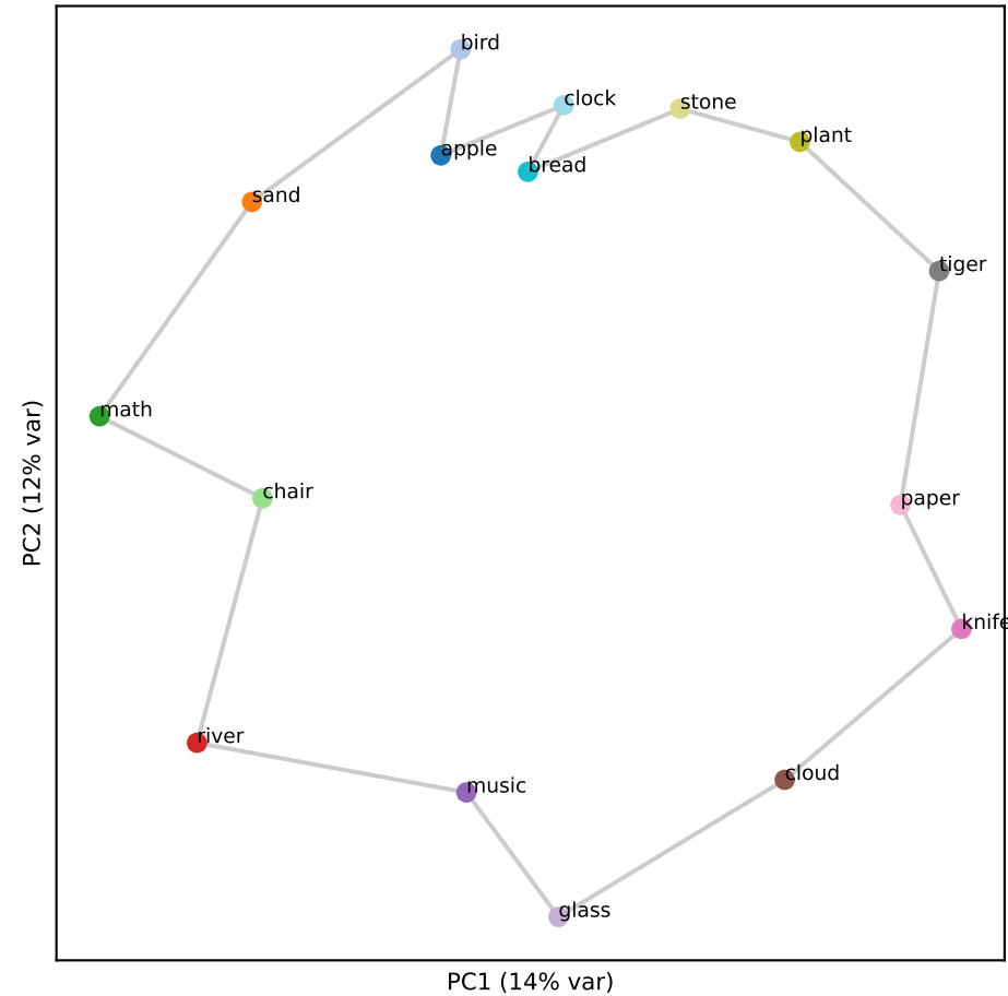
Llama L23 (RSA 0.81)
