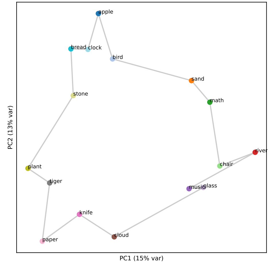
Qwen L31 (RSA 0.83)
