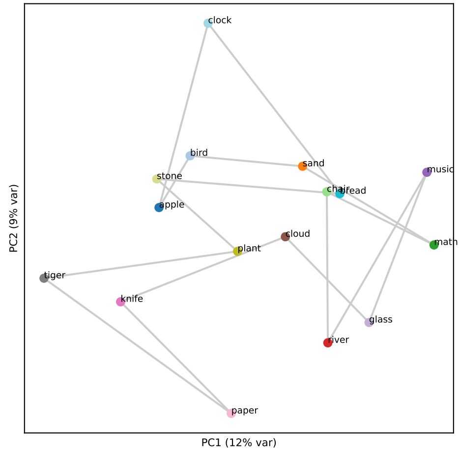
Qwen L28 (RSA 0.23)
