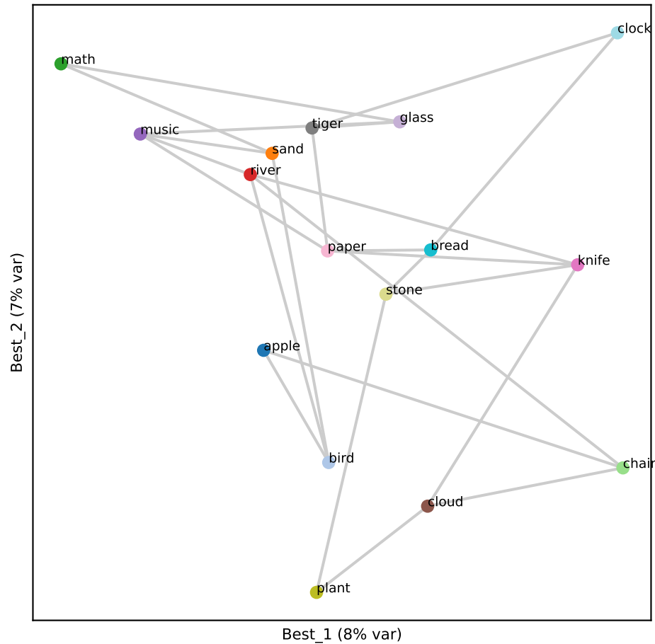
Gemma L2 (RSA 0.41)
