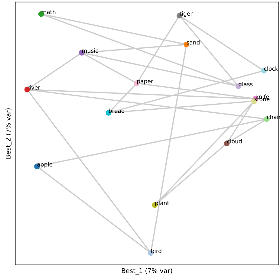
Llama L0 (RSA 0.28)
