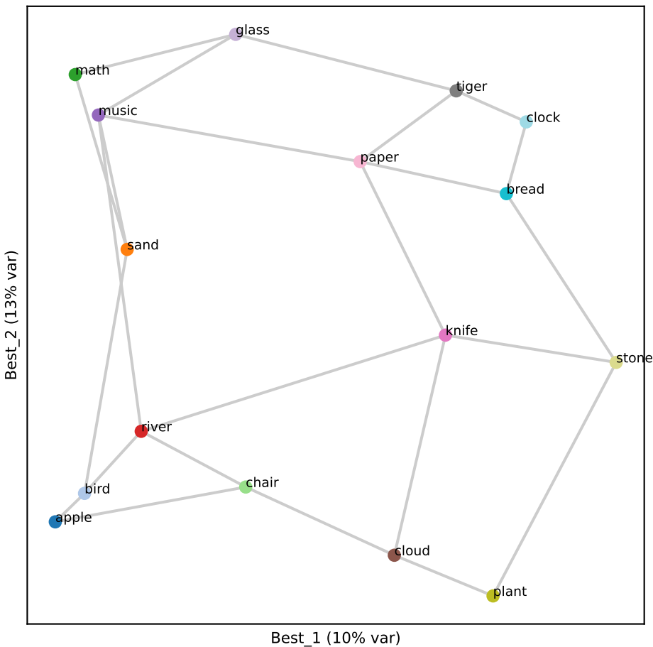
Llama L13 (RSA 0.81)
