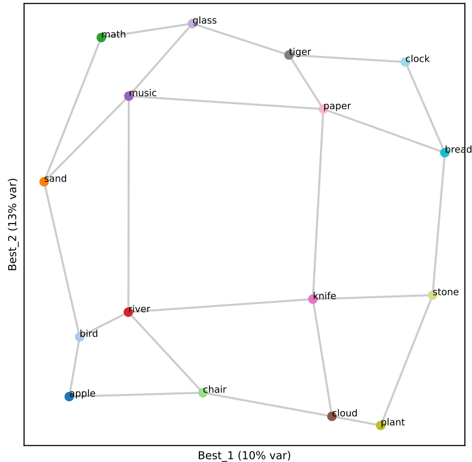
Gemma L34 (RSA 0.88)
