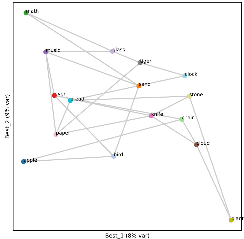
Llama L5 (RSA 0.31)
