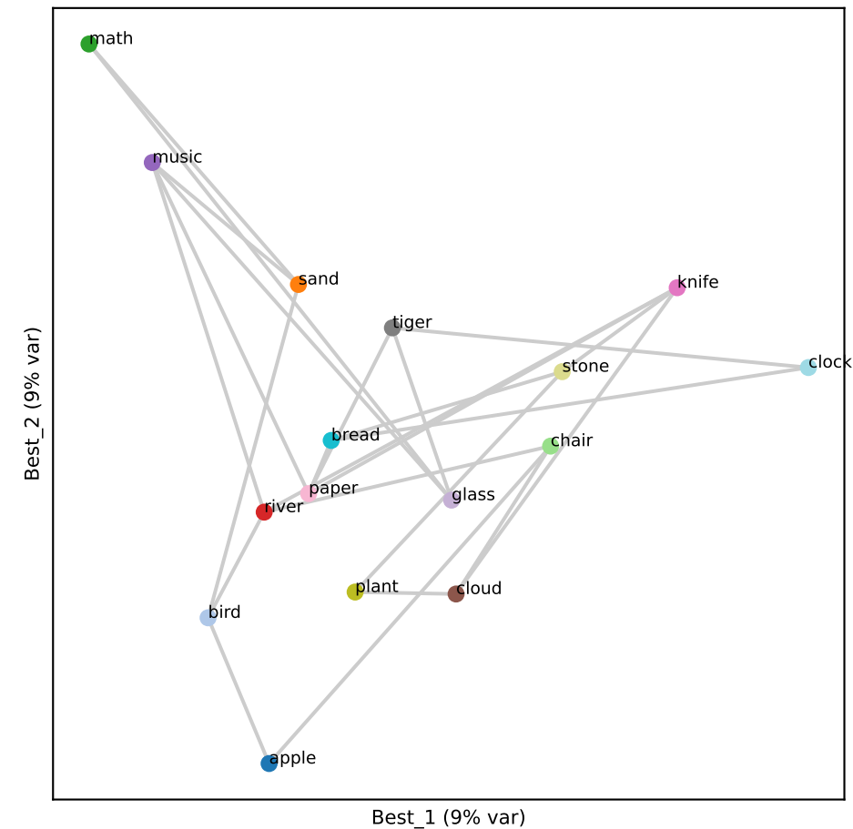
Qwen L9 (RSA 0.14)
