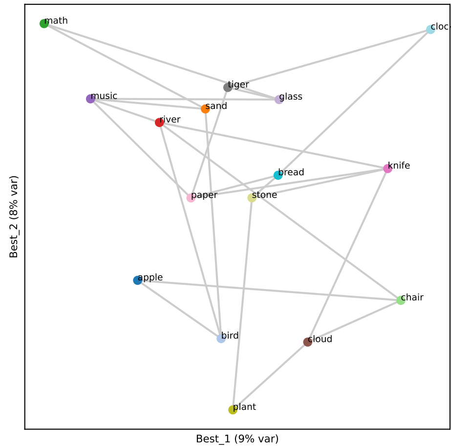
Gemma L4 (RSA 0.41)
