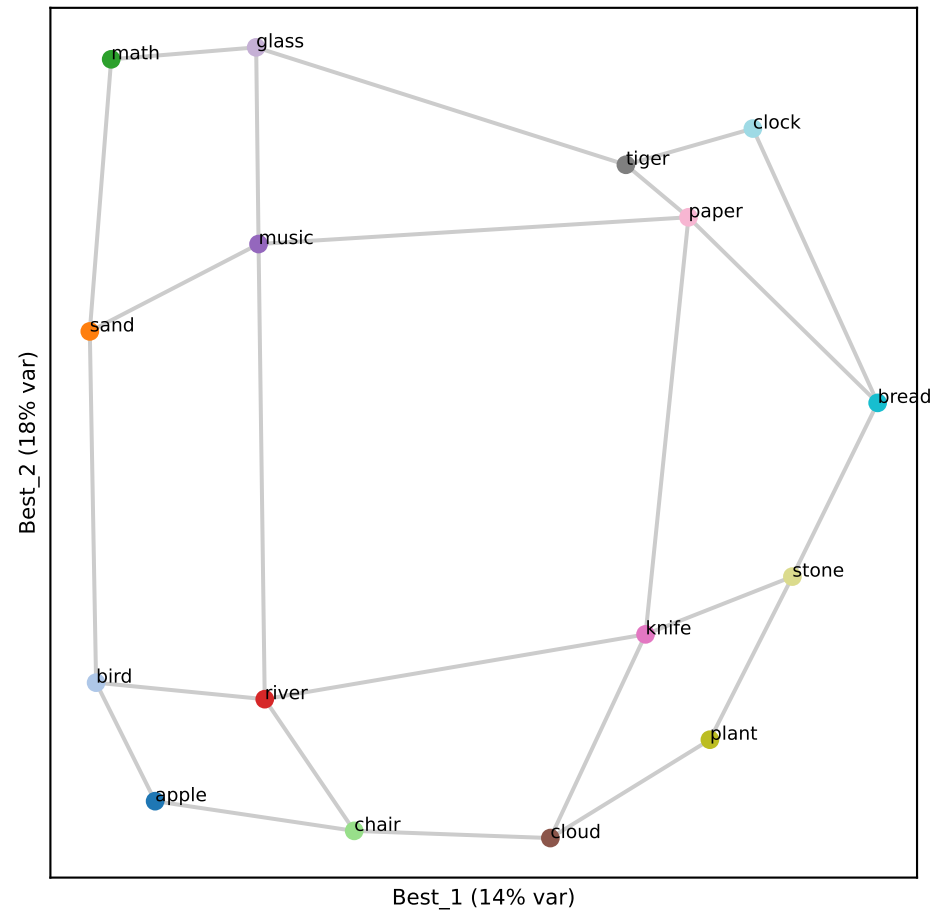
Llama L31 (RSA 0.86)
