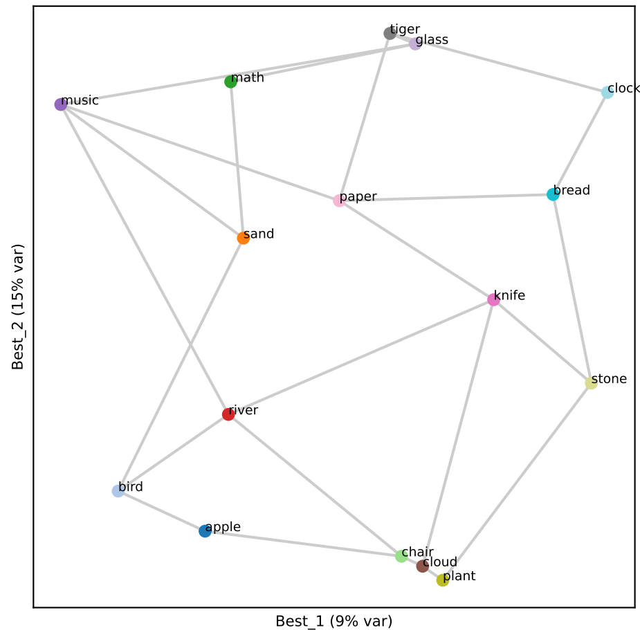
Gemma L17 (RSA 0.67)
