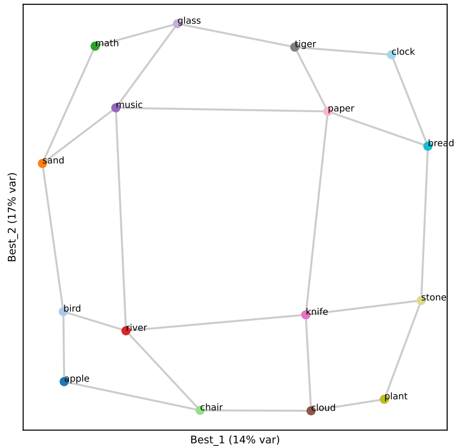
Gemma L37 (RSA 0.88)
