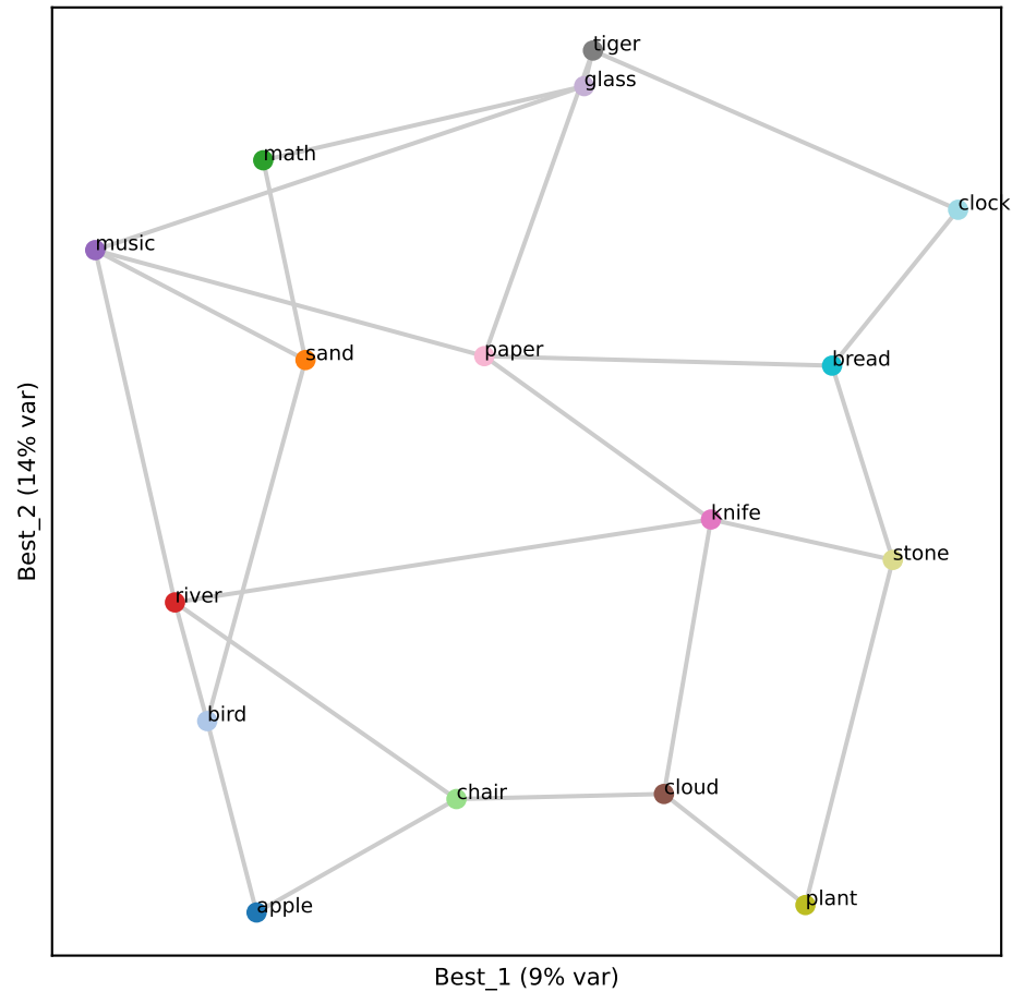
Gemma L27 (RSA 0.76)
