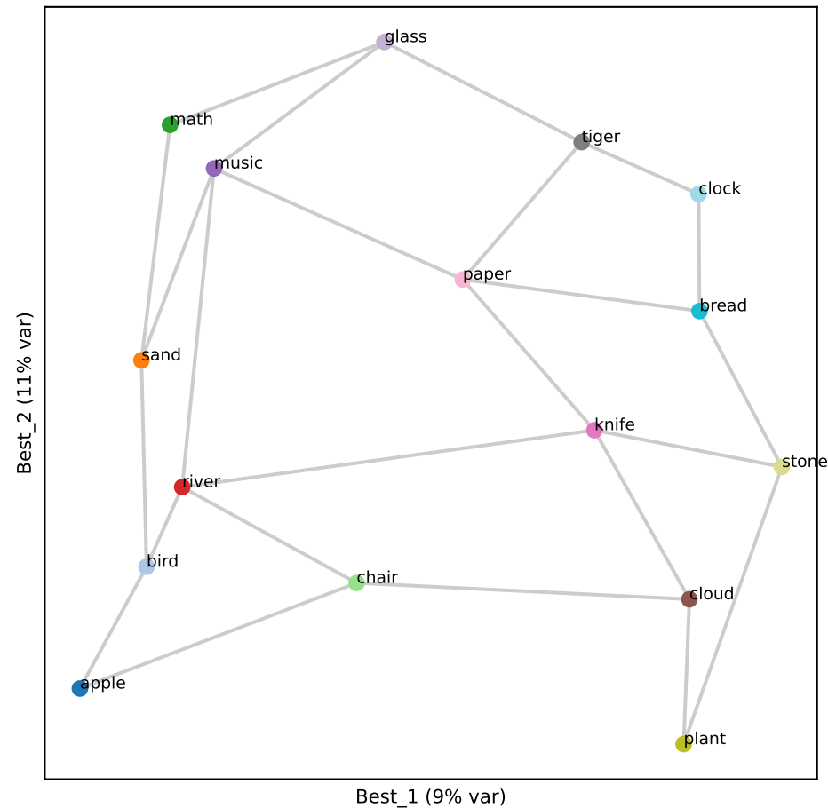
Llama L19 (RSA 0.80)
