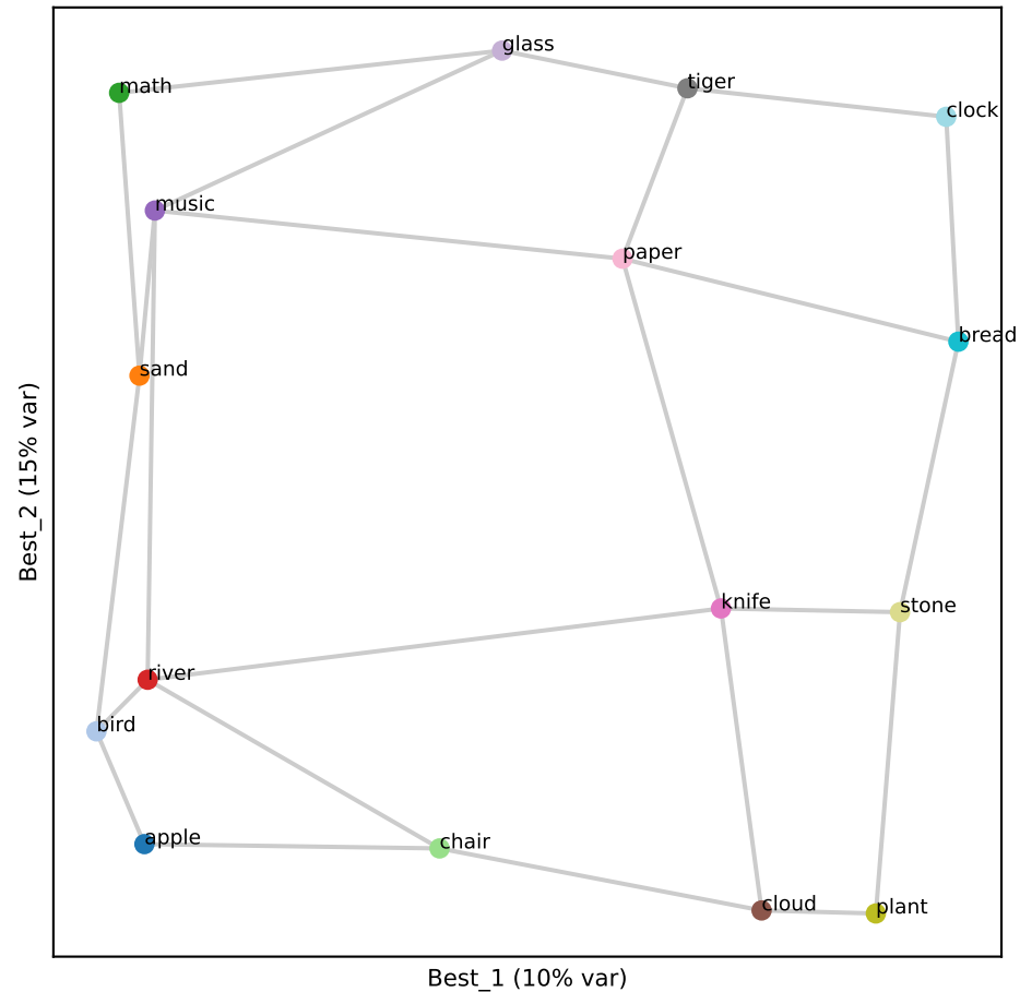
Gemma L29 (RSA 0.84)
