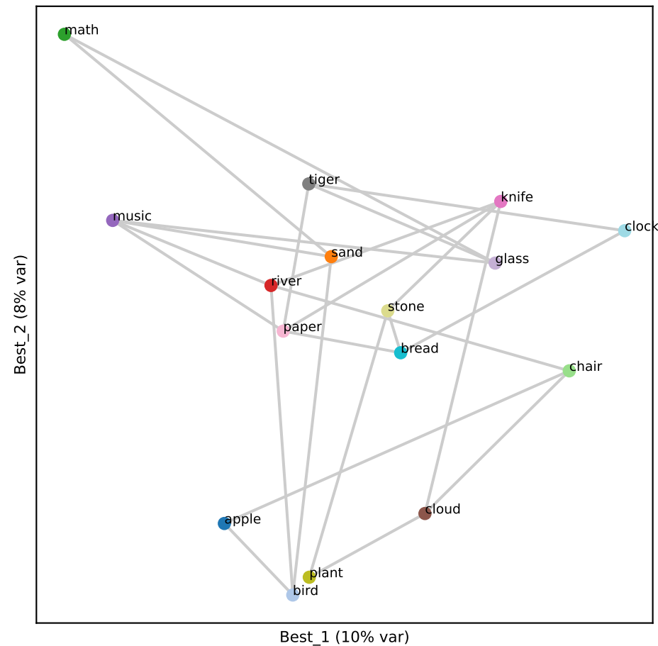
Gemma L10 (RSA 0.27)
