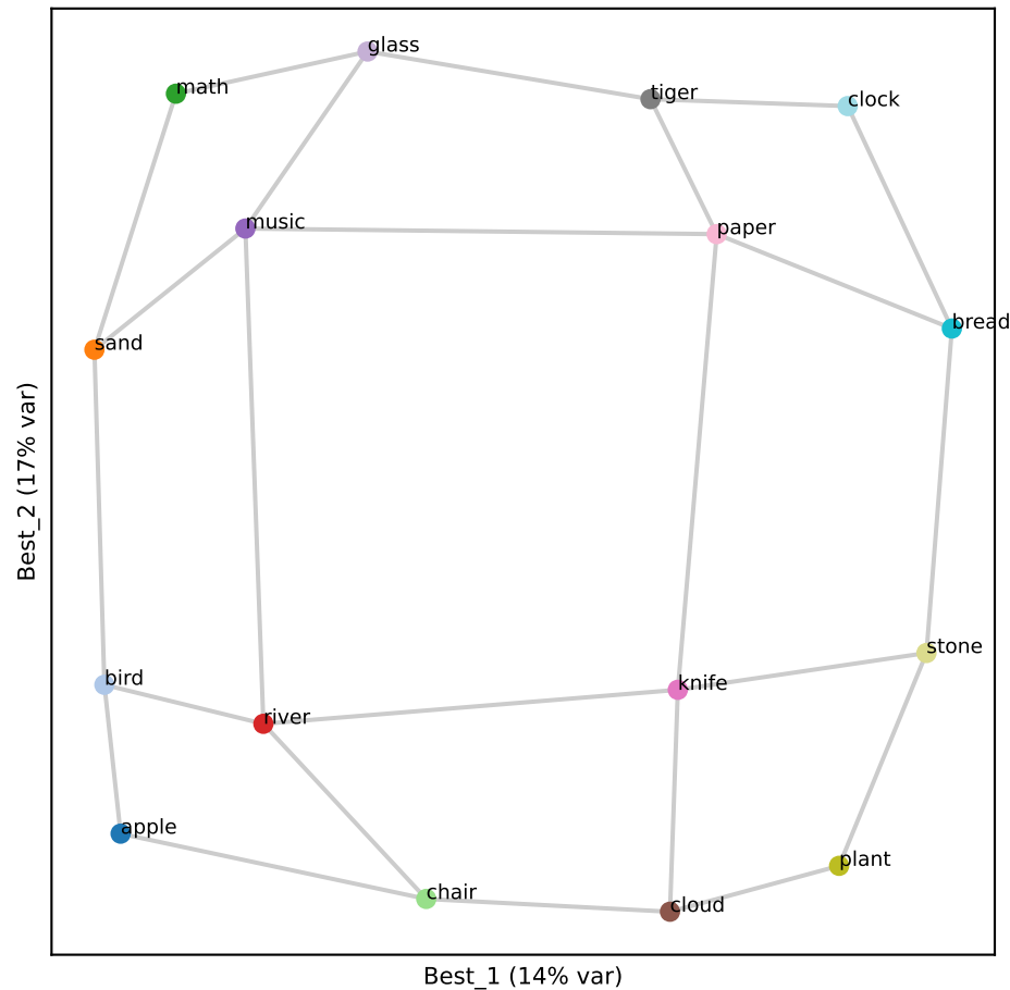
Gemma L38 (RSA 0.88)
