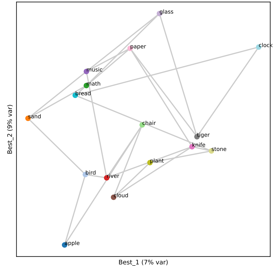
Qwen L28 (RSA 0.40)
