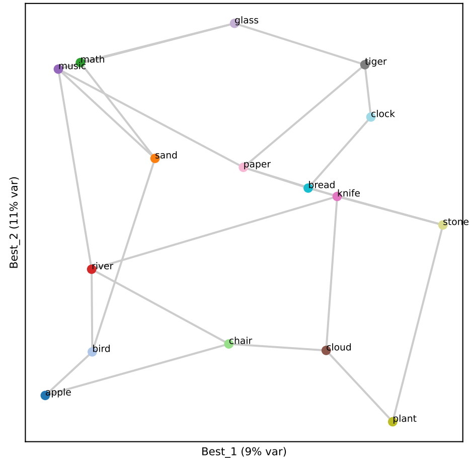
Llama L14 (RSA 0.68)
