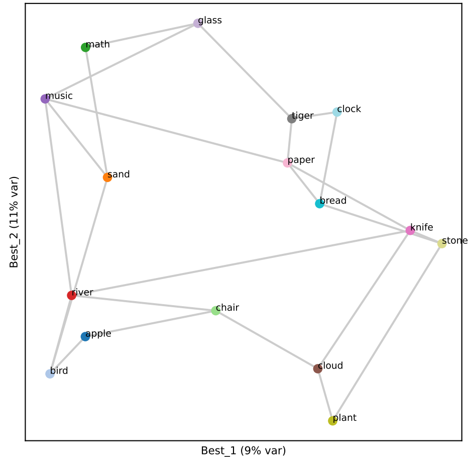
Llama L10 (RSA 0.67)
