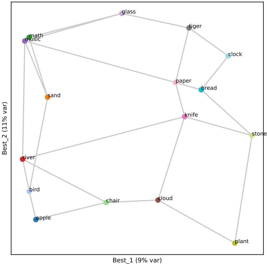
Llama L15 (RSA 0.77)
