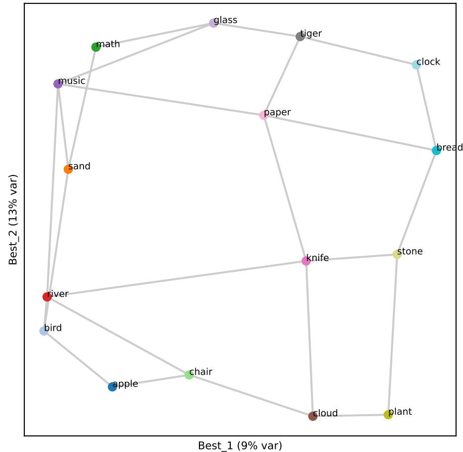
Gemma L28 (RSA 0.81)
