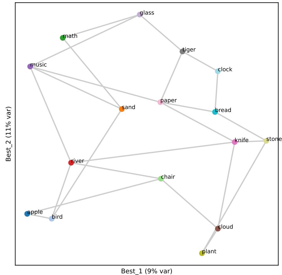
Llama L8 (RSA 0.62)
