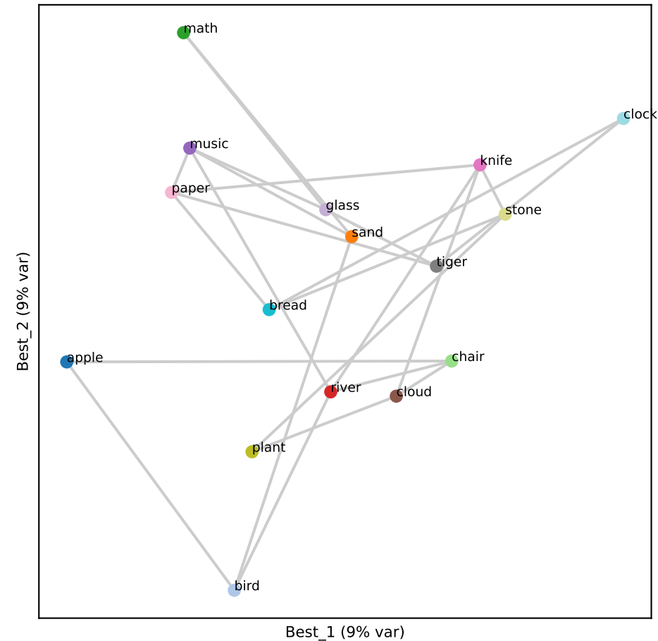
Qwen L13 (RSA 0.23)
