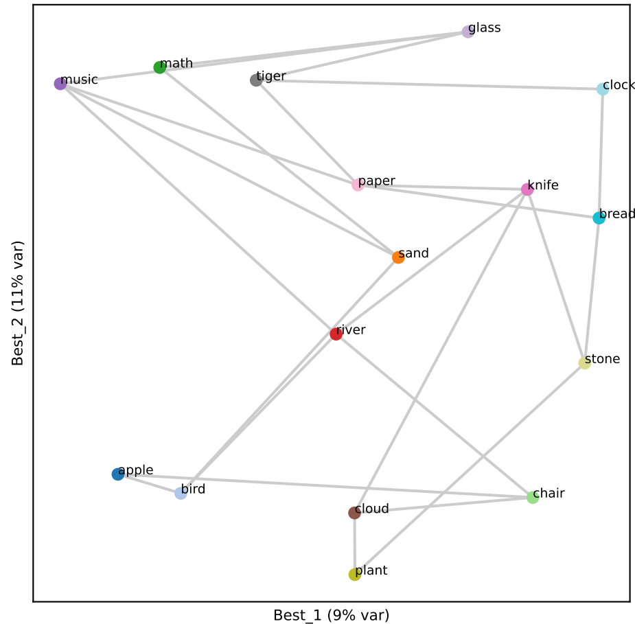
Gemma L15 (RSA 0.51)
