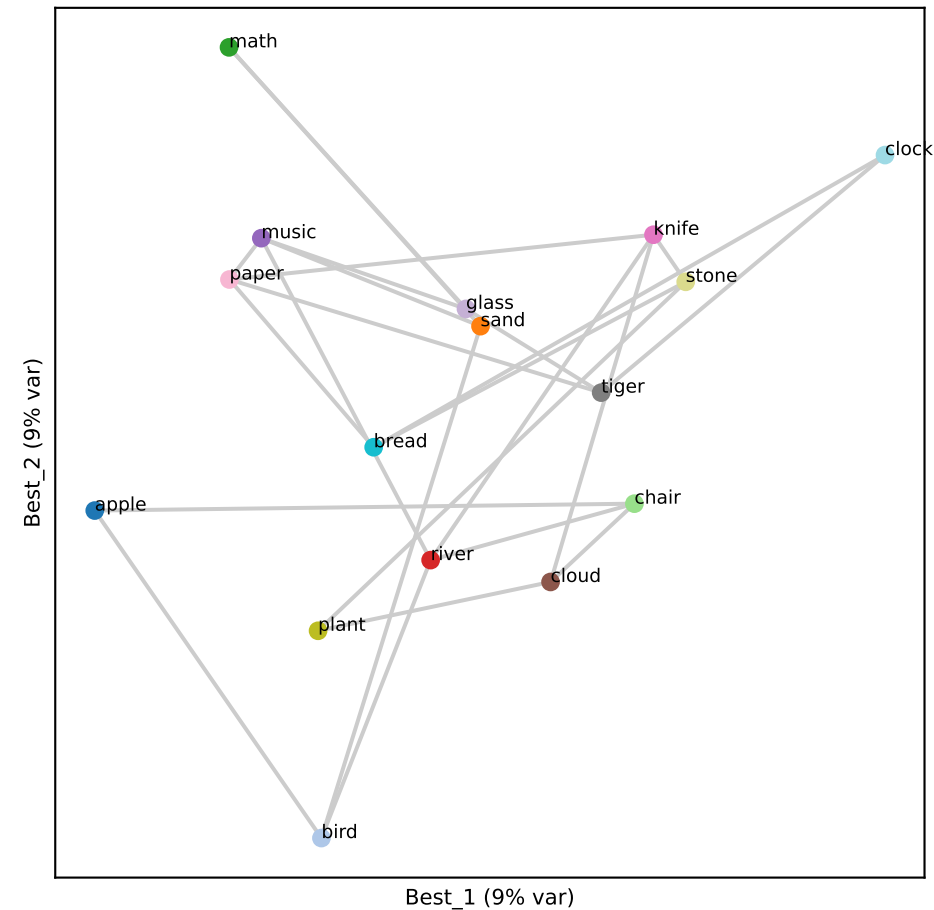
Qwen L12 (RSA 0.22)
