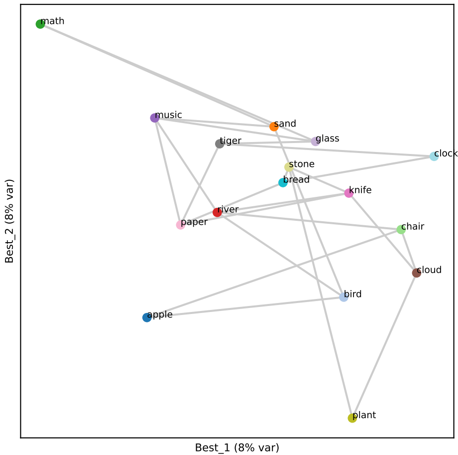
Llama L3 (RSA 0.33)
