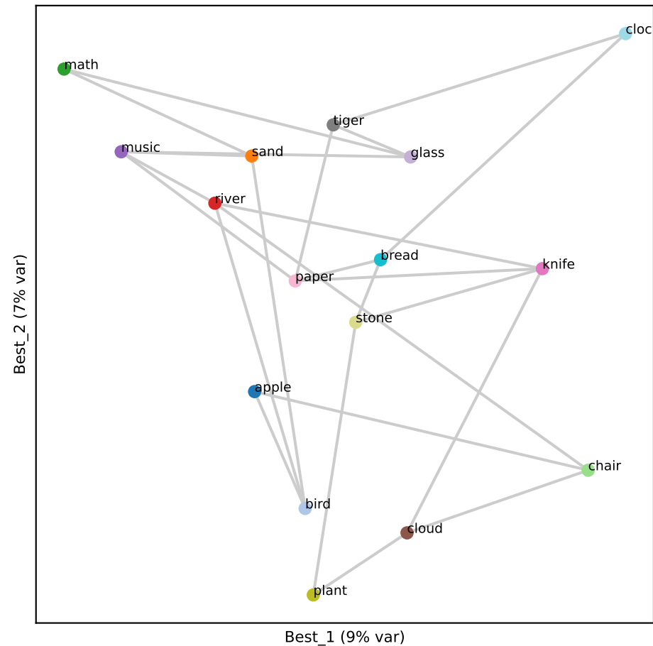
Gemma L3 (RSA 0.41)
