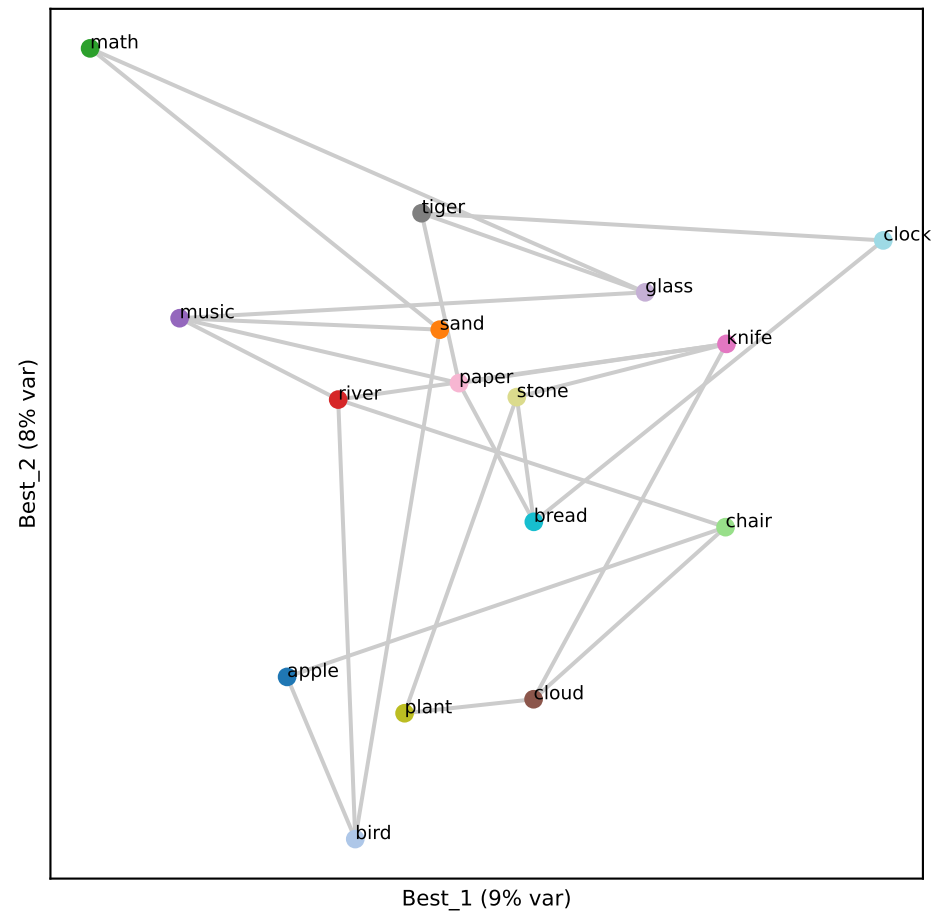
Gemma L6 (RSA 0.35)
