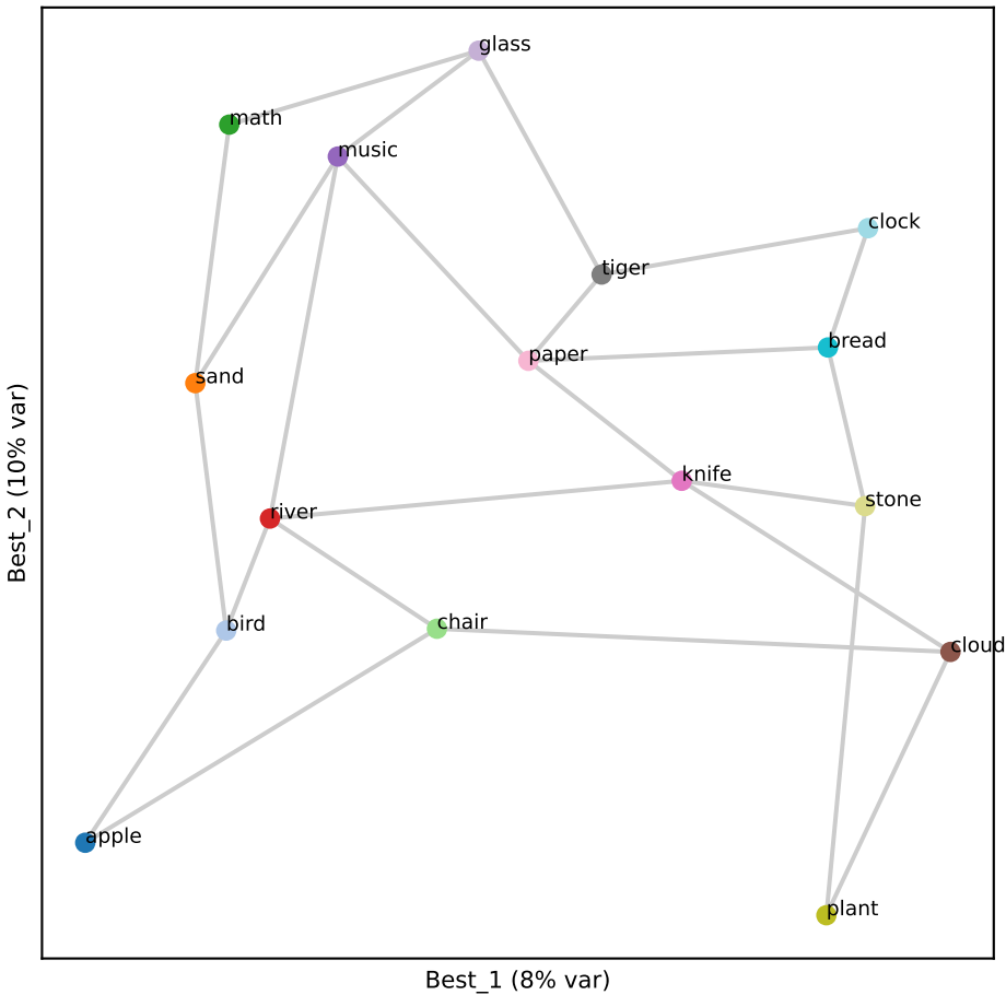
Llama L20 (RSA 0.72)
