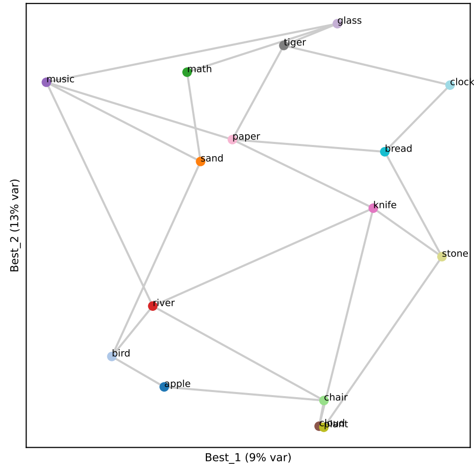
Gemma L19 (RSA 0.61)
