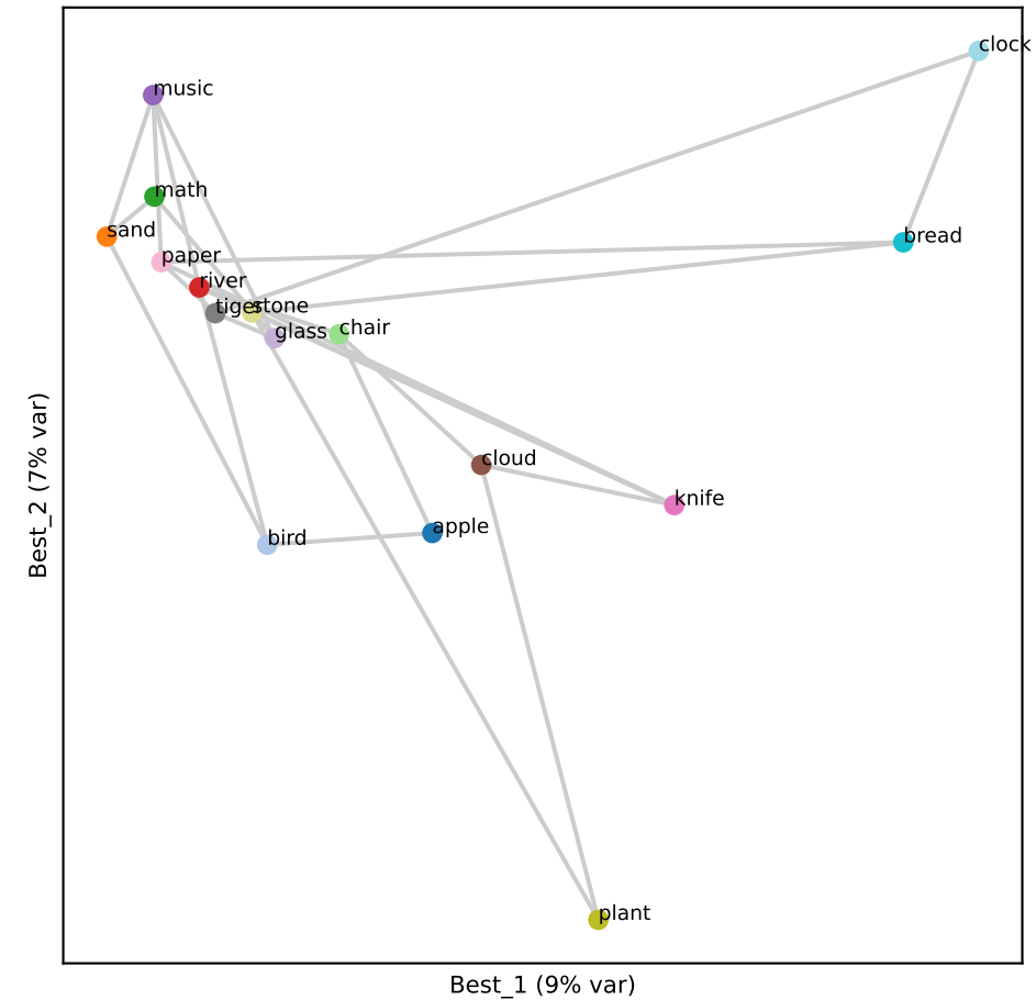
Qwen L2 (RSA 0.25)
