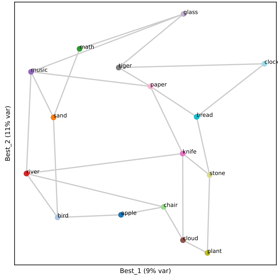
Gemma L30 (RSA 0.63)
