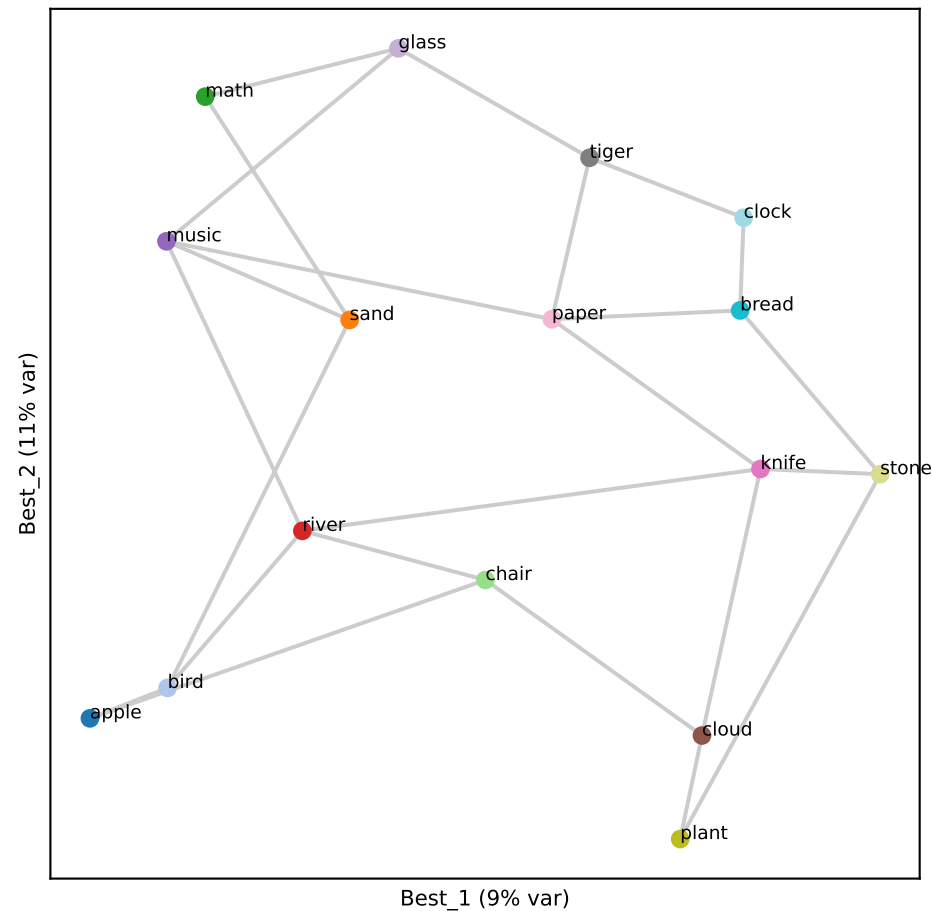
Llama L9 (RSA 0.71)
