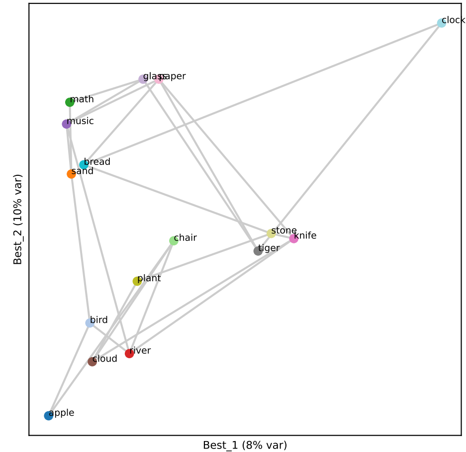
Qwen L26 (RSA 0.32)
