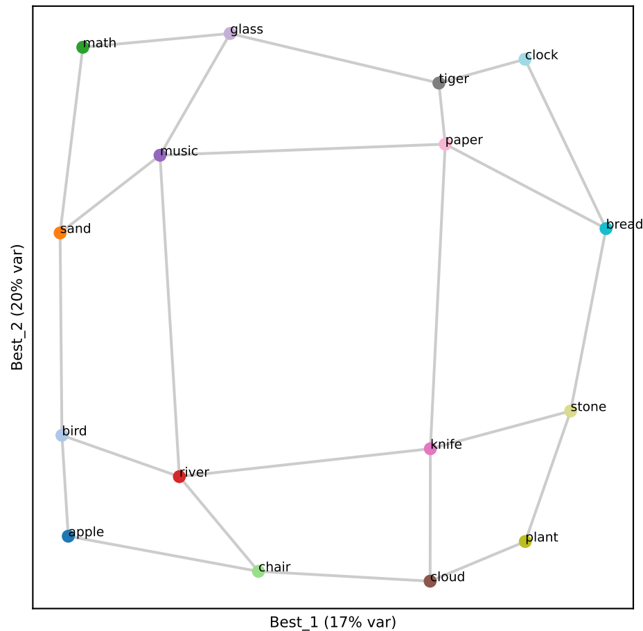
Gemma L40 (RSA 0.89)
