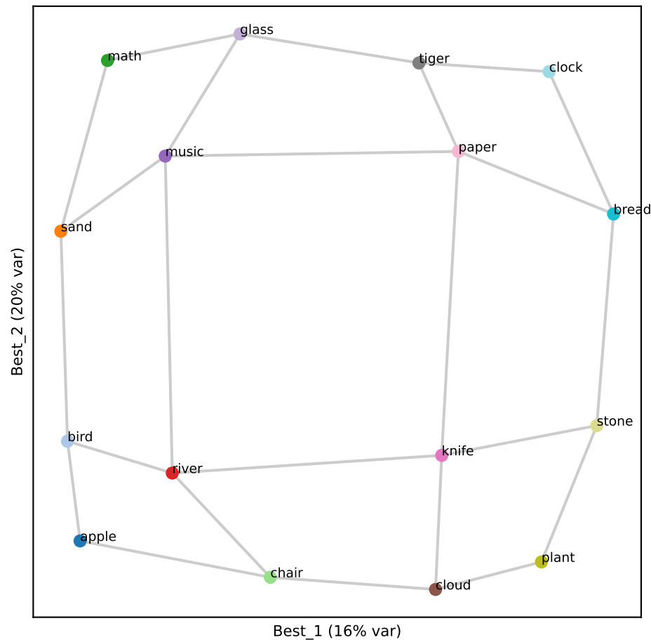
Gemma L39 (RSA 0.88)
