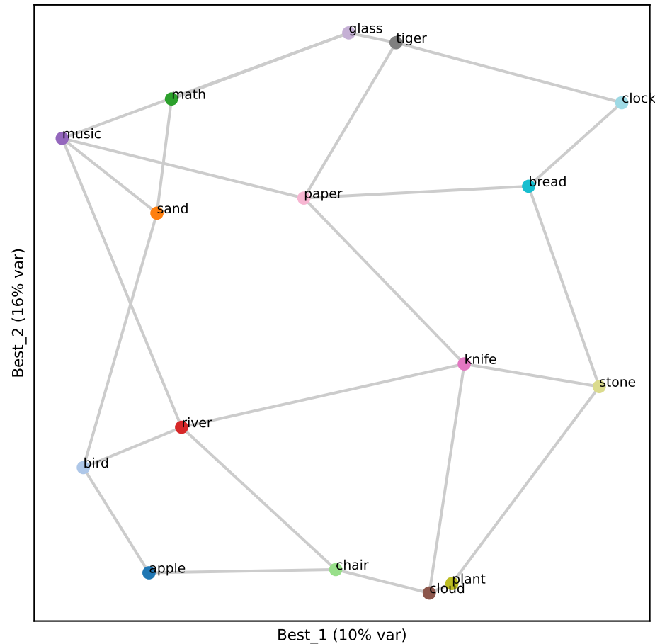
Gemma L23 (RSA 0.77)
