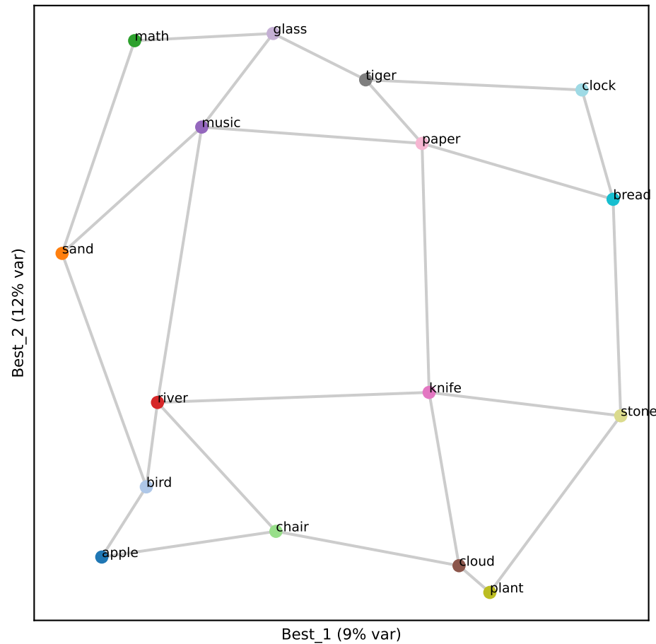
Gemma L32 (RSA 0.85)
