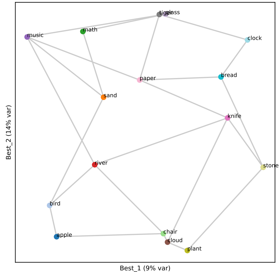
Gemma L16 (RSA 0.68)
