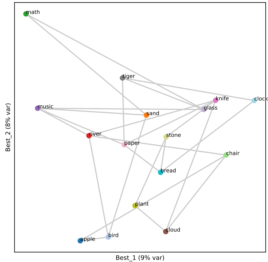
Gemma L7 (RSA 0.26)
