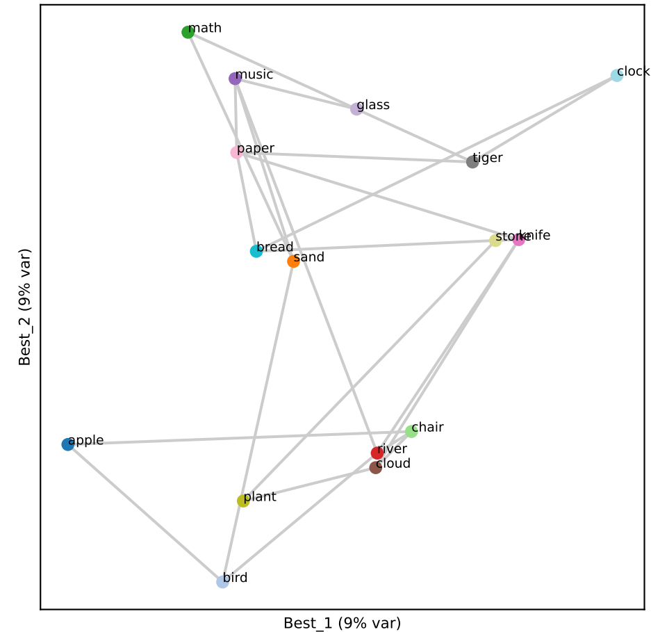
Qwen L19 (RSA 0.46)
