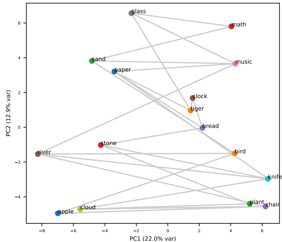
Llama L24 (grid RSA=+0.35)
