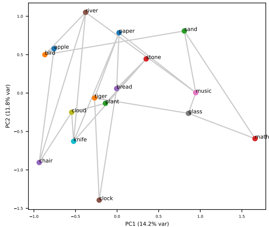
Llama L7 (grid RSA=+0.38)
