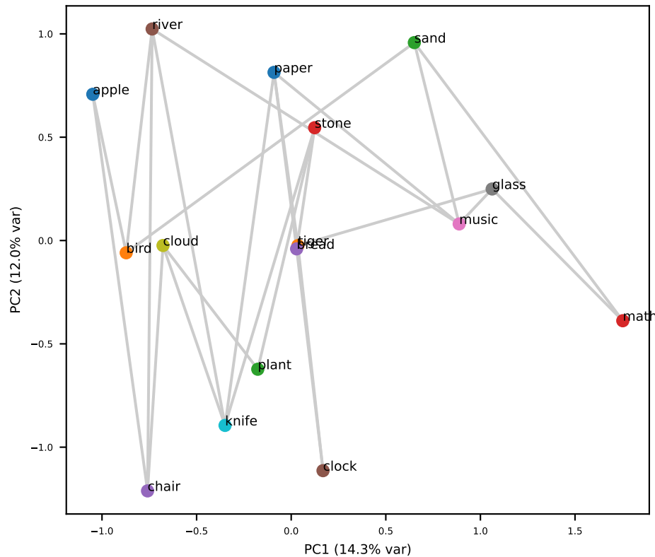
Llama L9 (grid RSA=+0.46)
