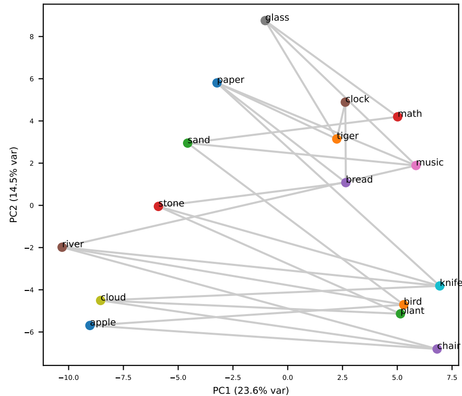
Llama L26 (grid RSA=+0.38)
