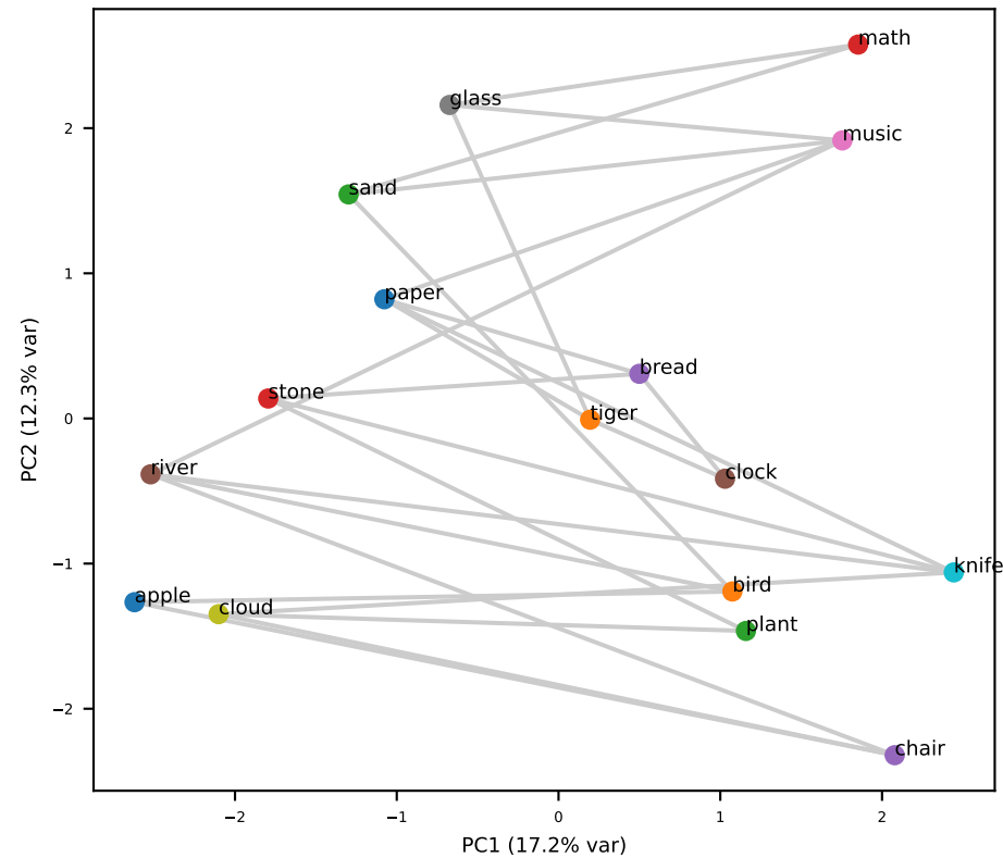
Llama L15 (grid RSA=+0.29)
