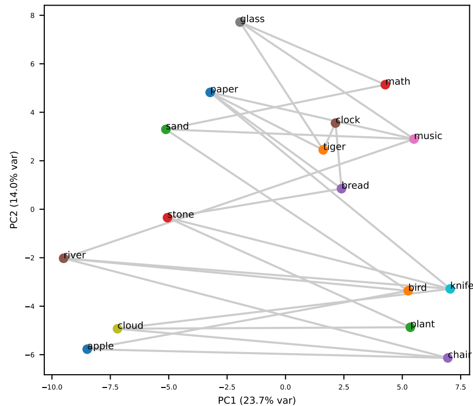
Llama L25 (grid RSA=+0.37)
