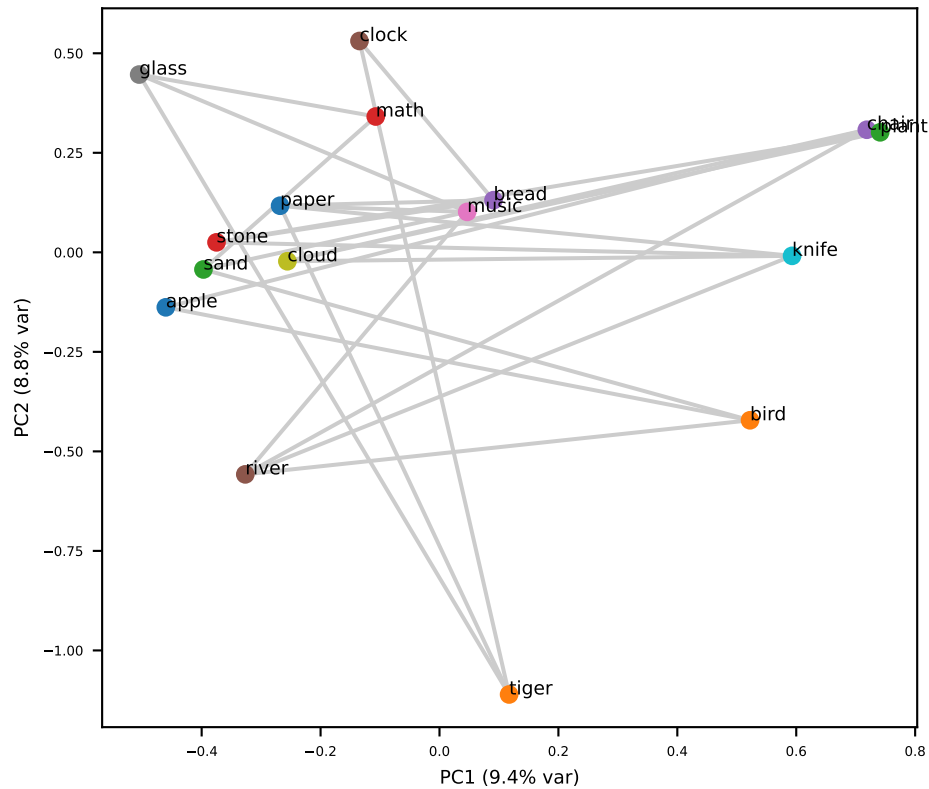
Llama L1 (grid RSA=+0.20)
