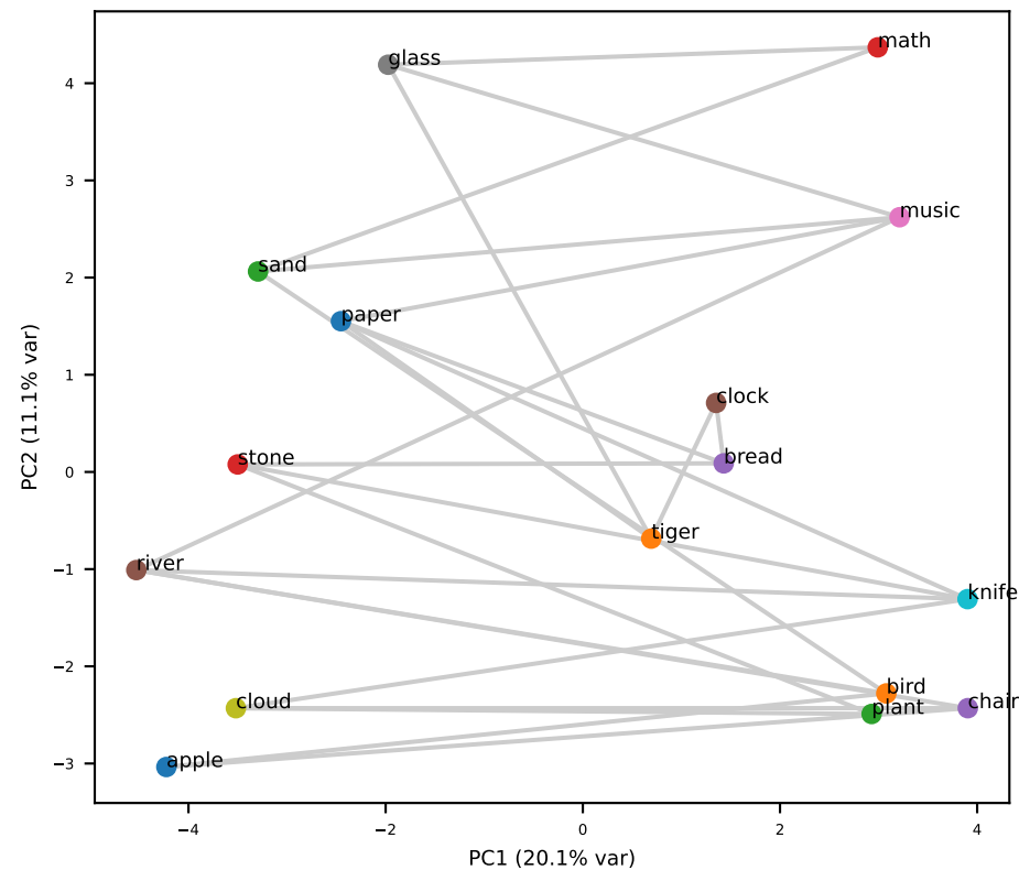
Llama L20 (grid RSA=+0.22)
