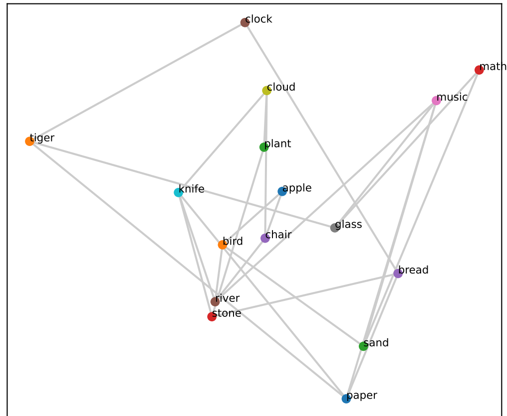
Qwen L9 (grid RSA=0.10, PCA corr=0.05)
