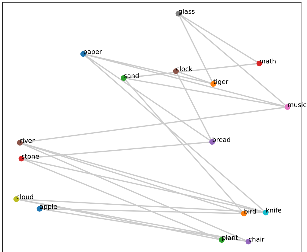
Gemma L35 (grid RSA=0.56, PCA corr=0.24)
