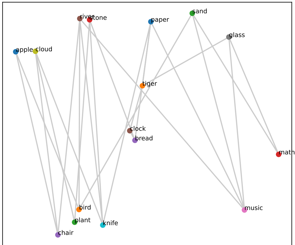
Gemma L30 (grid RSA=0.38, PCA corr=0.22)
