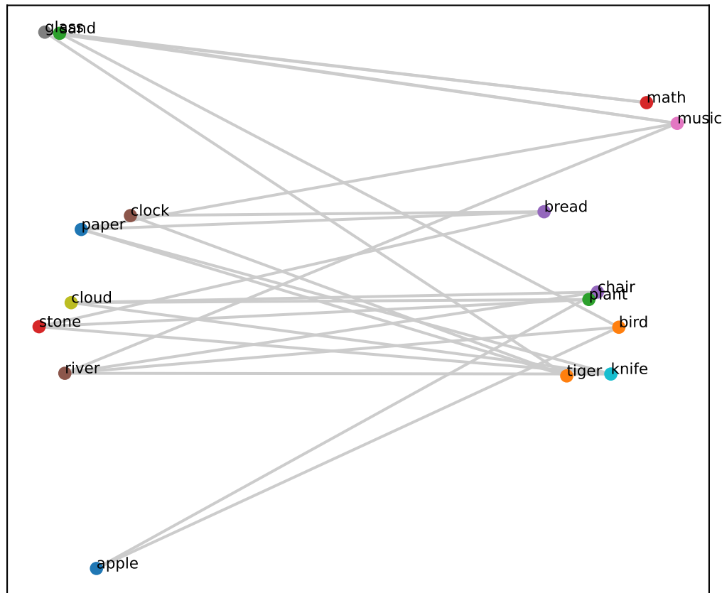
Qwen L28 (grid RSA=0.09, PCA corr=-0.01)
