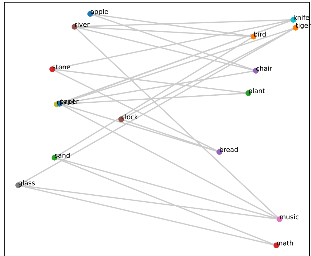
Qwen L20 (grid RSA=0.15, PCA corr=-0.04)
