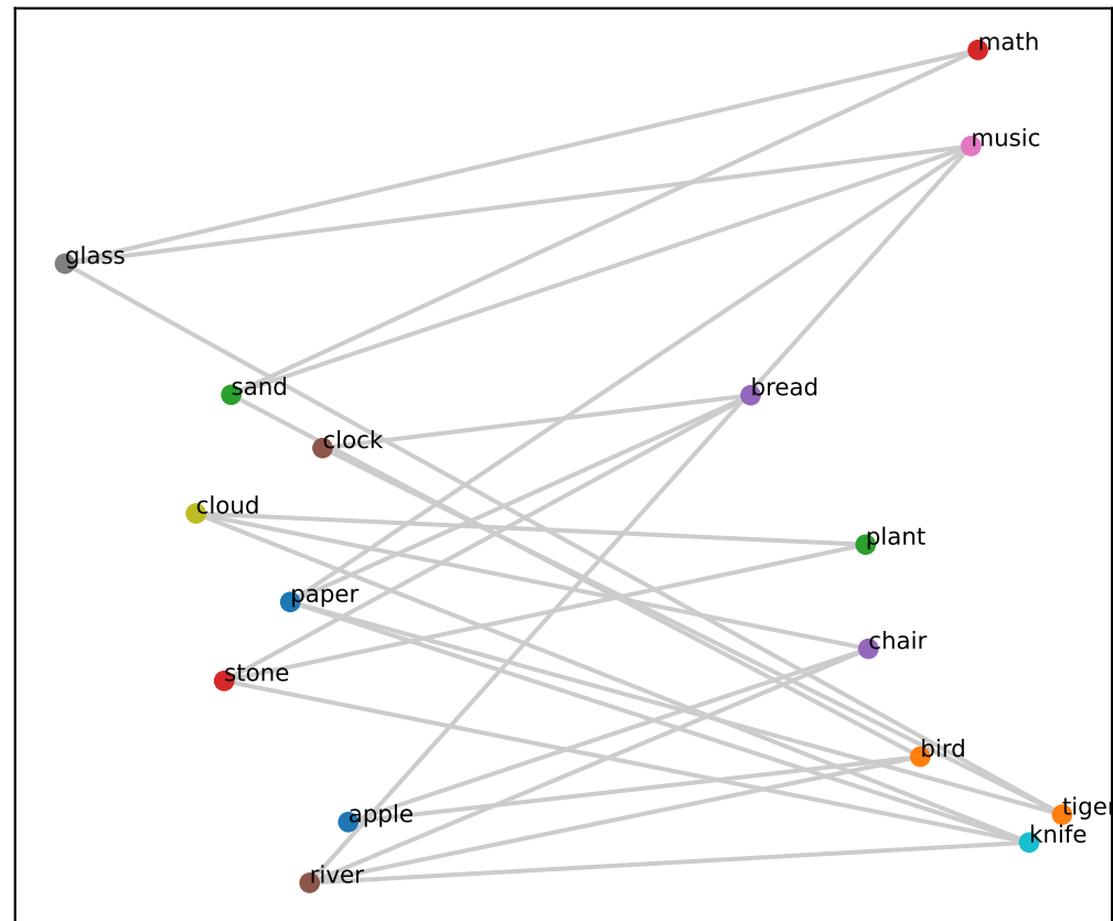
Qwen L21 (grid RSA=0.14, PCA corr=-0.06)
