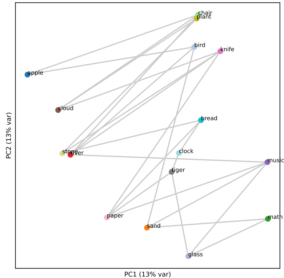
Gemma L31 (RSA 0.26)
