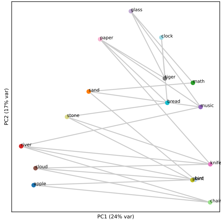
Llama L28 (RSA 0.19)
