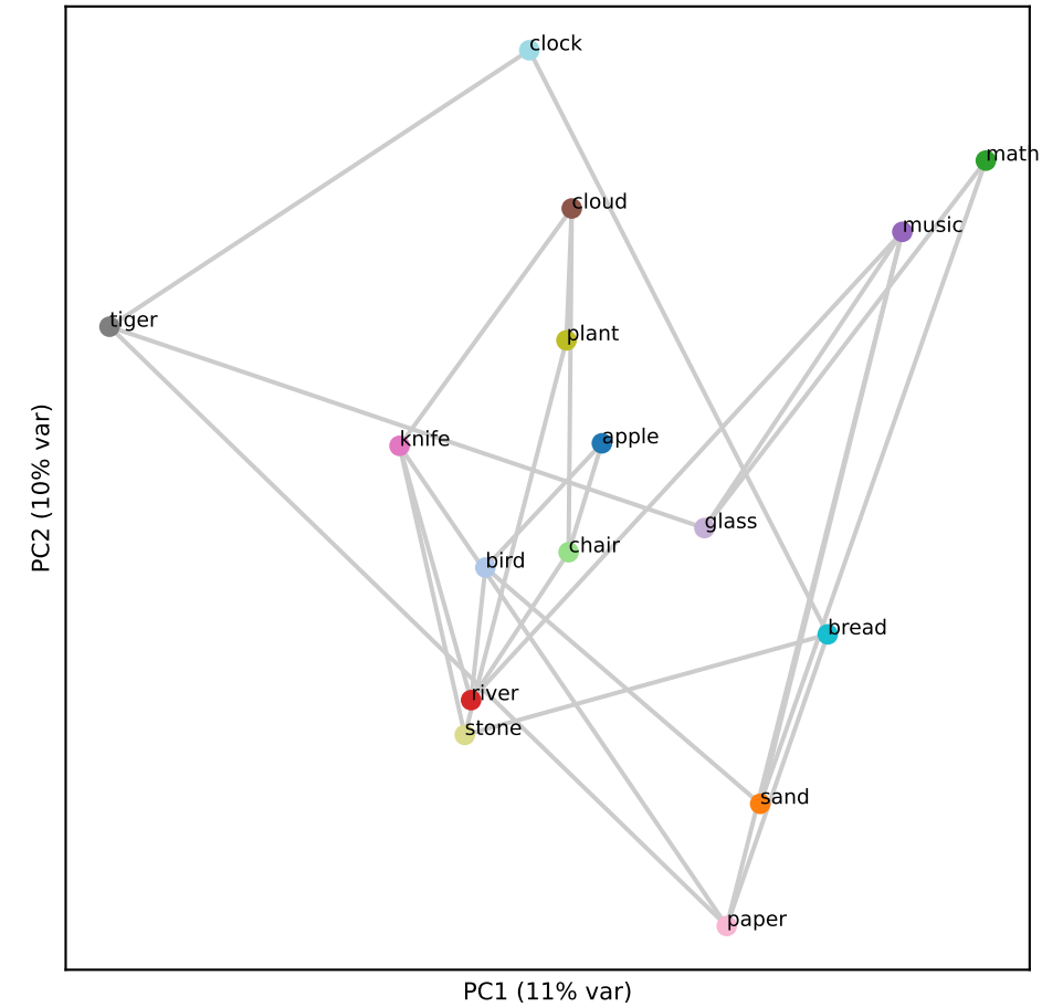
Qwen L9 (RSA 0.09)
