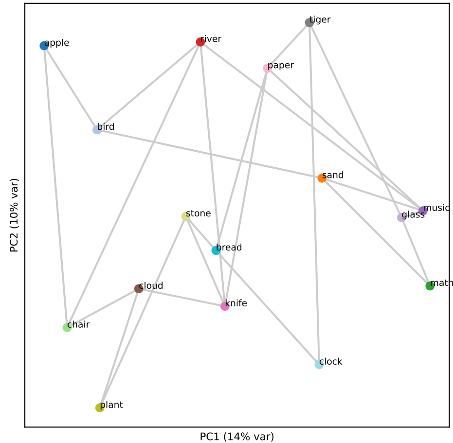
Gemma L19 (RSA 0.43)
