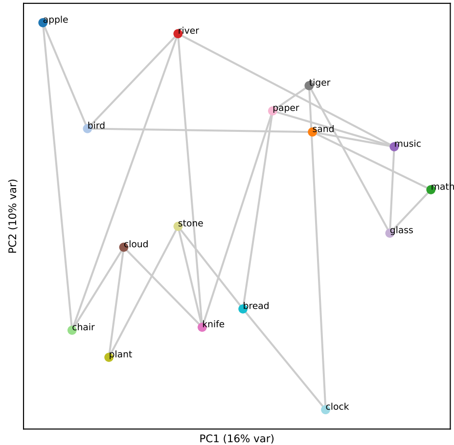
Gemma L18 (RSA 0.55)
