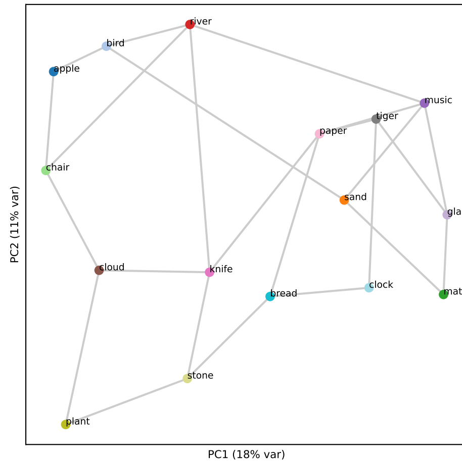
Gemma L21 (RSA 0.60)
