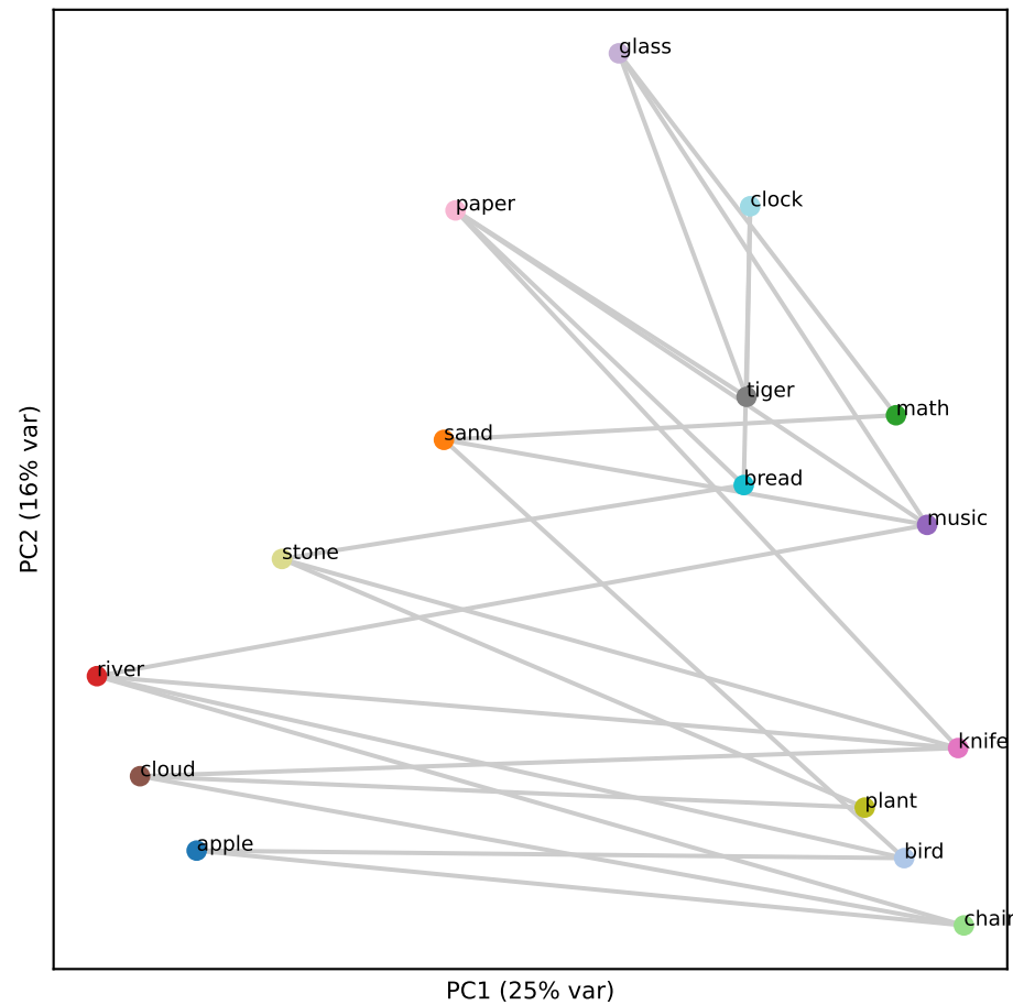
Llama L27 (RSA 0.16)
