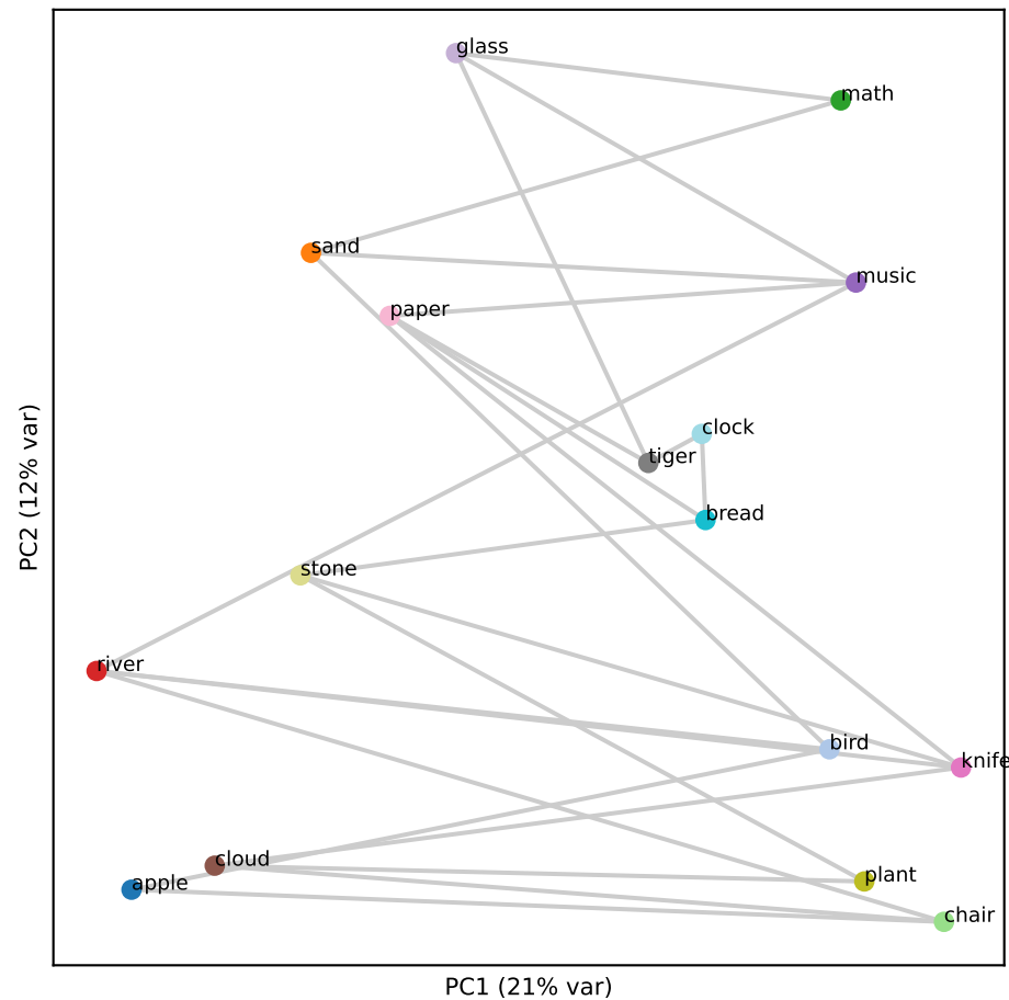
Llama L23 (RSA 0.18)
