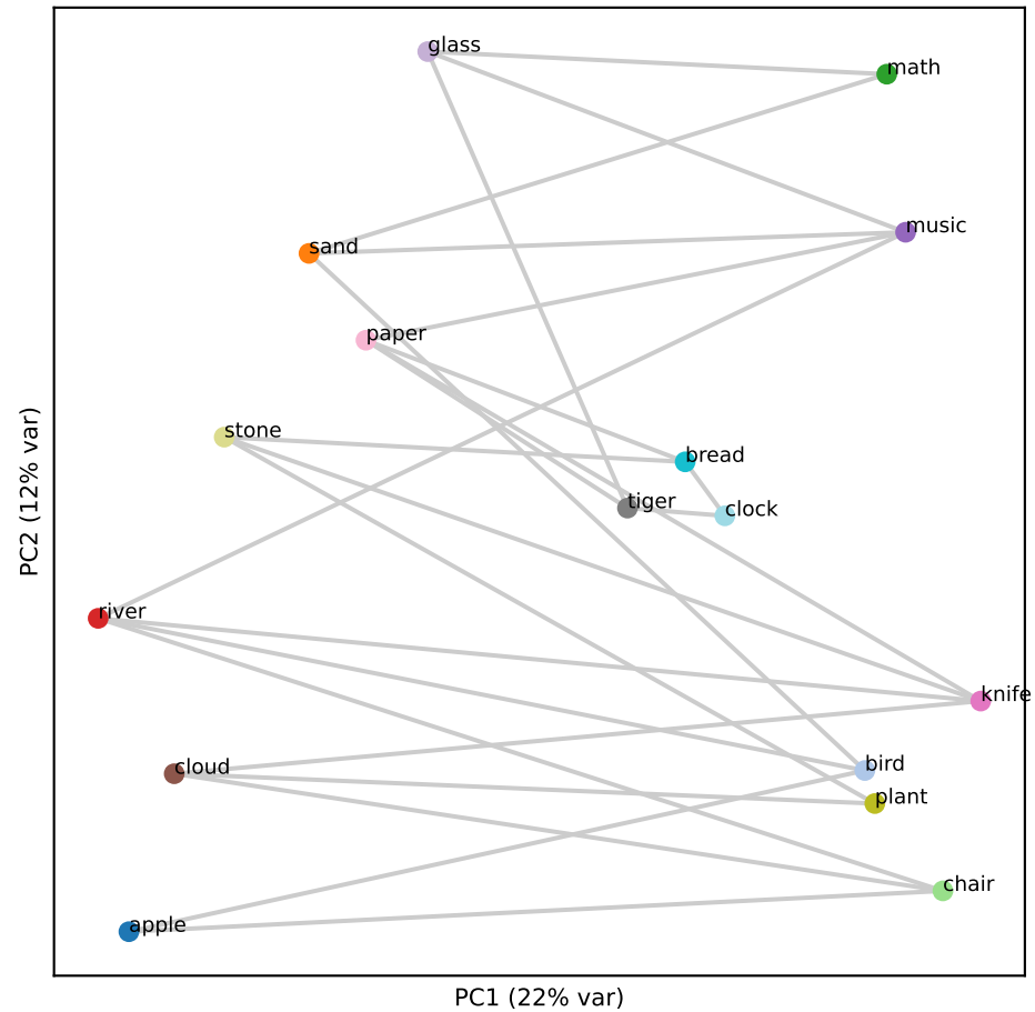
Llama L19 (RSA 0.11)
