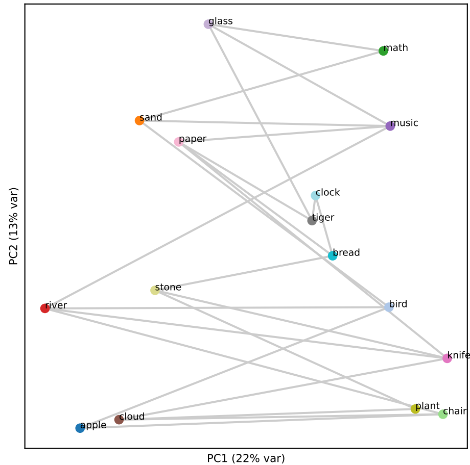
Llama L24 (RSA 0.16)
