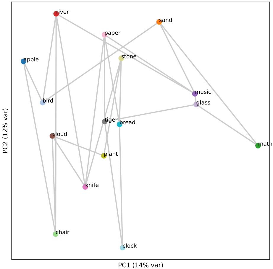
Llama L8 (RSA 0.29)
