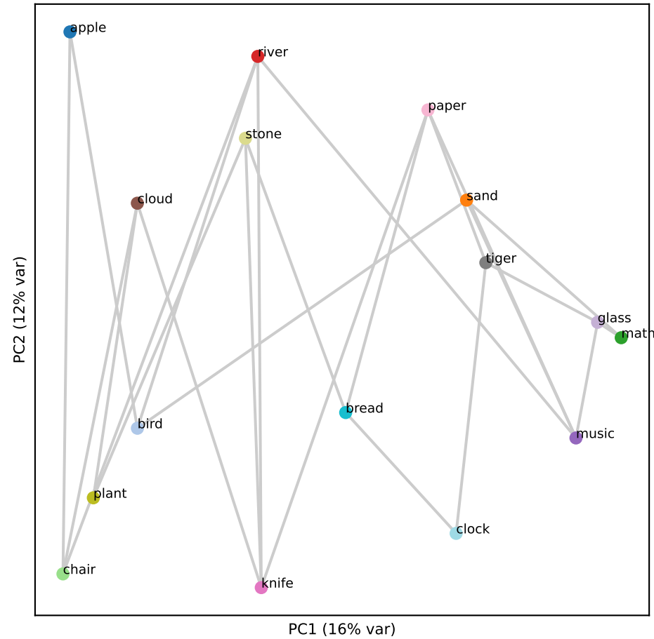
Gemma L24 (RSA 0.38)
