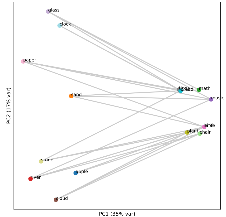
Qwen L34 (RSA 0.06)
