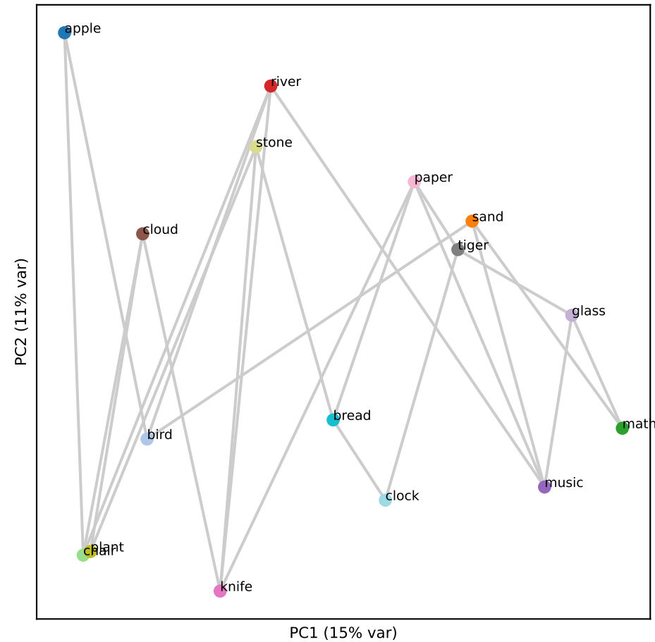
Gemma L27 (RSA 0.37)
