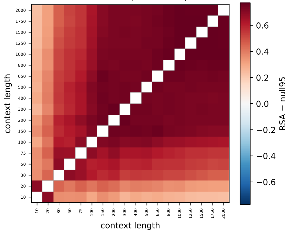
Gemma L14 (100% > null)
