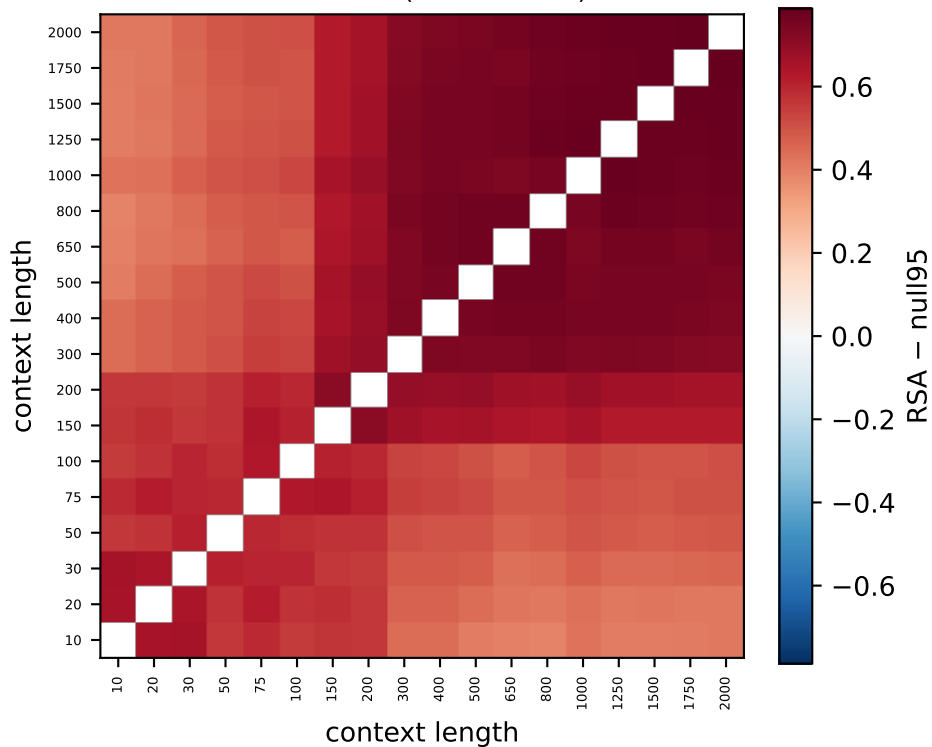
Llama L5 (100% > null)
