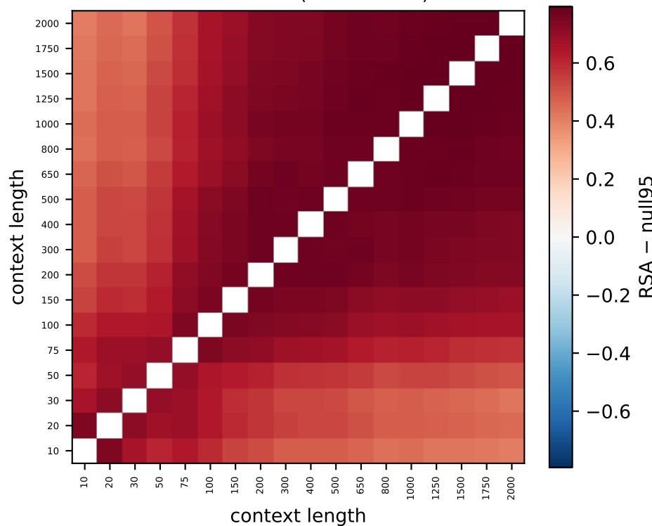
Gemma L13 (100% > null)
