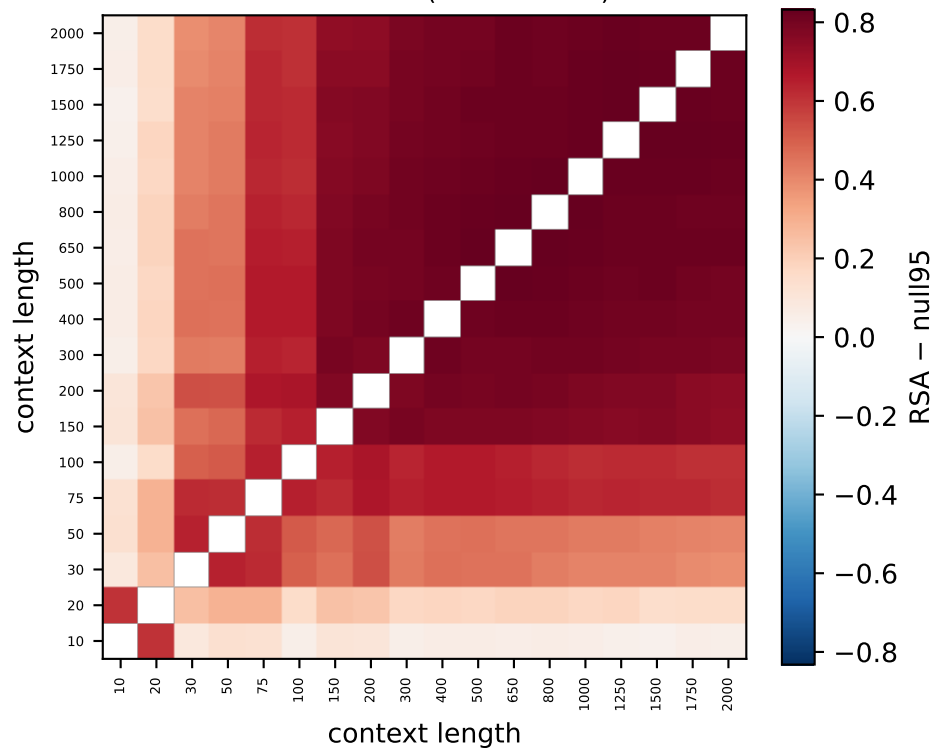
Gemma L20 (100% > null)
