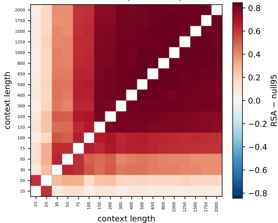
Gemma L21 (100% > null)
