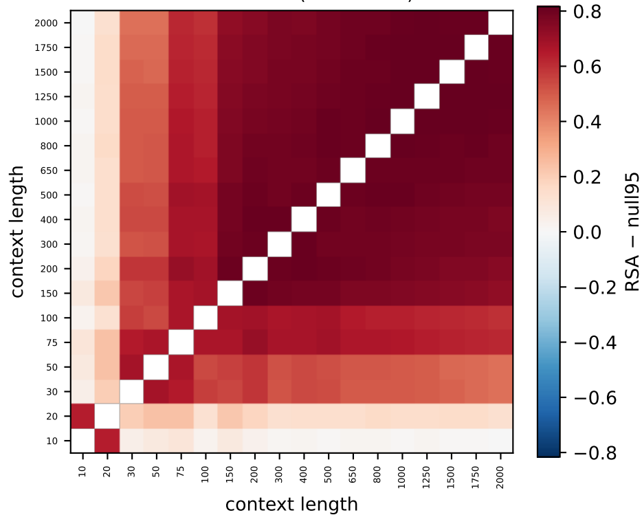
Gemma L19 (99% > null)
