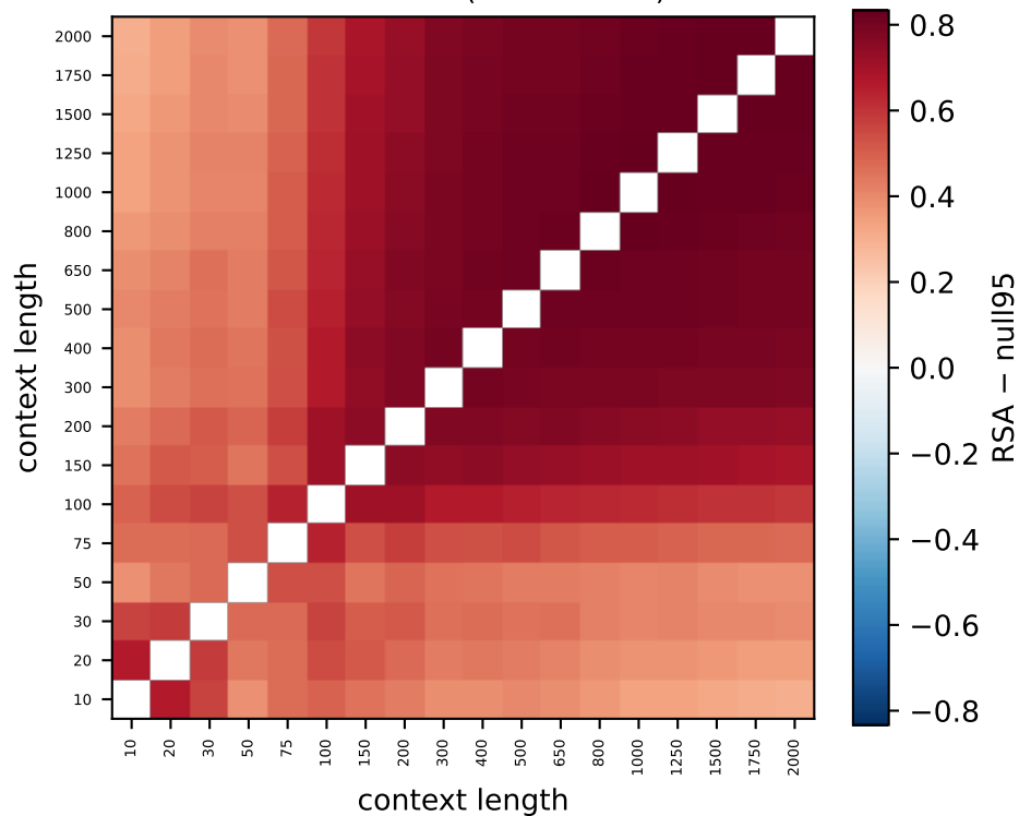
Gemma L35 (100% > null)
