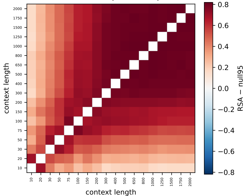
Gemma L25 (100% > null)
