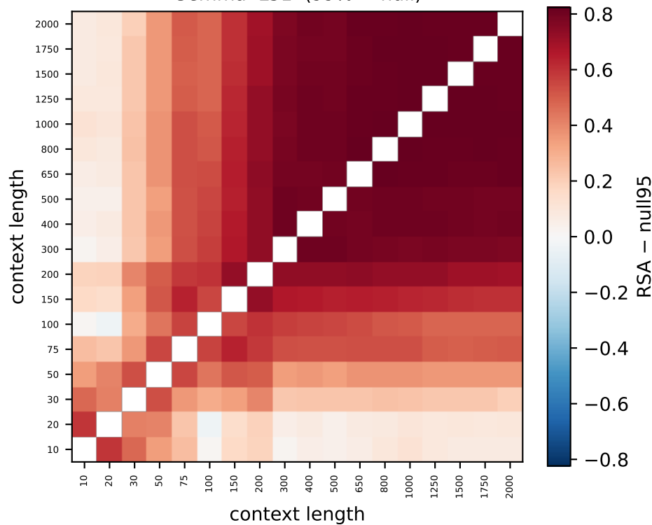
Gemma L31 (99% > null)
