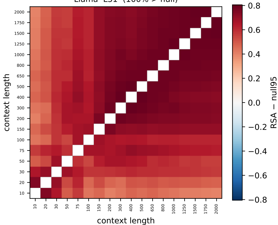
Llama L31 (100% > null)
