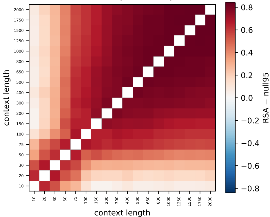
Llama L16 (100% > null)
