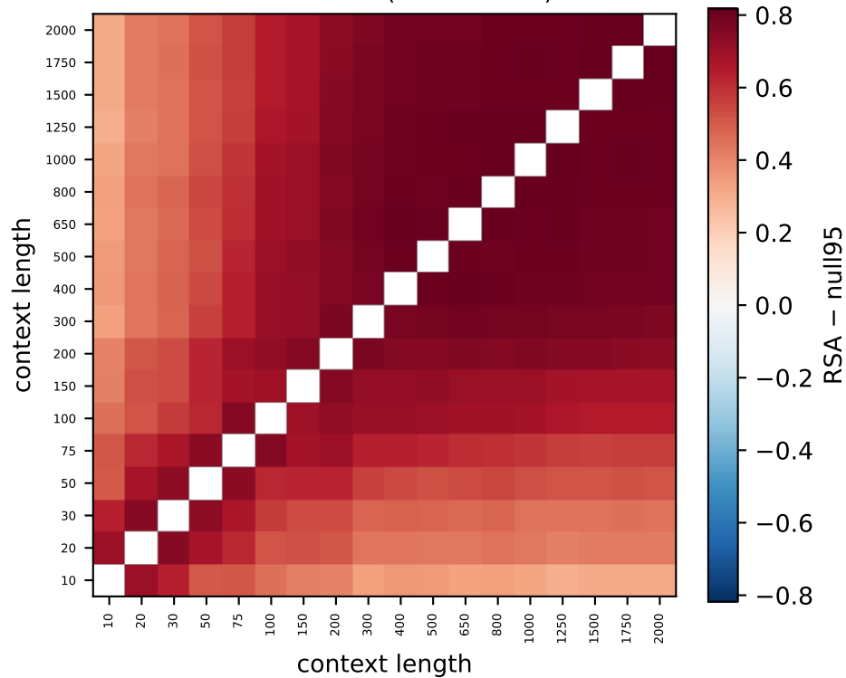
Gemma L26 (100% > null)
