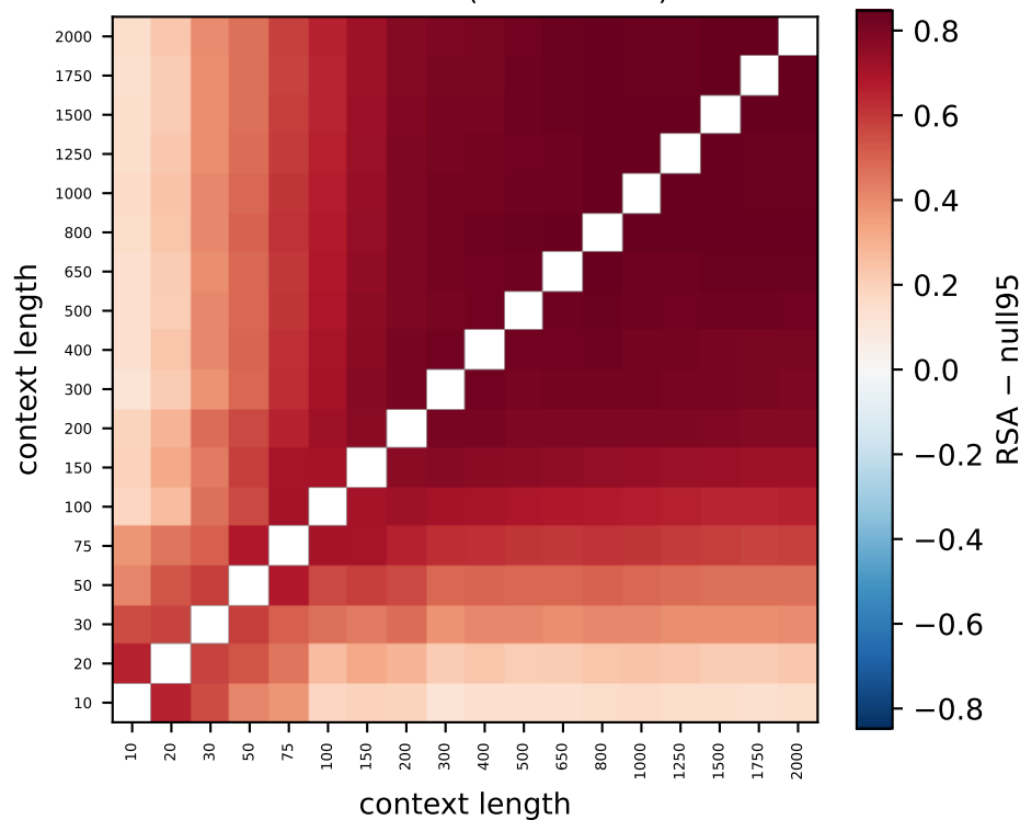
Gemma L29 (100% > null)
