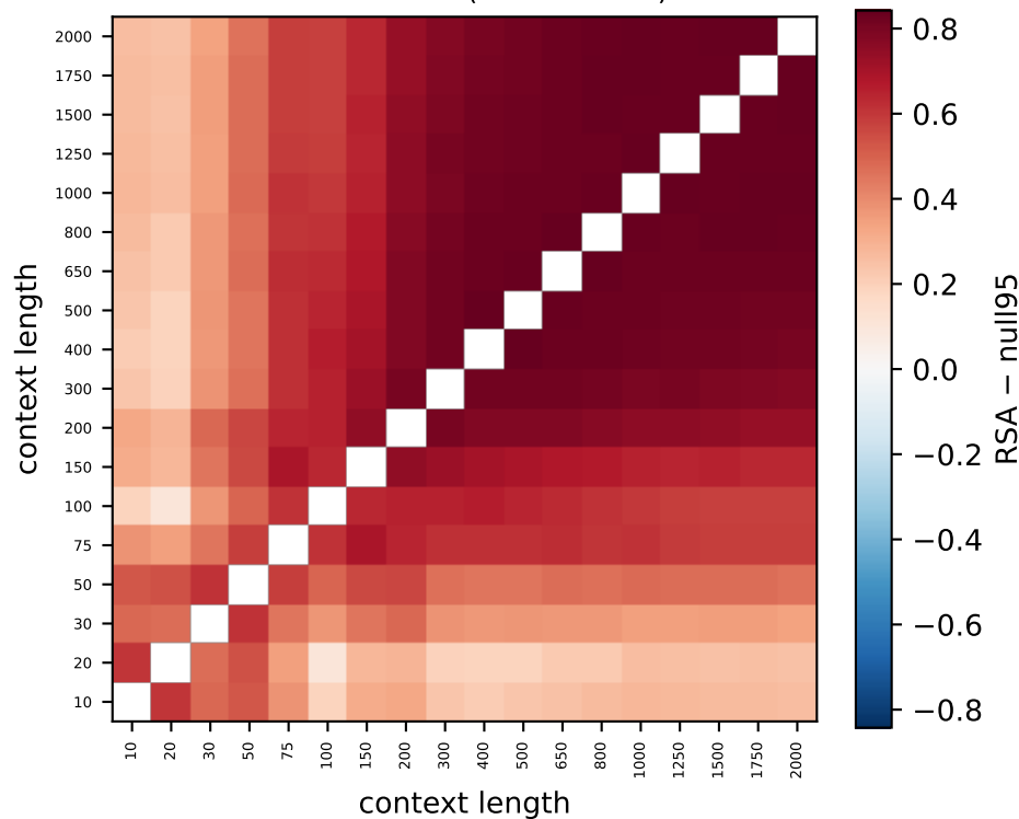
Gemma L33 (100% > null)
