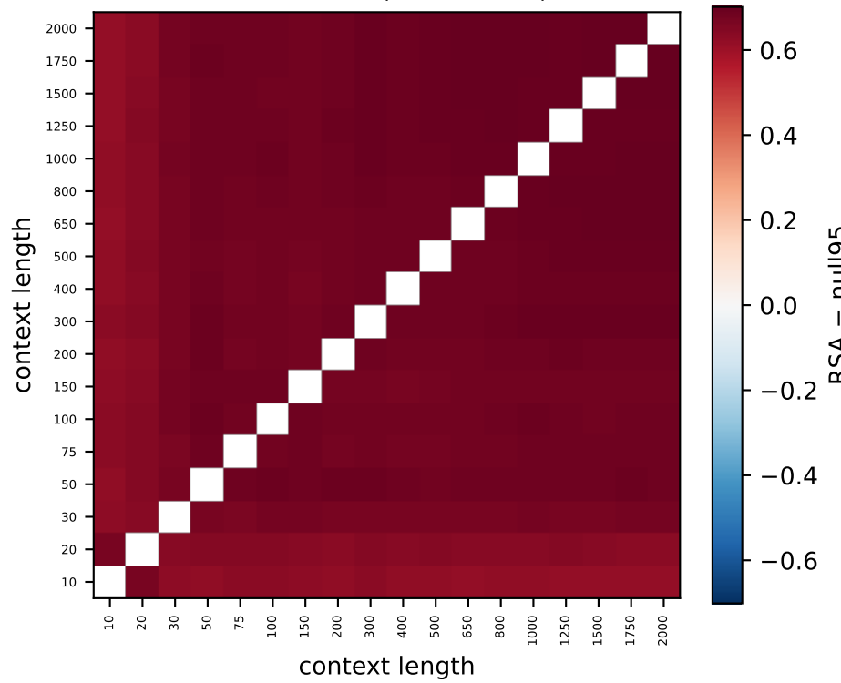
Gemma L0 (100% > null)
