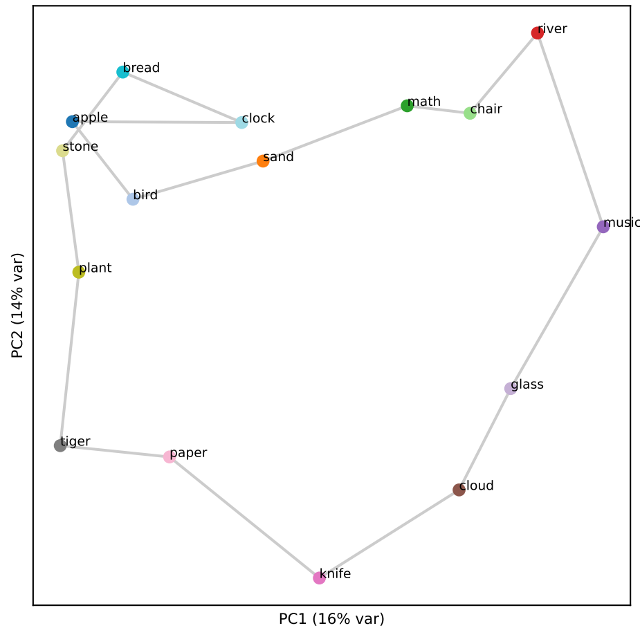
Gemma L26 (RSA 0.67)
