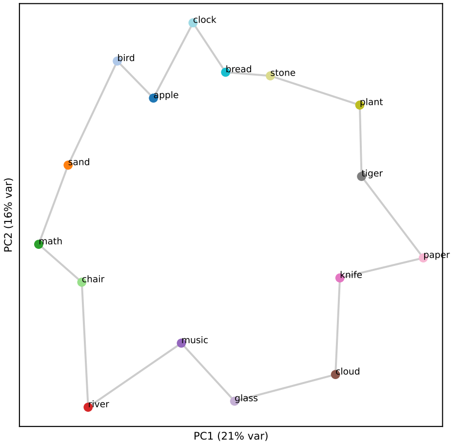
Llama L27 (RSA 0.88)
