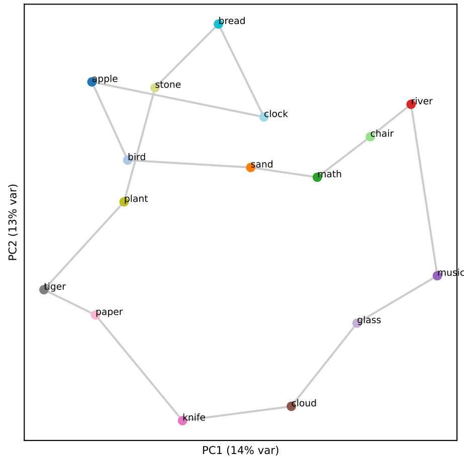
Gemma L19 (RSA 0.57)
