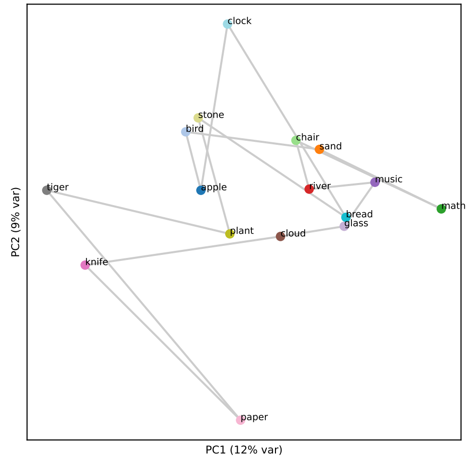
Qwen L25 (RSA 0.17)
