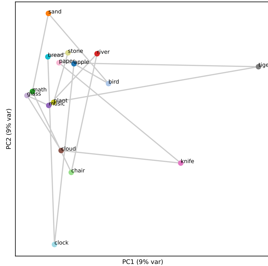
Gemma L2 (RSA -0.03)
