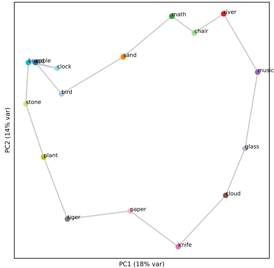
Gemma L27 (RSA 0.78)
