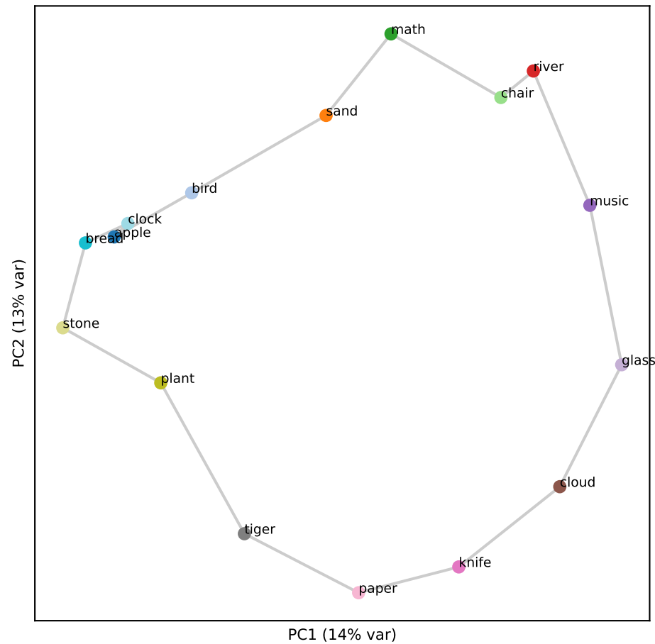
Gemma L33 (RSA 0.85)
