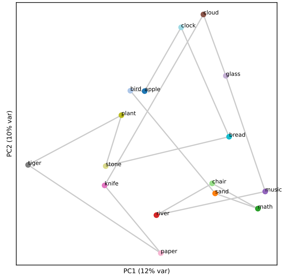
Qwen L17 (RSA 0.10)
