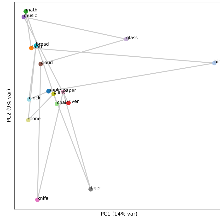
Qwen L8 (RSA 0.00)
