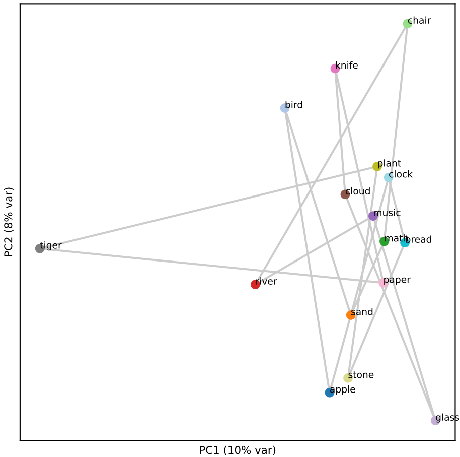
Llama L0 (RSA -0.11)
