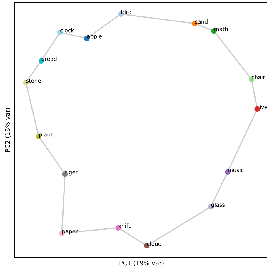
Gemma L38 (RSA 0.93)
