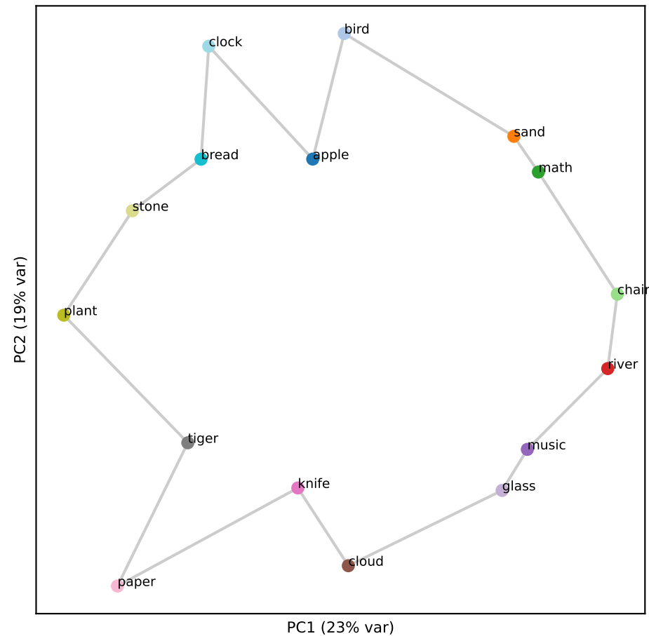
Gemma L41 (RSA 0.88)
