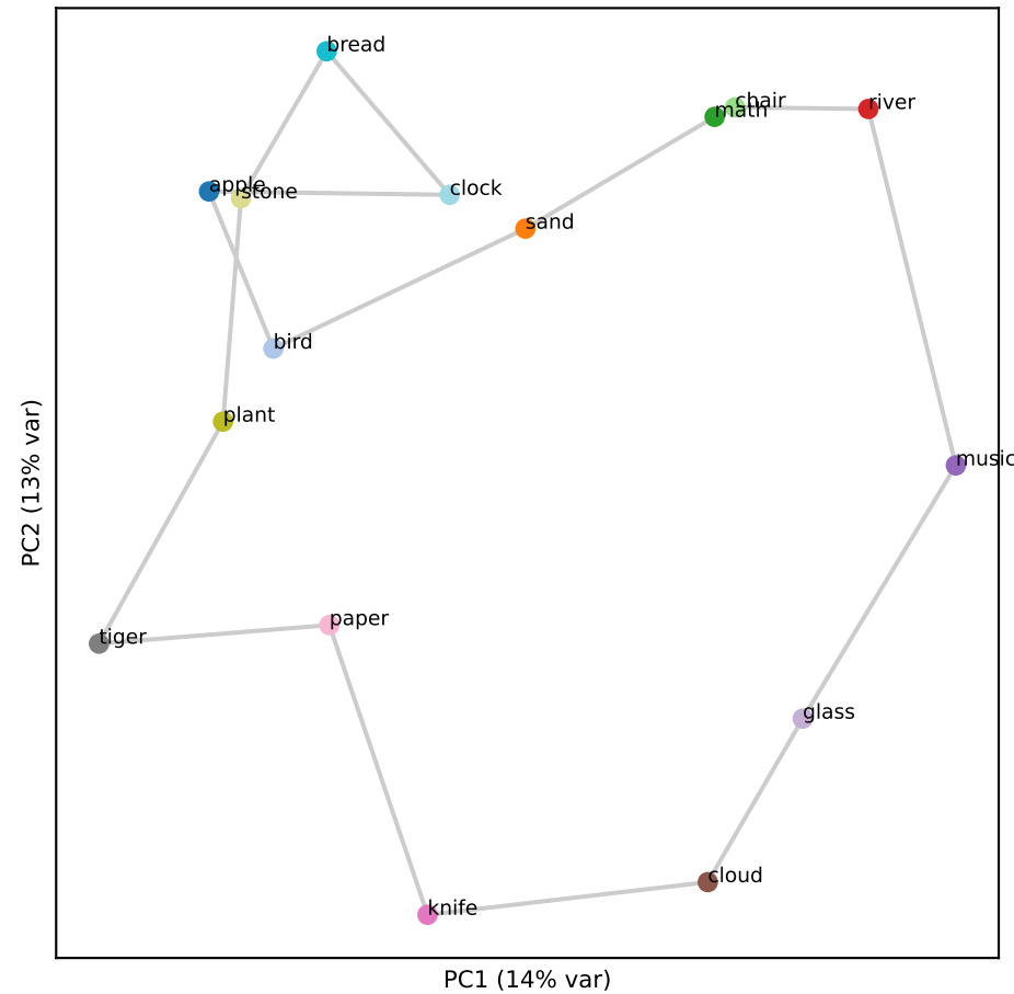
Gemma L16 (RSA 0.62)
