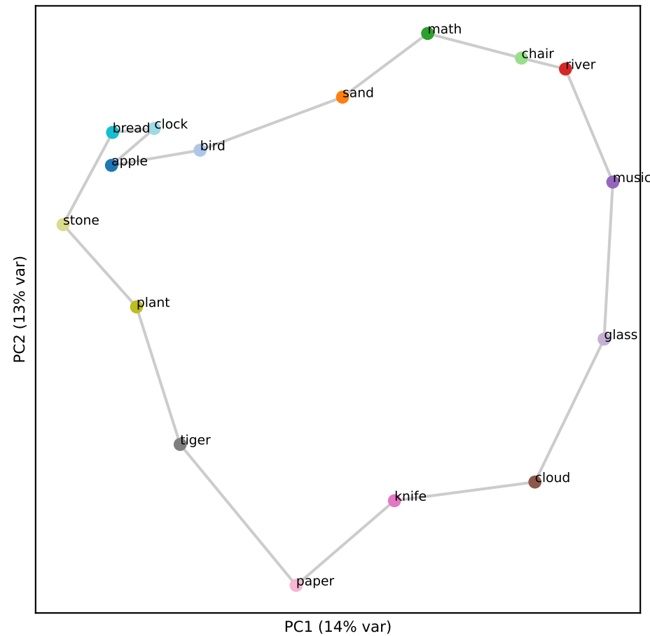
Gemma L32 (RSA 0.80)
