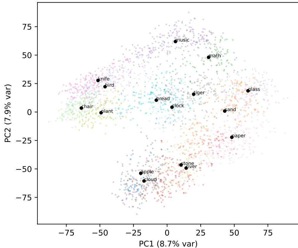
Gemma L28
