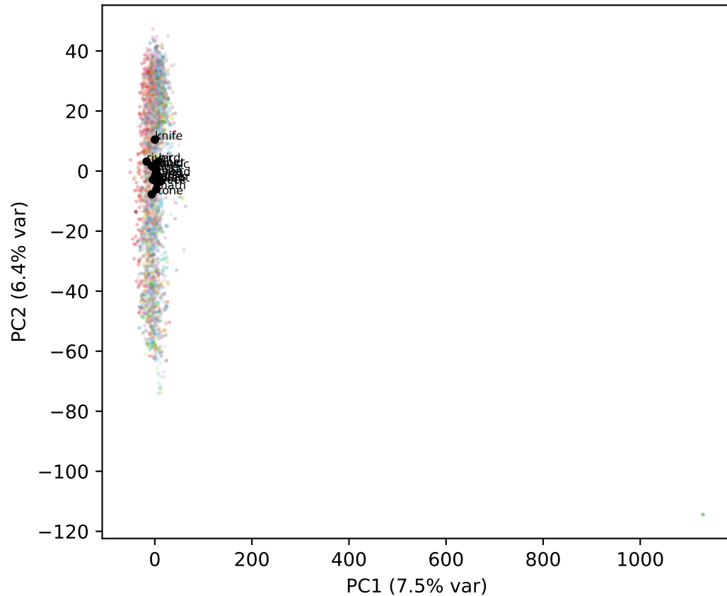
Gemma L16
