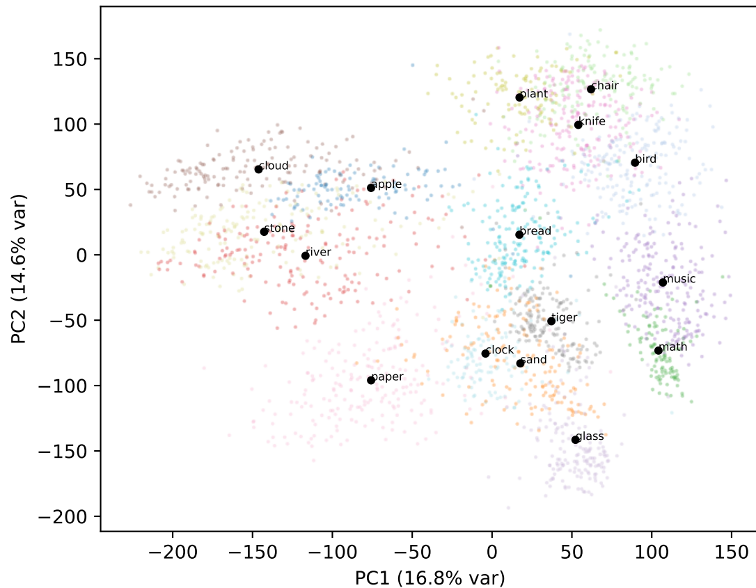
Gemma L40
