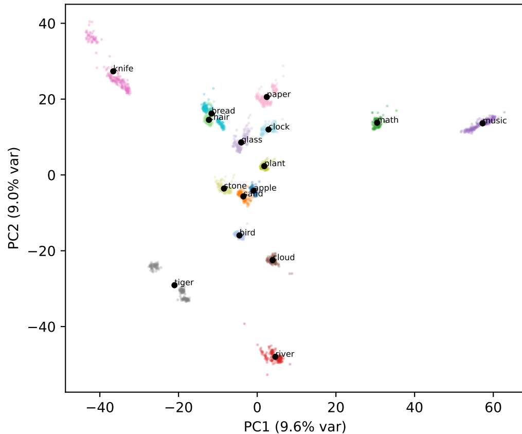
Gemma L5
