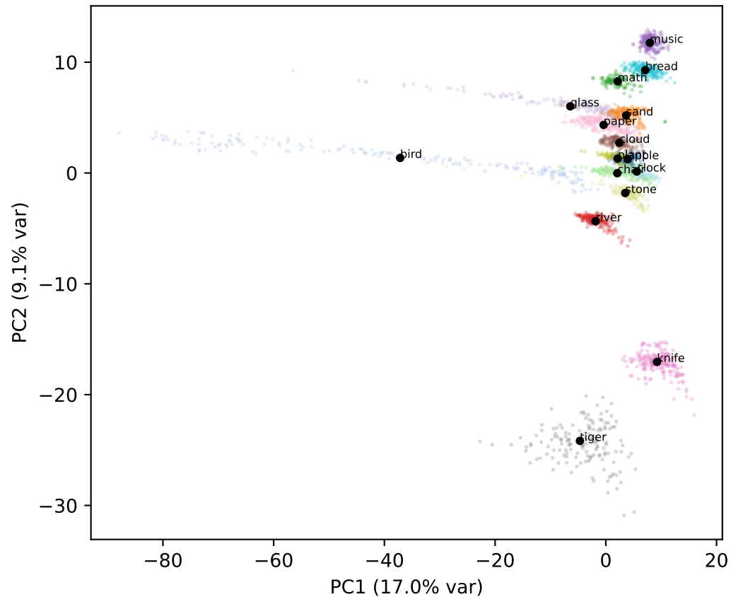
Qwen L5
