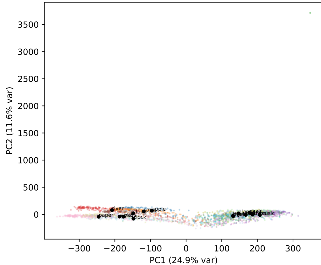
Qwen L34
