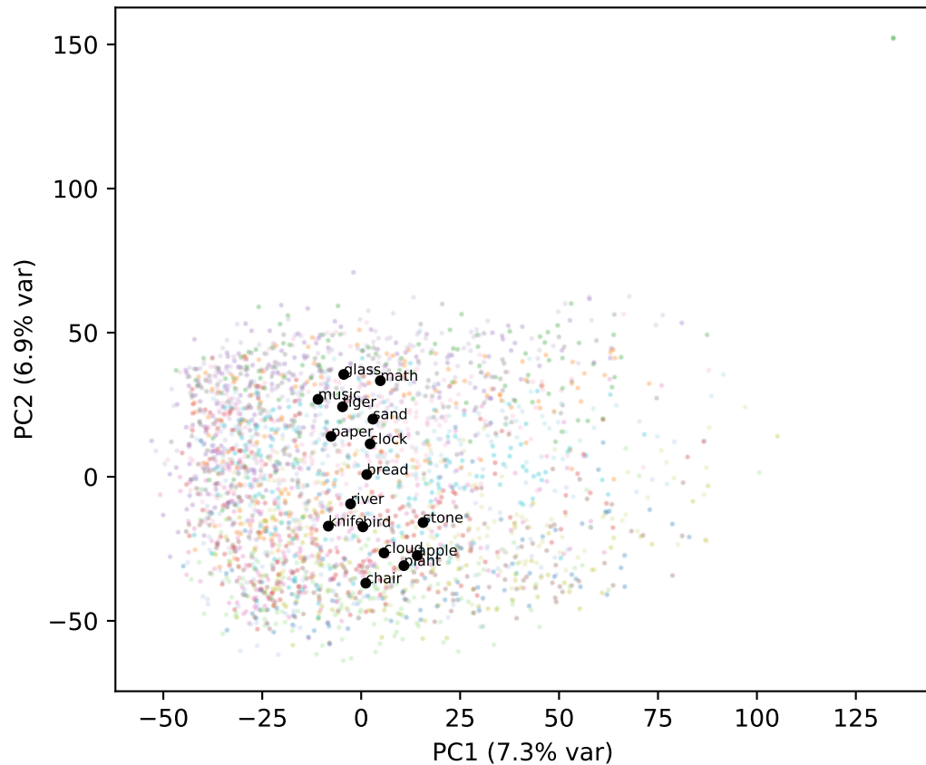
Gemma L23
