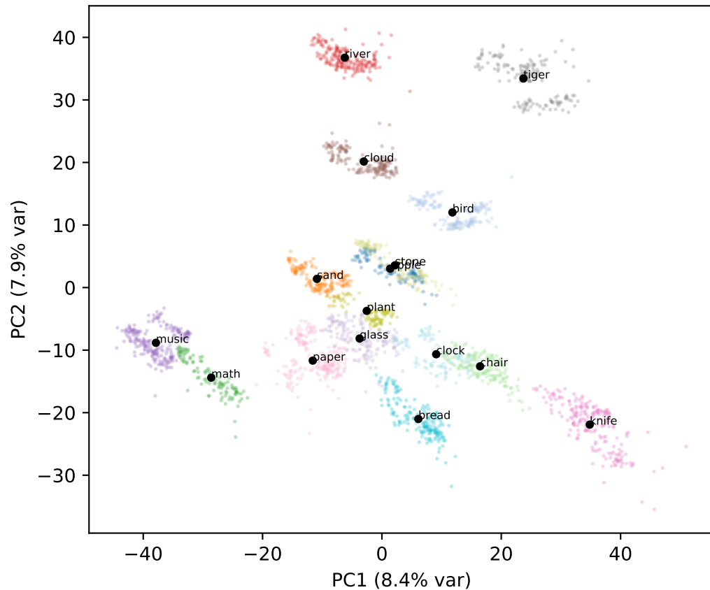
Gemma L8
