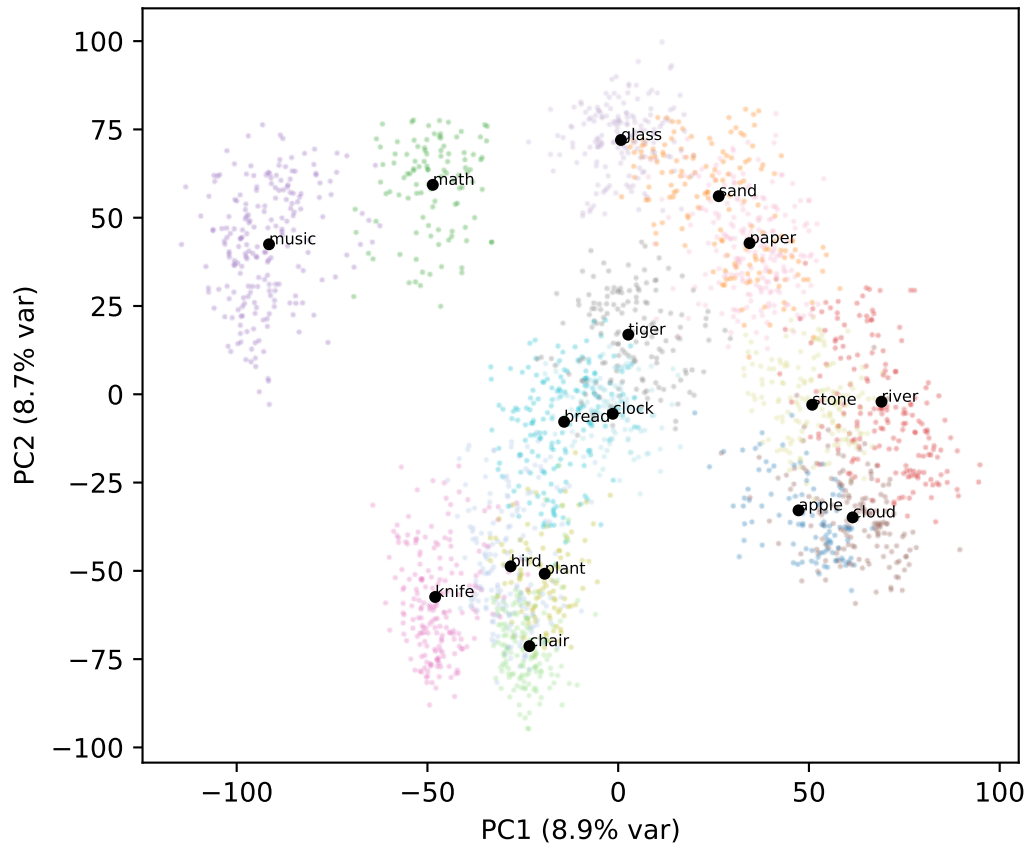
Gemma L30
