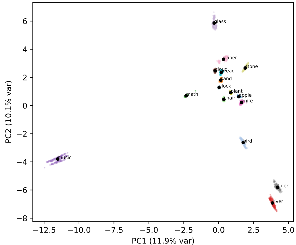
Qwen L0
