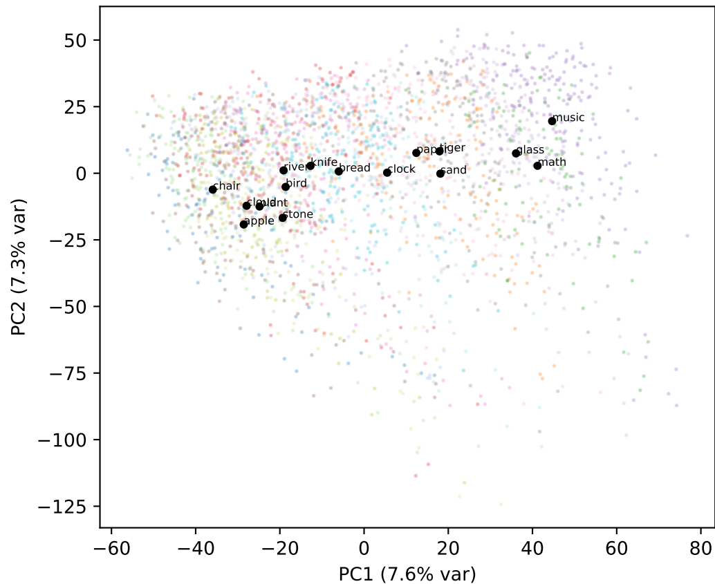
Gemma L26
