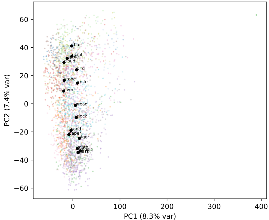
Gemma L25
