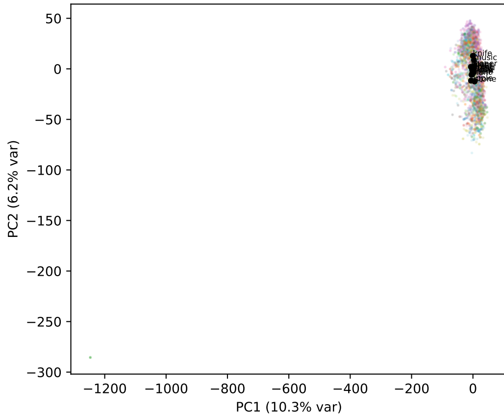
Gemma L19
