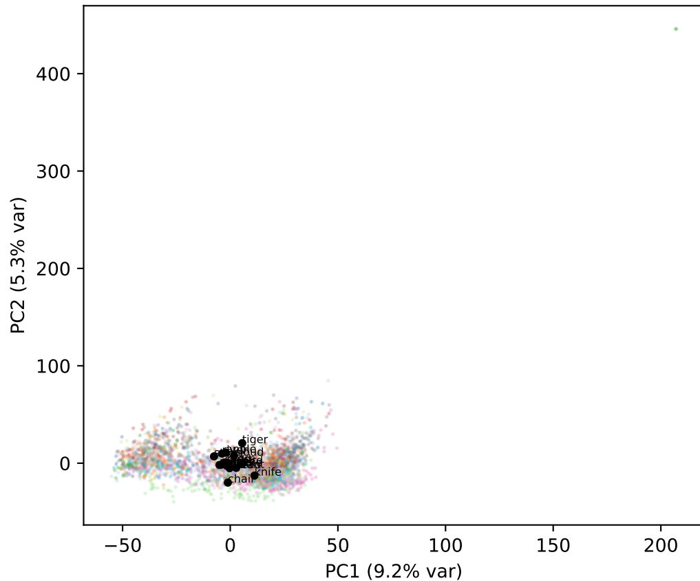
Gemma L14
