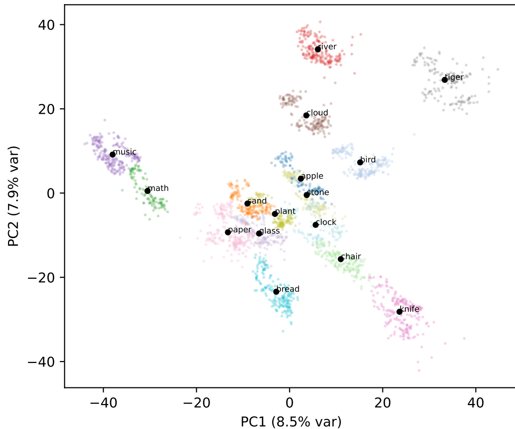
Gemma L9
