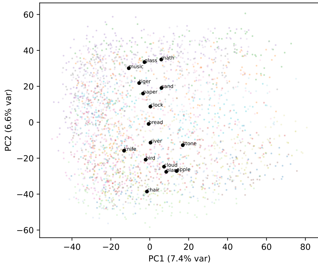
Gemma L24
