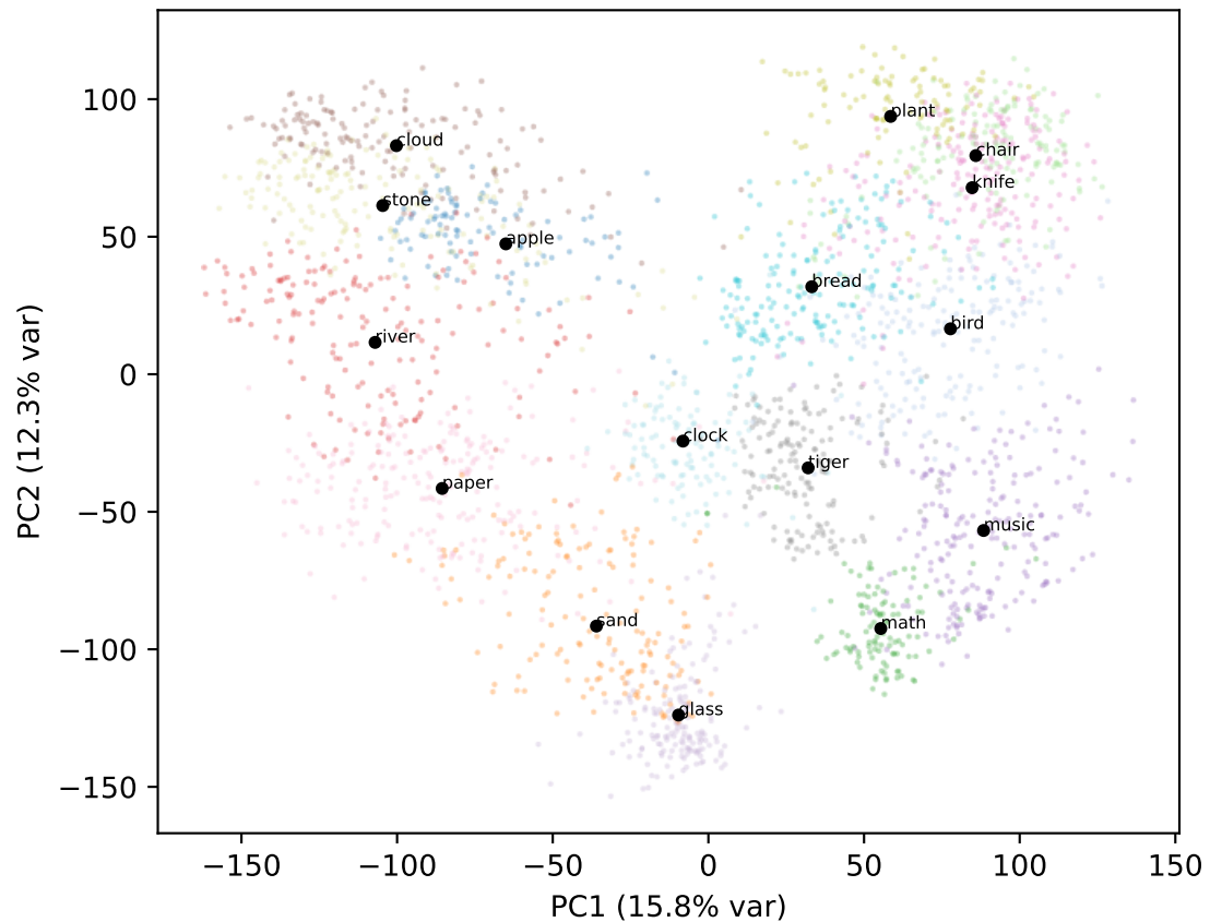
Gemma L38
