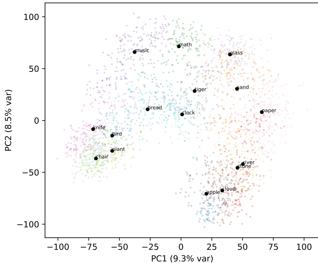
Gemma L31
