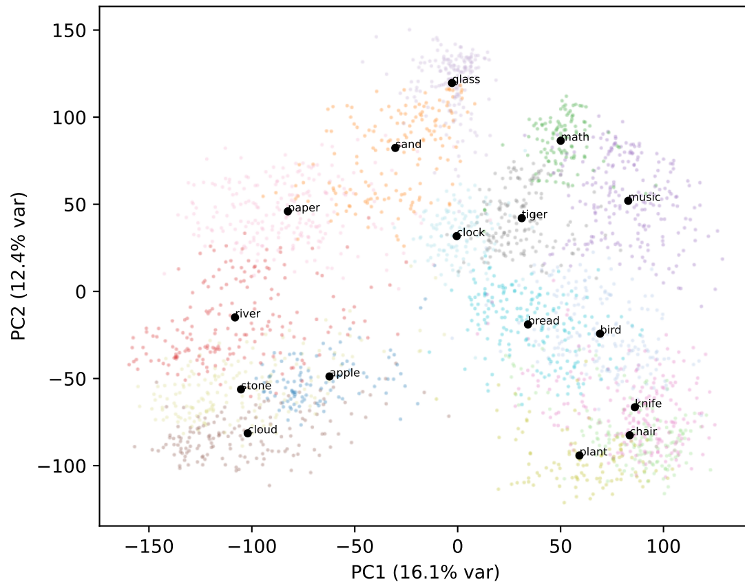
Gemma L37
