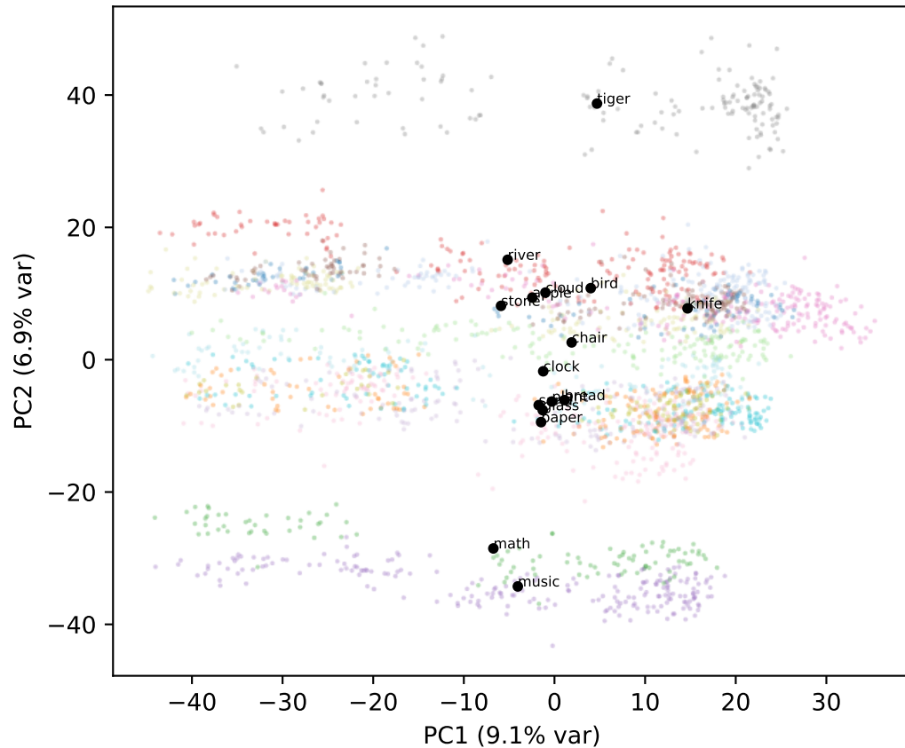
Gemma L11
