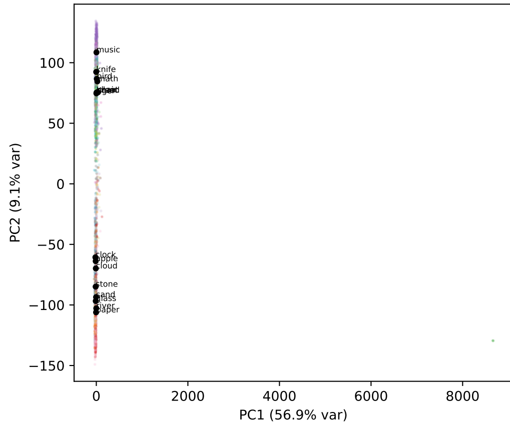
Qwen L30
