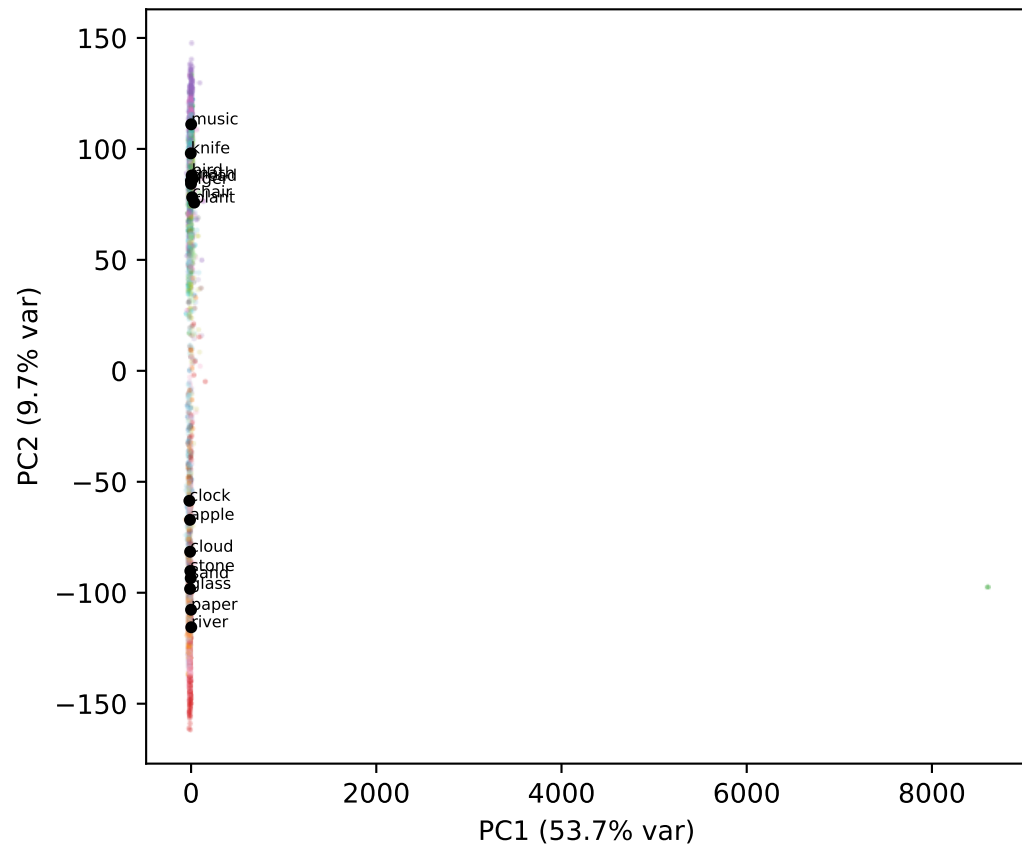
Qwen L31
