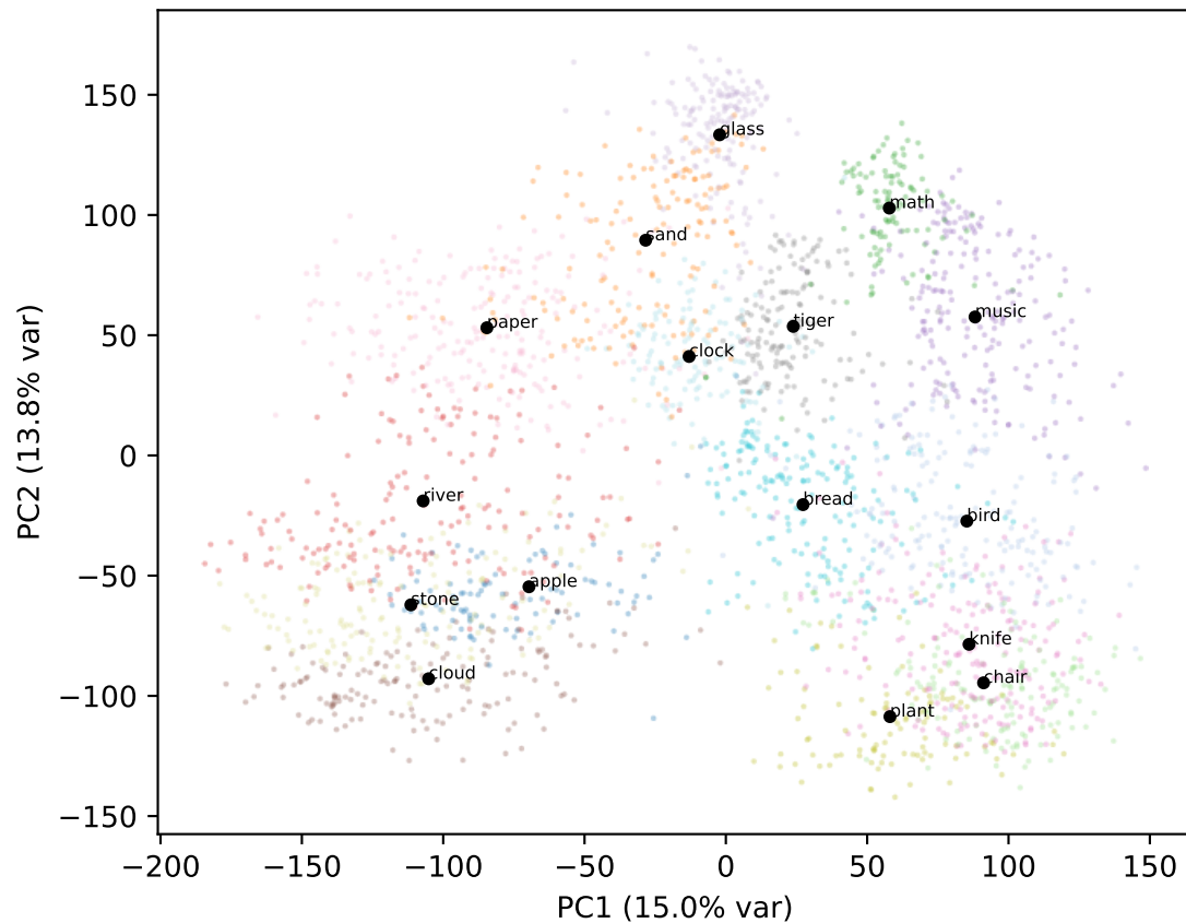
Gemma L39
