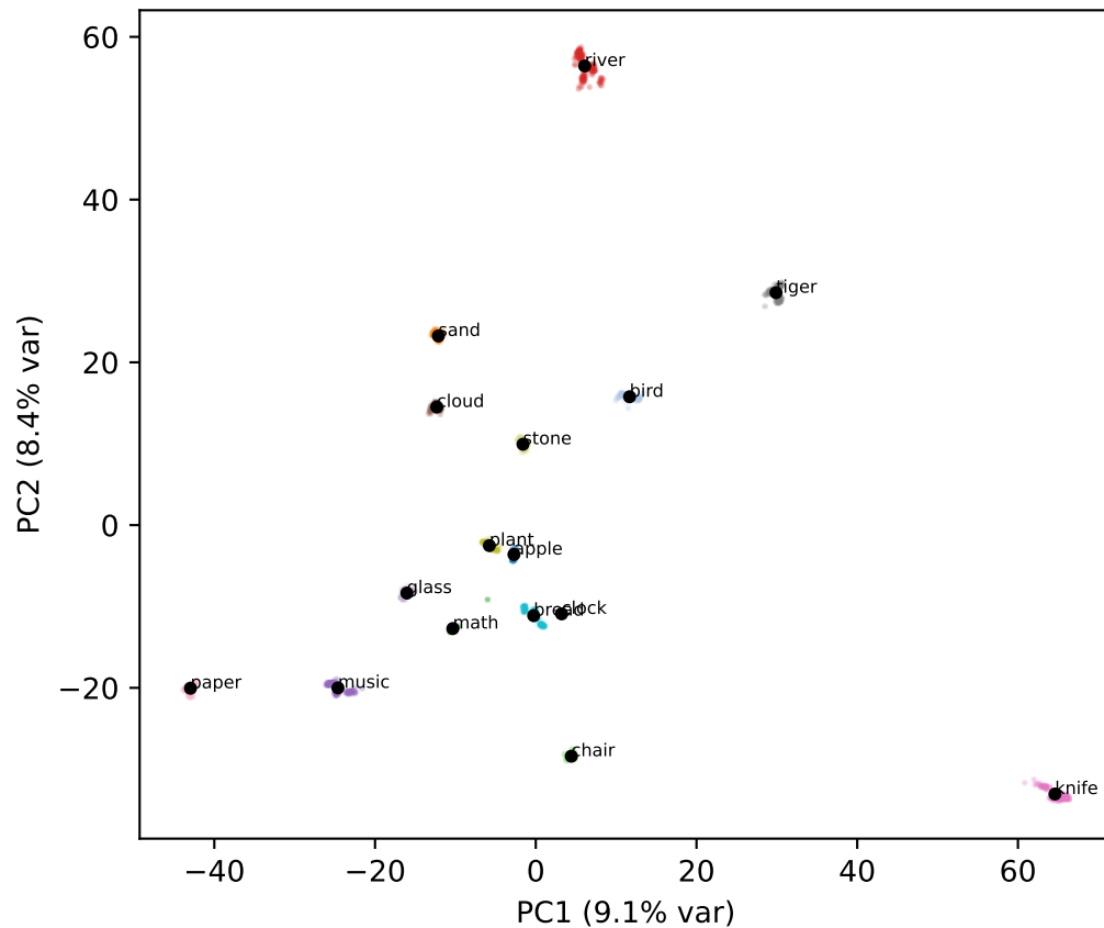
Gemma L1
