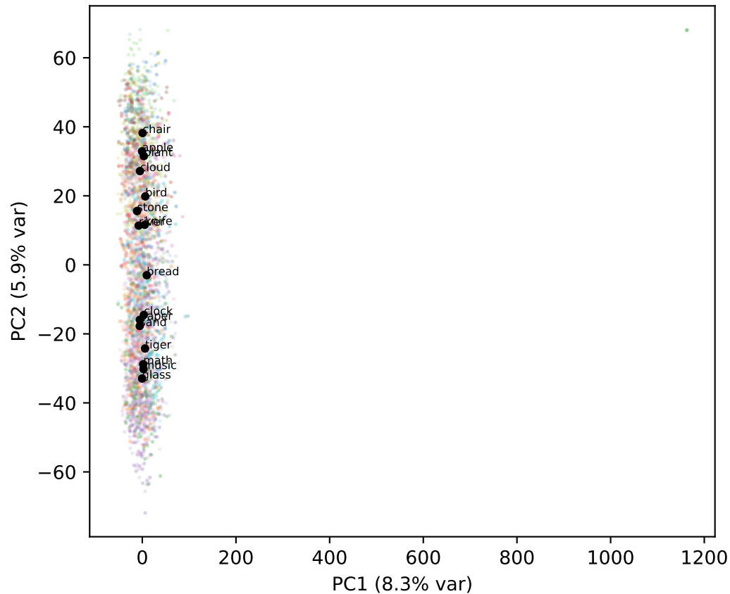
Gemma L20
