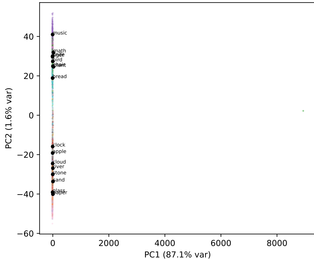
Qwen L23
