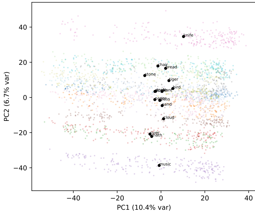
Gemma L12
