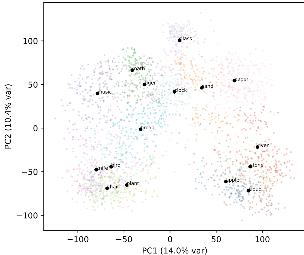
Gemma L35
