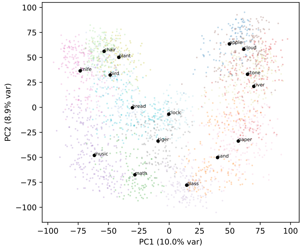
Gemma L32
