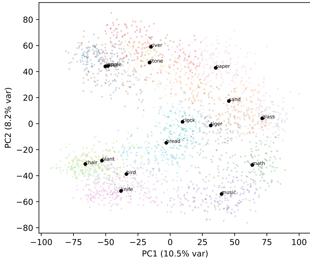
Gemma L29
