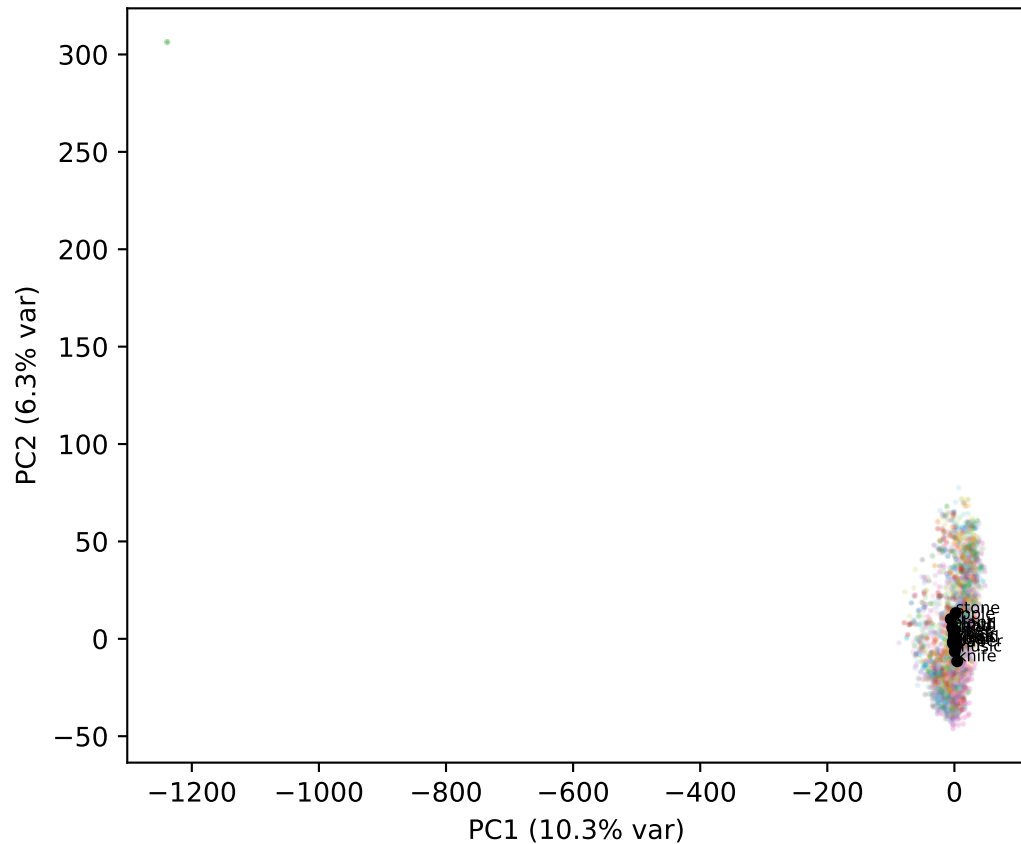
Gemma L18
