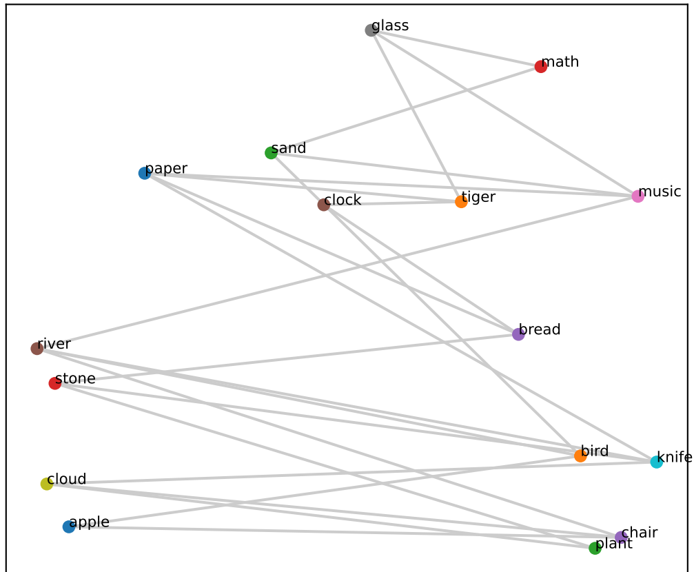
Gemma L34 (grid RSA=0.49, PCA corr=0.22)
