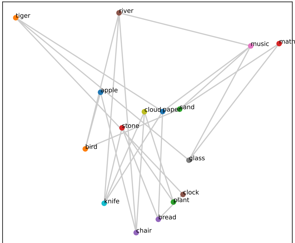
Gemma L12 (grid RSA=0.10, PCA corr=0.04)
