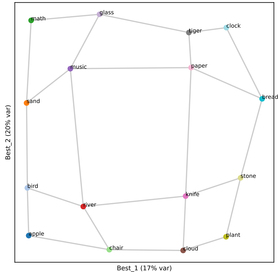
Gemma L40 (RSA 0.89)
