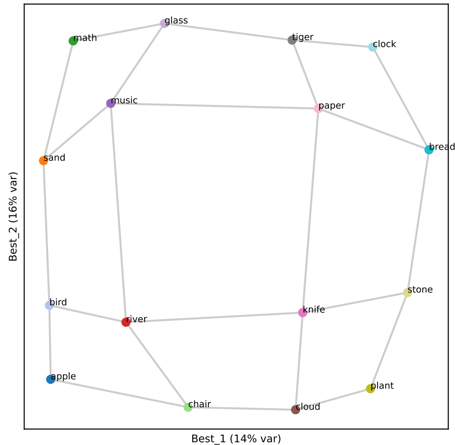
Gemma L38 (RSA 0.88)
