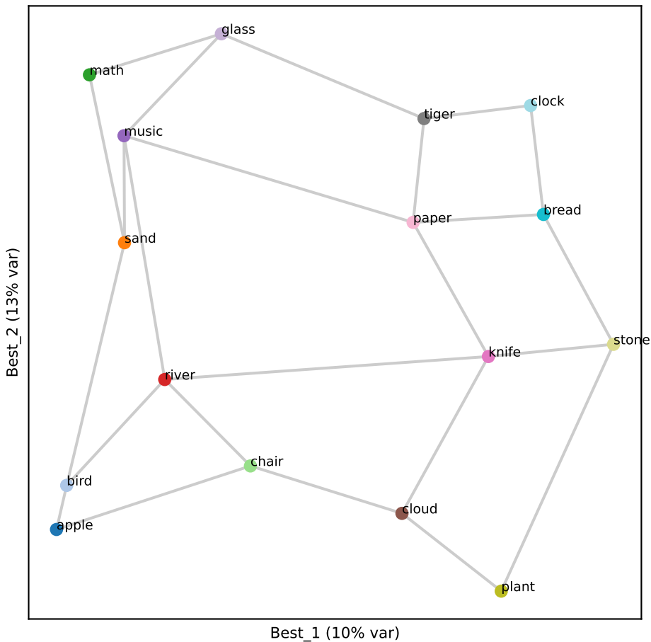
Llama L12 (RSA 0.81)
