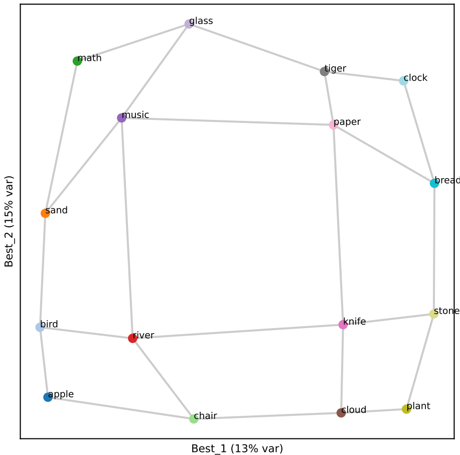
Llama L27 (RSA 0.87)
