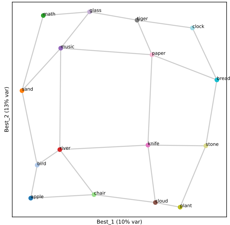
Gemma L34 (RSA 0.87)
