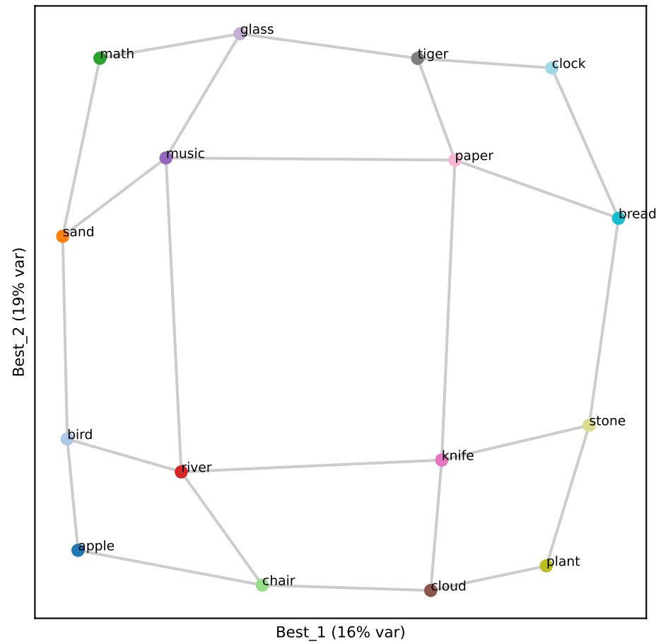
Gemma L39 (RSA 0.88)
