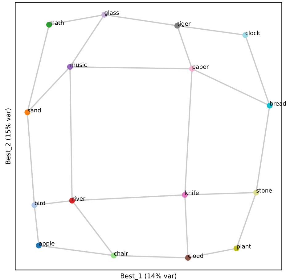
Gemma L36 (RSA 0.89)
