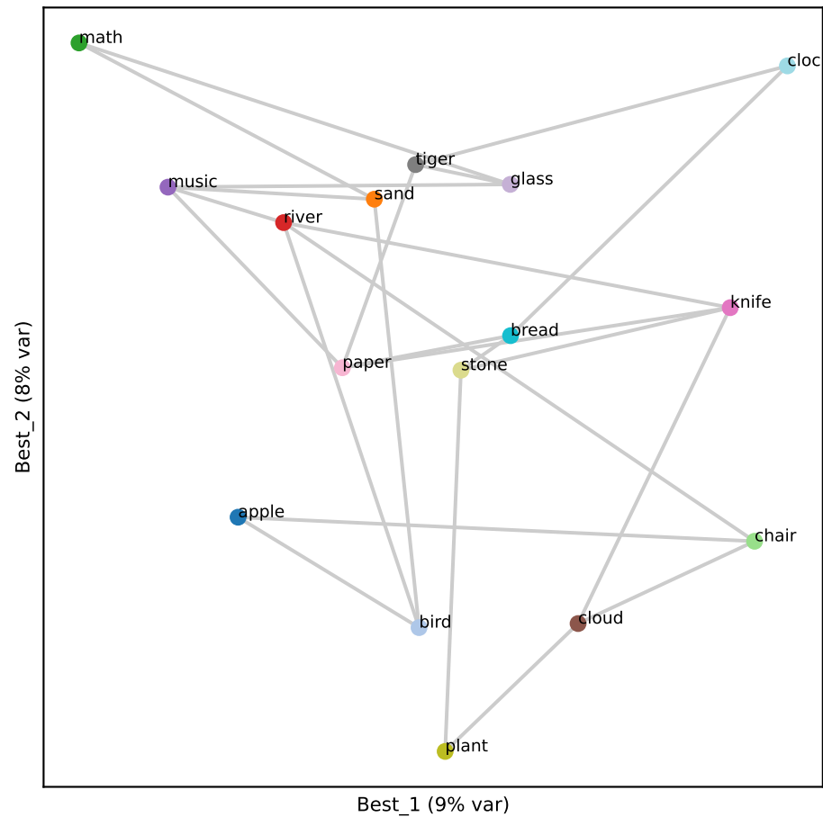
Gemma L4 (RSA 0.40)
