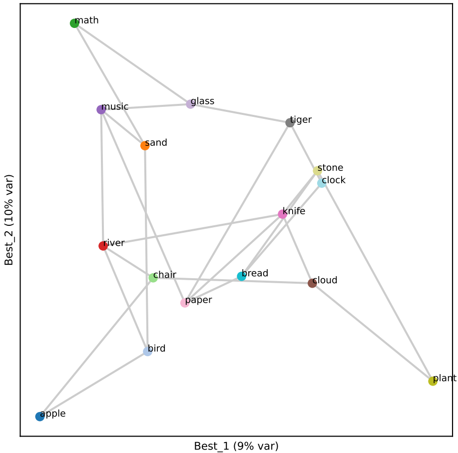
Llama L4 (RSA 0.46)
