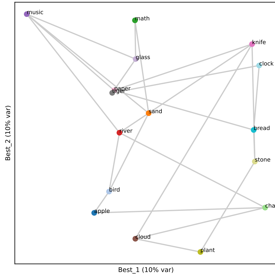
Gemma L13 (RSA 0.36)
