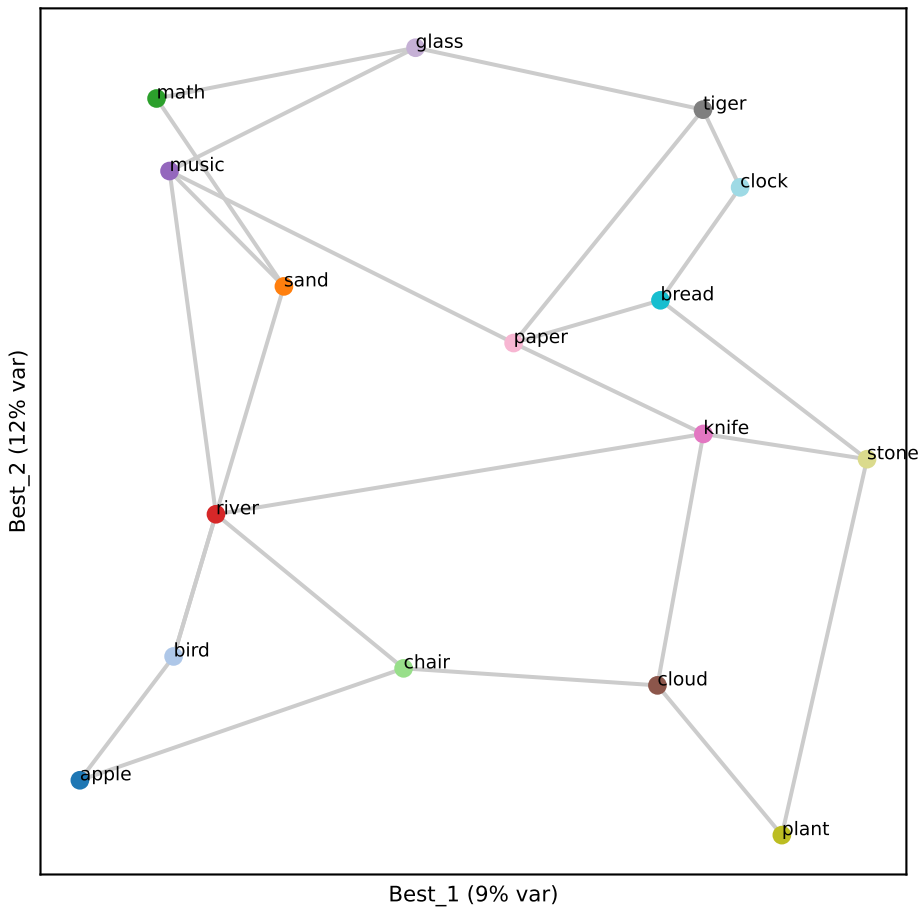
Llama L14 (RSA 0.73)
