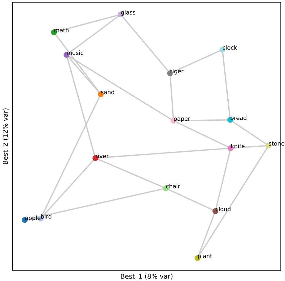
Llama L11 (RSA 0.66)
