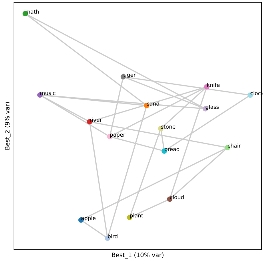
Gemma L9 (RSA 0.24)
