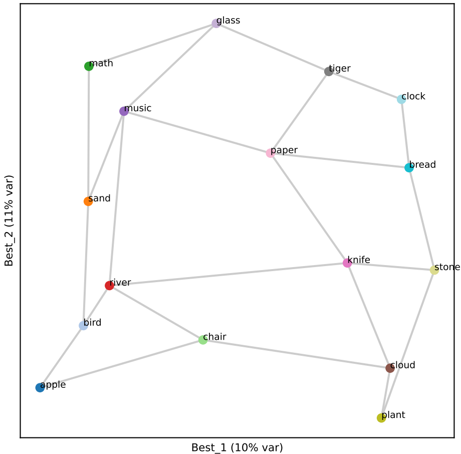
Llama L19 (RSA 0.80)
