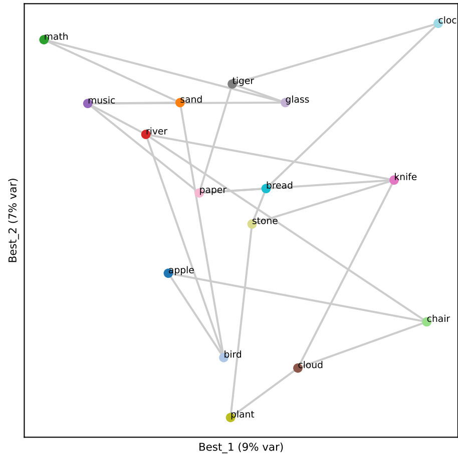
Gemma L3 (RSA 0.42)
