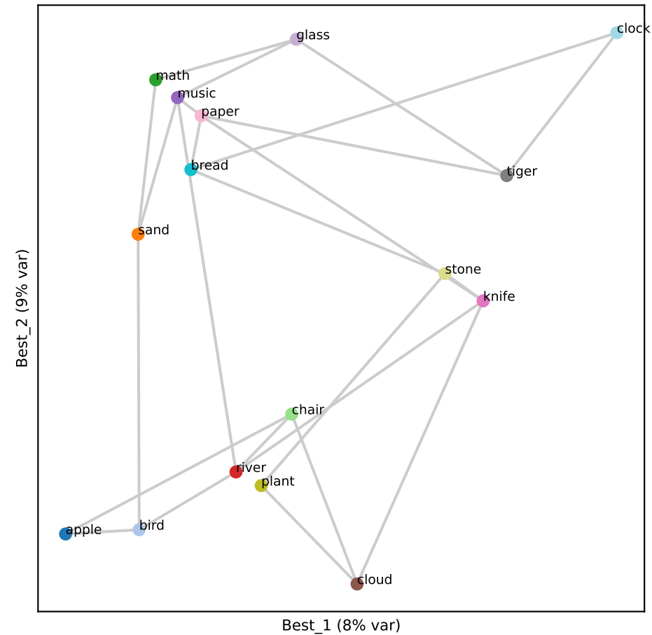
Qwen L22 (RSA 0.49)
