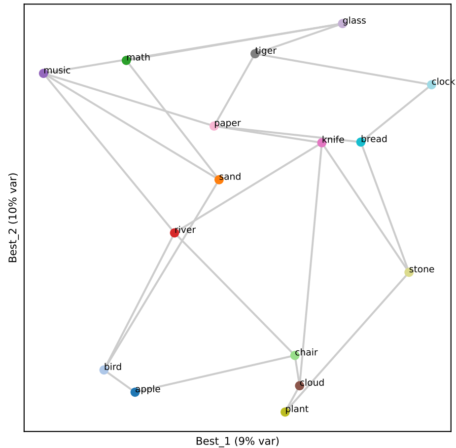
Gemma L15 (RSA 0.53)
