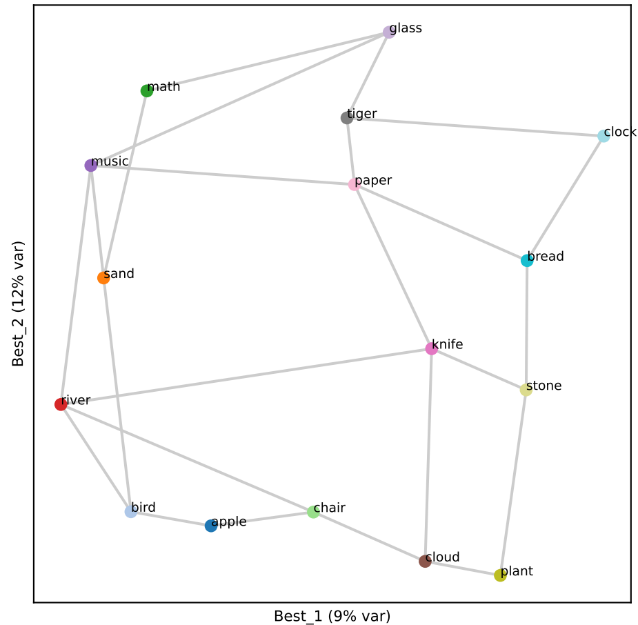
Gemma L30 (RSA 0.73)
