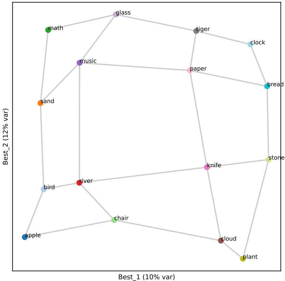
Llama L23 (RSA 0.86)
