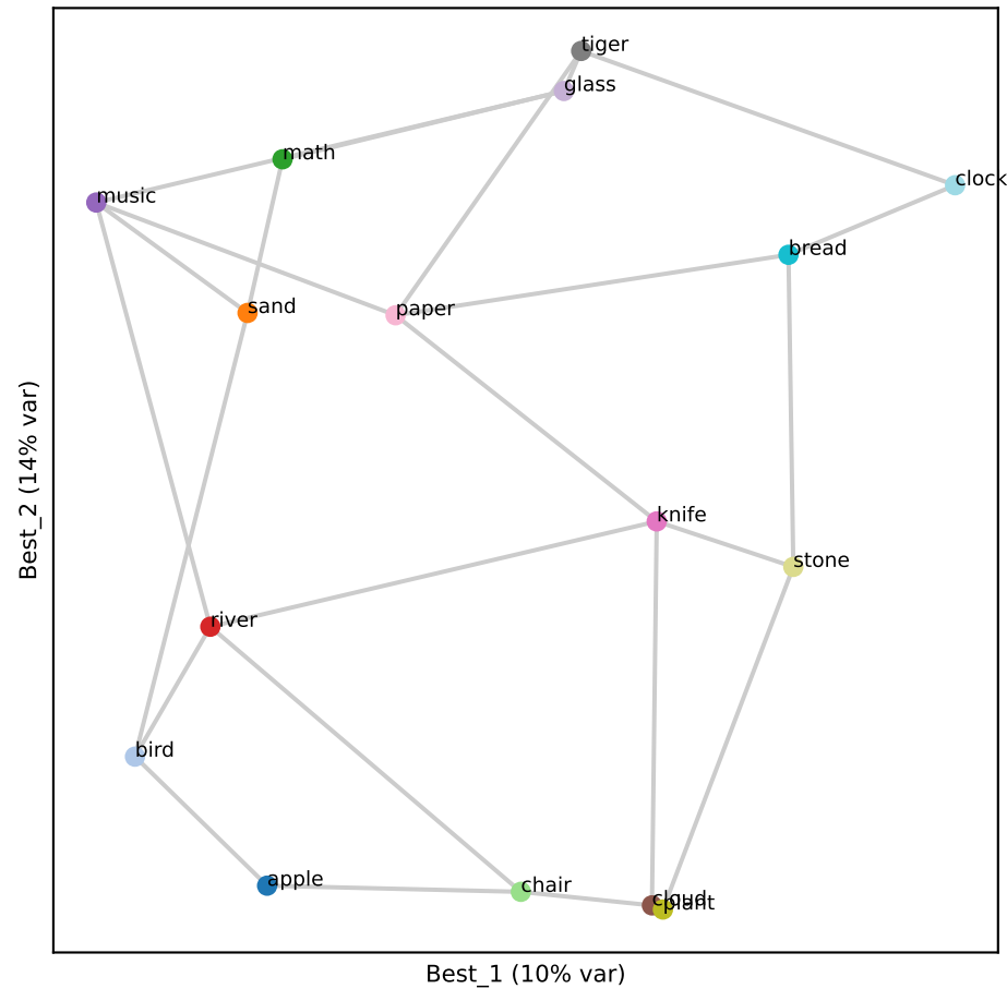
Gemma L20 (RSA 0.71)
