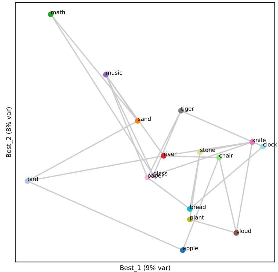
Qwen L8 (RSA 0.17)
