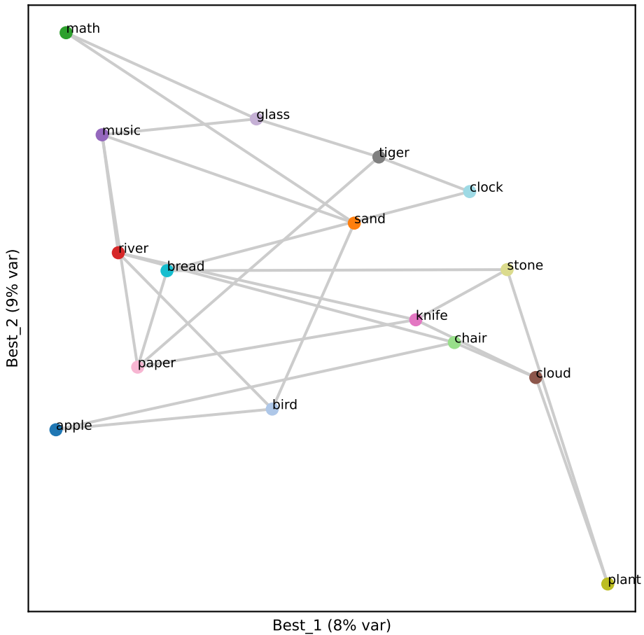
Llama L5 (RSA 0.33)
