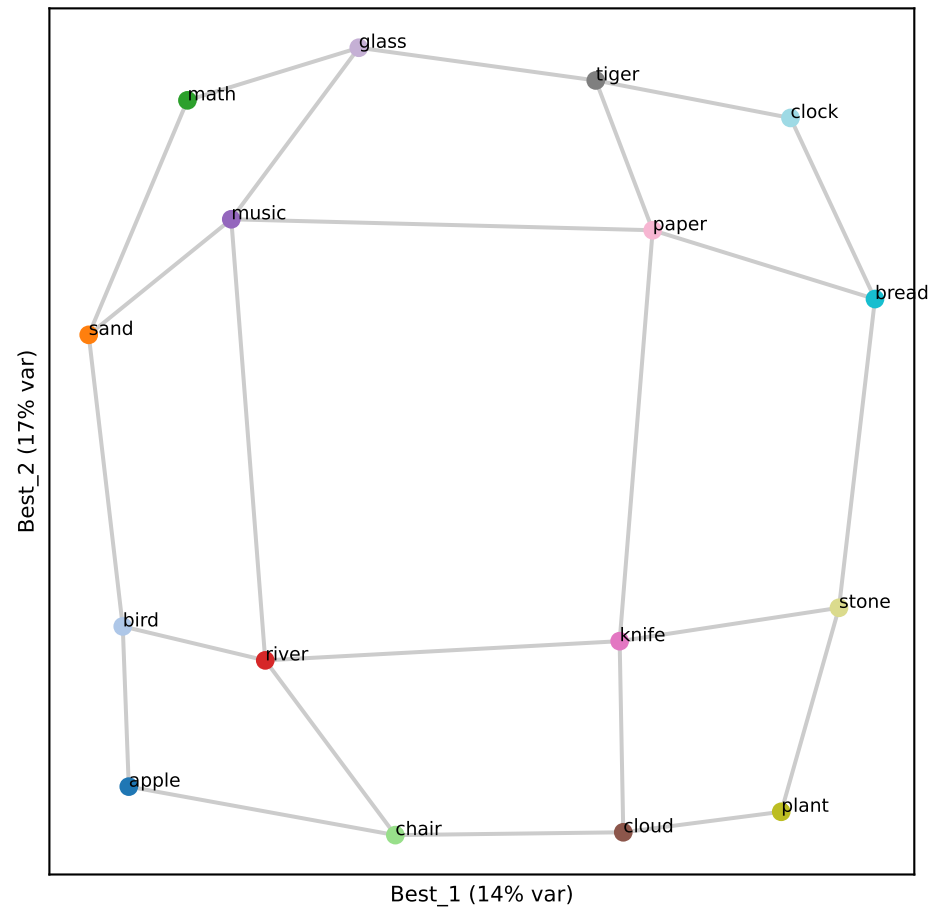
Gemma L37 (RSA 0.88)
