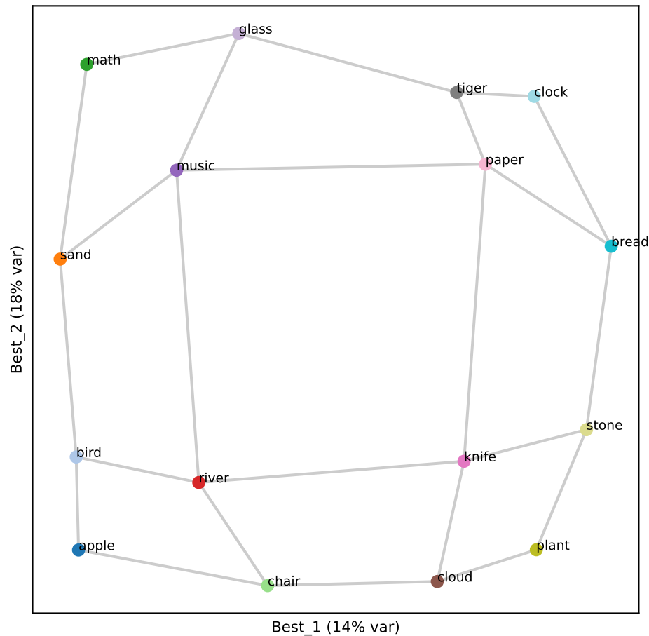
Llama L30 (RSA 0.88)
