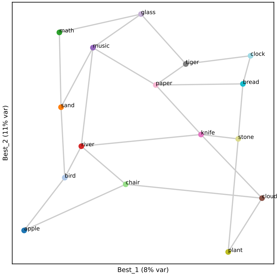
Llama L20 (RSA 0.73)
