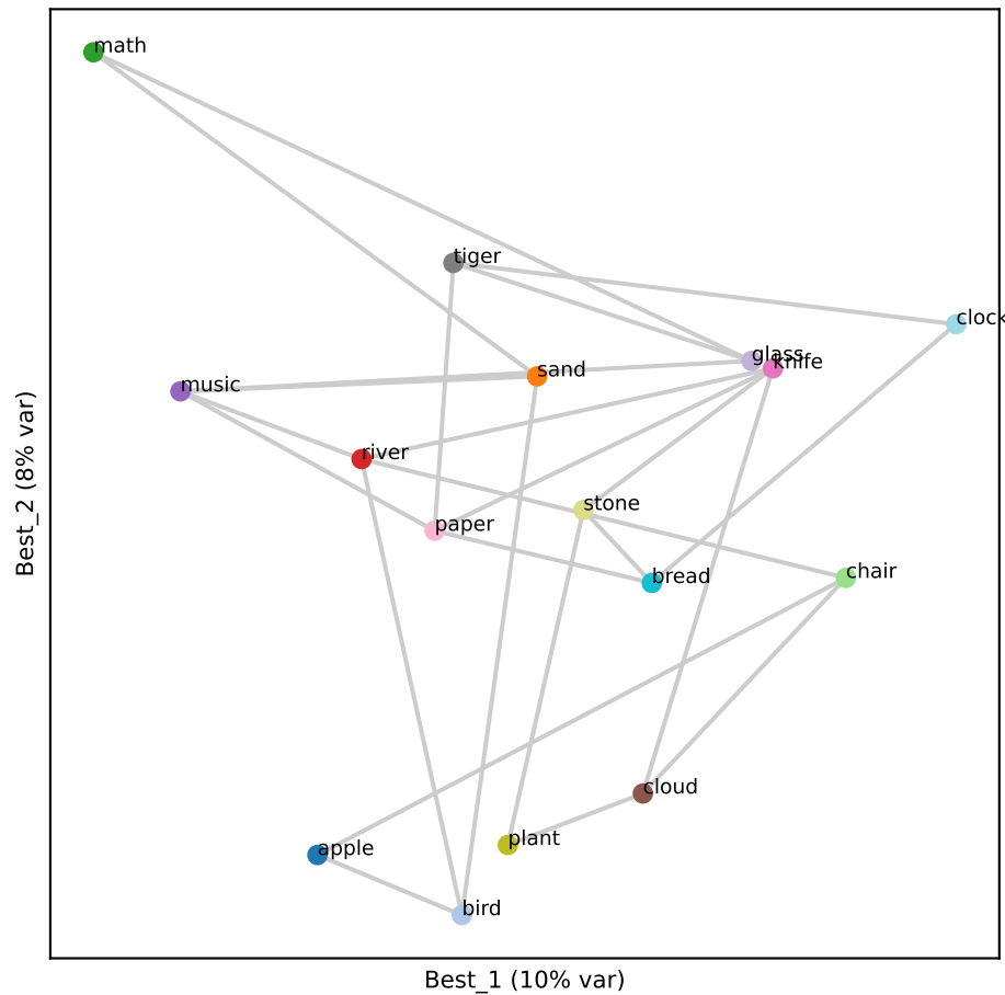
Gemma L8 (RSA 0.30)
