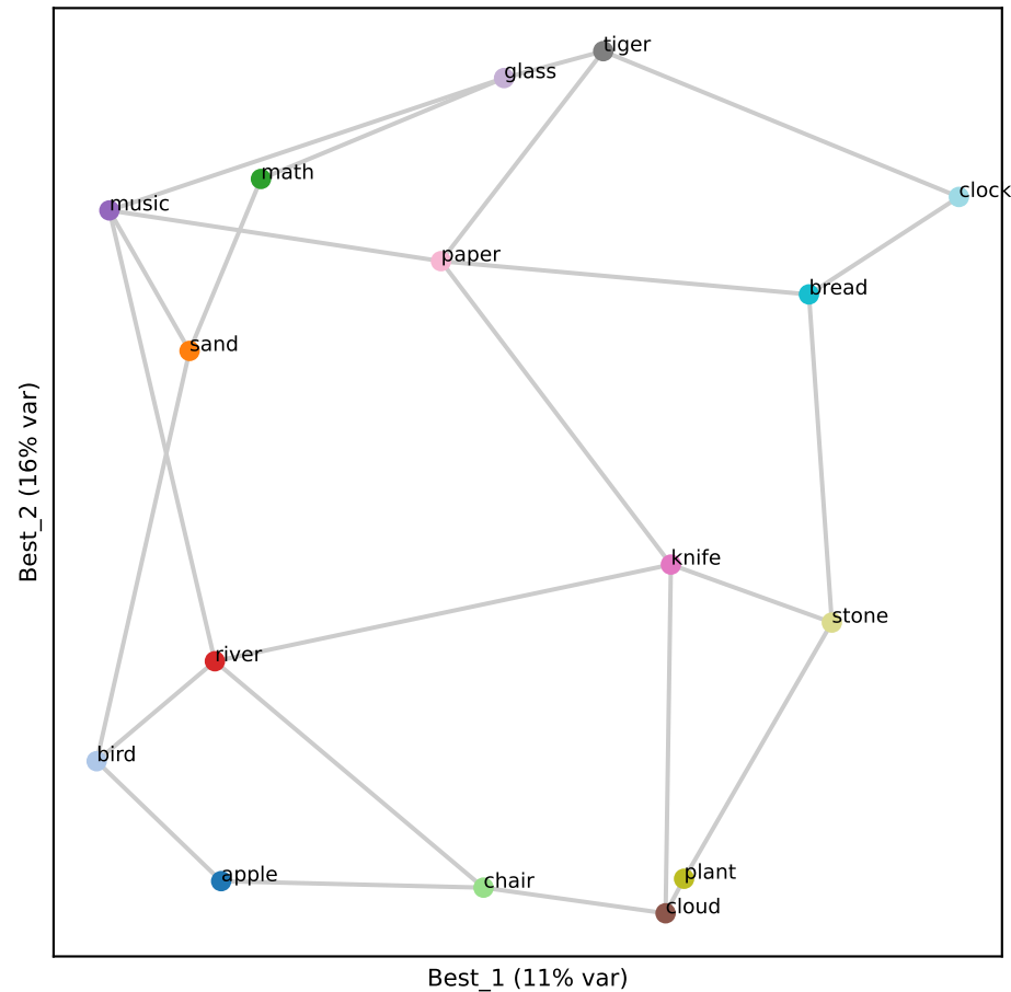
Gemma L25 (RSA 0.76)
