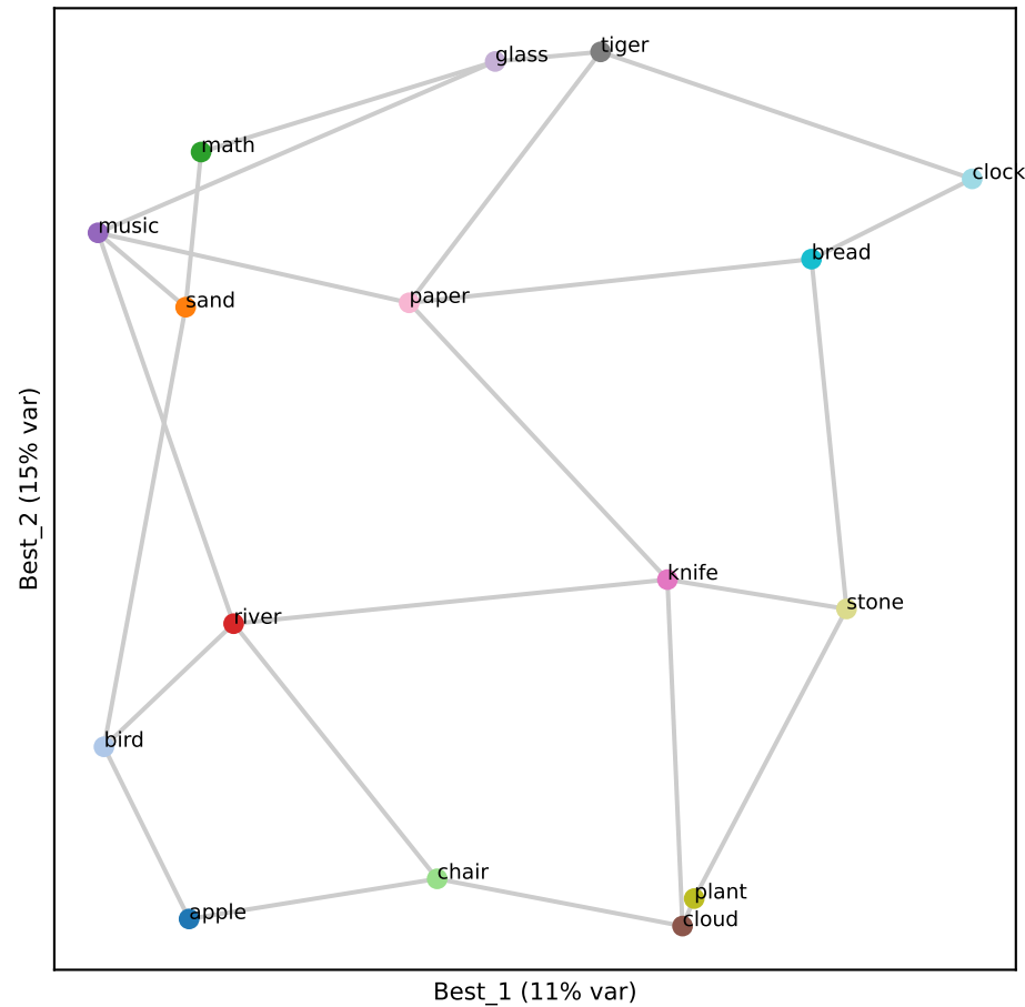
Gemma L23 (RSA 0.78)
