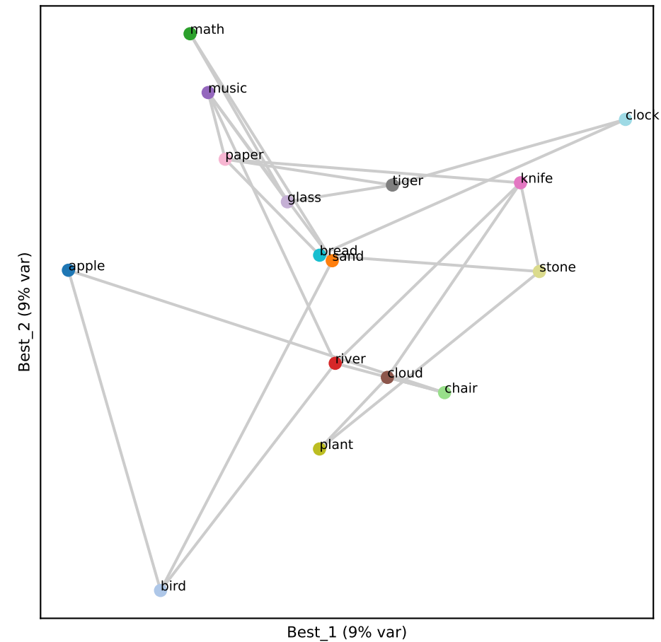
Qwen L16 (RSA 0.23)
