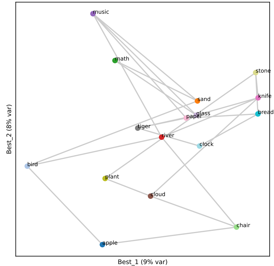
Qwen L4 (RSA 0.16)
