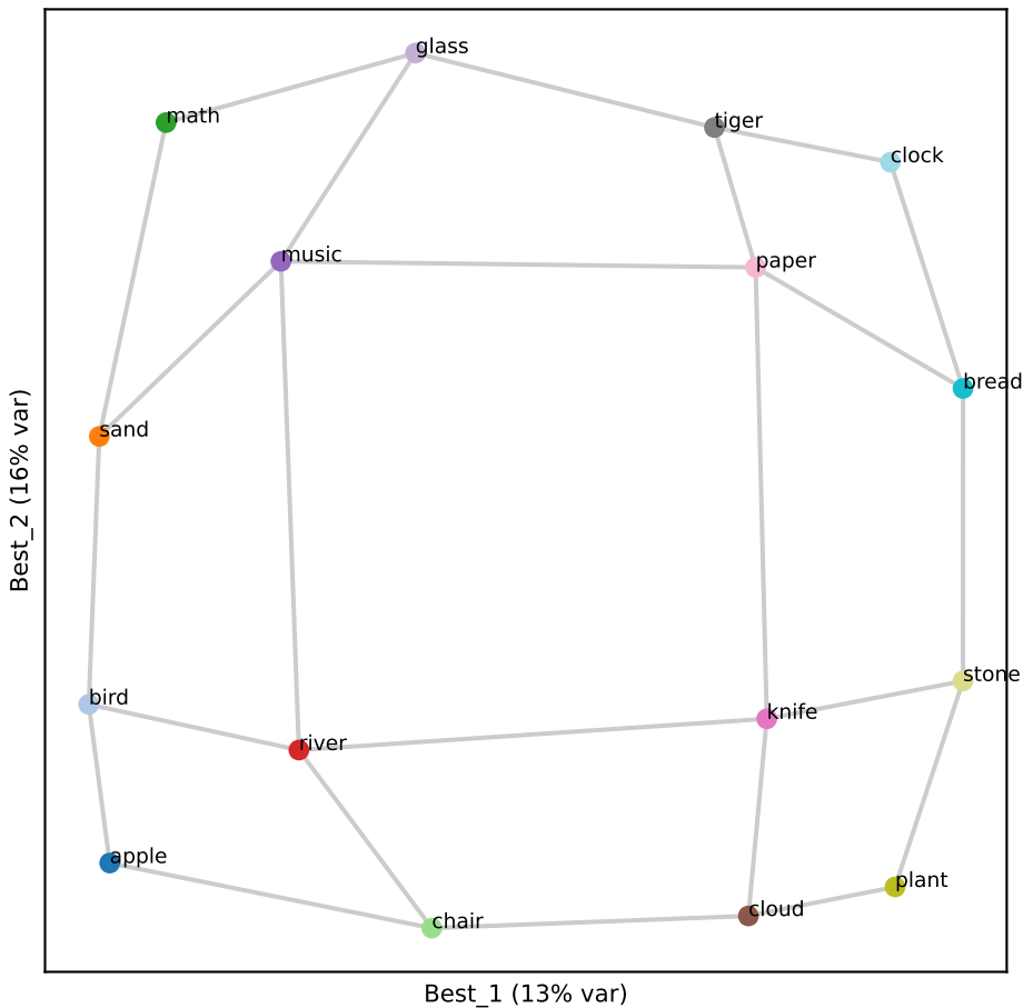
Llama L28 (RSA 0.87)
