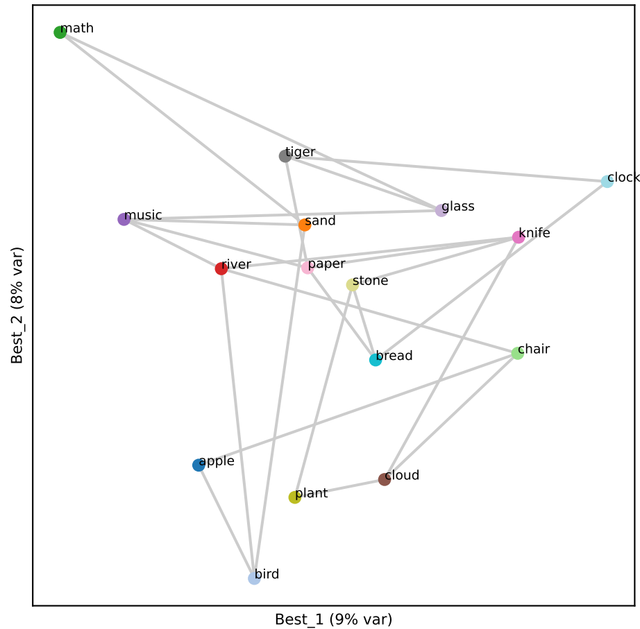
Gemma L6 (RSA 0.30)
