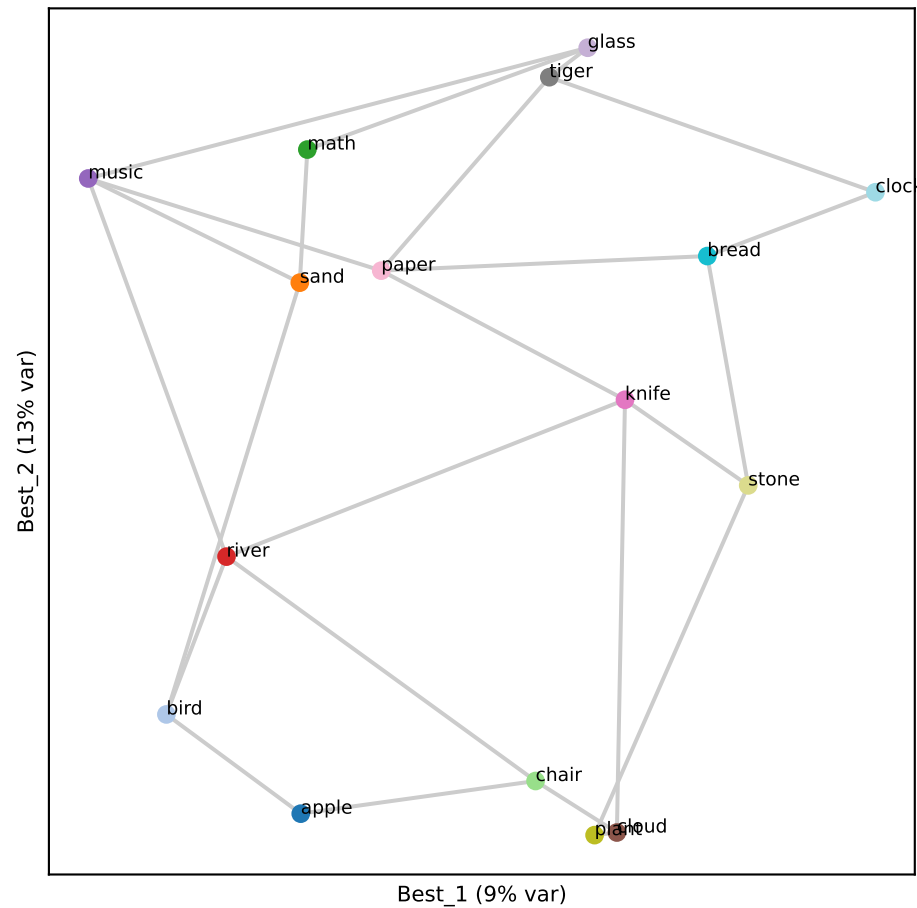
Gemma L19 (RSA 0.63)
