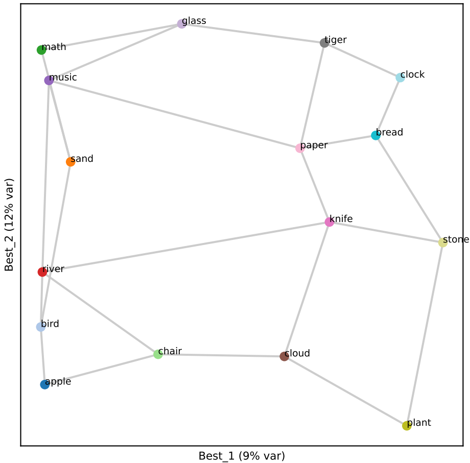
Llama L15 (RSA 0.80)
