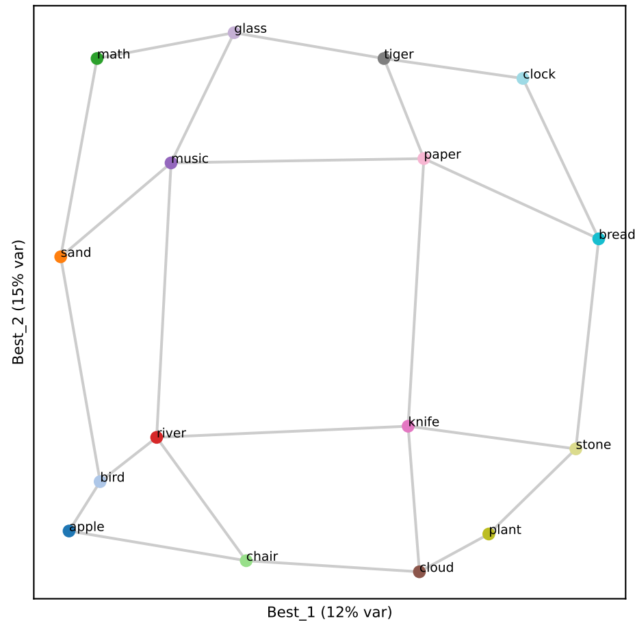
Gemma L35 (RSA 0.87)
