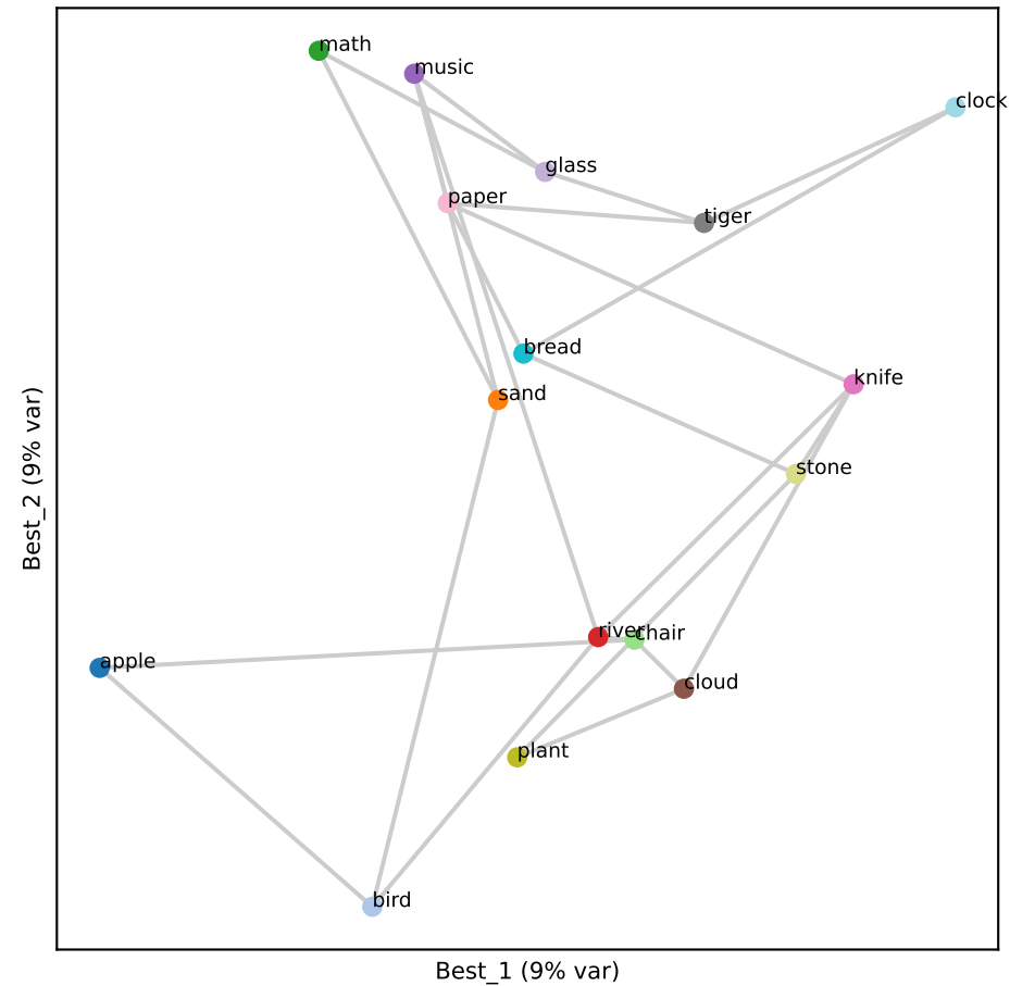
Qwen L20 (RSA 0.41)
