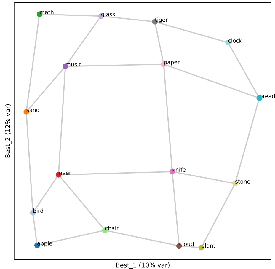
Gemma L33 (RSA 0.86)
