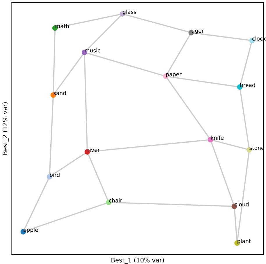
Llama L21 (RSA 0.82)
