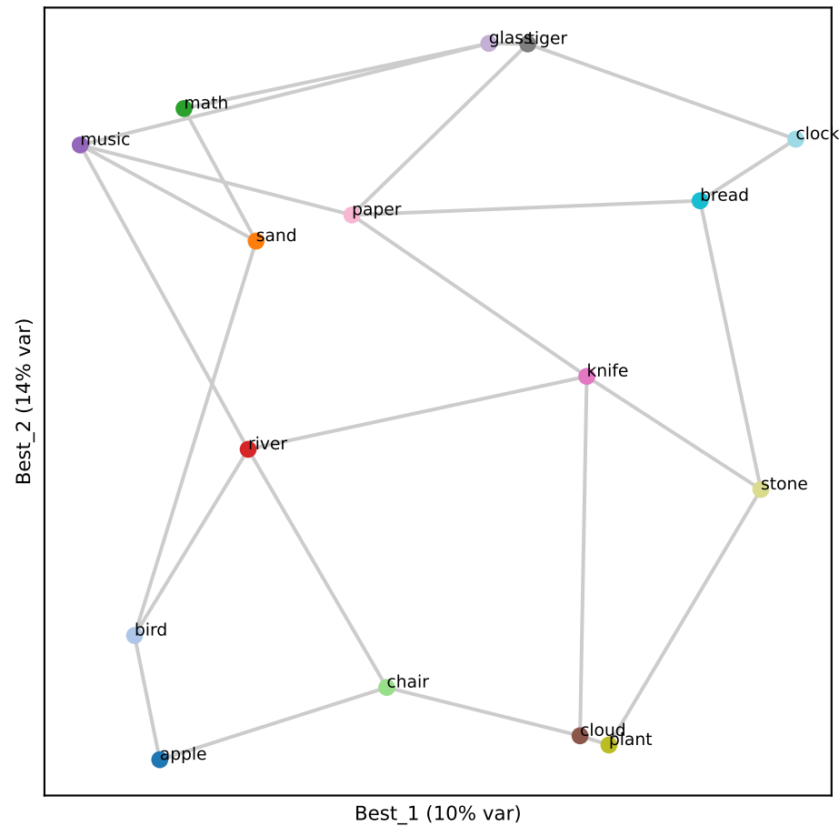
Gemma L18 (RSA 0.72)
