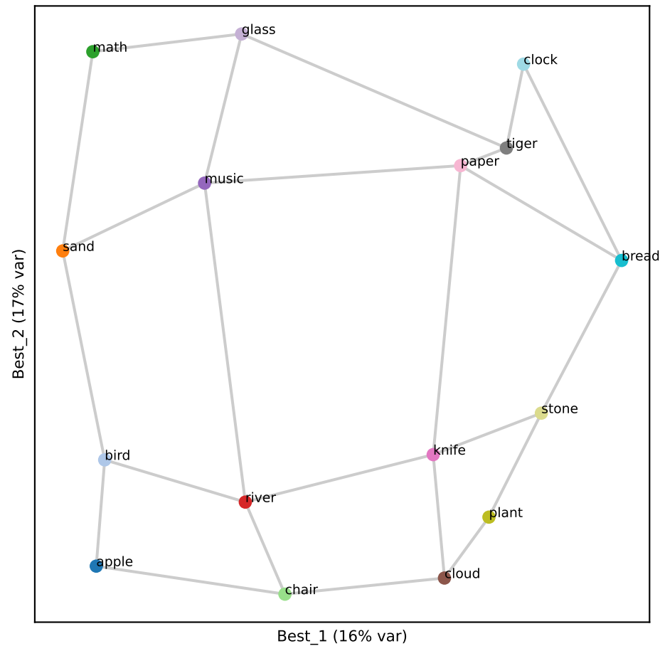
Gemma L41 (RSA 0.86)
