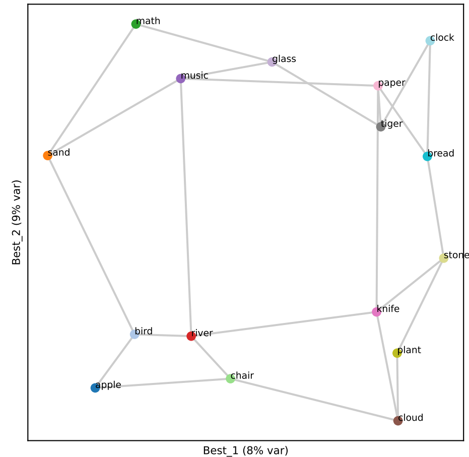
Qwen L30 (RSA 0.78)
