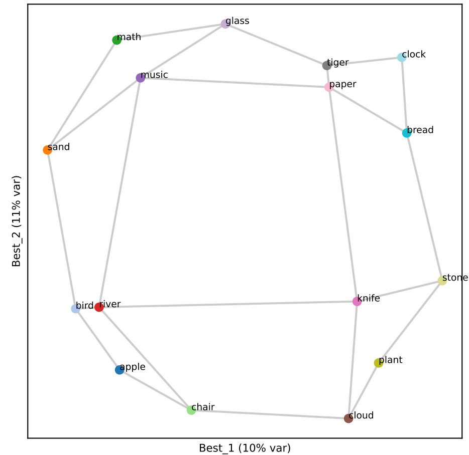
Qwen L33 (RSA 0.83)
