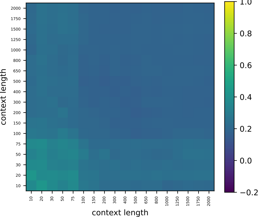
Llama L21 perm-null 95%
