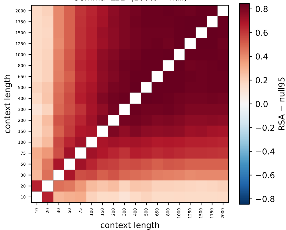
Gemma L21 (100% > null)
