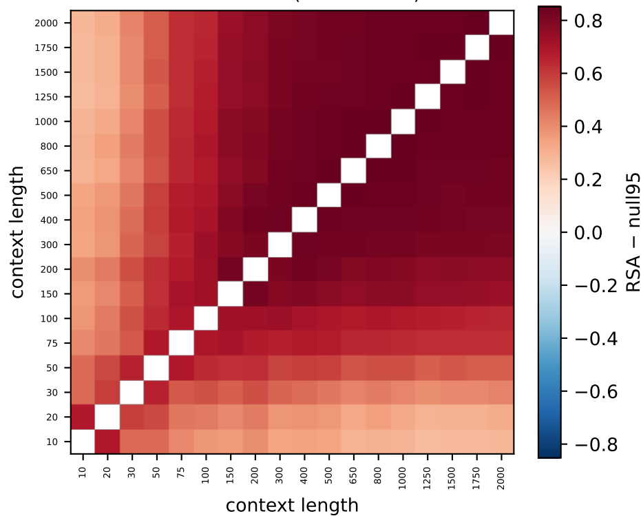
Gemma L24 (100% > null)
