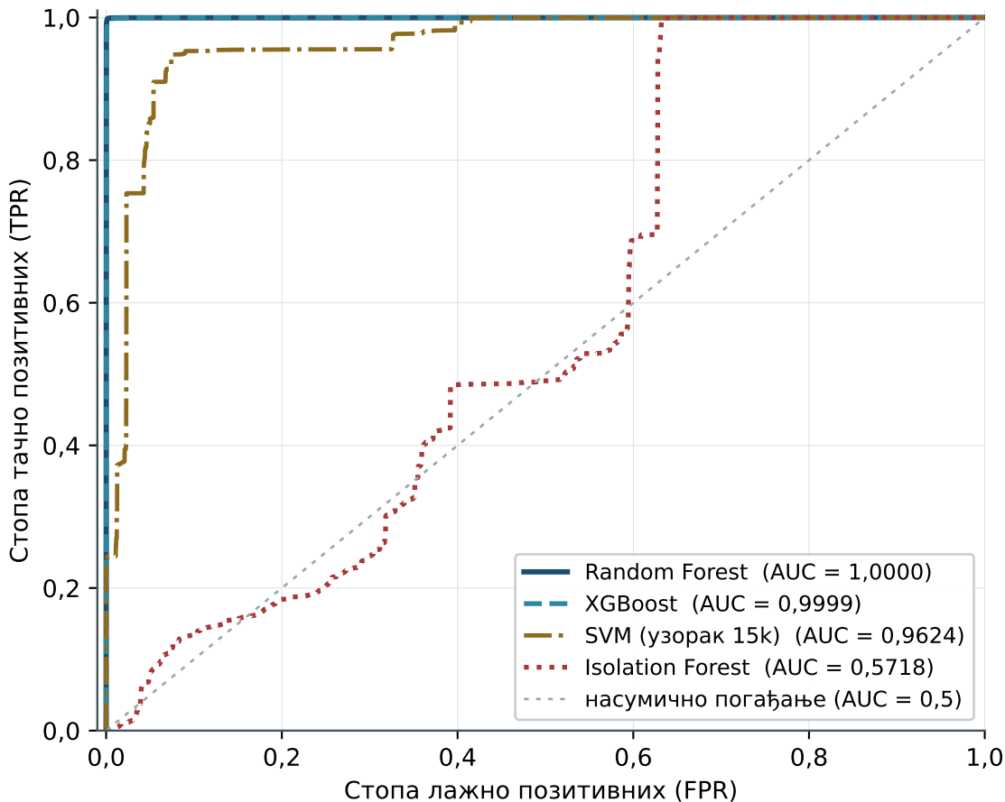
ROC криве примењених модела на тест скупу
