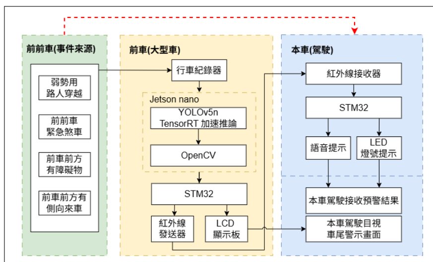
圖二：系統架構圖
