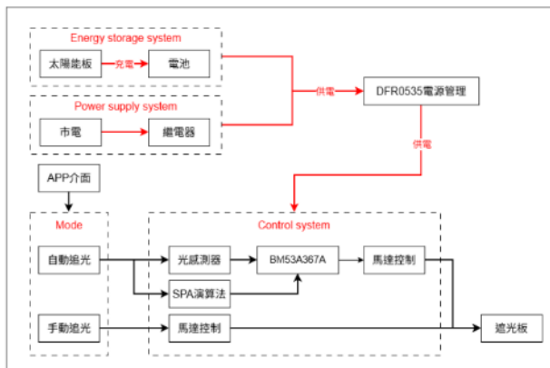
圖 1 系統架構圖
