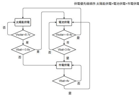
圖 9：供電切換邏輯流程圖
