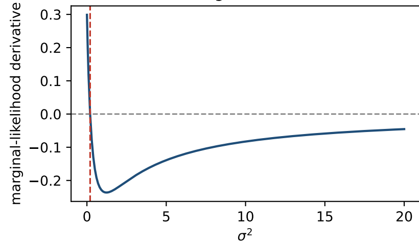
\sigma^2 tuning (root \approx 0.20 )
