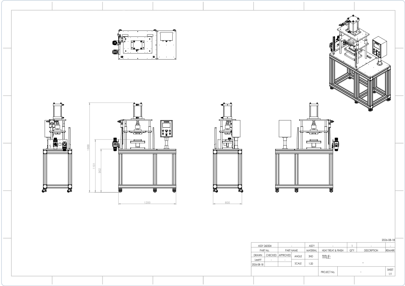
기구 도면 — 외형 치수(단위 mm), 축척 1:20
