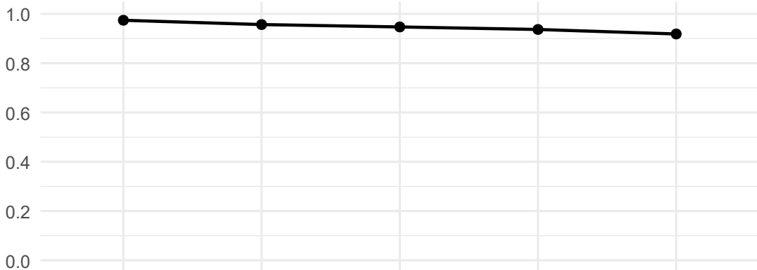
Sparse CCA
