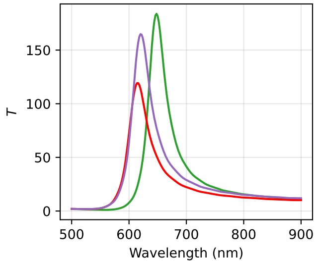
Mesh study: rod, longitudinal dipole, gap 5 nm
