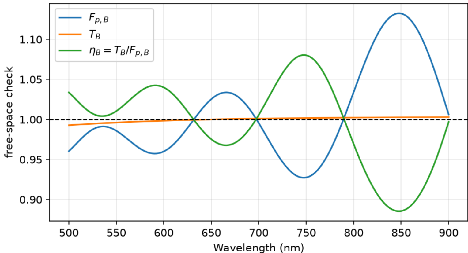
شکل 9. خروجی مرجع فضای آزاد F_{p,B} ، T_B و \eta_B . خط چین مقدار ایده آل یک را نشان می‌دهد. نوسان منظم F_{p,B} با بازتاب ضعیف از PML یا درونیابی منبع سازگار است و \eta_B > 1 در 748 \text{ nm} غیرفیزیکی بودن آن را آشکار می‌کند.
