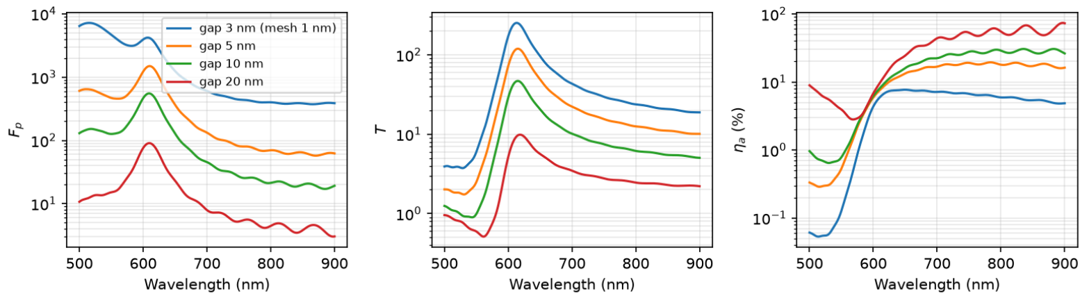
شکل 5. پویش گاف برای نانومیل با دوقطبی طولی: F_p (چپ)، T (وسط) و \eta_a (راست) در گاف‌های 3 (مش 1 nm)، 5، 10 و 20 nm.
