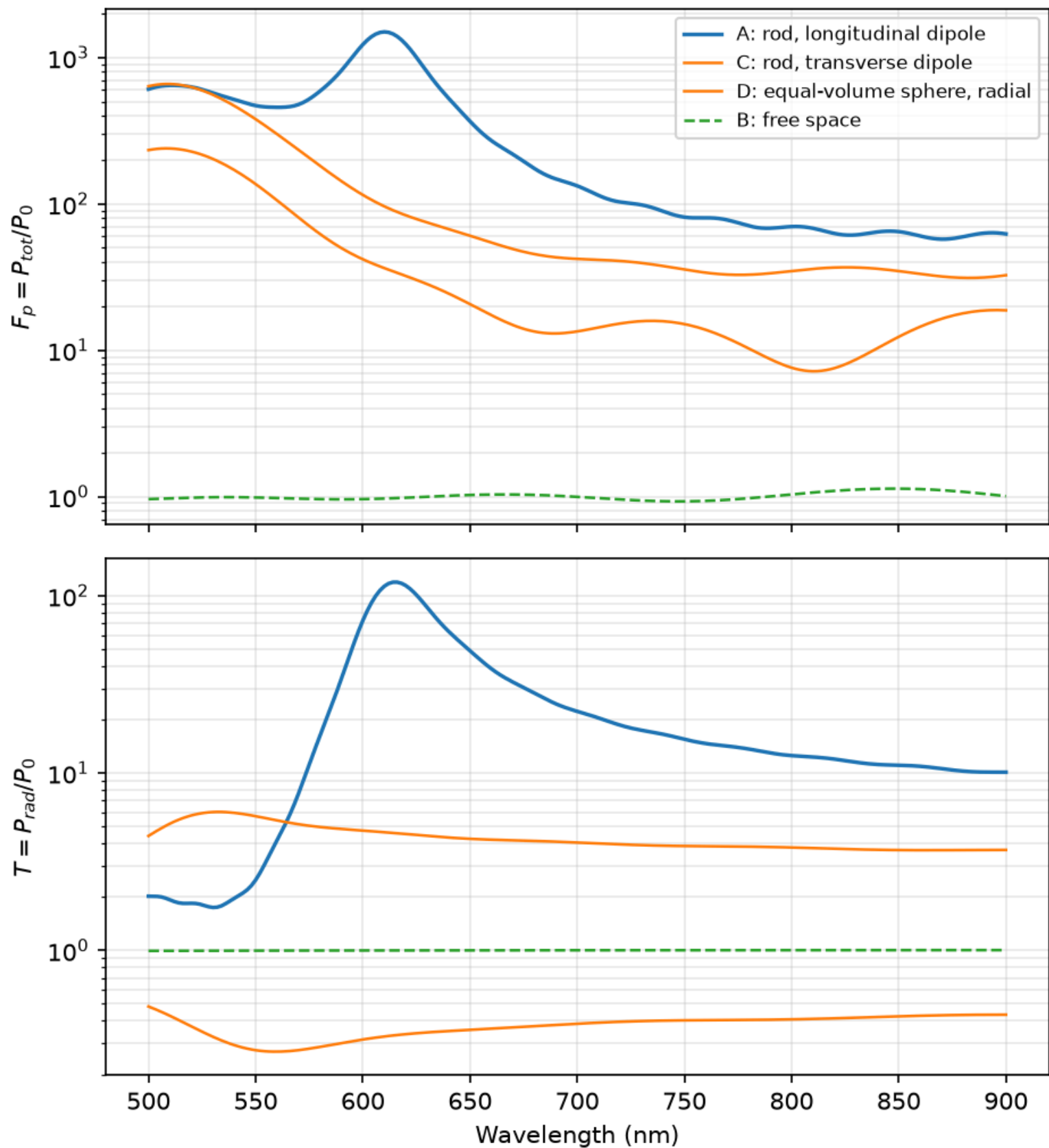
شکل 2. فاکتور پورسل (بالا) و تقویت توان تابشی (پایین) حالت‌های A (نانومیله، طولی)، C (نانومیله، عرضی)، D (کره‌ی هم‌حجم، شعاعی) و مرجع فضای آزاد B، همه با تعریف خام و محور لگاریتمی، مستقیماً از فایل‌های ۲۰۱ نقطه‌ای.
