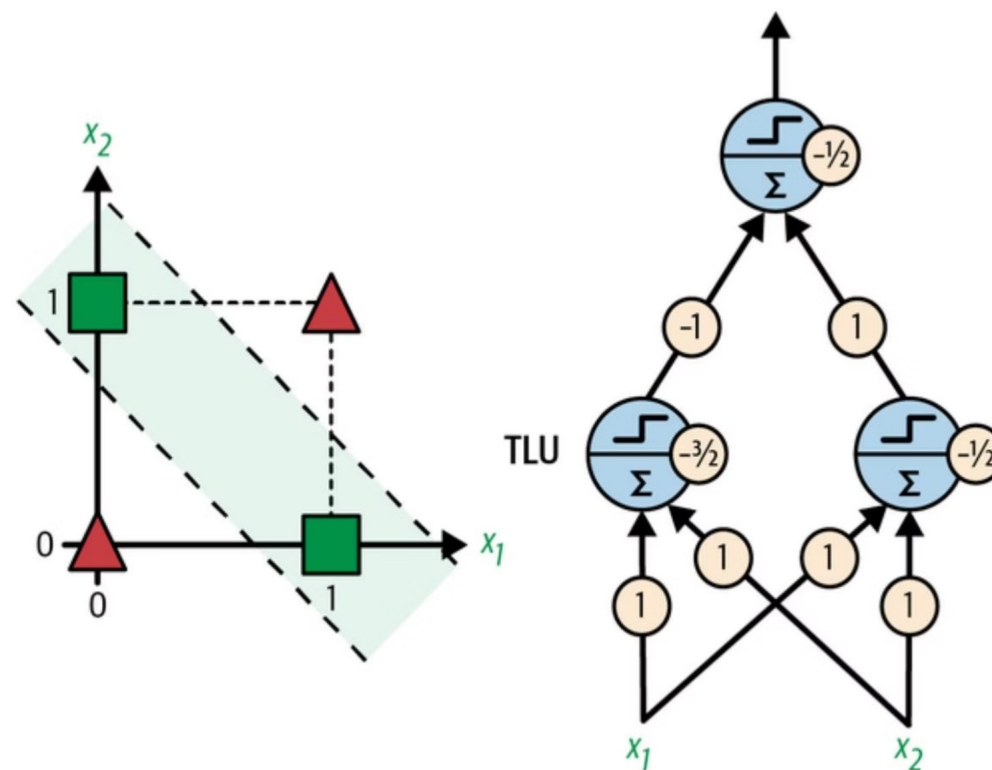
그림 10-6. XOR 분류 문제와 이를 해결하는 MLP
