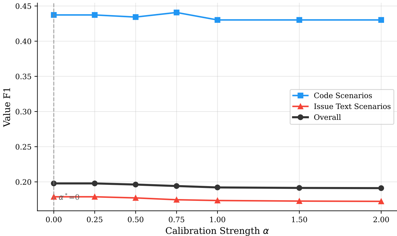
Bayesian Calibration: Value F1 vs \alpha (qwen-plus)
