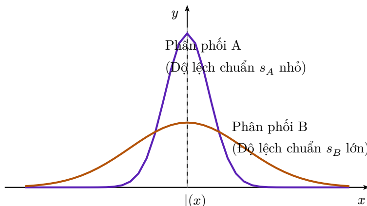
Hình 2. So sánh hai phân bố tần suất có cùng giá trị trung bình mẫu |(\bar{x})| nhưng độ lệch chuẩn khác nhau ( s_A < s_B )
