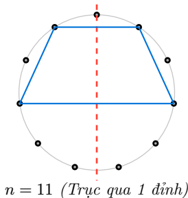
n = 11 (Trục qua 1 đỉnh)
