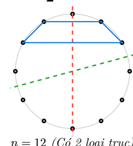
n = 12 (Có 2 loại trục)
