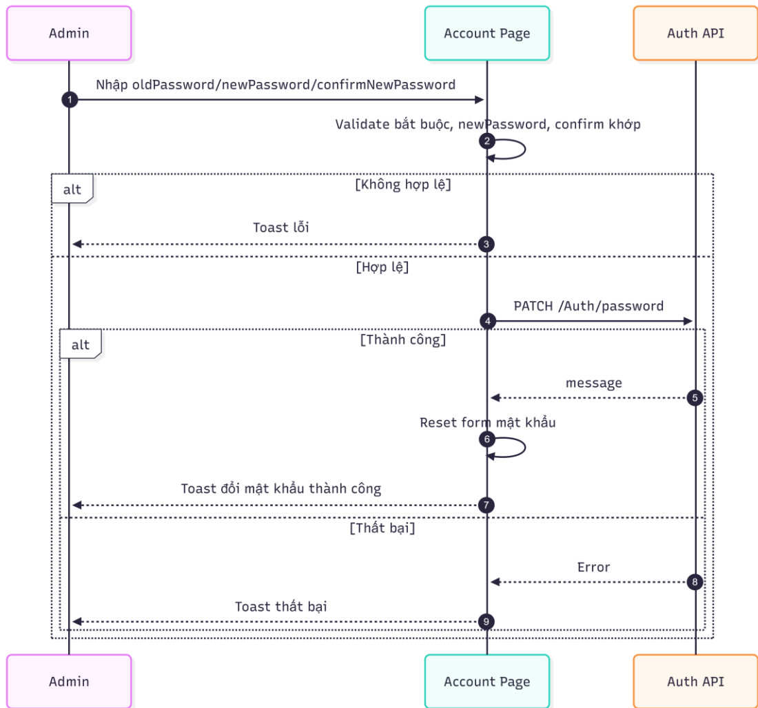
22_DoiMatKhauMoTaiKhoan.png
