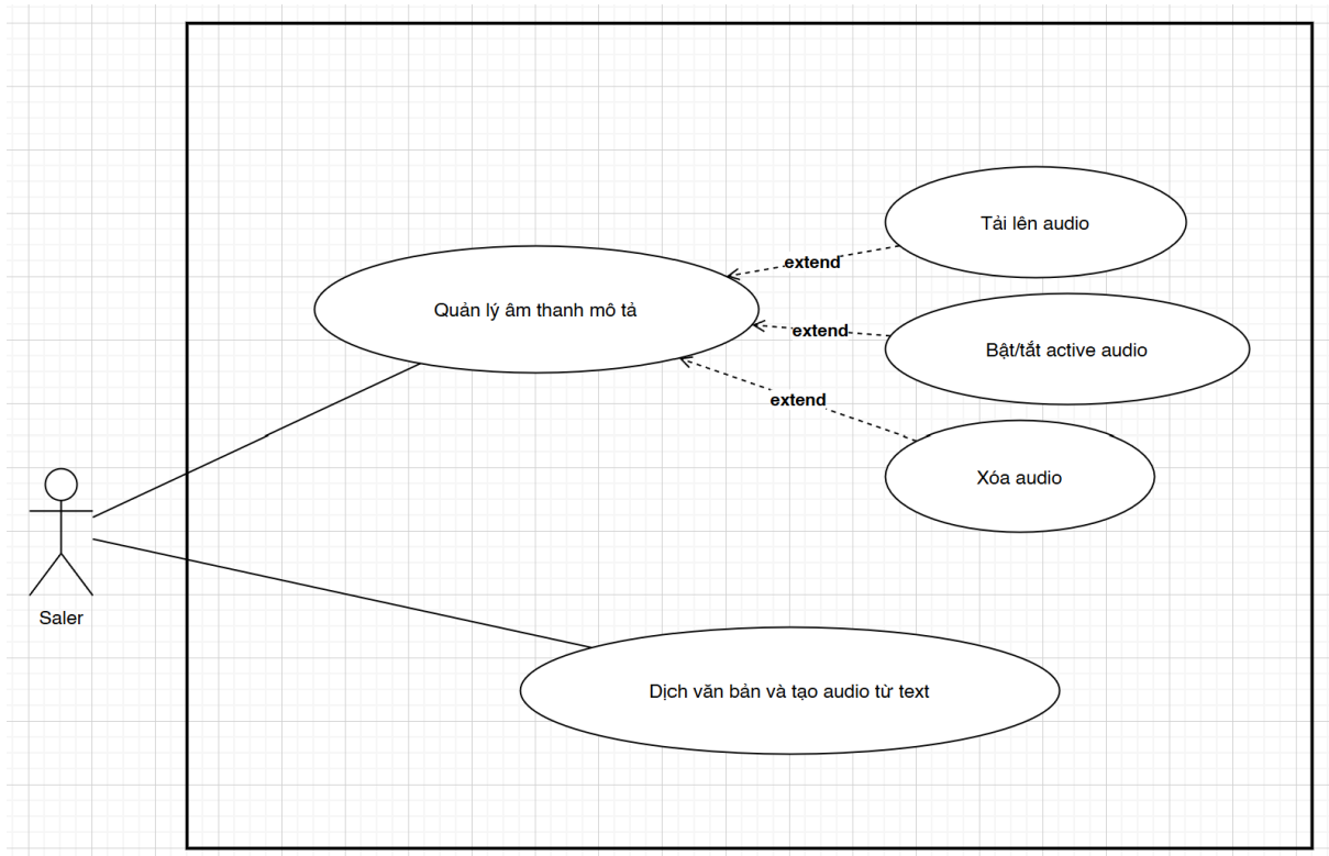
AmThanh.png
