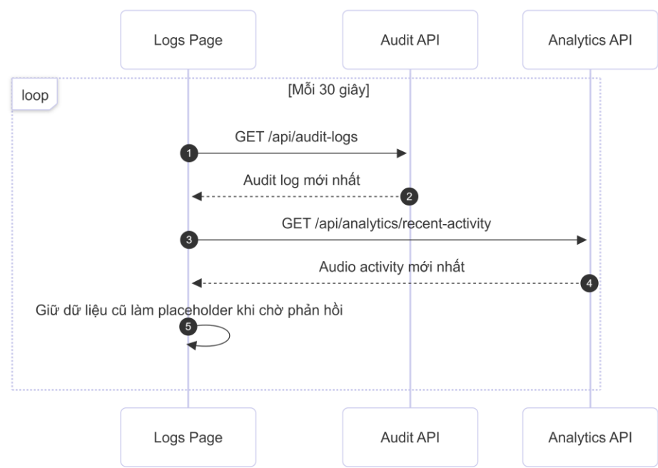
16_TuDongCapNhat.png
