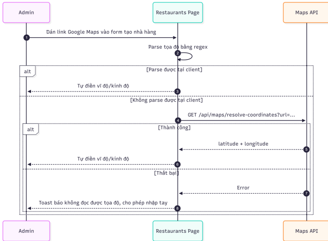
10a_DienToaDoaGGMMap.png
