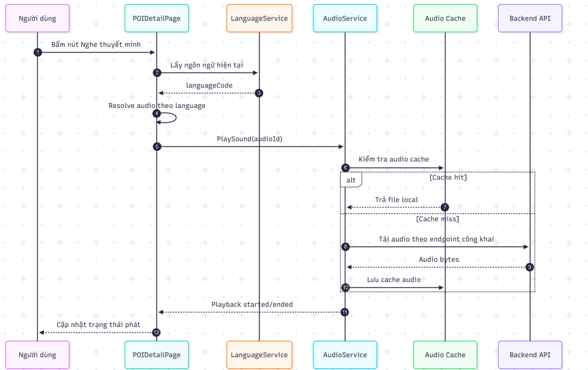
ChiaSePOL.png
