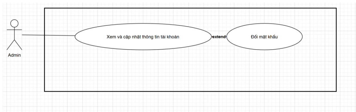
TaiKhoan.png
