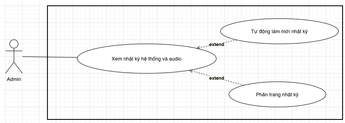
NhatKiHeThong.png
