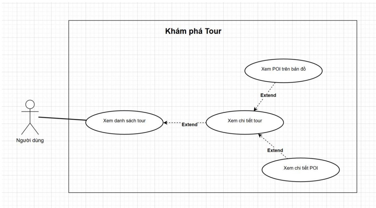
KhamPhaTour.png
