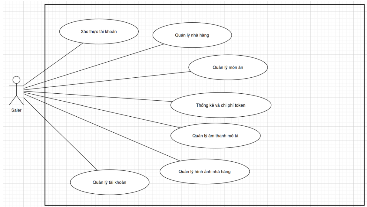
TongQuat.png
