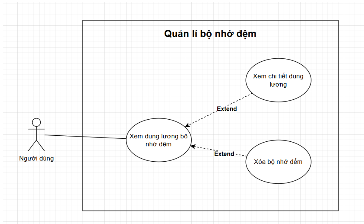
QuanLiBoNhoDem.png
