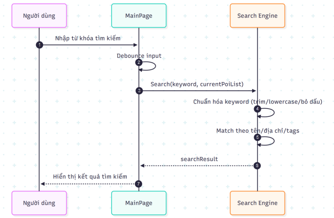
LocPOL.png
