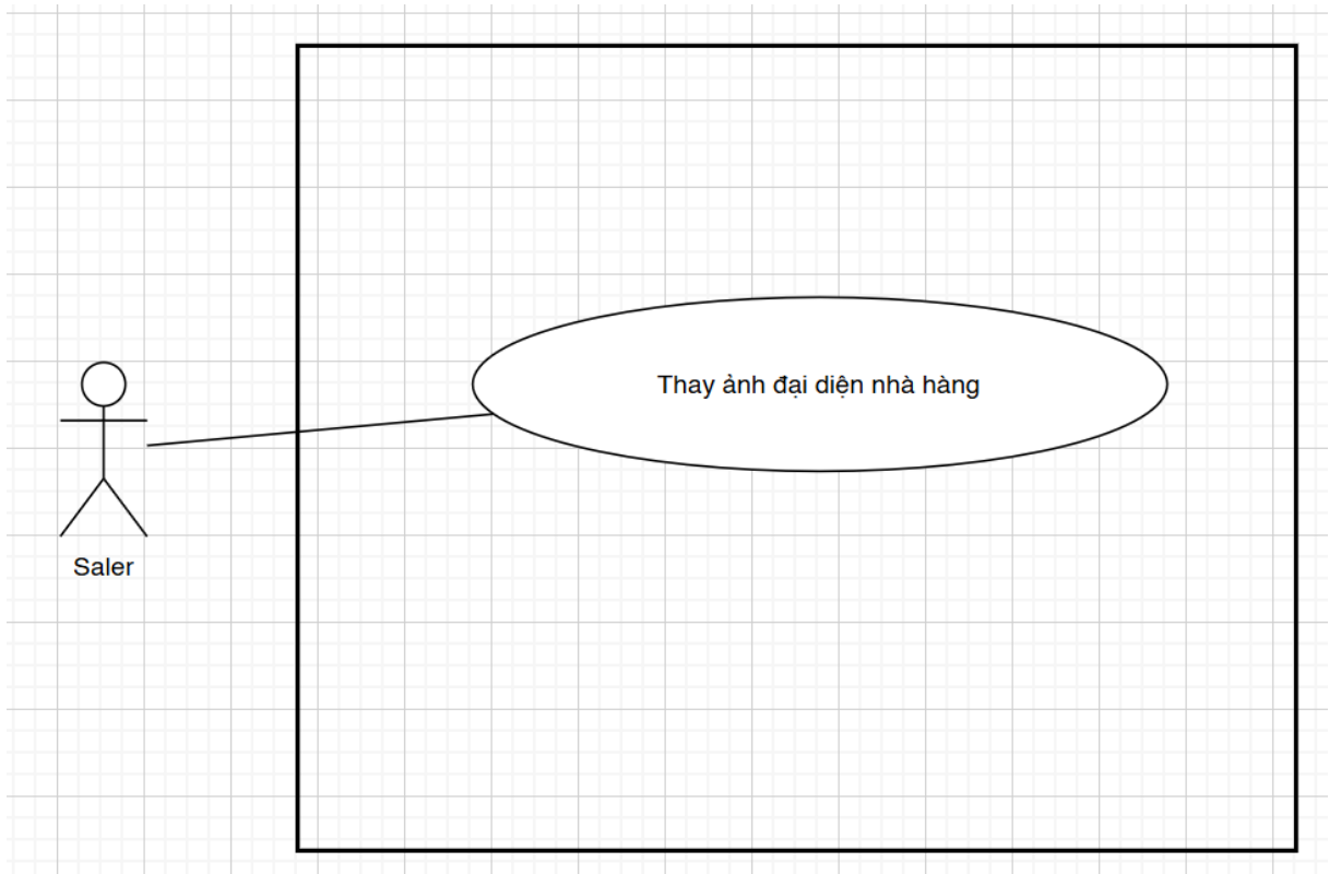
AnhDaiDien.png
