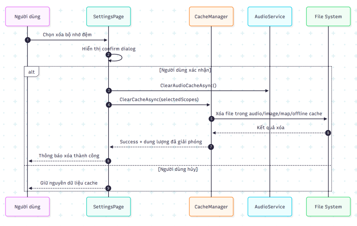
XoaBoNhoDem.png
