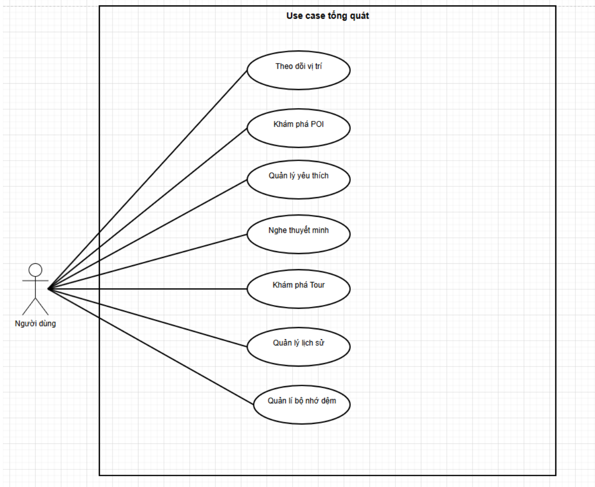
TongQuat.png
