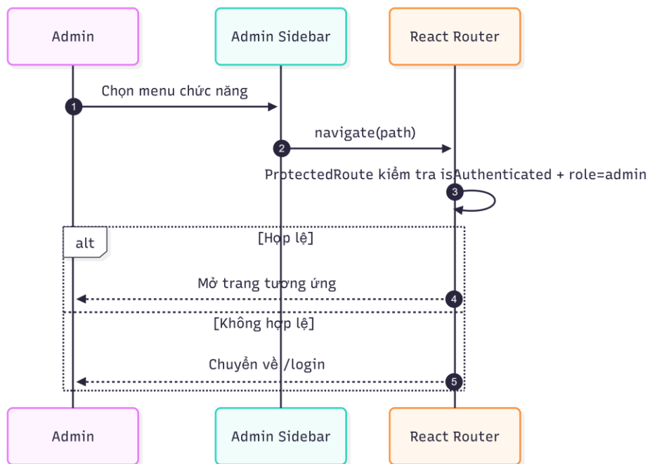
1_KiemTraDangNhap.png
