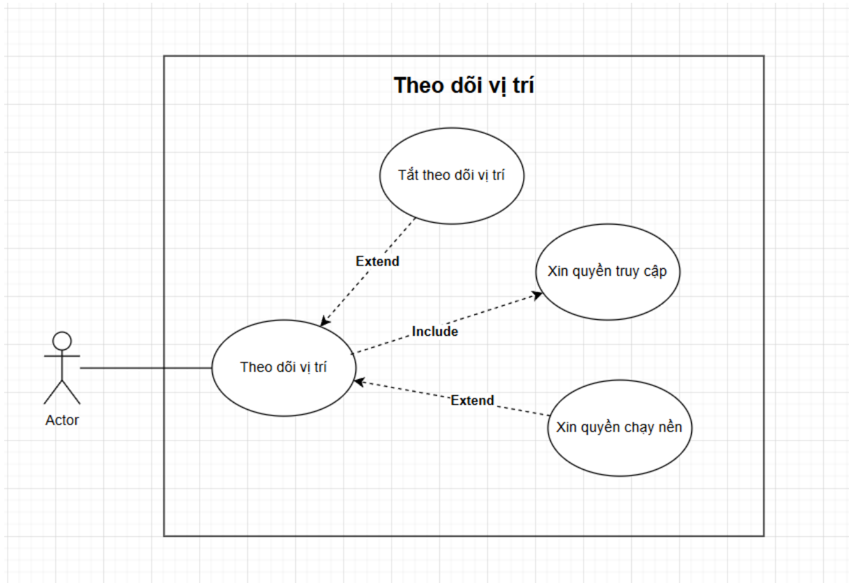
TheoDoiViTri.png
