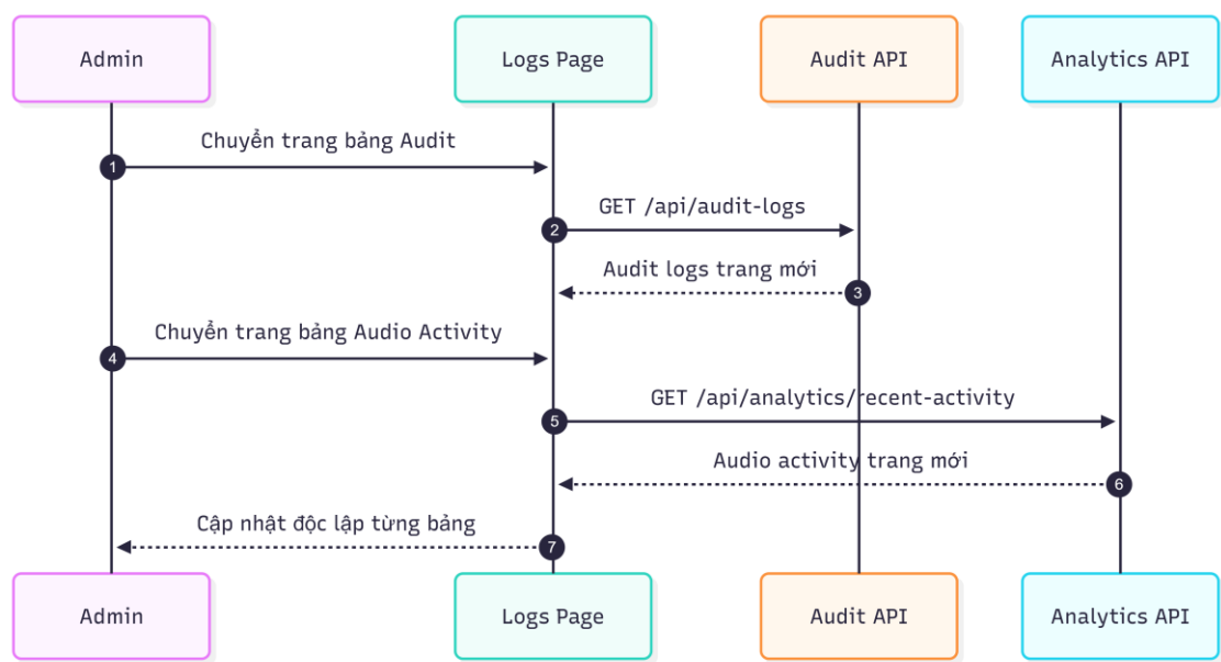
16_TuDongCapNhat.png
