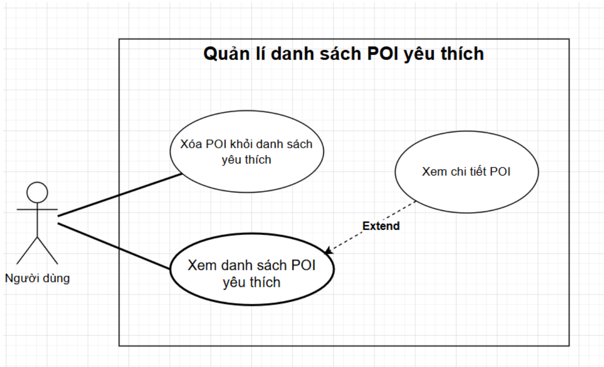
QuanLiDanhSachYeuThich.png
