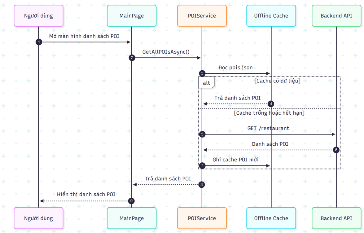
TimKiemPOi.png
