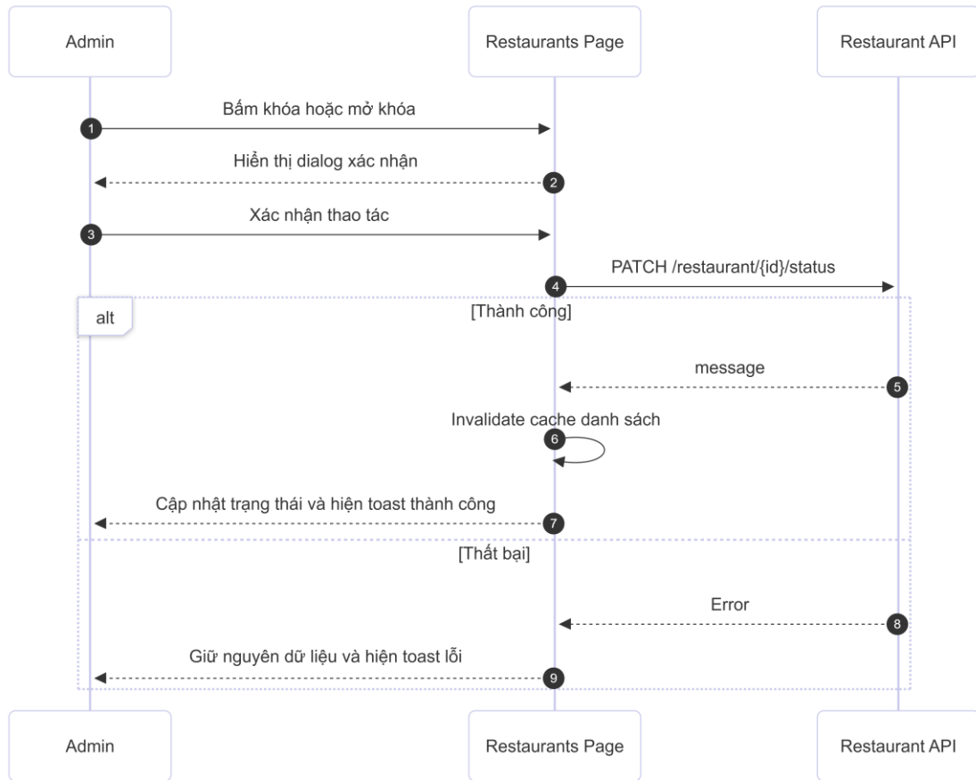
11_KhoaNhaHang.png
