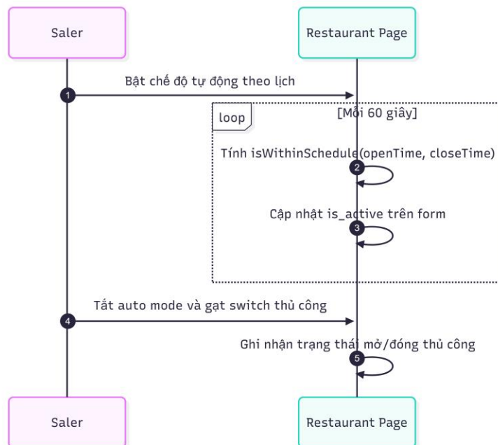
8_CapNhatThongTinNhaHang.png
