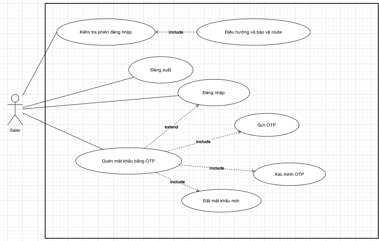
XacThuc.png
