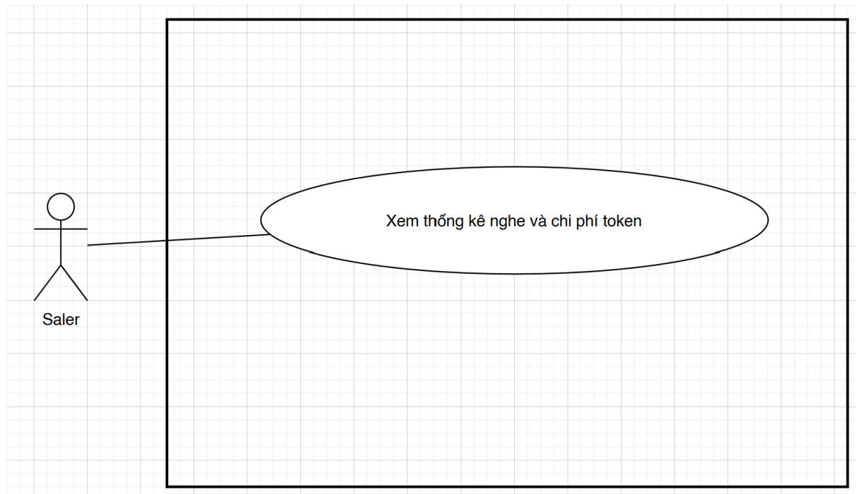
ThongKe.png
