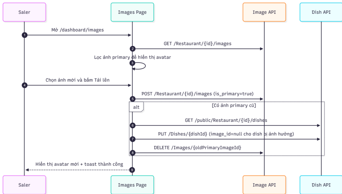
15_ThayAnhDaiDienNhaHang.png
