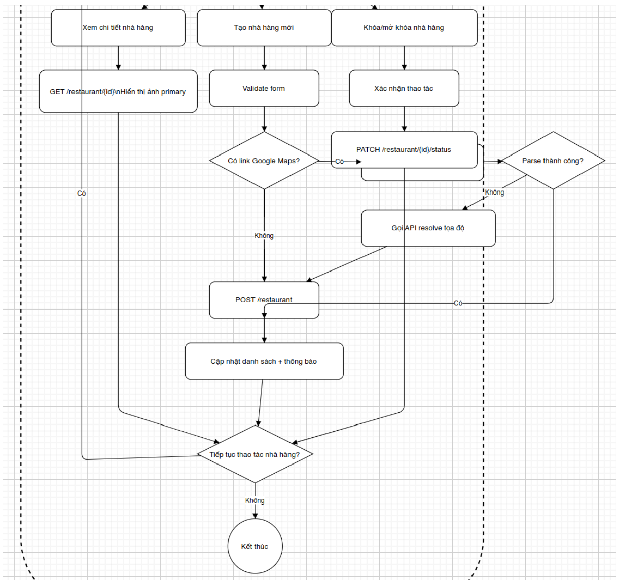
2.png
