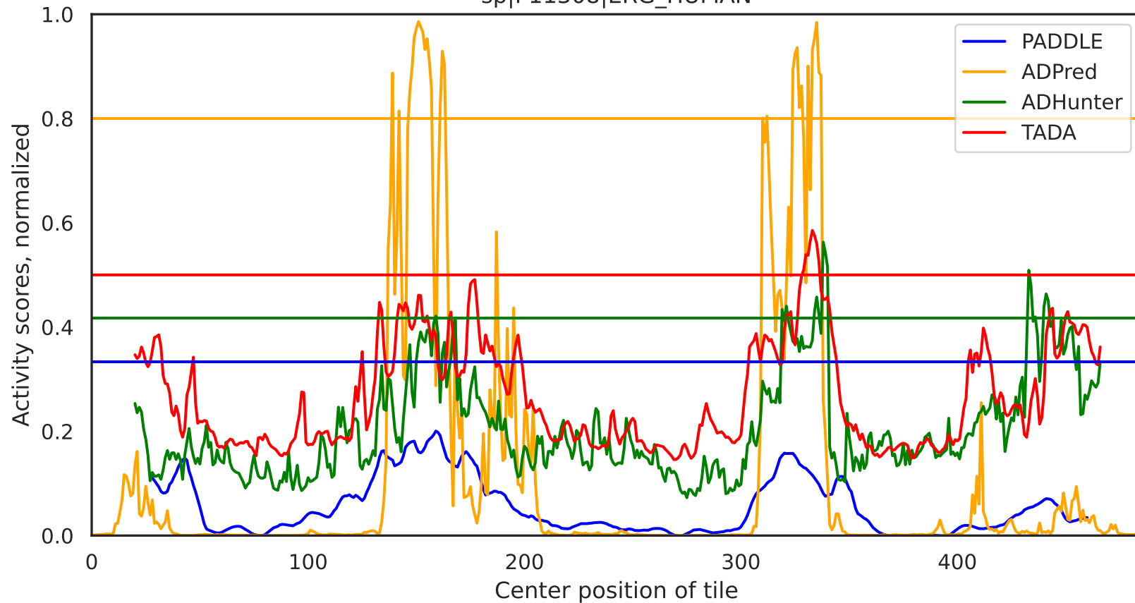
sp|P11308|ERG_HUMAN
