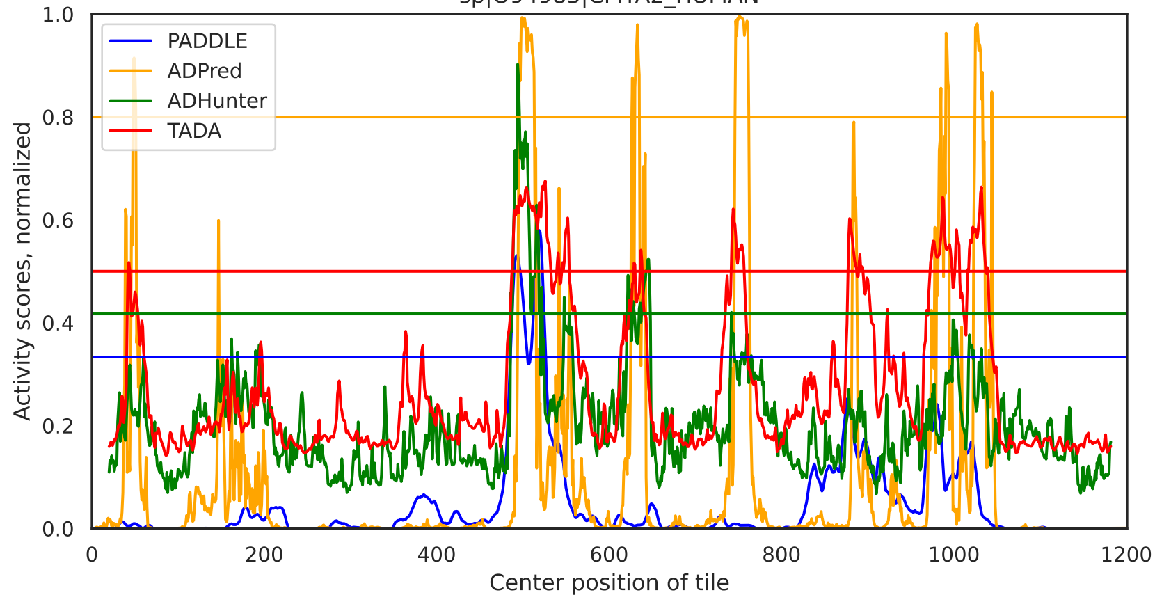
sp|O94983|CMTA2_HUMAN
