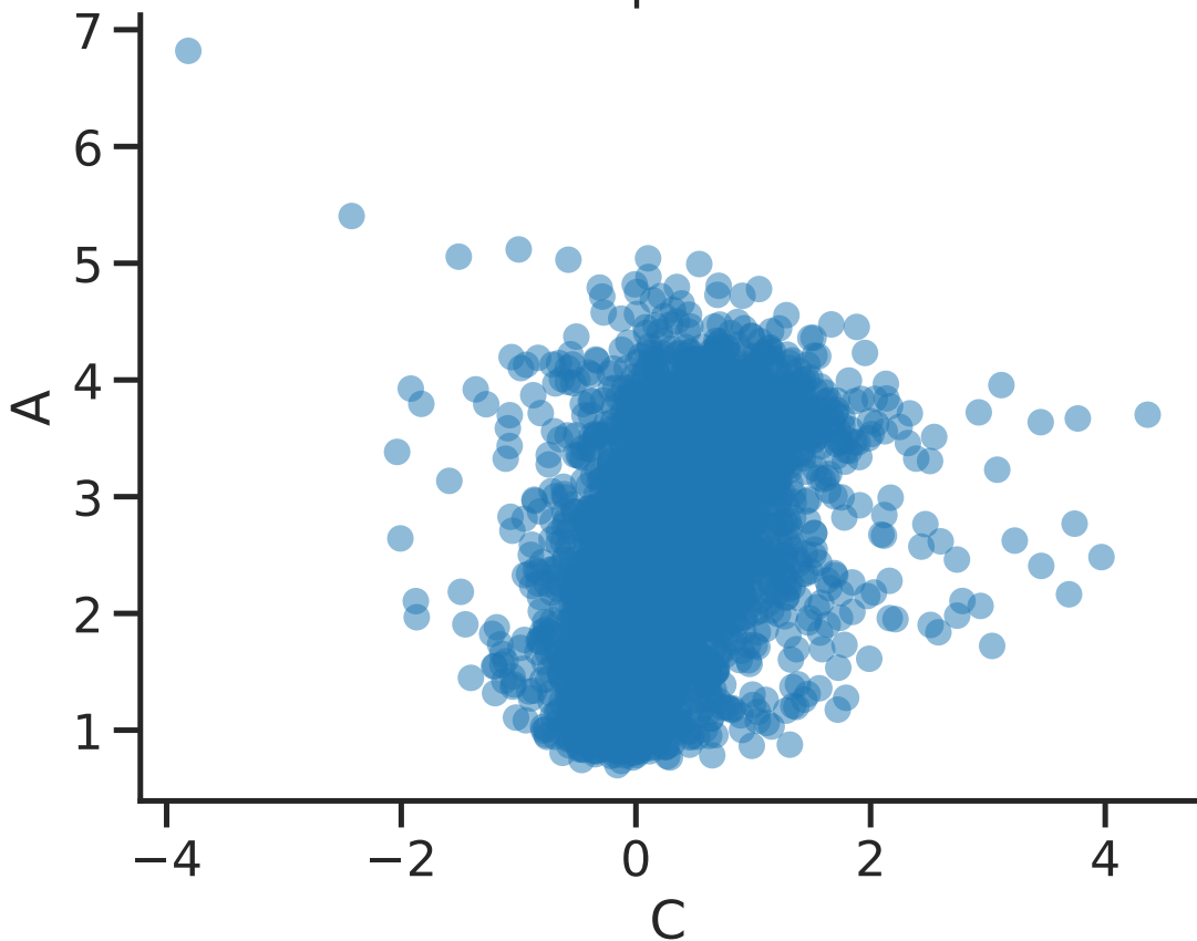
GCN4: Exponential Fit
